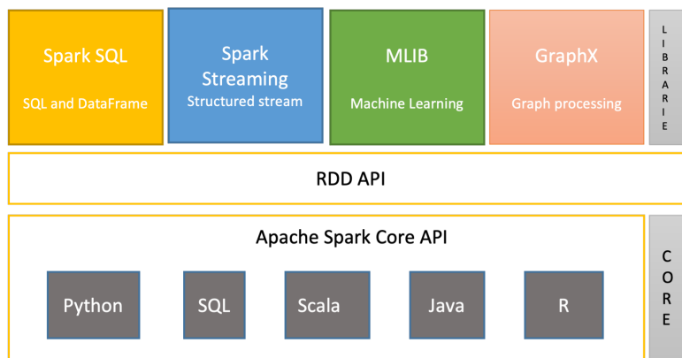
FIGURE 6.3 – Écosystème de Apache Spark.
