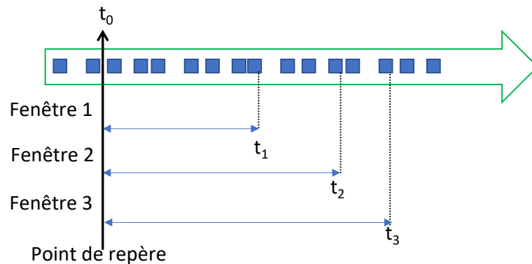
FIGURE 4.2 – Fenêtre physique point de repère.
