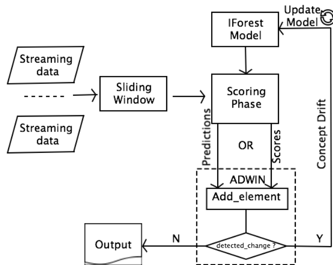
FIGURE 5.3 – Workflow de la méthode IForest ASD basée sur ADWIN : PADWIN IFA si les prédictions sont utilisées, SADWIN IFA si les scores sont considérés. Figure inspirée de DING et FEI (2013).
