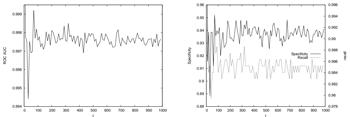
FIGURE 3.7 – Performances de IForest pour différents nombres d'arbres ( t ).
