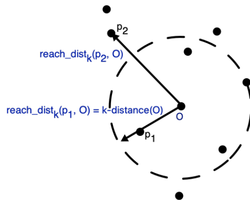
FIGURE 2.2 – reach\_dist_k(p_1, O) et reach\_dist_k(p_2, O) pour k = 5 .
