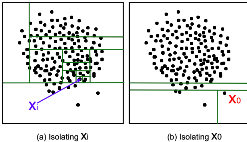
FIGURE 2.4 – Les données anormales ( X_0 ) sont plus rapidement isolées que les données normales ( X_i ).
