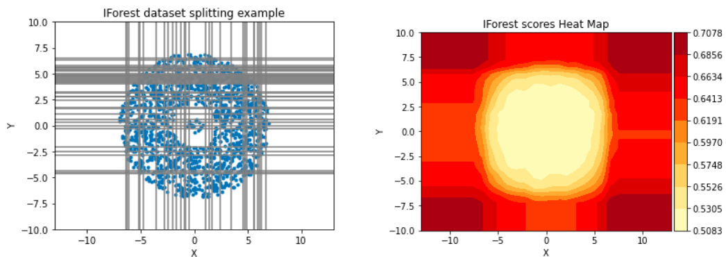
FIGURE 3.1 – Exemple de scissions des noeuds par IForest avec sa heat map basée sur les scores associés : présence de zones sombres artificielles. X et Y sont les coordonnées des données.
