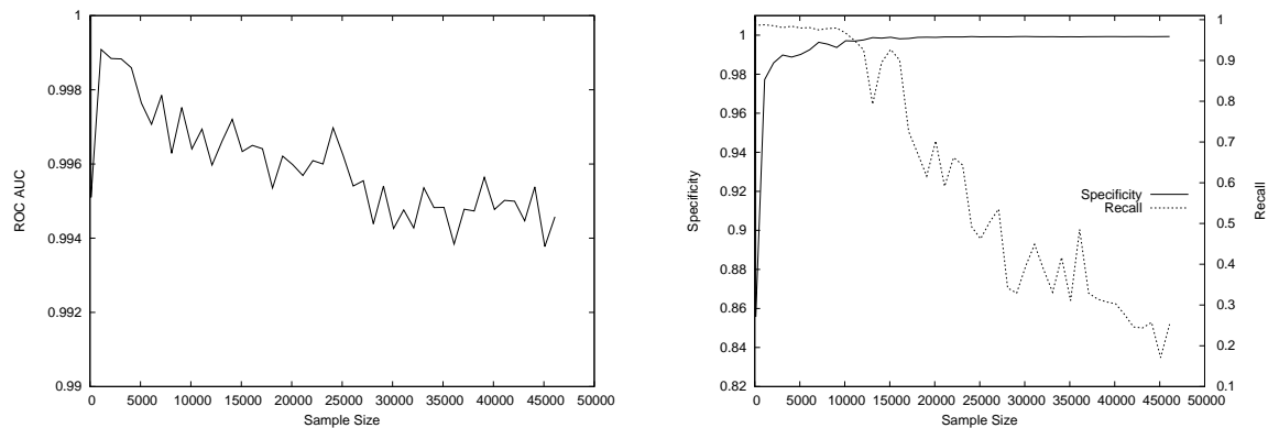
FIGURE 3.5 – Performances de IForest avec différentes tailles d'échantillon ( \psi ).
