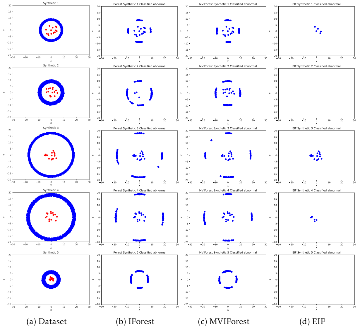
FIGURE 3.12 – Données classées anormales par IForest, EIF et MVIForest respectivement dans les jeux de données Synthetic_1, Synthetic_2, Synthetic_3, Synthetic_4 and Synthetic_5 .
