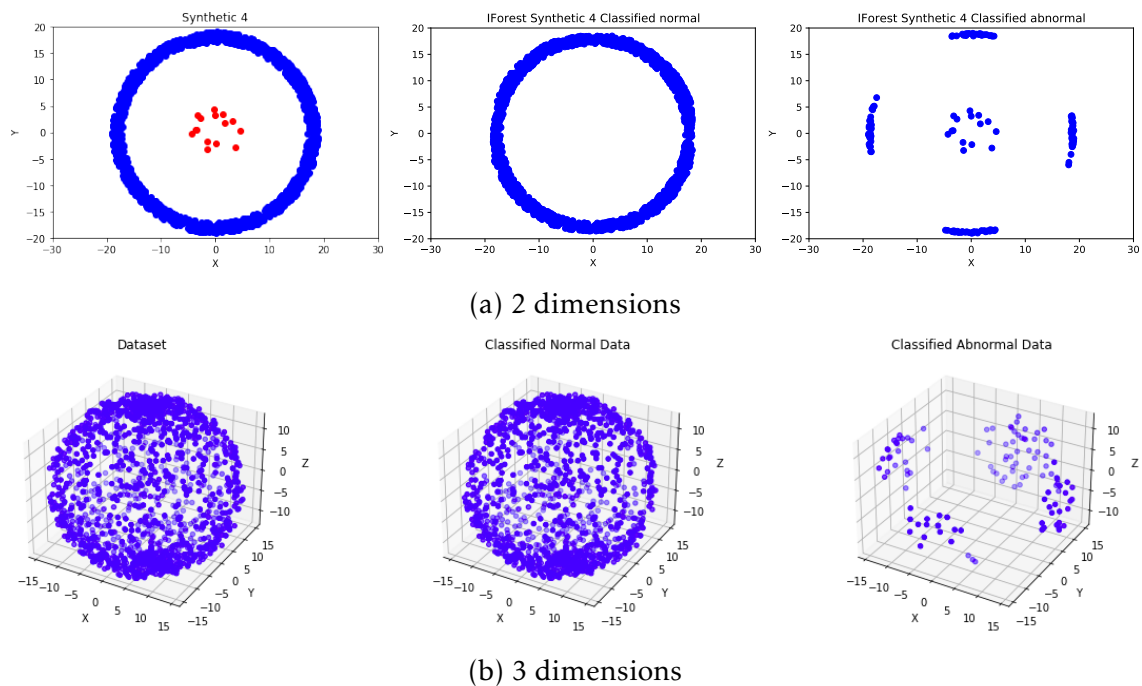
FIGURE 3.9 – Résultats de l'exécution de IForest sur des jeux de données de 2 et 3 dimensions.
