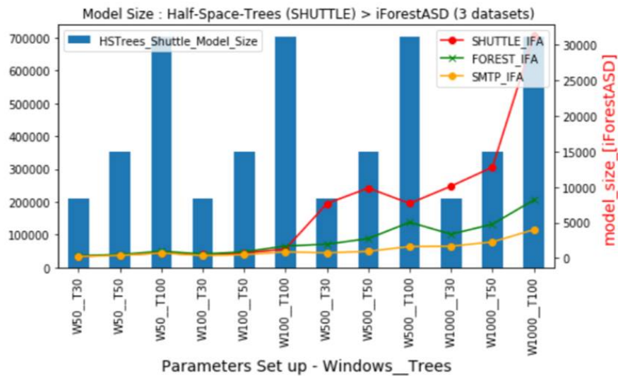
FIGURE 4.6 – Mesure de la taille du modèle (Kilo-octets) : Nous avons fixé la taille de la fenêtre (50, 100, 500, 100) et varié le nombre d’arbres (30, 50, 100). Pour chaque paramètre, nous avons exécuté HSTrees (barplot - axe Y à gauche) avec Shuttle et IForest ASD (Lignes - axe Y à droite) pour chaque jeu de données - 36 mesures - et avons tracé les lignes (Axe Y à droite). HST est \approx 20x plus grand que IFA
