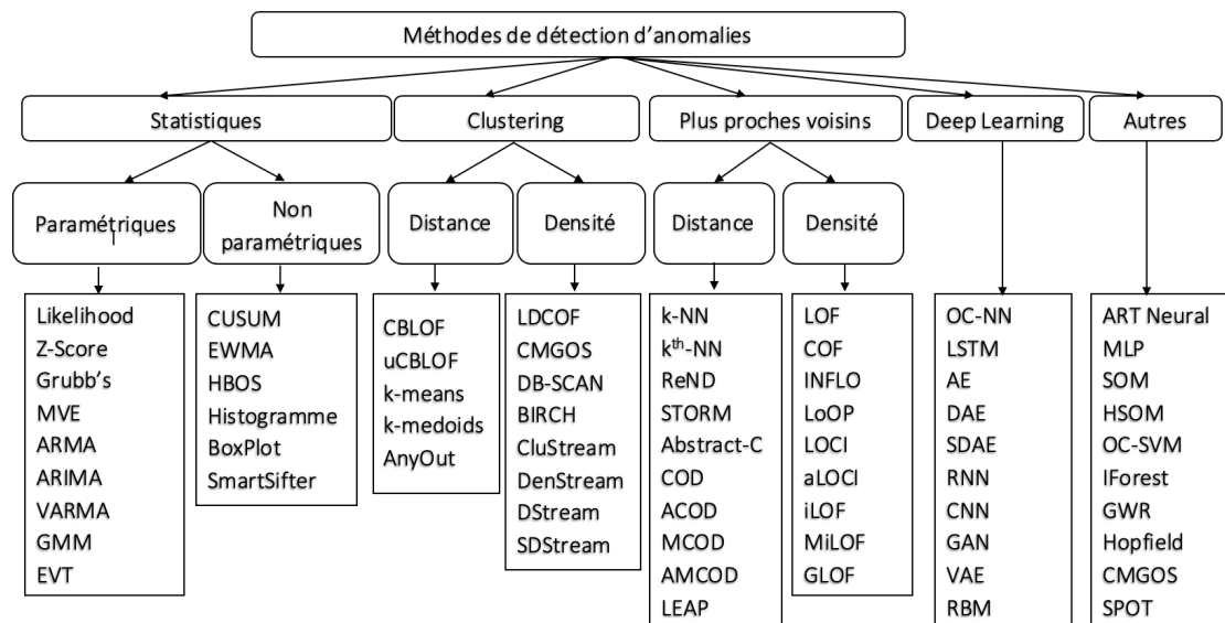
FIGURE 2.1 – Classification des différentes techniques de détection d'anomalies.
