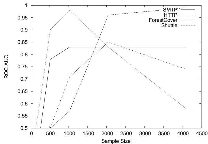
FIGURE 3.6 – Impacts de la taille de l'échantillon sur les résultats de IForest. Évaluation sur quatre (4) jeux de données réels.
