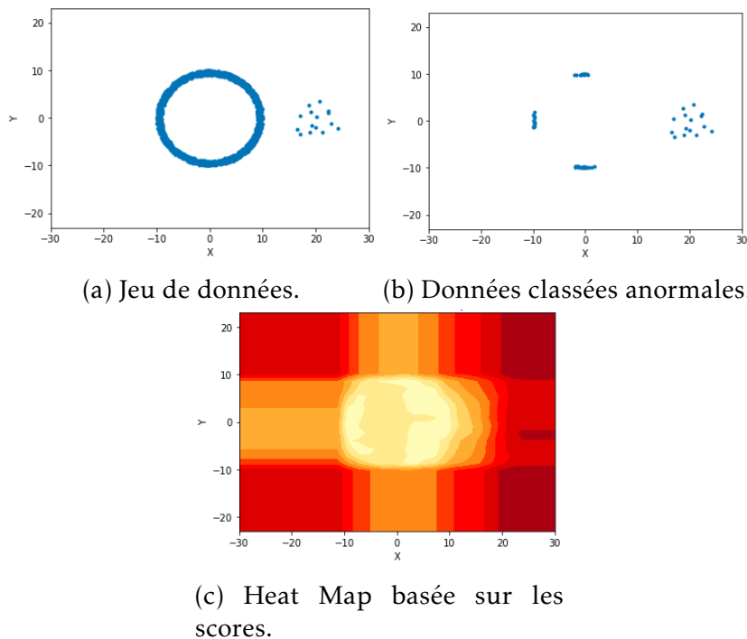
FIGURE 3.8 – Impacts de la distribution des données sur IForest.
