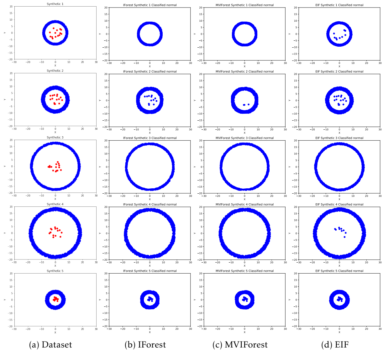
FIGURE 3.11 – Données classées normales par IForest, EIF et MVIForest respectivement dans les jeux de données Synthetic_1, Synthetic_2, Synthetic_3, Synthetic_4 and Synthetic_5 .
