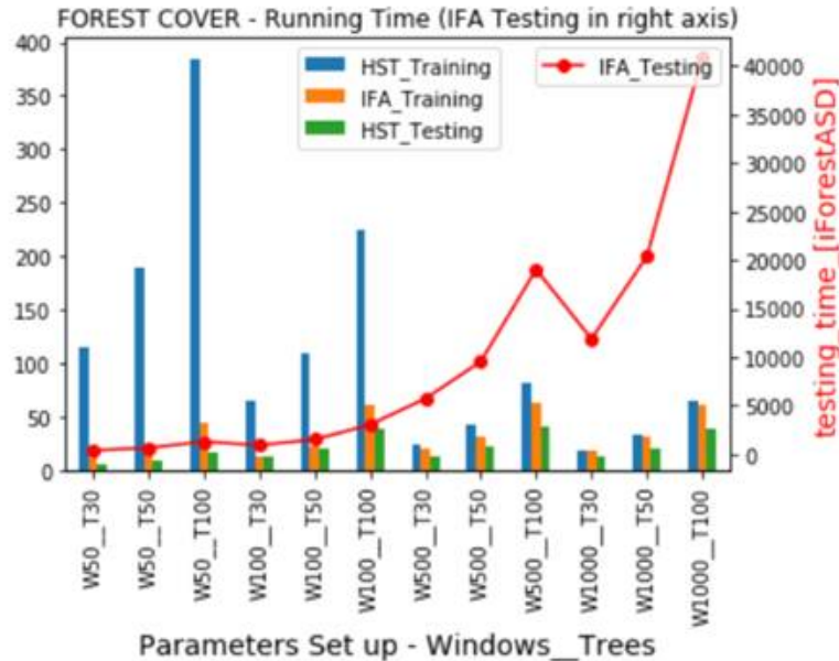
FIGURE 4.7 – Mesure du temps d'exécution (en secondes) : Jeu de données Forest-Cover - nous avons fixé la taille de la fenêtre (50, 100, 500, 100) et varié le nombre d'arbres (30, 50, 100) pour comparer le temps d'exécution de HST et IForest ASD. Le temps de test de IForest ASD est représenté dans une autre échelle sur l'axe Y de droite et tracé en ligne rouge.
