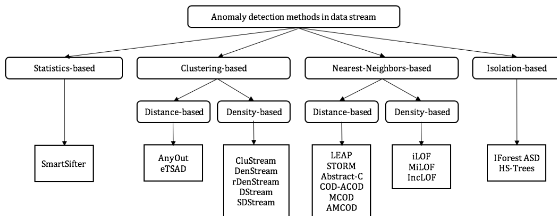
FIGURE 4.4 – Classification des méthodes de détection d'anomalies dans les flux de données.
