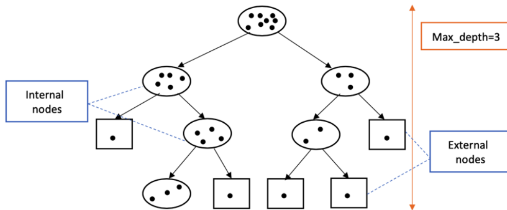
FIGURE 2.5 – Exemple d'arbre ( iTree ) avec \psi = 8 .
