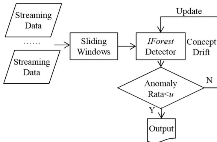
FIGURE 4.5 – Workflow de l’algorithme Isolation Forest ASD pour la détection de drift implémenté dans scikit-multiflow. Image extraite du papier original (DING et FEI, 2013).
