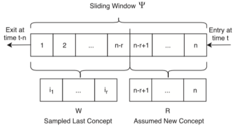
FIGURE 5.4 – La stratégie de mémoire utilisée par RAAB et al. dans RAAB et al. (2020) pour la détection du concept drift : à chaque pas de temps, r échantillons sont sélectionnés aléatoirement. Ils sont comparés aux r échantillons les plus récents de la fenêtre parmi les n échantillons stockés dans une fenêtre glissante \Psi .
