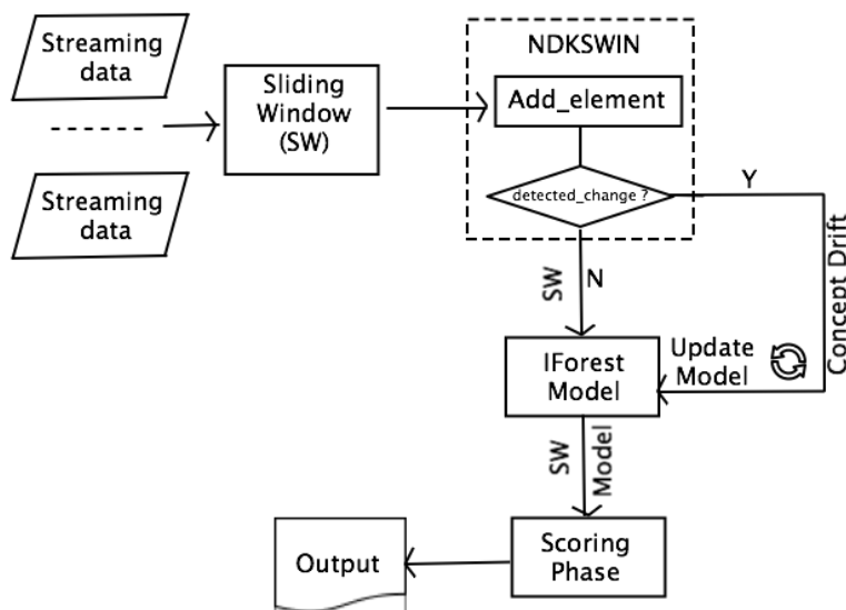
FIGURE 5.5 – Workflow de IForest ASD basé sur NDKSWIN (NDKSWIN IFA).
