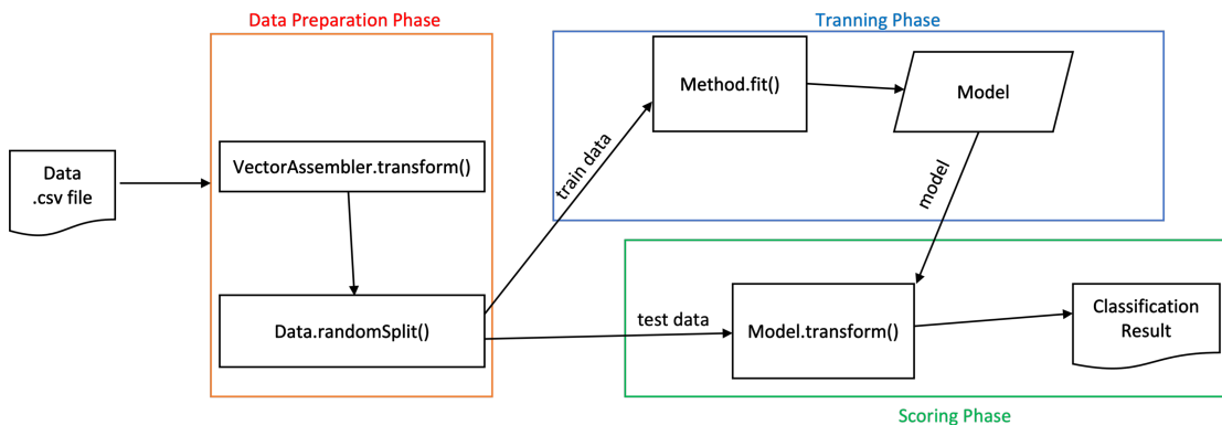
FIGURE 6.4 – Architecture générale d'un algorithme de machine learning utilisant MLib
