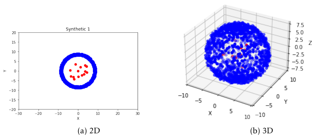
FIGURE 3.3 – Dataset Synthetic_1 : Forte densité des données normales (ND++), faible densité des données anormales (AD+) et petite distance entre les données normales et anormales (dAN+).
