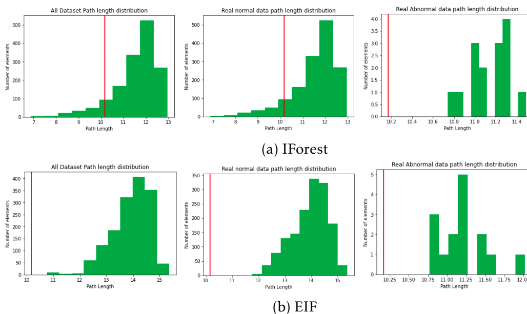
FIGURE 3.13 – Distribution de la longueur des chemins obtenus avec une exécution de IForest et EIF sur le jeu de données Synthetic_5.
