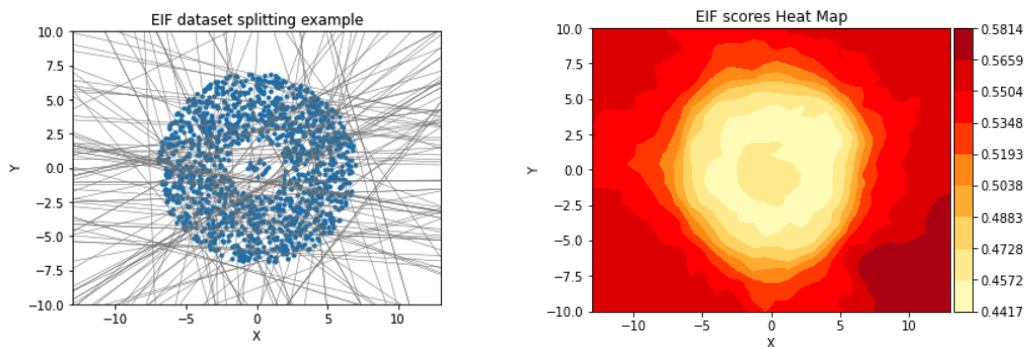
FIGURE 3.2 – Exemple de scissions des noeuds par EIF avec sa heat map basée sur les scores : disparition des zones sombres artificielles. X et Y sont les coordonnées des données.
