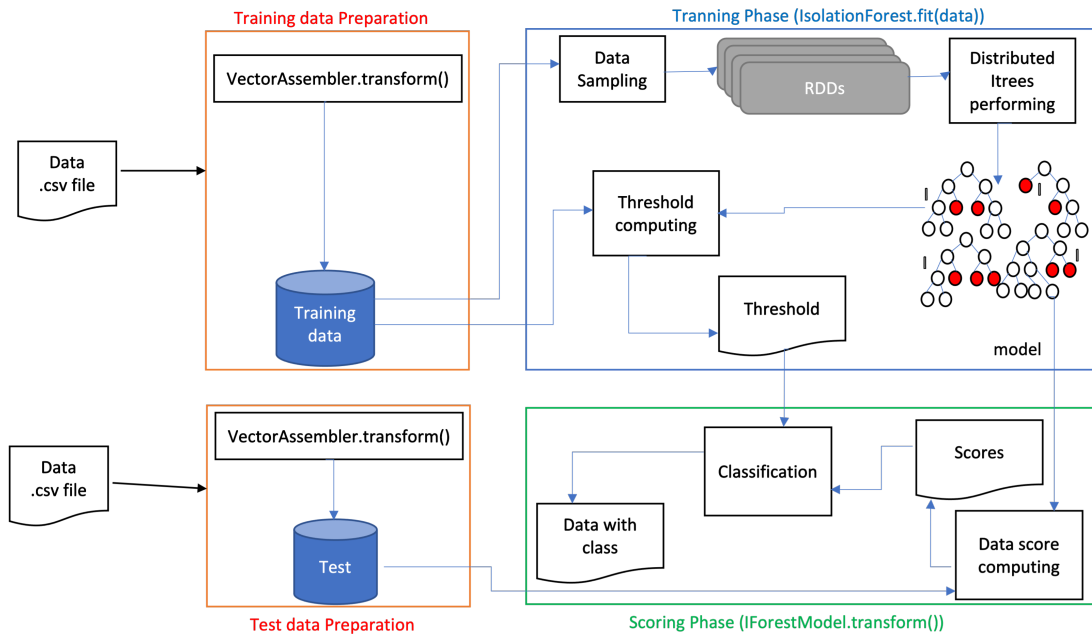
FIGURE 6.5 – Architecture général de LDIForest et de FDIForest
