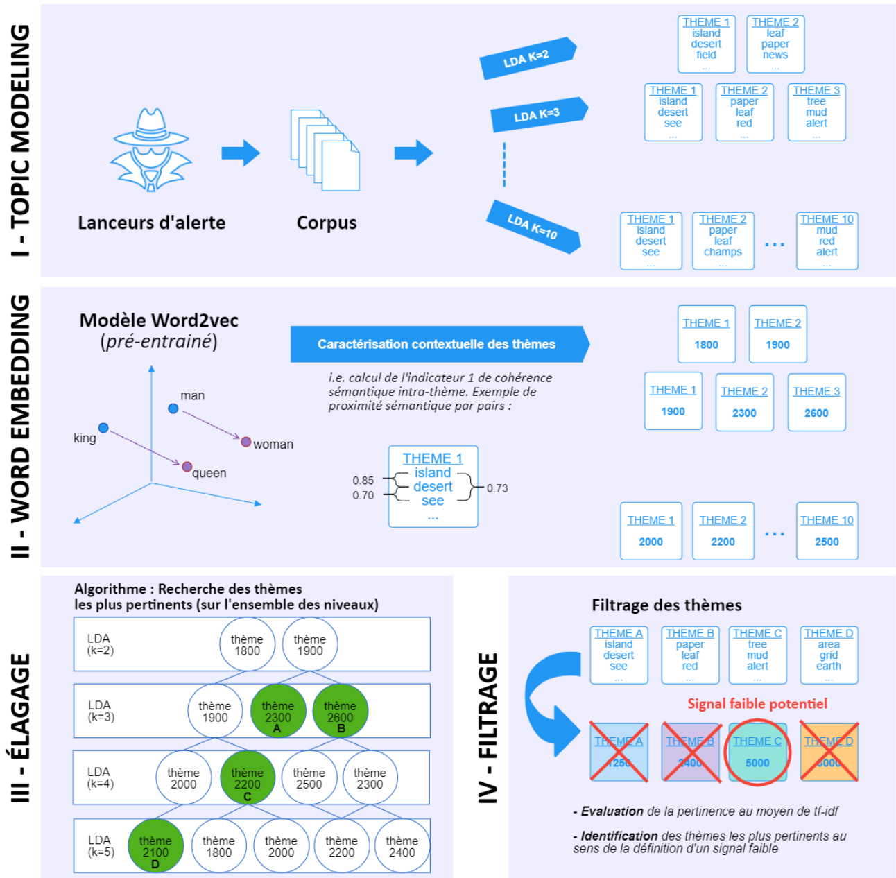
FIGURE 1.6 – La première partie de la chaîne de traitement utilise une approche de Topic Modeling et de Word Embedding. L’algorithme que nous proposons dans le chapitre 2 permet d’extraire les thèmes les plus pertinents sur plusieurs niveaux de LDA au moyen d’un indicateur basé sur Word2Vec. Le filtrage permet de récupérer les mots pertinents dans chaque thème selon notre définition du signal faible.
