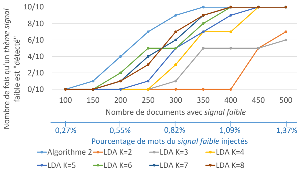
FIGURE 2.23 – Résultats de l'algorithme 2 comparé aux 7 LDAs originaux paramétrés avec k variant de 2 à 8 sur la détection d'un thème signal faible dans les thèmes déterminés par l'approche de modélisation thématique multi-niveaux. Dans chaque document, nous insérons 3 séries de 4 mots du Thème Droit (signal faible). L'identification du thème signal faible est réalisée par le calcul de la somme des poids des mots n'appartenant qu'à un des 5 Thèmes (Economie, Histoire, Informatique, Médecine et Droit (Signal faible)). Le thème est identifié signal faible lorsque la valeur du Thème Droit est la plus importante.
