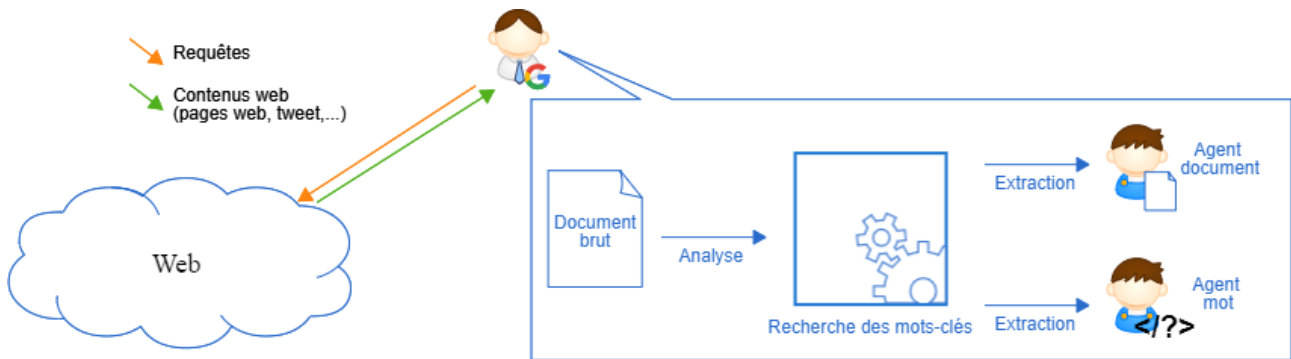
FIGURE 3.12 – Un agent de recherche effectue des requêtes dans un moteur de recherche avec des mots-clés d'un thème (e.g. signal faible potentiel). Pour chaque document trouvé, il extrait le segment de document le plus pertinent contenant les mots-clés de la requête et l'ajoute aux documents déjà présents dans le corpus d'étude afin d'enrichir les données.
