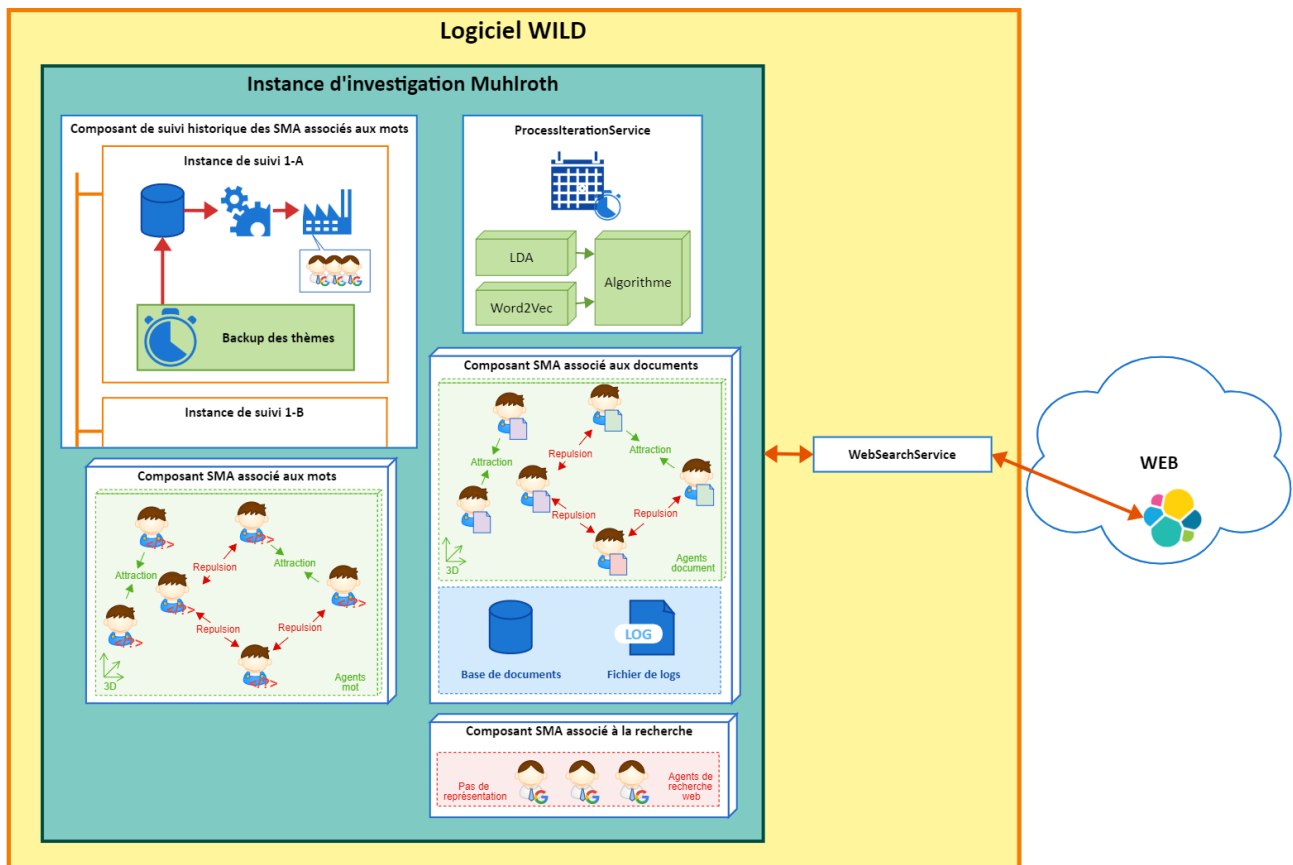
FIGURE 4.6 – Composants et services utilisés pour l'expérimentation sur la base documentaire de Mühlroth
