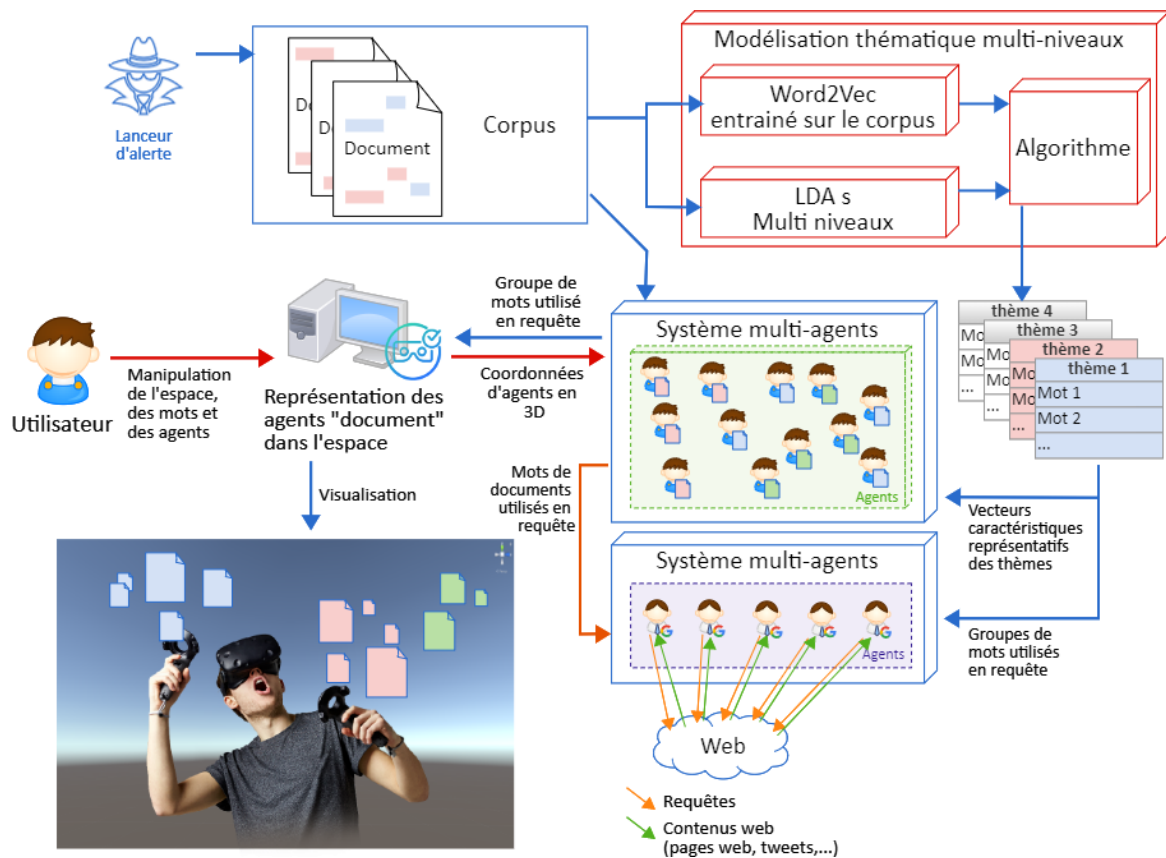
FIGURE 3.5 – Schéma de la chaîne de traitement. Les thèmes obtenus par la modélisation thématique multi-niveaux décrite au chapitre 2 ainsi que le corpus de documents sont injectés dans les systèmes multi-agents. Une interface visuelle et interactive permet à l'utilisateur d'interagir avec le système. Ce dernier effectue alors des recherches sur le Web afin d'enrichir le corpus de nouveaux documents en rapport avec les thèmes trouvés et ceux sélectionnés par l'utilisateur. Lorsque l'utilisateur choisit de manière interactive un document, les requêtes sont construites à partir des mots-clés présents dans le document et découverts dans les thèmes. Actuellement, l'interface utilisateur permet uniquement une interaction classique simple de type clic souris.
