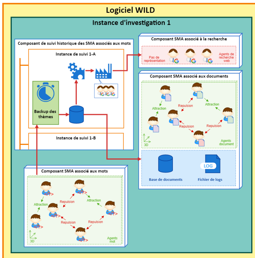
FIGURE 3.24 – Le composant effectuant le suivi historique sauvegarde les thèmes et leur liste de mots-clés afin d'étudier leur évolution. Ces mots-clés permettent la construction de nouveaux agents de recherche.
