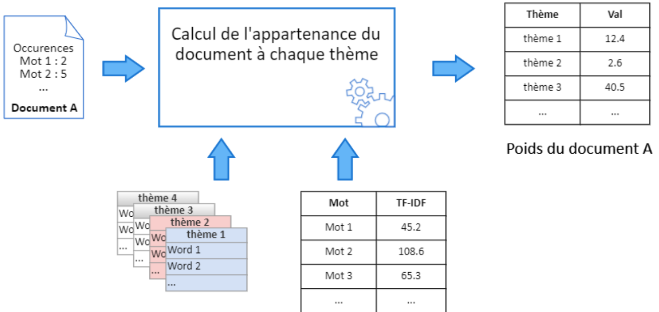
FIGURE 3.7 – Pour chaque document est calculé un vecteur caractéristique composé de n valeurs, chacune d’elles définit la composante du document associée à un thème. Ce vecteur caractéristique permet l’application des forces d’attraction/répulsion dans le système multi-agents construit. Pour chaque thème, et chaque document, nous calculons le nombre d’occurrence des mots du thème présents dans le document en prenant en compte leur rareté et le fait que ces mots soient présents dans peu de documents (grâce à leur valeur de tf-idf ).
