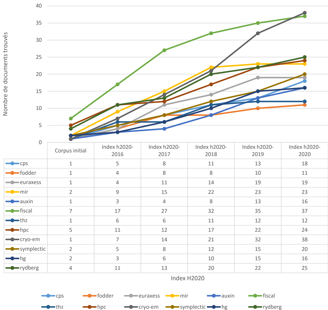
FIGURE 4.5 – Evolution, pour chaque index, du nombre de documents rapportés par les mots-clés les plus pertinents.
