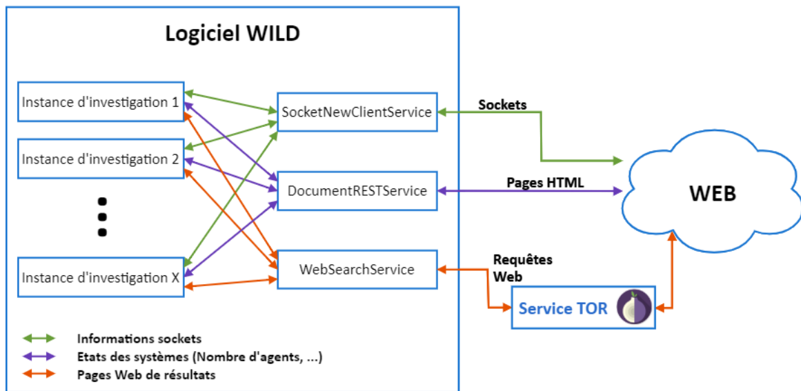
FIGURE 3.15 – Vue globale du logiciel WILD et des différents services connectés servant d'interface pour l'accès au Web.
