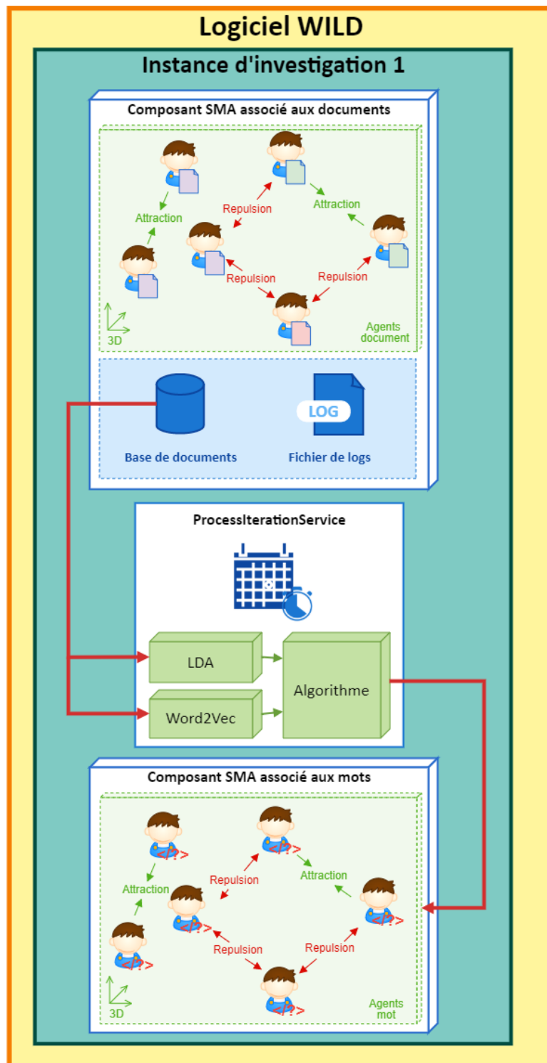
FIGURE 3.20 – Le service du processus itératif agit comme un orchestrateur et planifie la phase de modélisation thématique. Les thèmes sont mis à jour et les mots associés à ces thèmes sont de nouveau injectés dans le composant multi-agent associé aux mots.
