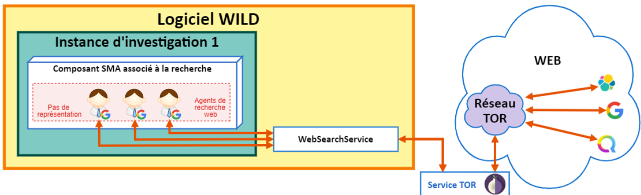
FIGURE 3.17 – Présentation des échanges de données entre les agents de recherche, le service “WebSearchService”, le service TOR et les moteurs de recherche. Les agents effectuent leurs requêtes auprès du service de recherche Web. Celui-ci lance la requête sur les moteurs de recherche au travers du service TOR.
