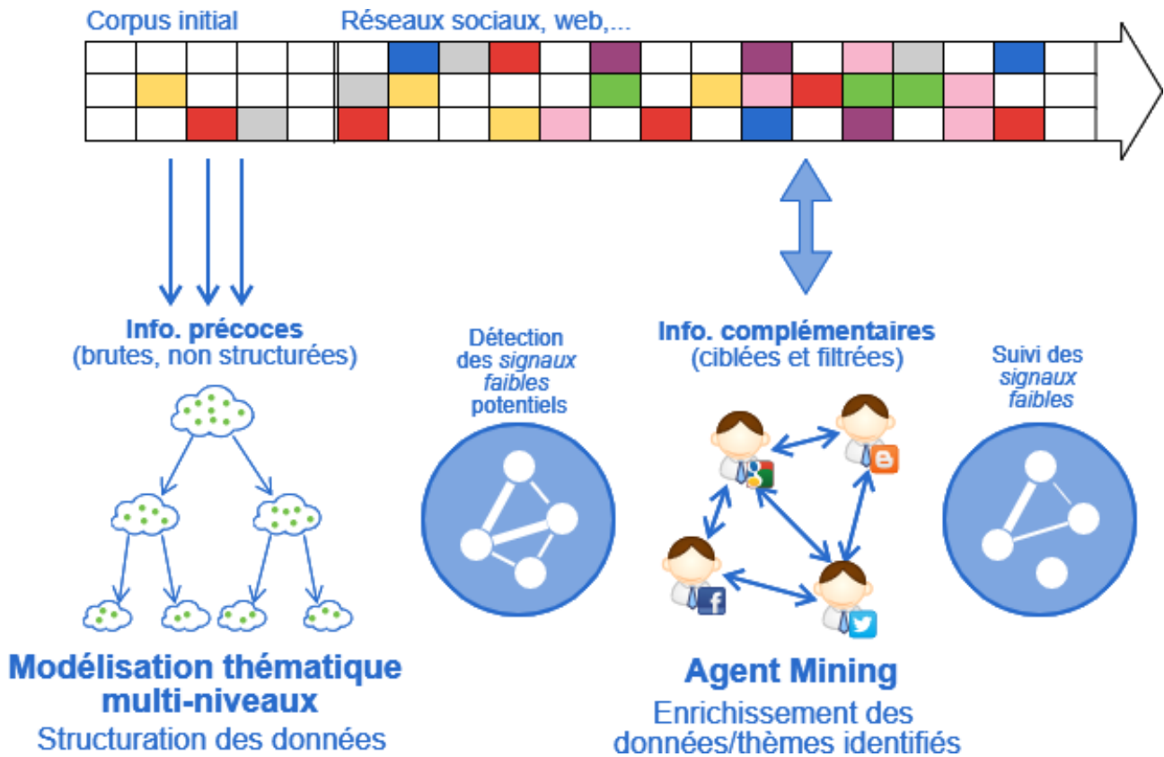
FIGURE 2 – Stratégie de détection des signaux faibles. Elle passe par l'analyse de l'information précoce apportée par un lanceur d'alerte et l'extraction des collections de mots associées aux Thèmes découverts. Ces informations permettent ensuite de mieux cibler la phase de data mining pour la détection des signaux faibles. Chaque rectangle de couleur représente une source d'information (ex : documents) exploitée.
