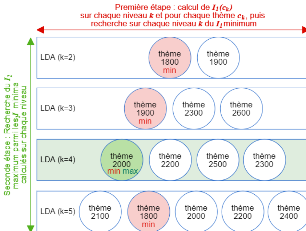
FIGURE 2.13 – Représentation de l'application de l'algorithme 1 sur les différentes partitions LDA obtenues pour k \in \{2...5\} . Les partitions sont organisées par niveau : la partition obtenue pour k = 2 est au niveau le plus haut. Les niveaux sont représentés par des rectangles. Les valeurs pour chaque thème sont celles de l'indicateur I_1 . Les cercles rouge et vert représentent les plus petites valeurs de chaque niveau de LDA. Parmi ces valeurs, la plus élevée correspond à LDA 4 ( k = 4 ), désignant la partition la plus cohérente au sens du critère contextuel.
