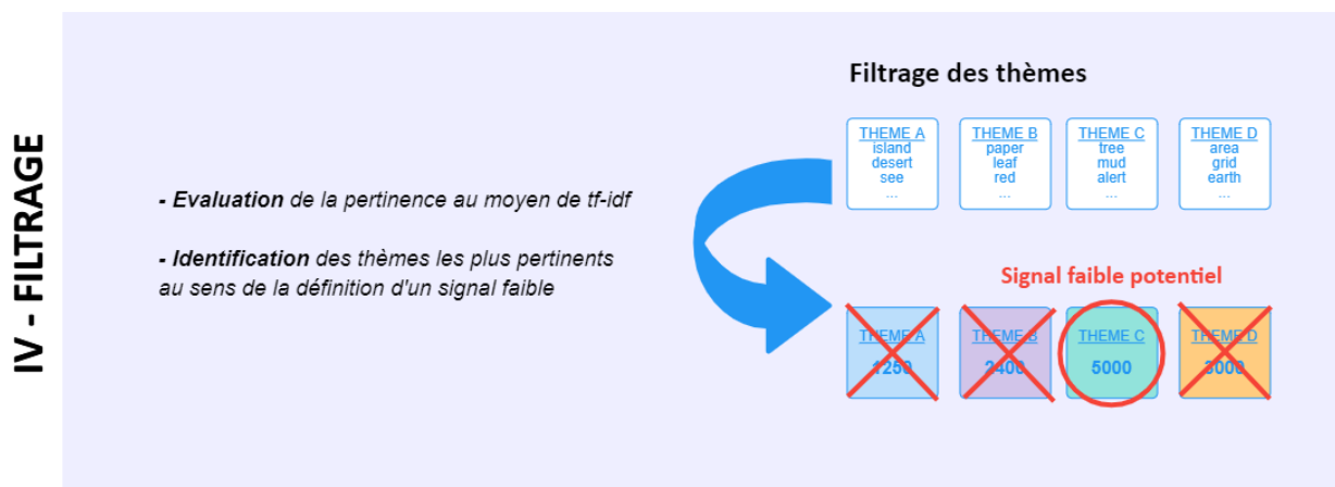
FIGURE 2.10 – Filtrage des thèmes au moyen d'une évaluation de la pertinence au moyen de tf-idf . Nous identifions les thèmes signaux faibles potentiels.
