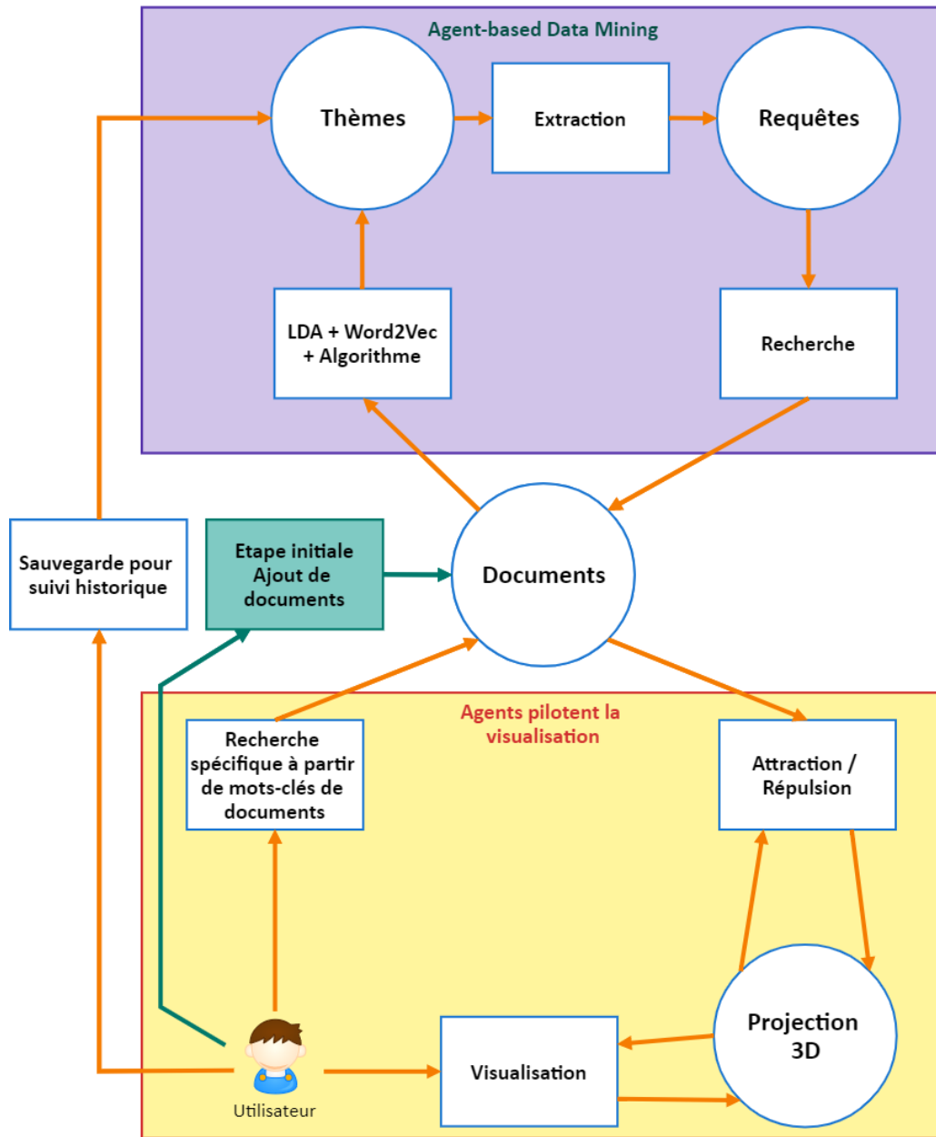
FIGURE 3.26 – Présentation fonctionnelle de la chaîne de traitement et du sens de transfert des données entre fonctions.
