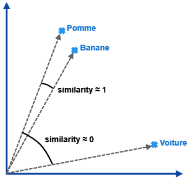
FIGURE 2.5 – Projection en 2 dimensions de la similarité contextuelle de mots. Une valeur de similarité proche de 1 indique des mots utilisés dans des contextes similaires, inversement, 0 pour des mots avec un faible lien contextuel.
