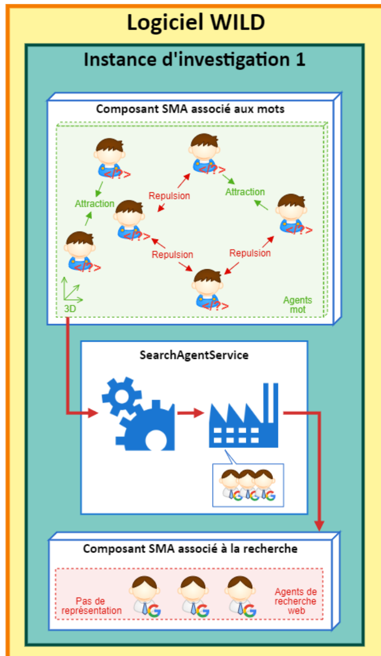
FIGURE 3.22 – Le service d’agents de recherche produit, à partir de groupes de mots provenant des thèmes, de nouveaux agents de recherche. Ces agents sont en charge de la récupération des sections de texte pertinentes afin d’augmenter le corpus initial. Ce corpus est ensuite ré-analysé par le service du processus itératif (cf. section 3.4.2.4) qui met en œuvre l’approche de modélisation thématique multi-niveaux (approche conjointe LDA/Word2Vec). Les thèmes et leurs mots-clés associés sont alors mis à jour et de nouvelles recherches sont lancées.
