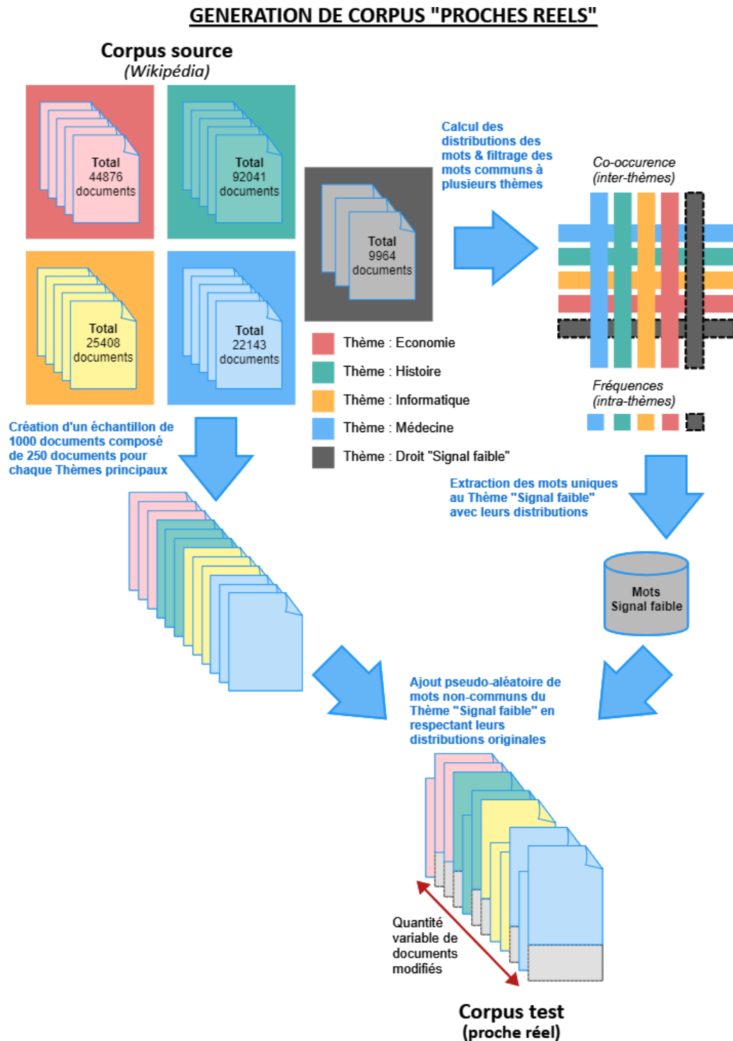
FIGURE 2.22 – Méthode de génération du corpus “proche du réel” qui consiste en l’injection de mots dits “non-communs” empruntés au Thème signal faible ( Droit en l’occurrence ) en respectant leur distribution originale. Ces mots non-communs sont identifiés par une étude de co-occurrence entre Thèmes.
