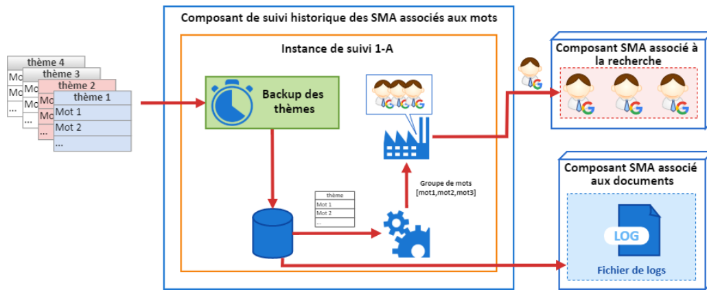
FIGURE 3.25 – Le composant effectuant le suivi prend en entrée les thèmes et les listes de mots-clés apportés par le composant SMA associé aux mots. Pour chacun d’entre eux, des agents de recherche sont créés à partir de combinaison de groupes de mots. Le composant enregistre l’évolution des valeurs tf-idf dans les logs.
