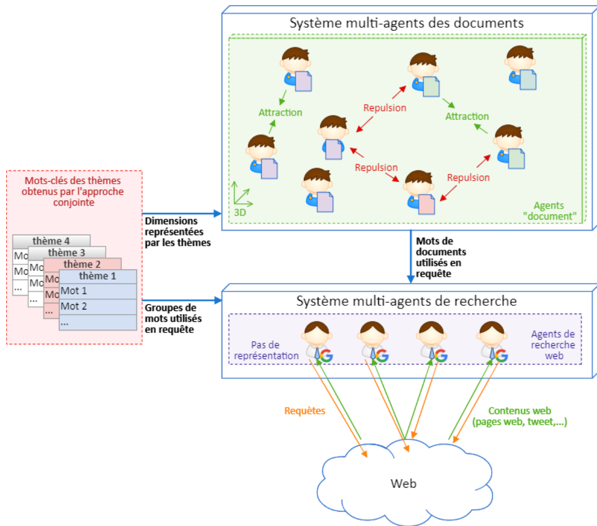
FIGURE 3.6 – Les agents “document” interagissent les uns avec les autres grâce à des actions de type attraction/répulsion. Les agents de recherche construisent des requêtes à partir des mots associés aux différents thèmes obtenus lors de la modélisation thématique multi-niveaux et éventuellement présents dans les documents sélectionnés par l'utilisateur (renforcement) (cf. Chapitre 2).
