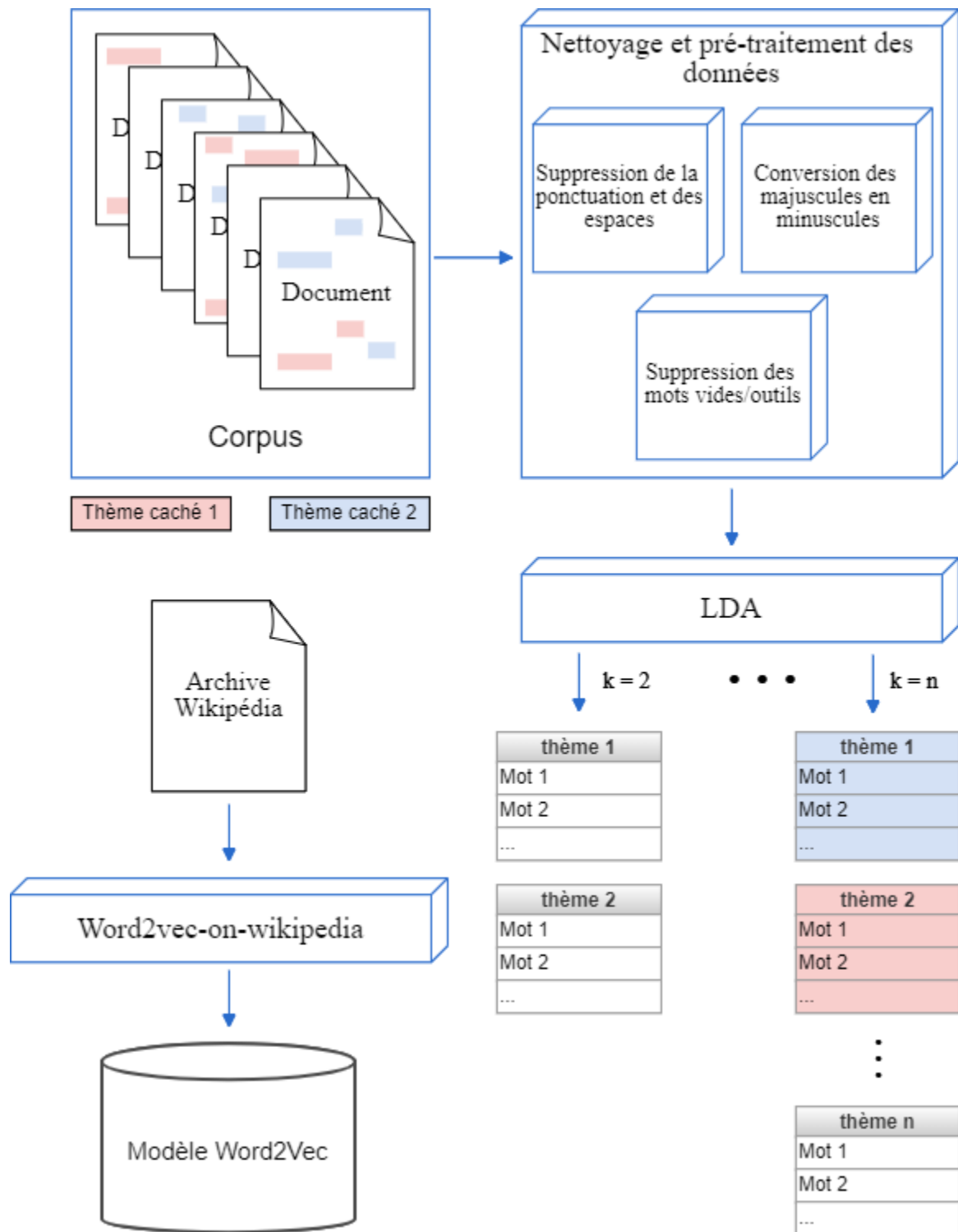
FIGURE 1.2 – Représentation des traitements utilisés sur les différentes sources de données. Les résumés des articles référencés par Mühlroth [MG18] correspondent au corpus. Nous appliquons différentes techniques de nettoyage pour rendre les données exploitables par l’approche de modélisation thématique utilisée. Nous appliquons LDA, nous lançons plusieurs expérimentations en faisant varier le nombre de thèmes. Pour notre approche de plongement de mots qu’est Word2Vec, nous utilisons un dump des articles provenant du Wikipédia Anglais pour entraîner un modèle au moyen de l’outil Word2vec-on-wikipedia.
