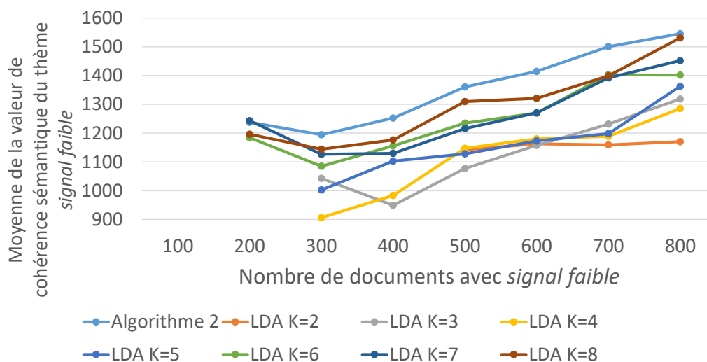
FIGURE 2.24 – Moyenne sur 10 tests de la valeur de cohérence sémantique du thème signal faible “détecté” avec l’algorithme 2 comparée aux 7 LDAs originaux paramétrés avec k variant de 2 à 8. L’algorithme 2 détecte le thème signal faible avec la plus grande valeur de cohérence comparée à celles de LDA.
