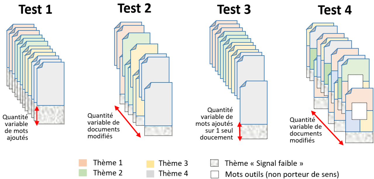
FIGURE 2.16 – Construction des 4 corpus de tests artificiels. Les mots du Thème signal faible sont injectés en quantité variable dans chaque document du corpus (test 1), ou bien dans une quantité variable de documents (test 2), ou encore en quantité variable dans un seul document avec (test 3) ou sans mots-outils (test 4)
