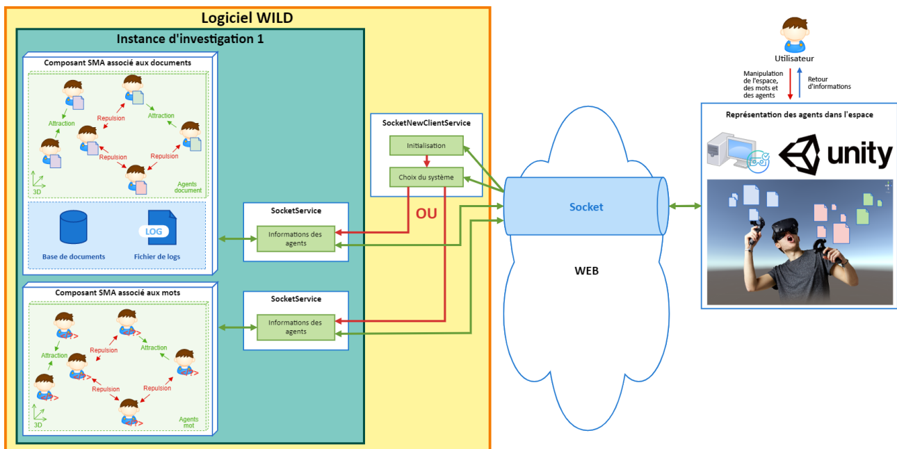
FIGURE 3.19 – Présentation des échanges de données via une socket entre un client de visualisation sous Unity et le logiciel WILD. Le service écoute sur un port, attendant la connexion de clients et le choix des informations sur l'instance qu'il souhaite afficher. La connexion est passée au service qui échange ces informations avec le client connecté.
