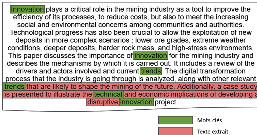
FIGURE 3.13 – L’agent de recherche identifie la position des mots-clés (en vert) dans le document. Il extrait du document le segment de texte le plus pertinent contenant l’ensemble des mots-clés. Dans cet exemple, la requête était composée des mots-clés “innovation”, “trends” et “technical”. La section de couleur rouge correspond à la section récupérée pour former un nouvel agent “document”.
