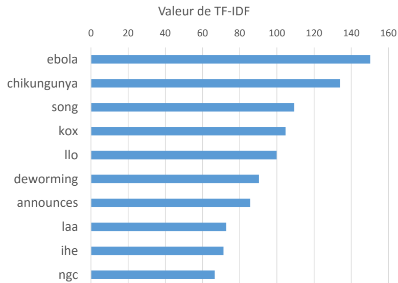
FIGURE 2.27 – Liste des mots du corpus ayant les plus grandes valeurs de pondération tf-idf . On remarque que les mots clés du thème signal faible détecté sont parmi les premiers de la liste.
