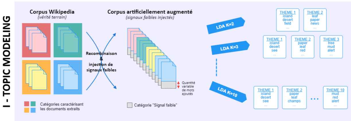
FIGURE 2.7 – Etape de génération du corpus de test sur la base d'un jeu de données extrait de Wikipédia. Nous appliquons LDA sur l'ensemble des documents, tout en faisant varier le nombre de thèmes.
