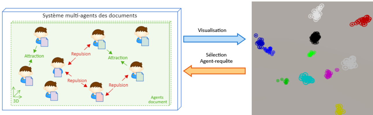
FIGURE 3.10 – L'utilisateur visualise les documents du système multi-agents dans un espace en 3D. Chaque document est représenté par un point dans l'espace. L'utilisateur peut sélectionner un agent pour le transformer en agent-requête. Les autres agents de l'espace vont s'organiser autour de cet agent que l'utilisateur aura sélectionné en utilisant les forces d'attraction/répulsion calculées entre paires d'agents à partir des N composantes des vecteurs caractéristiques.
