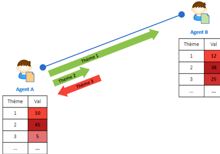
FIGURE 3.8 – Chaque agent "document" a un vecteur caractéristique qui décrit les liens du document avec chaque thème. Ces liens servent à calculer les forces d'attraction et répulsion de l'agent "document" A. La somme des forces résultantes s'ajoute à celles calculées aux itérations précédentes.
