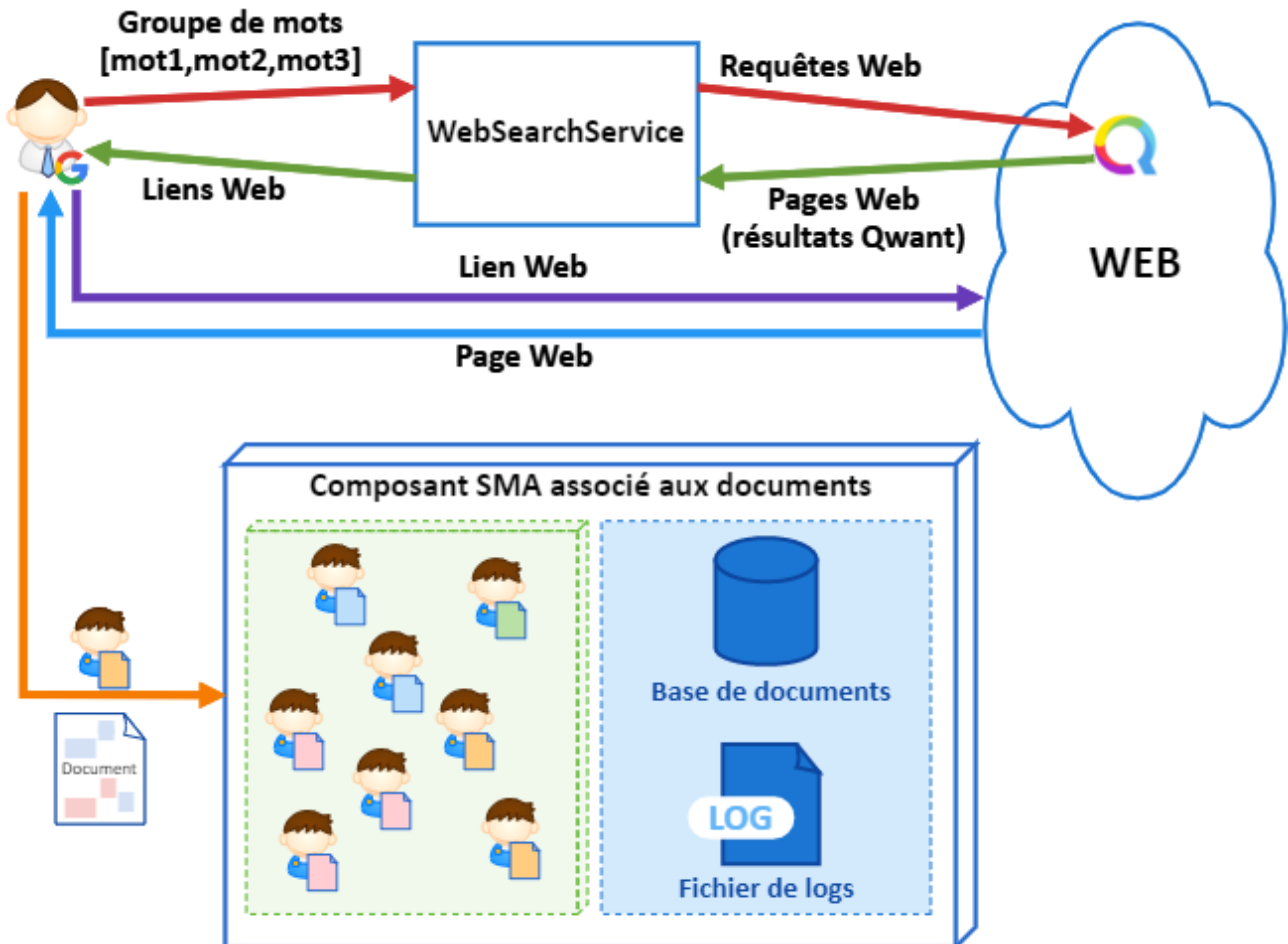
FIGURE 3.18 – Un agent de recherche utilise les liens Web fournis par le service de recherche Web, suite à ses requêtes, pour transformer en agents “document” les pages Web après extraction du contenu pertinent (voir 3.3.3.1)
