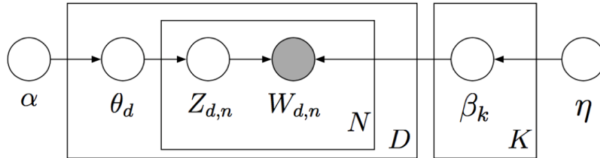
FIGURE 2.3 – Représentation graphique de LDA
