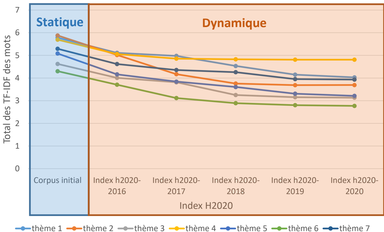
FIGURE 4.3 – Evolution de la valeur de tf-idf pour chaque thème. Le corpus initial regroupe les articles des années 2014-2015. La valeur est calculée sur les 20 premiers mots de chaque thème après qu'ils aient été triés.
