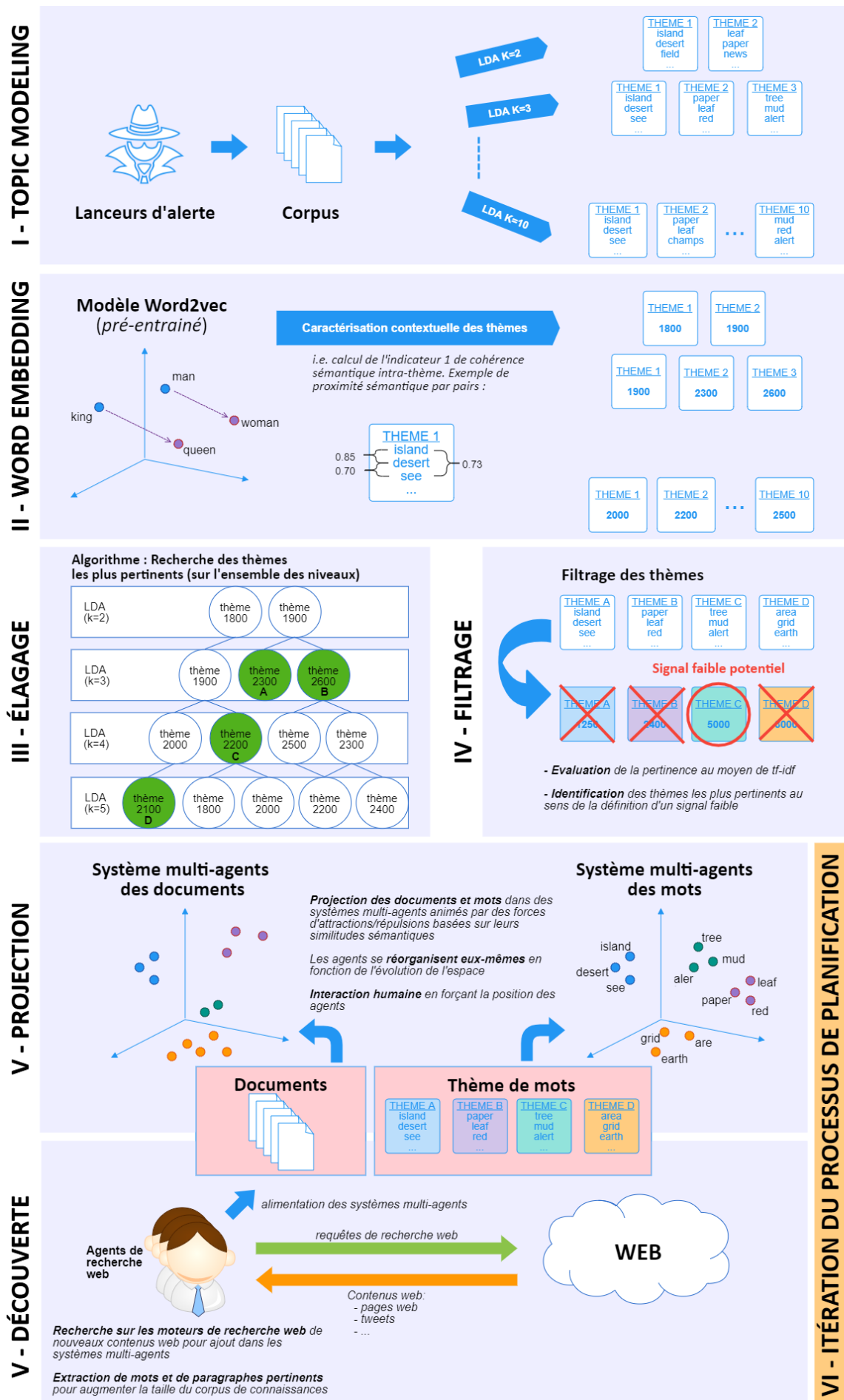
FIGURE 4 - Les différentes étapes pour extraire les signaux faibles
