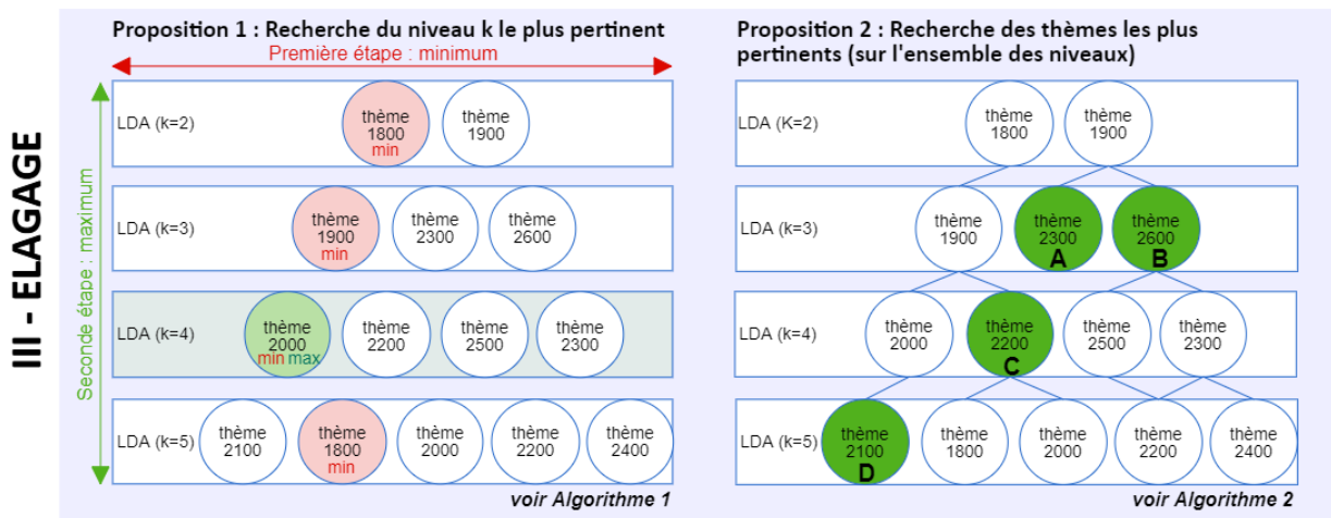
FIGURE 2.9 – La proposition 1 montre la recherche du niveau de l'arborescence donnant les thèmes les plus cohérents au sens du critère de ressemblance. La proposition 2 montre l'élagage des thèmes reliés entre eux dans l'arborescence au moyen d'un critère de ressemblance. L'objectif est dans ce deuxième cas de rechercher les thèmes les plus cohérents sur l'ensemble de l'arborescence.
