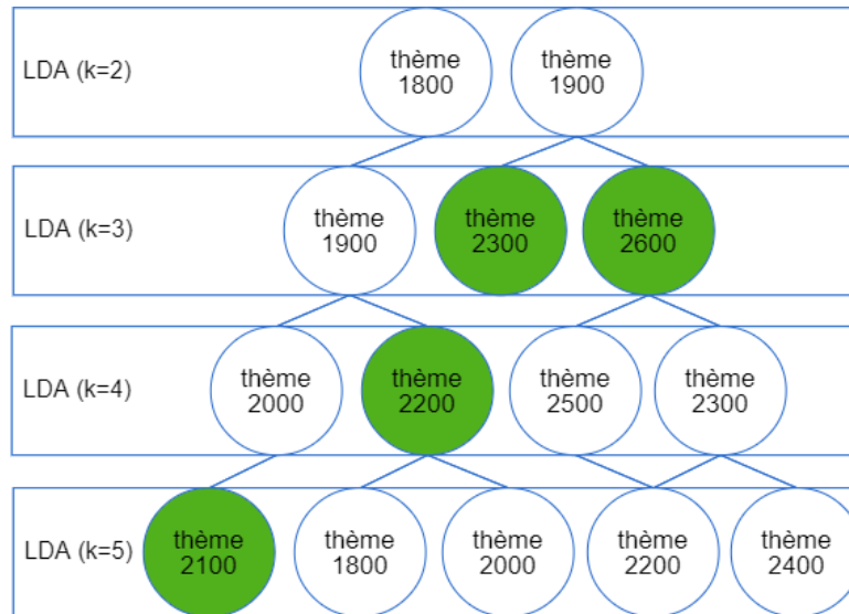
FIGURE 2.14 – Représentation de l’algorithme 2 sur les différentes partitions LDA obtenues pour k \in \{2 \dots 5\} après avoir construit l’arborescence en utilisant l’indicateur de ressemblance I_2 . Un lien est formé entre chaque thème de niveau k et un thème de niveau k + 1 si la valeur de l’indicateur I_2 est supérieure à un seuil défini arbitrairement. Les partitions sont organisées par niveau : la partition obtenue pour k = 2 est au niveau le plus haut. Les niveaux sont représentés par des rectangles. Les thèmes ont tous été triés dans une liste par ordre croissant selon l’indicateur I_1 sans distinction du niveau k (cf. Tableau 2.2). Nous sélectionnons le premier élément de la liste et supprimons ses fils et parents avec les méthodes Parents(c_k) et Fils(c_k) . Cette tâche est exécutée jusqu’à ce que la liste soit vide. Les éléments récupérés forment les thèmes les plus pertinents selon l’algorithme 2.
