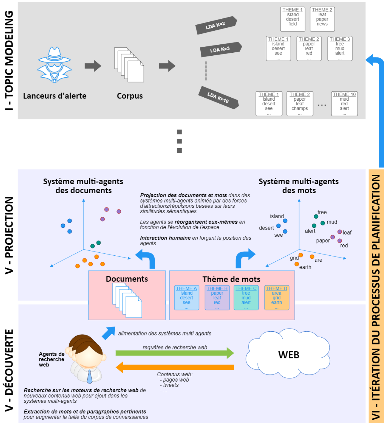
FIGURE 1.7 – La seconde partie de la chaîne de traitement met en œuvre une solution d'agent mining, une combinaison de méthodes de data mining et de système multi-agents. Les documents du corpus sont projetés dans un système multi-agents animés par des forces d'attraction/répulsion construites sur des similitudes sémantiques (pour les documents) ou de contexte (pour les mots). Des agents de recherche enrichissent le système de nouveaux documents par des requêtes sur des moteurs de recherches (tel que Qwant) à partir des mots-clés des thèmes identifiés.
