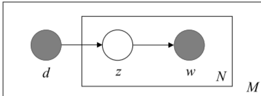
FIGURE 2.2 – Représentation graphique de pLSA
