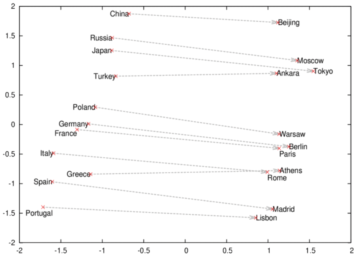
FIGURE 2.6 – Exemple de termes (pays et leur capitale) projetés en deux dimensions par Analyse en composantes principales (PCA) appliquée à leurs descripteurs Word2Vec. Pendant l'apprentissage, aucune information n'est fournie sur le concept de capital. Le modèle est entraîné sur un corpus de Google News. Inspiré du travail de Mikolov [MSC + 13, MCCD13]
