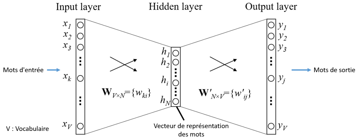
FIGURE 2.4 – Représentation graphique du plongement de mots
