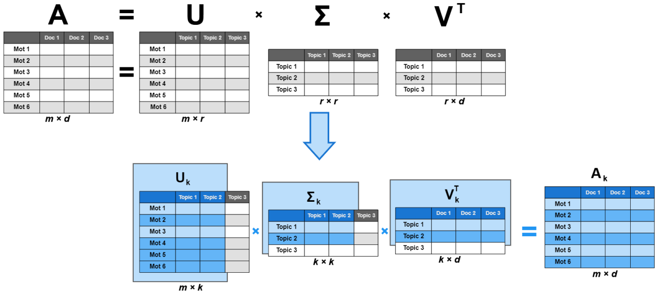
FIGURE 2.1 – Représentation graphique de LSA
