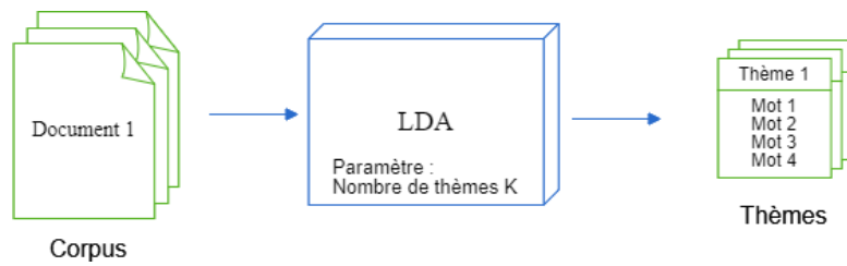
FIGURE 2.12 – Mise en œuvre de LDA sur un corpus de documents. En sortie, nous obtenons un ensemble de thèmes dont le nombre est spécifié en paramètre d’entrée.
