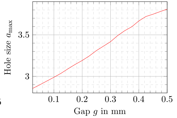
(d) Corresponding hole size a_{\max} .
