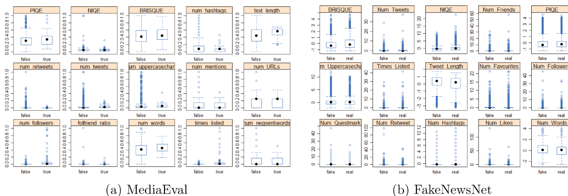
FIGURE 3.6 – Distribution des classes vraie et fausse pour les 15 caractéristiques les plus importantes
