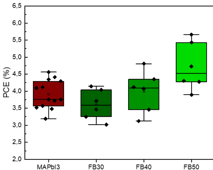
Figure 42: Variation du PCE des cellules solaires des pérovskites \text{MA}_{1-y}\text{FA}_y\text{PbI}_{3-x}\text{Br}_x en fonction du taux de \text{FBr}/(\text{MAI}+\text{FABr}) introduit dans la solution de conversion (en vert), comparé au PCE de la simple pérovskite \text{MAPbI}_3 (en rouge)
