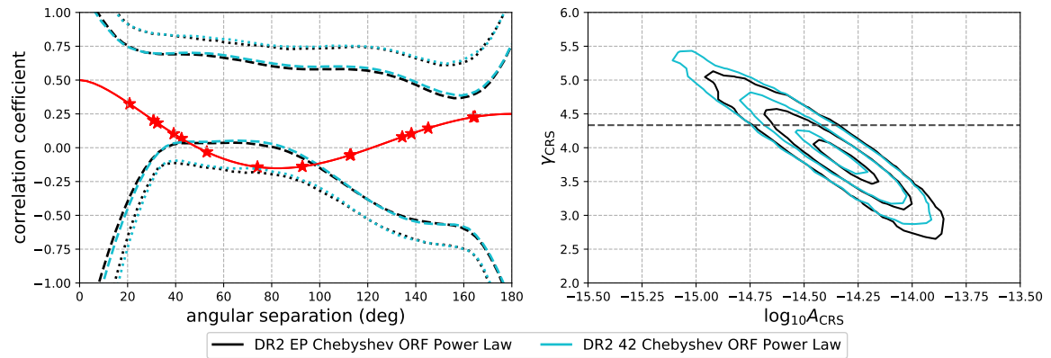
Figure 1: Distributions posterieures des corrélations spatiales (à gauche), et de l’amplitude et de l’indice spectral de la loi de puissance (à droite) décrivant le CRS avec corrélations en paramètres libres obtenues avec l’EPTA DR2 - 6 pulsars, soit avec ENTERPRISE (EN), soit avec FORTYTWO (42). Les courbes en tirets et en pointillés dénotent les régions crédibles respectivement à 95% et 99.7%. La courbe rouge correspond aux corrélations Hellings-Downs théoriques, et les étoiles rouges montrent les séparations angulaires entre les six pulsars considérés.
