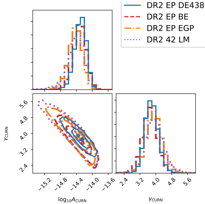
Figure 5: Distributions postérieures de l’amplitude et de l’indice spectral du CURN obtenues sans modèle décrivant les erreurs contenues dans les SSEs (DE438), ou bien en utilisant BAYESEPHM (BE), EPHEMGP (EGP) ou LINIMOSS (LM).
