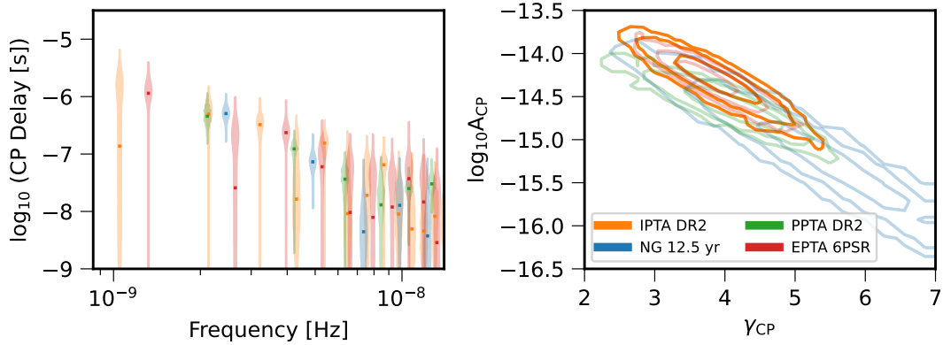
Figure 3: Comparaison des spectres (à gauche) et des distributions posterieures de l'amplitude et de l'indice spectral des lois de puissance (à droite) obtenues avec les plus récents jeux de données de NANOGrav, PPTA et l'EPTA, ainsi qu'avec l'IPTA DR2. Figure provenant de Antoniadis et al. 2022.
