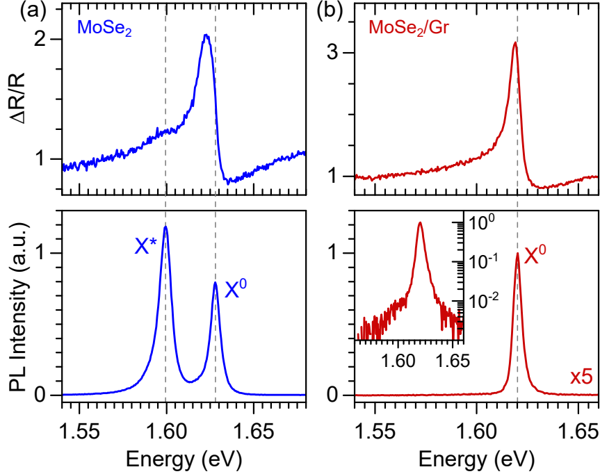
Figure 2: Identification de X^0 . Spectres de DR (en haut) et PL (en bas) de MoSe 2 (a) et de MoSe 2 /1LG (b) encapsulés par hBN. Les spectres ont été acquis à une température de 4 K, dans le régime d'excitation linéaire et en utilisant une laser continu avec une énergie de 2,33 eV.
