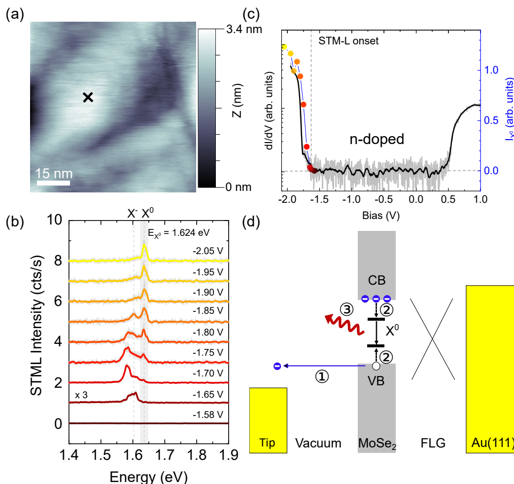
Figure 11: Mécanisme d'excitation. (a) Image STM d'une zone sur la surface MoSe 2 /FLG. L'image a été acquise sous une tension de -2 V et un courant de 5 pA. (b) Spectres de STML enregistrés à différentes polarisations sur la position marquée en (a). Les lignes pointillées correspondent à la position des résonances X^0 et X^- . Ces spectres ont été enregistrés à un courant de 30 pA. (c) Spectre de conductance différentielle pris au même endroit que dans (b). Le spectre est superposé avec l'intensité intégrée de la ligne X^0 en fonction de la tension appliquée. L'accord entre les deux supporte un scénario d'injection de charge pour le mécanisme d'excitation. Le code de couleur correspond à celui utilisé dans la figure (b). (d) Diagramme énergétique du mécanisme d'excitation. Premièrement, un électron est extrait de la bande de valence, laissant un trou derrière lui. Ensuite, un exciton est formé lorsque les électrons natifs du TMD se lient au trou. Enfin, l'exciton se recombine et émet un photon.
