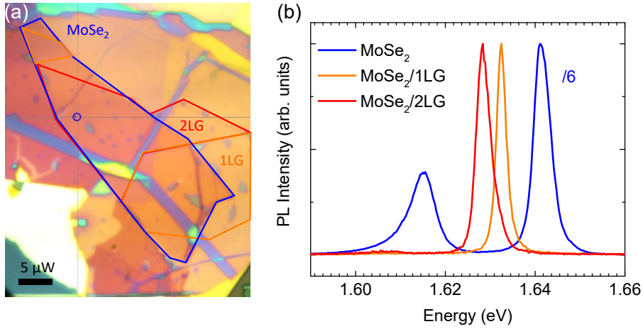
Figure 4: Spectre the PL à basse température de MoSe 2 /1LG encapsulée par hBN et déposé sur SiO 2 (a) Image de microscopie optique d'un échantillon composé par trois zones: MoSe 2 , MoSe 2 /1LG et MoSe 2 /2LG encapsulées par hBN. (b) spectres de PL correspondants aux trois zones principales de l'hétérostructure. Les spectres ont été enregistrés à 14 K, en utilisant une excitation laser à 1,96 eV continue et sous une intensité proche de 100 μW/μm 2 .
