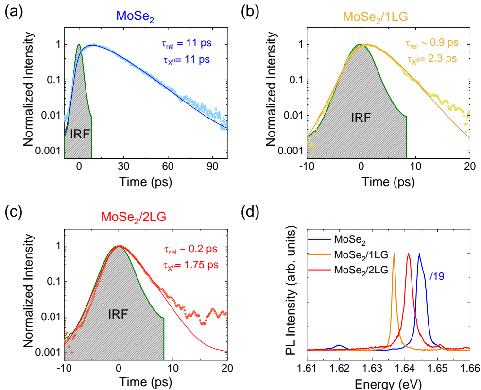
Figure 5: Dynamique excitonique à basse température. TRPL de l'émission de l'exciton neutre dans la zone de MoSe 2 (a) MoSe 2 /1LG (b) and MoSe 2 /2LG (c). (d) Spectres de PL correspondant aux zones du MoSe 2 , MoSe 2 /1LG and MoSe 2 /2LG. Tous les spectres ont été enregistrés à 14K et avec un laser pulsé à 722 nm dans le régime linéaire.
