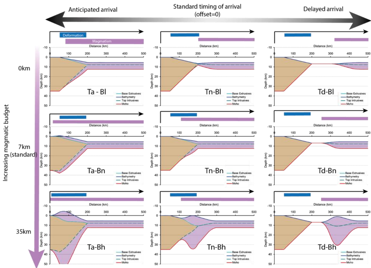
Figure 8: Marge équilibré résultant d'un modèle. L'axe horizontal tout en haut représente le timing relatif d'arriver du magma comparé au standard. L'axe vertical représente le budget magmatique initial. En brun est représenté la croûte continentale et en violet est représenté le magmatisme. Le diagramme au-dessus de chaque marge montre le timing relatif de la production magmatique (violet) par rapport à l'amincissement crustal (bleu).
