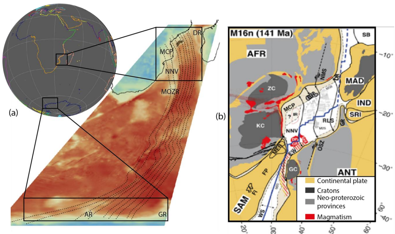
Figure 1: Le système conjugué Mozambique-Antarctique. (a) Carte de la bathymétrie avec les lignes de transport de Seton et al., 2012. (b) Reconstruction de Schimschal and Jokat, (2019). AFR: Afrique, ANT: Antarctique, IND: Inde, MAD: Madagascar, SAM: Amérique du Sud, SRI: Sri Lanka, DR, Davie Ridge, EW: Explora Wedge, FI: Falkland Islands, FP: Falkland Plateau, GC: Grunehogna Craton, GP: Galathea Plateau, GR: Gunnerus Ridge, IND: India, IR: Inharrime Ridge, KC: Kaapvaal Craton, MAD: Madagascar, MCP: Mozambique Coastal Plains, MEB: Maurice Ewing Bank, MozR: Mozambique Ridge, RLS: Riser Larsen Sea.
