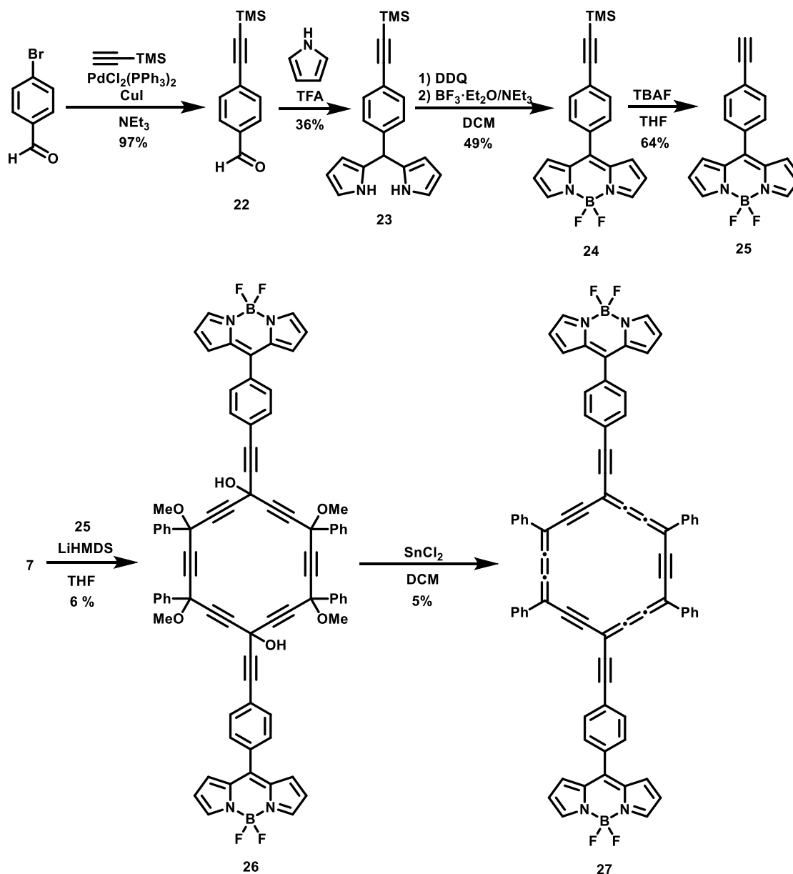
Schéma 3. Synthèse du carbo -benzène 27 à portant 2 fluorophores BODIPY
