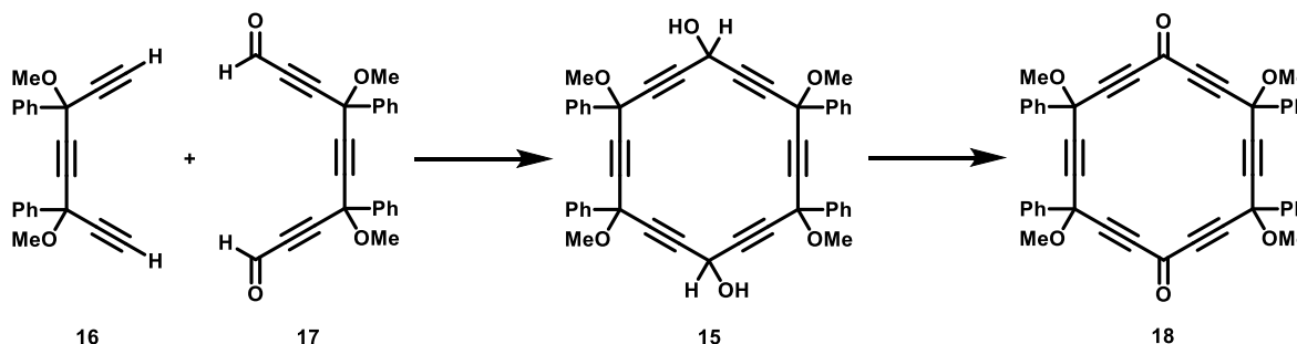
Esquema 3. Estrategia de ciclización [8+10] para la síntesis del [6]periciclinodiol 15
