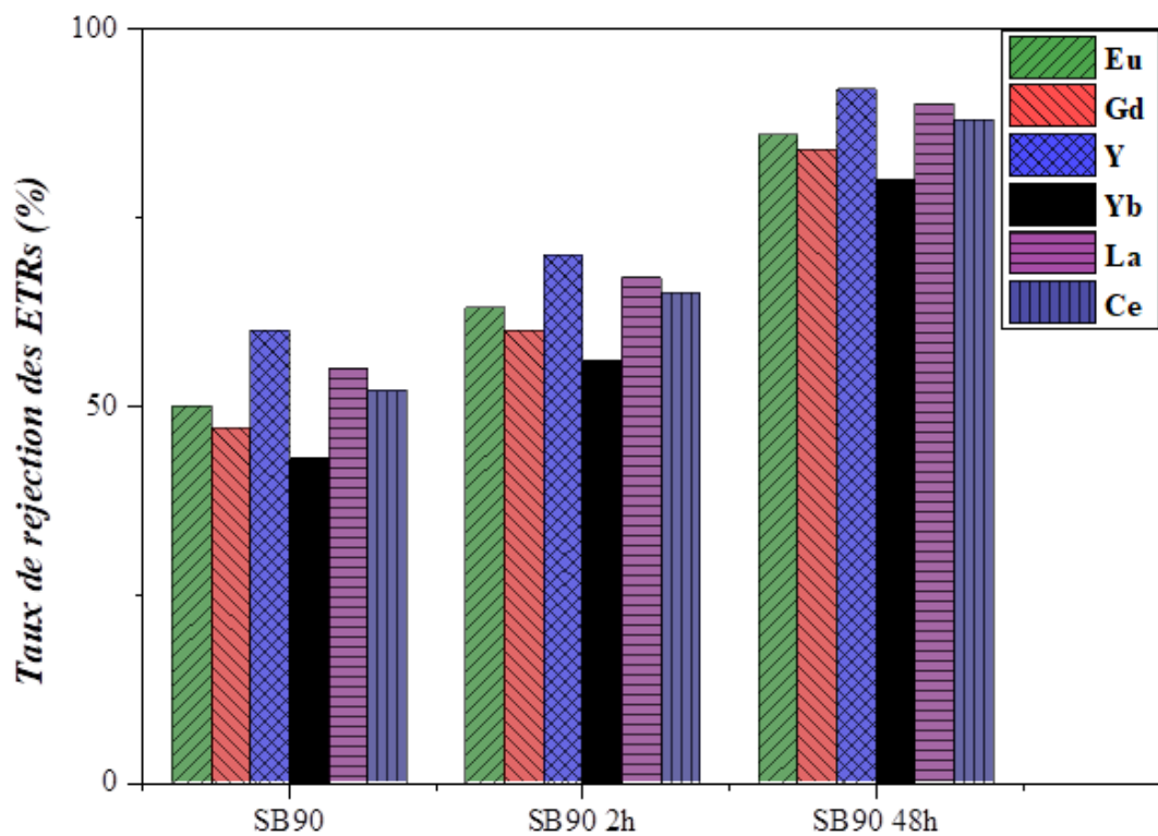
Figure C. 39 Taux de rejection des ETRs par les membranes SB90.
