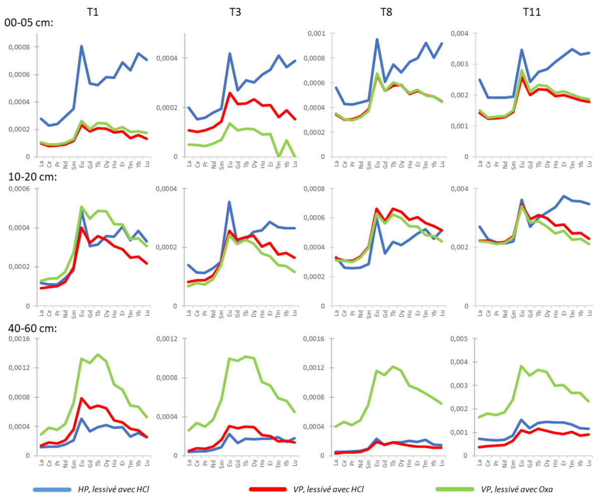
Figure 78: Spectres en REE des solutions de lessivage analysées à différents temps (T1: 13 heures, T3: 3 jours, T8 : 28 jours et T11 : 150 jours). Les concentrations en REE sont normalisées par rapport à la concentration du sol total de l'horizon correspondant.
