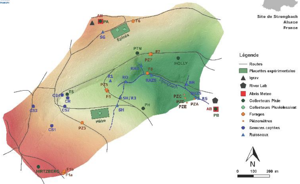
Figure 12: Equipements de l'OHGE sur le bassin versant du Strengbach.
