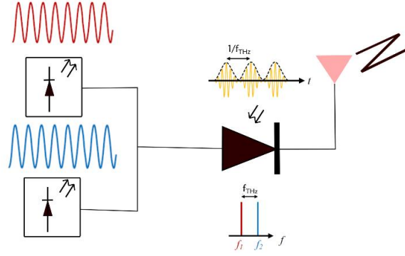
Figure 4.1. Illustration de la génération THz par photomélange
