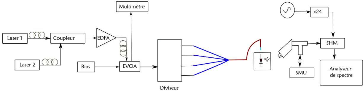
Figure 4.31. Banc expérimental de la caractérisation en puissance du réseau d'UTC-PD
