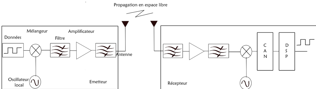
Figure 1.4. Synthèse d'une chaîne de radiocommunication
