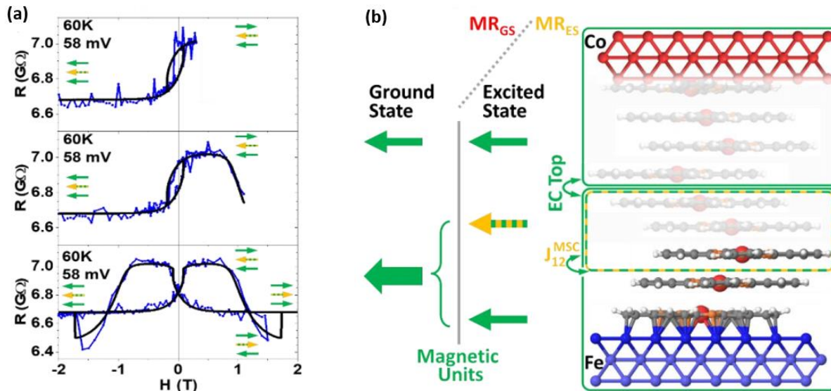
Figure 12. Magnétorésistance par retournement de spin. (a) Les mesures de magnéto-transport effectuées à T=60K et V=58mV révèlent trois commutations de résistance dues à l'inversion de magnétisation de trois unités magnétiques (flèches vertes et jaunes/vertes). (b) Schéma des unités magnétiques contribuant au MR_{GS} et au MR_{ES} . Dans l'état fondamental, la chaîne de spin moléculaire de CoPc forme une unité relativement plus dure avec l'interface Fe|CoPc et l'électrode inférieure de Fe (représentée par la grande boîte verte inférieure qui contient également une boîte verte/jaune), cependant, dans son état excité à spin inversé, la chaîne de spin moléculaire de CoPc agit comme une unité magnétique distincte (représentée par la boîte verte/jaune et la flèche) avec un champ coercitif et contribue uniquement au MR_{ES} . La partie imparfaitement contrôlée de la jonction apparaît semi-transparente. Les termes de couplage ECTop et J_{12}^{MSC} du modèle macrospin entre les unités centrales et supérieure/inférieure sont représentés. Voir les textes pour plus de détails. L'ajustement [représenté par la ligne noire dans le panneau (a)] a été effectué en utilisant les paramètres K_t/M_t=0.26T , \theta_{Mt}=60^\circ , K_b/M_b=4.95T , \theta_{Mb}=-4^\circ , ECTop=-0.05T , J_{12}^{MSC}=1.28T , R_0=6.68G\Omega , MR_{GS}=-2.4\% et MR_{ES}=5.1\% . [63]
