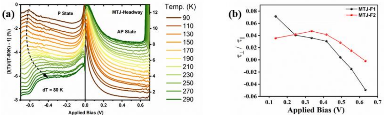
Figure 6. (a) Tracés \hat{I} plots calculés à partir de I(V) s consécutifs réalisés à \Delta T = T_2 - T_1 = 80K , à l'état P (à gauche) et à l'état AP (à droite) pour le dispositif MTJ-H. Le grand saut dans \hat{I}_{AP} ( V > 0 ) est dû à l'effet STT lui-même. (b) Rapport du couple hors plan sur le couple dans le plan (calculé à partir du rapport de torqance respectif) par rapport à la polarisation appliquée pour les dispositifs MTJ-F1 (noir) et MTJ-F2 (rouge).
