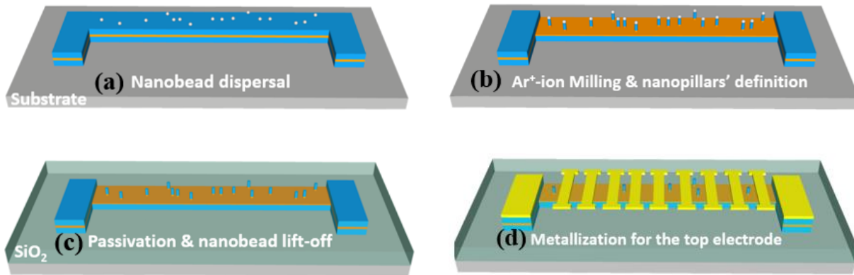
Figure 10. Présentation schématique du processus des nanobilles. (a) Étape I : dispersion de nanobilles de silice sur la surface supérieure de l'empilement de tricouches hybrides, ces nanobilles de silice servent de masque d'ombre pour l'étape II, (b) Étape II : étape de gravure par ions \text{Ar}^+ pour fabriquer les nanopiliers, (c) Étape III : étape de décollement des nanobilles et de passivation pour encapsuler les nanopiliers, (d) Étape IV : étape de métallisation pour déposer les électrodes supérieures.[63]
