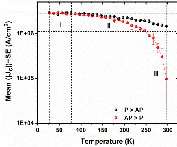
Figure 5. Tracé de la densité de courant critique |J_C| pour les dispositifs MTJ-F à (a) P > AP , (b) AP > P , commutation STT.
