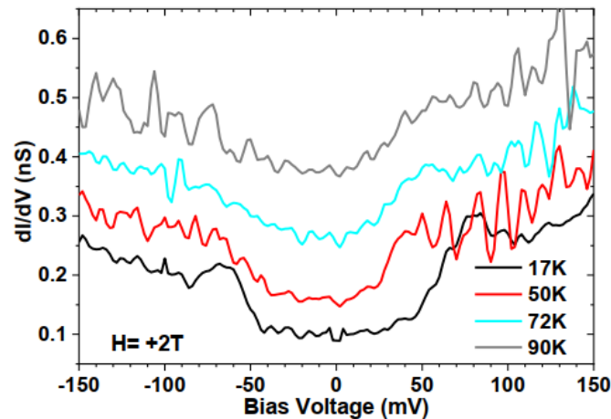
Figure 11. Excitation par retournement de spin. Données de conductance différentielle ou dI/dV(V) à H= +2T pour différents points de température (T) acquises pour la nanopillar de taille 500nm fabriquée à partir d'un empilement de Si|SiO x ||Cr(5)|Fe(50)|CoPc(20)|Co(10)|Cr(5).[63]
