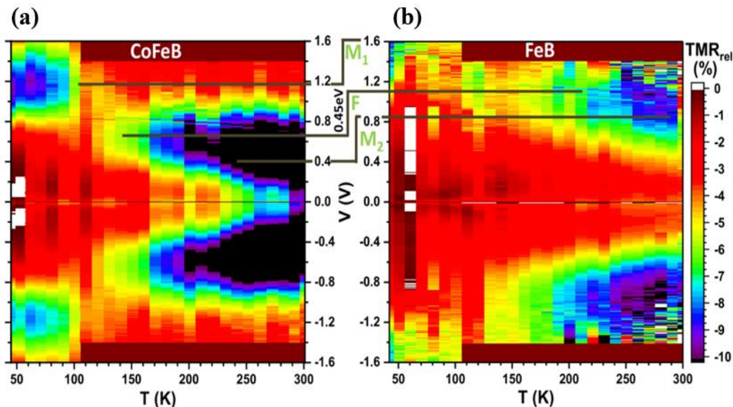
Figure 1. Tracés 3D de TMR rel pour les dispositifs MTJ avec l'électrode supérieure (a) CoFeB et (b) FeB. Les axes x, y et z représentent respectivement la température, la polarisation appliquée et l'amplitude du TMR rel . L'échelle de couleur représente l'axe z ou l'amplitude du TMR rel . Le déplacement de 0,45 eV dans les états occupés vers les valeurs d'énergie plus élevées par rapport à l'énergie de Fermi est évident lorsque l'électrode FM supérieure est remplacée par du FeB au lieu du FeCoB.[20]
