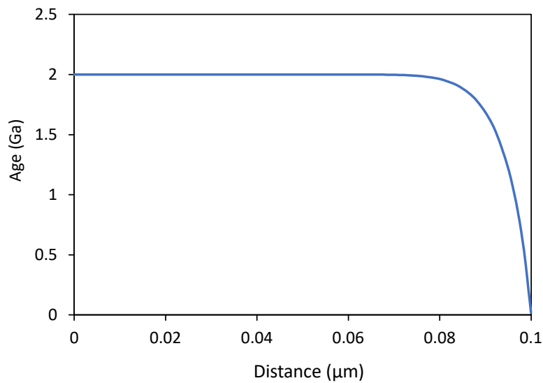
FIG. 8.5 – Profil cœur-bordure d'une phlogopite de 0.1mm de rayon ayant résidé à T = 1000^{\circ}\text{C} et P = 30 kbar pendant 2Ga. Elle préserve un âge moyen de 1.79 Ga.
