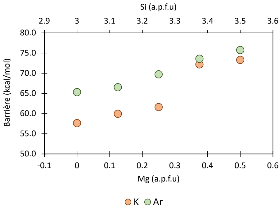
FIG. 6.5 – Variation des barrières de migration de l' 40 Ar et K en fonction de la concentration en Si et Mg.
