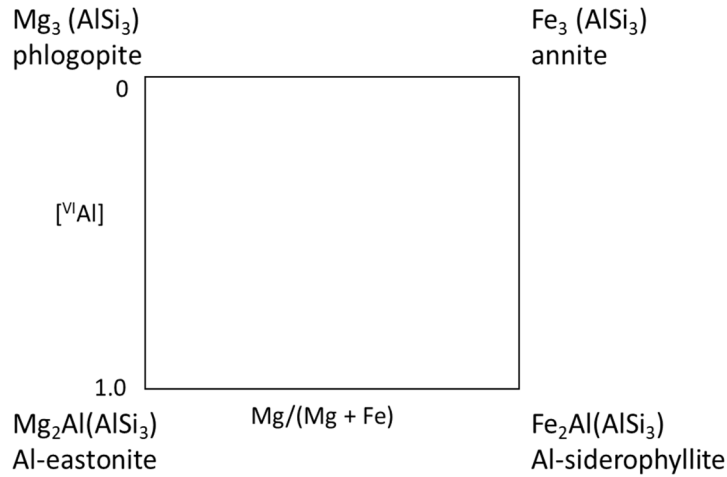
FIG. 2.11 – Plan idéal des biotites dans lequel les seules substitutions possibles sont Mg \leftrightarrow Fe^{2+} et la substitution de Tschermak : ^{VI}Al + ^{IV}Al \leftrightarrow (Fe^{2+}, Mg) + Si . Seuls les cations tétraédriques et octaédriques sont mentionnés dans les formules des pôles pures.
