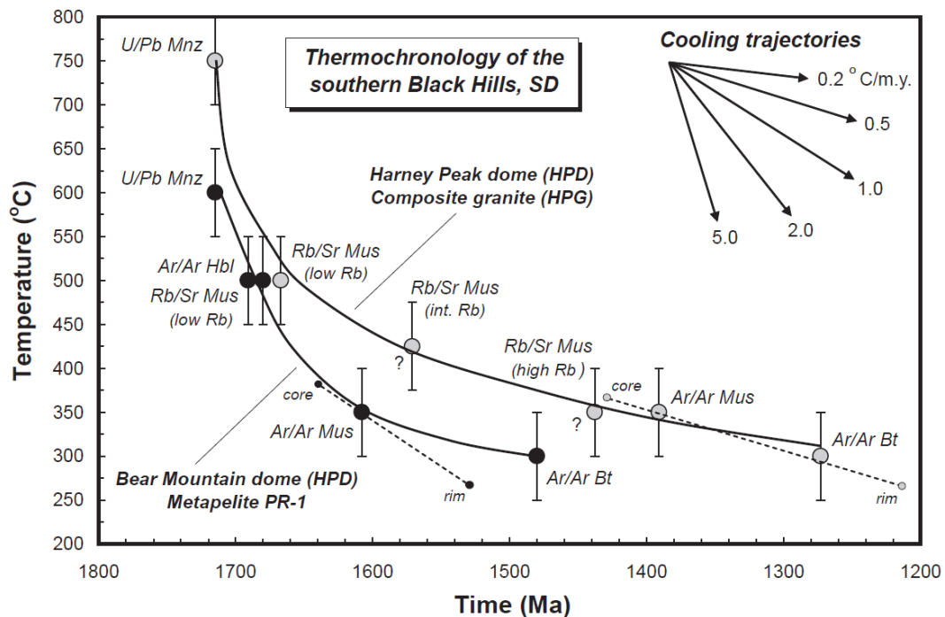
FIG. 3.2 – Histoire thermique post-magmatique de la partie sud des Black Hills reconstruite sur la base de plusieurs thermochronomètres. Le granite de Harney Peak s'est d'abord refroidi à une vitesse de 2 à 4 °C/Ma puis a connu un refroidissement lent de 0.5 à 0.1 °C/Ma (Dahl et Foland, 2008).
