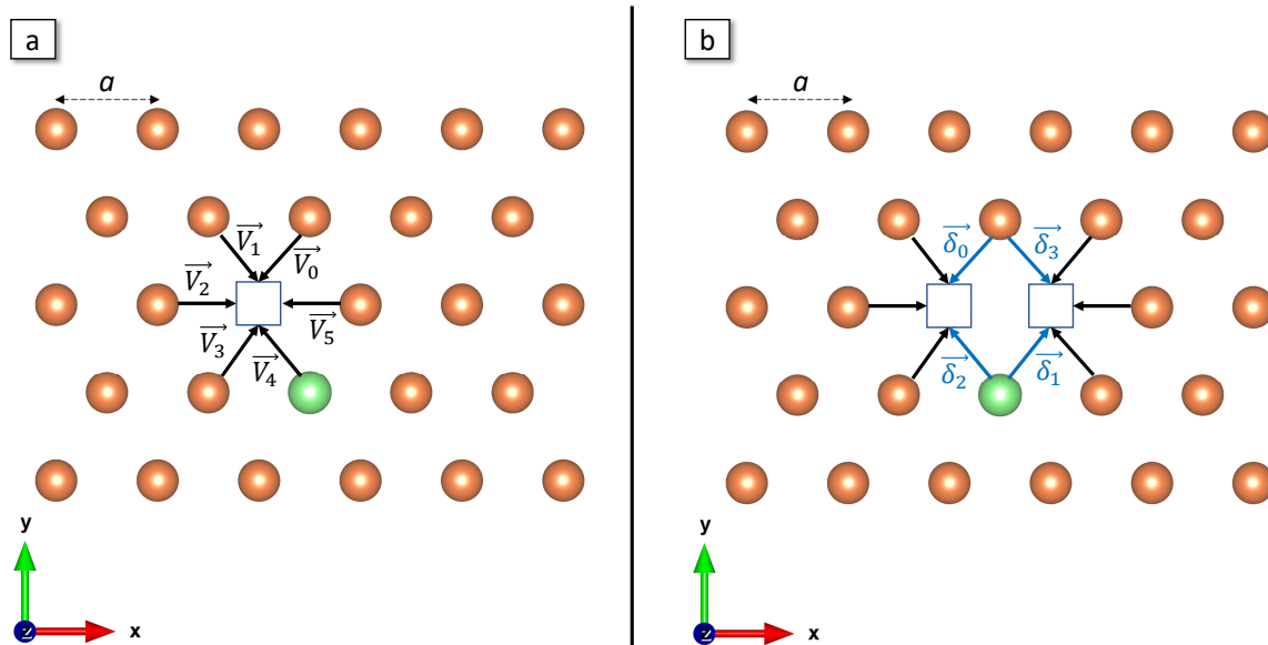
FIG. 5.7 – Géométrie de la diffusion lacunaire dans le plan interfoliaire. a) Diffusion via des lacunes simples. b) Diffusion via des lacunes doubles. Les cercles oranges et verts correspondent respectivement aux atomes de K et ^{40}\text{Ar} . \square représente la lacune, \vec{V}_i correspondent aux vecteurs déplacement et \vec{\delta}_i indique les migrations préservant les doubles lacunes.
