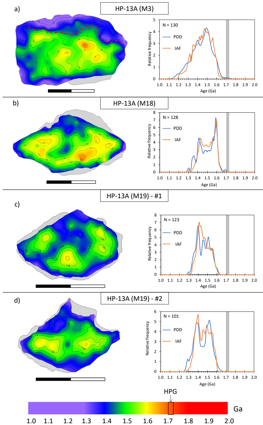
FIG. 3.6 – Cartographie in situ des âges ^{40}\text{Ar}/^{39}\text{Ar} dans les grains de l'échantillon HP-13A (pluton central). Tous les grains montrent un rajeunissement cœur → bordures et la présence des sous-domaines conservant des âges \geq 1.60 Ga. La ligne rouge tiretée délimite les délaminations périphériques. Les courbes PDD et IAF montrent des distributions similaires. La barre verticale grise représente l'âge de mise en place du HPG. La barre d'échelle est de 1 mm.
