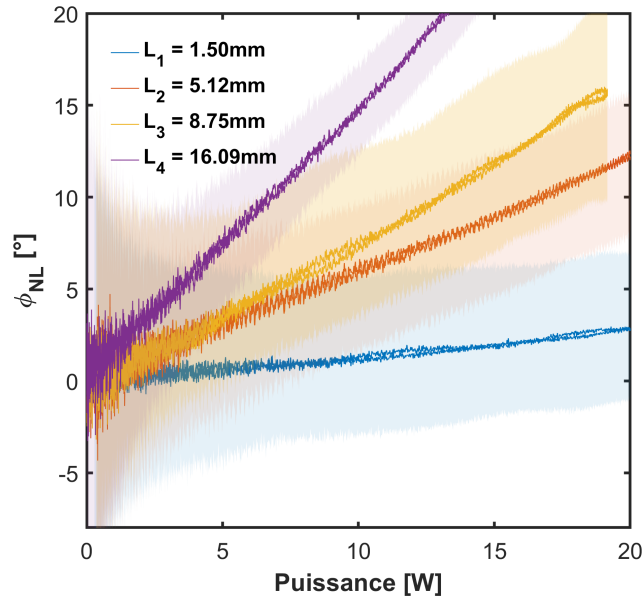
FIGURE 3.12 – Mesures non-linéaires pour des guides d’ondes de largeur w = 1,2 \mu\text{m} et de différentes longueurs, le déphasage non-linéaire est représenté en fonction de la puissance crête à l’intérieur du guide.
