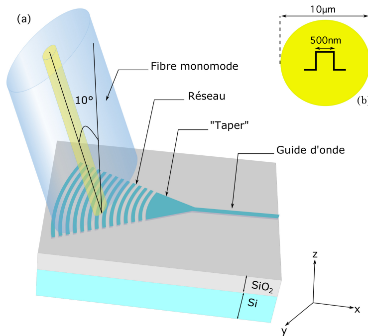
FIGURE 1.13 – Schéma représentatif du couplage par réseau. (a) Strucutre de réseau coupleur SOI, composé d'un réseau de diffraction et un "taper". La fibre optique injecte la lumière dans le guide d'onde ou la collecte. (b) Comparaison des dimensions du cœur d'une fibre SMF 28 et d'un guide d'onde.
