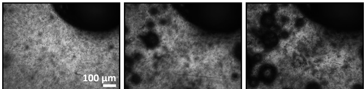
FIGURE 3.8 – Cliché expérimental d'une solution de SDS- CaCl 2 pour trois températures 50 °C, 60 °C et 70 °C. La concentration de CaCl 2 est 0,4 M/L et celle du SDS est de 1,7 mM/L. La turbidité observée est remarquablement marquée.
