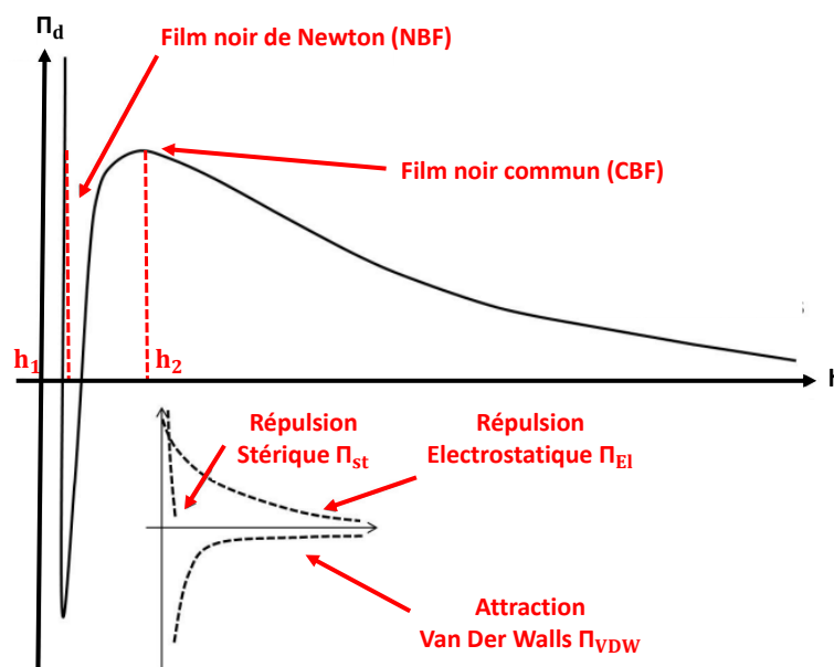
FIGURE 1.12 – Pression de disjonction en fonction de l'épaisseur d'un film. [71]
