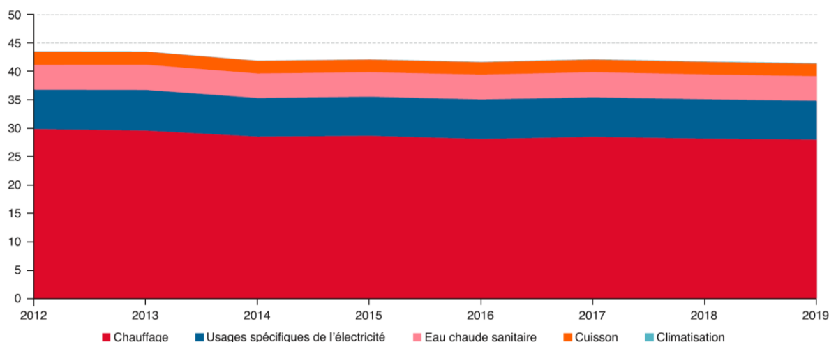
Figure I-4: Consommation finale énergétique du secteur résidentiel, par usage, France métropolitaine ( Bilan énergétique de la France pour 2019, 2021 )
