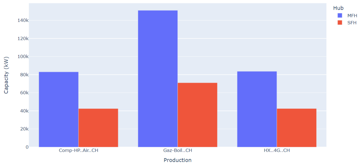
Figure V-43: Dimensionnement des composants de chauffage dans les bâtiments SFH et MFH – objectif exergétique – (SE, NR)
