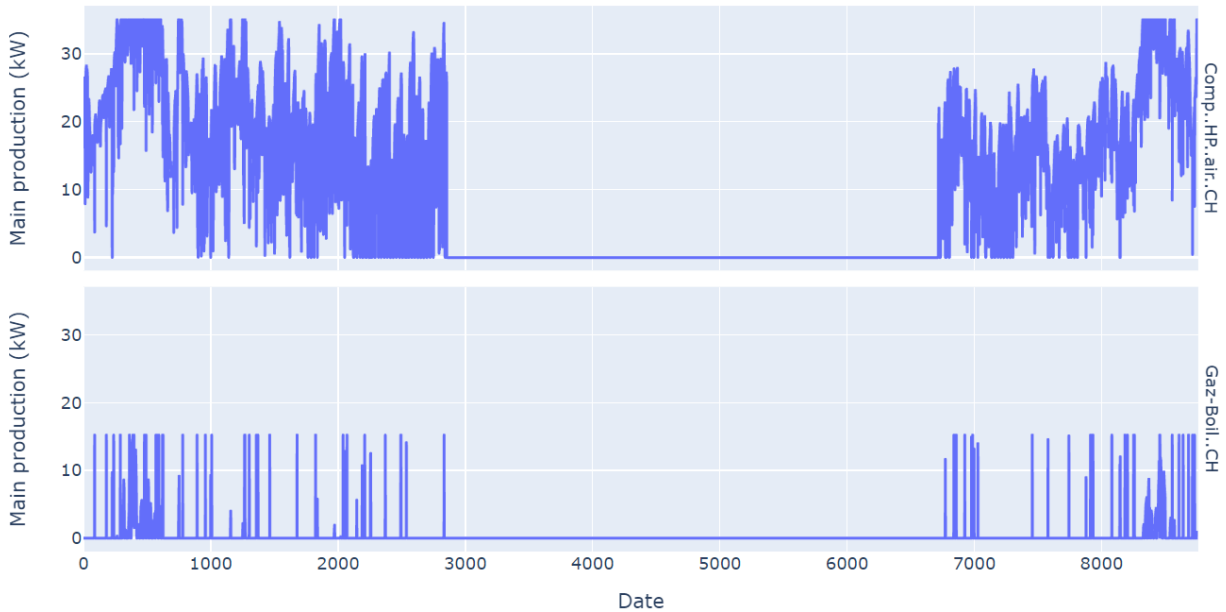
Figure II-11: Vérification modèle – répartition de la production entre PAC et chaudière gaz. En ordonnée, la puissance thermique utile.
