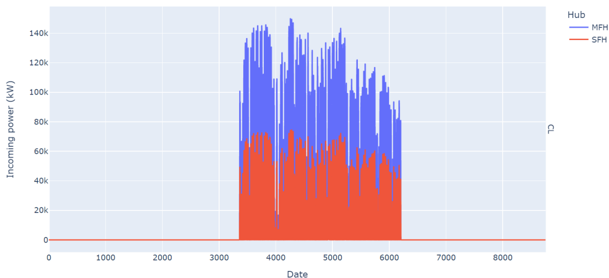
Figure V-46: Demande en climatisation des deux bâtiments SFH et MFH (SE, HR)
