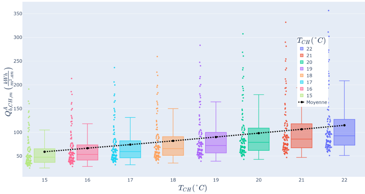
Figure IV-16 : Demande annuelle surfacique en chauffage selon la température de consigne, en Belgique
