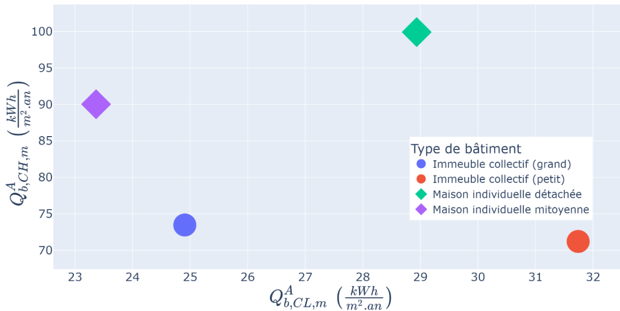
Figure IV-12: Demandes annuelles surfaciques en chauffage et en climatisation issues du modèle adapté, par taille de bâtiments. Tous pays confondus hors ES, BG et IT.
