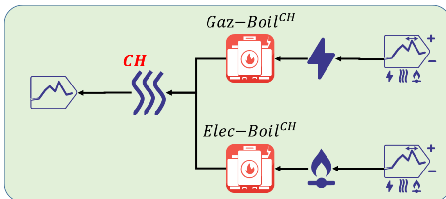
Figure V-23: Composants des hubs SFH et MFH en architecture NN (partie 2/2)
