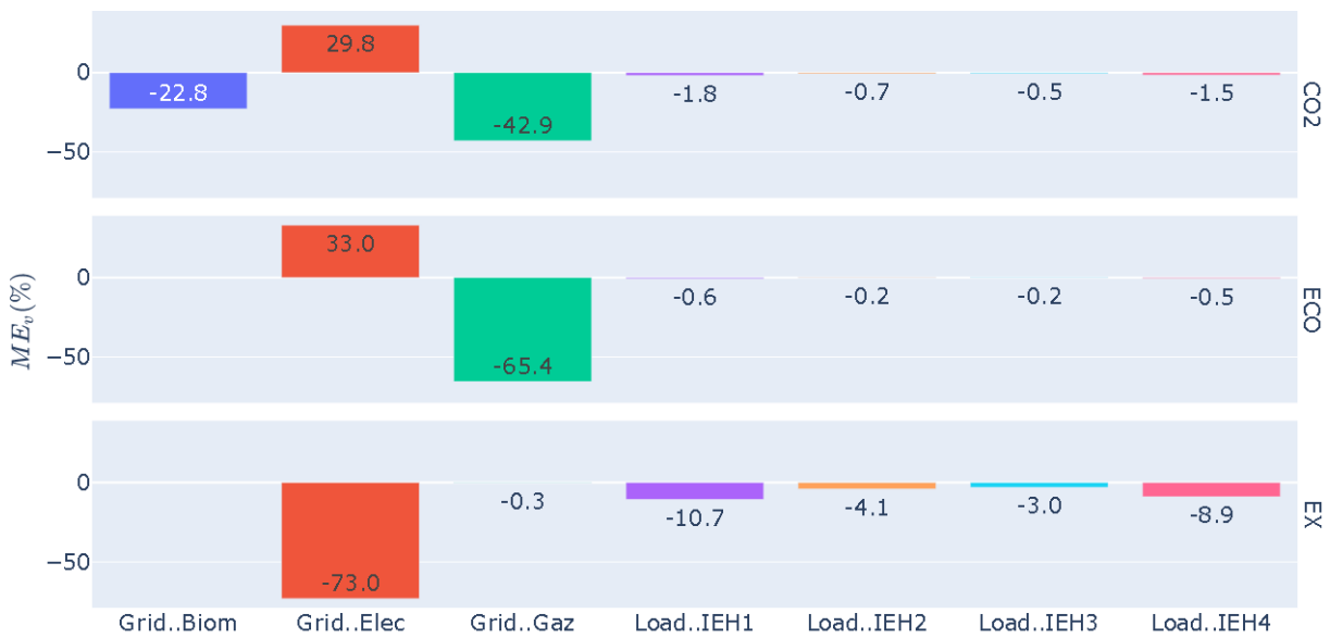
Figure V-33: Mix énergétique de la meilleure architecture thermique – par fonction objectif – (IT, NR)
