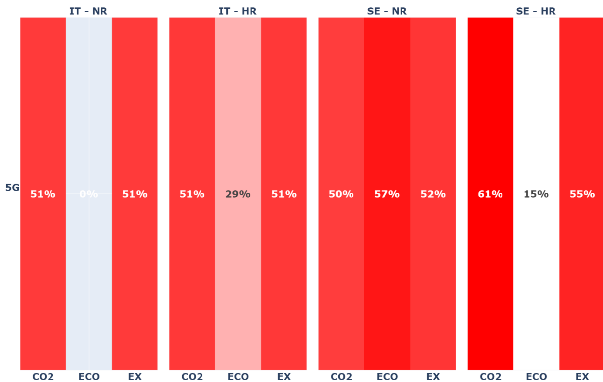
Figure IV-11: Facteur de charge annuel des composants Network en centrale CPP en fonction du couple (pays, scénario de rénovation) et de la fonction objectif – architecture NN_5G
