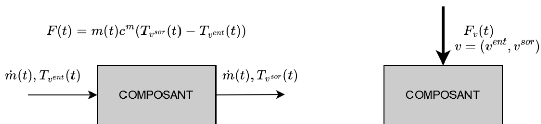
Figure II-5: Usage du vecteur thermique "en paire" v .
