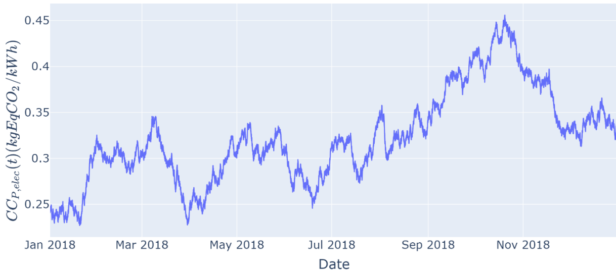
Figure II-16: Exemple avancé – facteur d'émission du vecteur électrique
