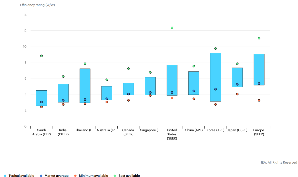
Figure 2: Performances des climatiseurs à compression sur le marché, par région du monde (International Energy Agency, 2020).
