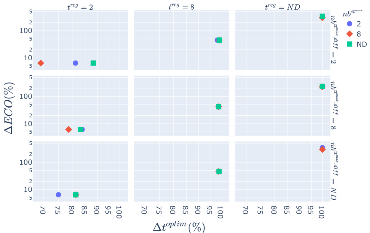
Figure III-13: Réduction temporelle – cas d'étude : compromis temps-précision des différents cas de supports réduits. Echelle logarithmique en abscisses et en ordonnées.
