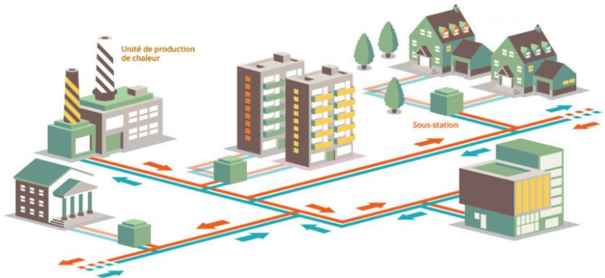
Figure 3: Schéma de principe d'un RDC (ADEME, 2022)
