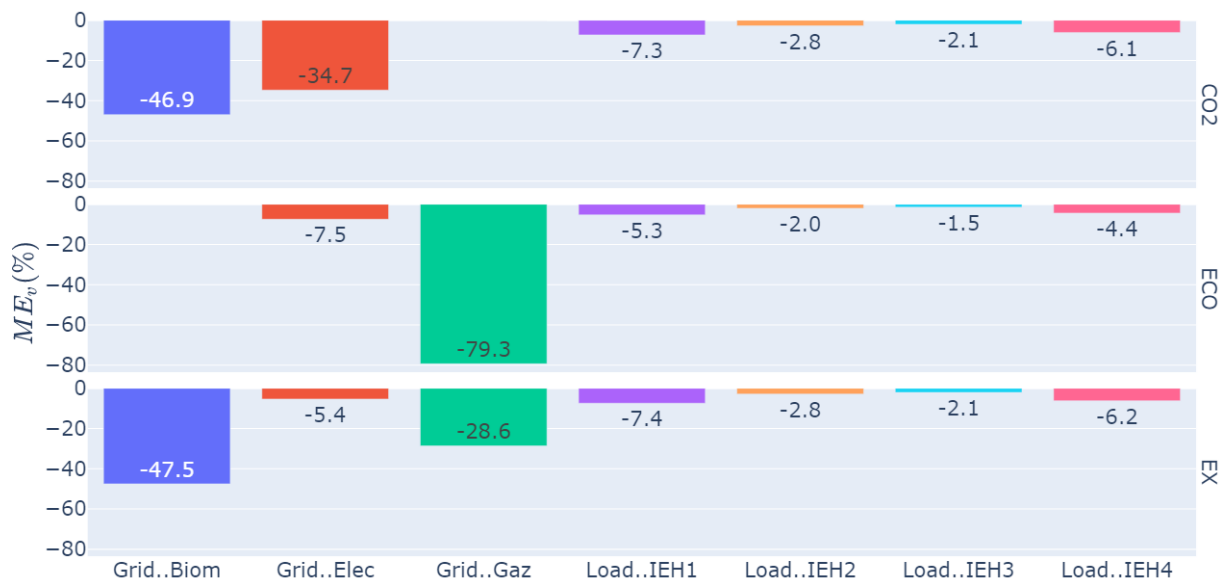
Figure V-42: Mix énergétique de la meilleure architecture thermique – par fonction objectif – (SE, NR)
