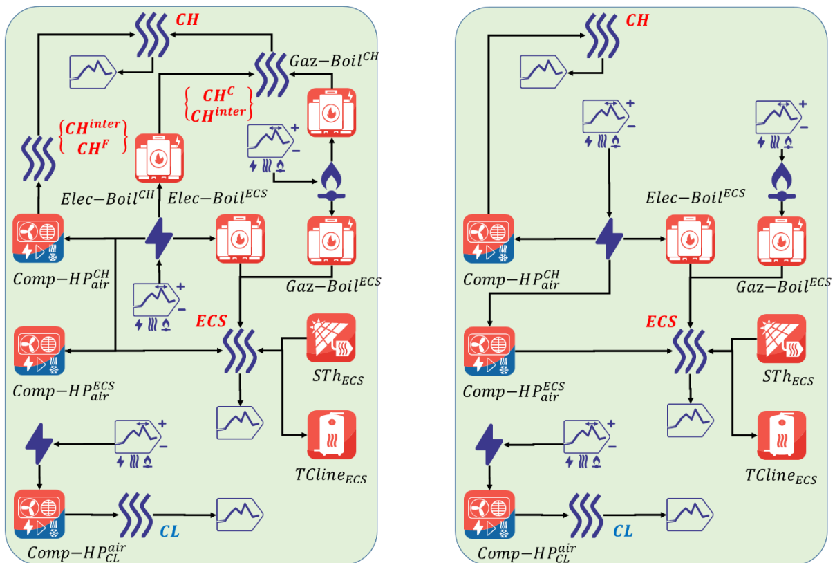
Figure V-22: Composants des hubs SFH et MFH en architecture NN (partie 1/2). A gauche, scénario r = NR . A droite, scénario r = HR .
