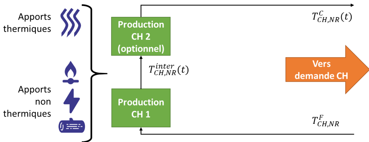
Figure V-9: Agencement des composants CH en local technique de bâtiment non rénové
