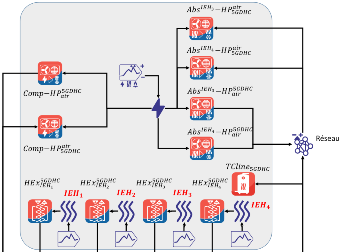
Figure V-18: Composants du hub CPP en architecture 5GDHC
