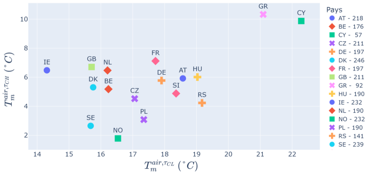
Figure IV-10: Températures moyennes de l'air dans le modèle adapté, par saison. En légende, associée au pays, la durée de la saison de chauffe en jours.
