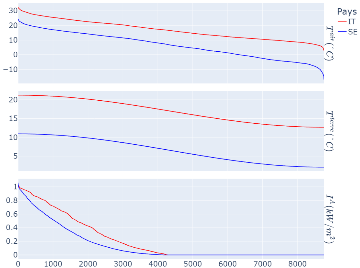
Figure III-1: Données météorologique
