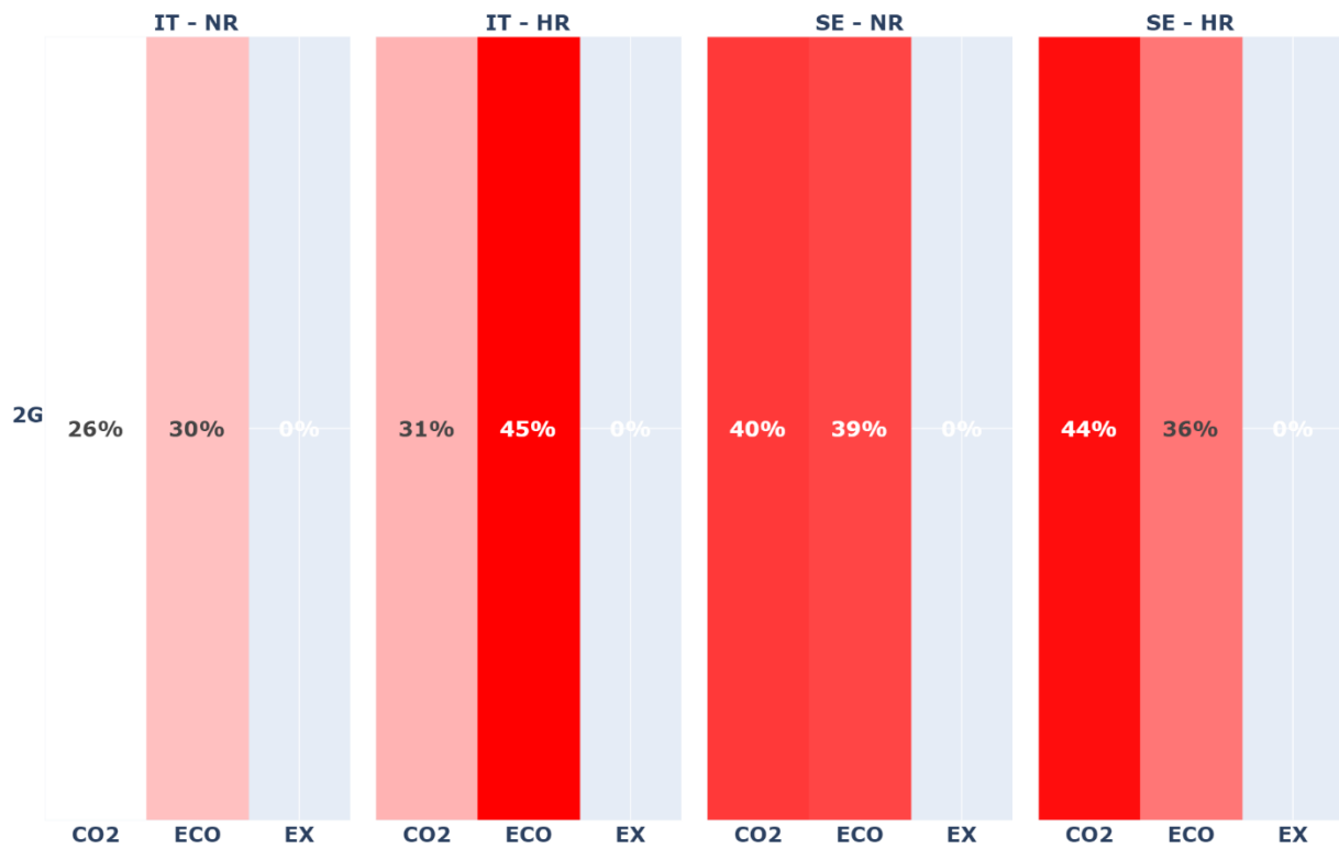
Figure IV-10: Facteur de charge annuel des composants Network en centrale CPP en fonction du couple (pays, scénario de rénovation) et de la fonction objectif – architecture NN_2G
