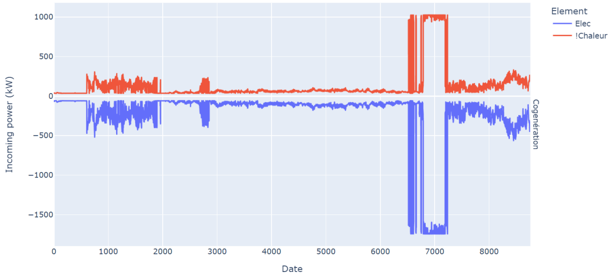
Figure II-19: Exemple avancé – productions de l'unité de cogénération
