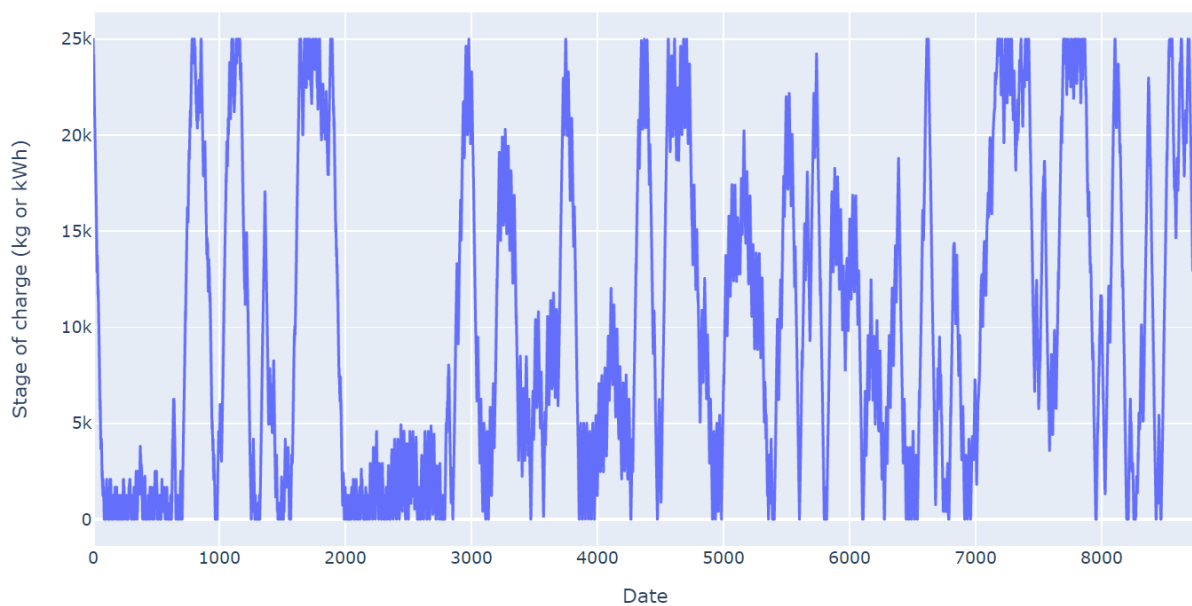
Figure II-21: Exemple avancé – évolution de l'état de charge du stockage de chaleur
