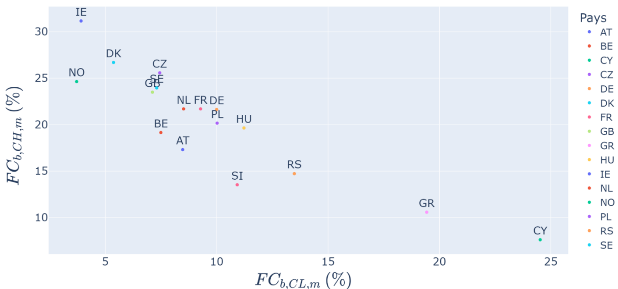
Figure IV-13: Facteurs de charge en chauffage et en climatisation, par pays
