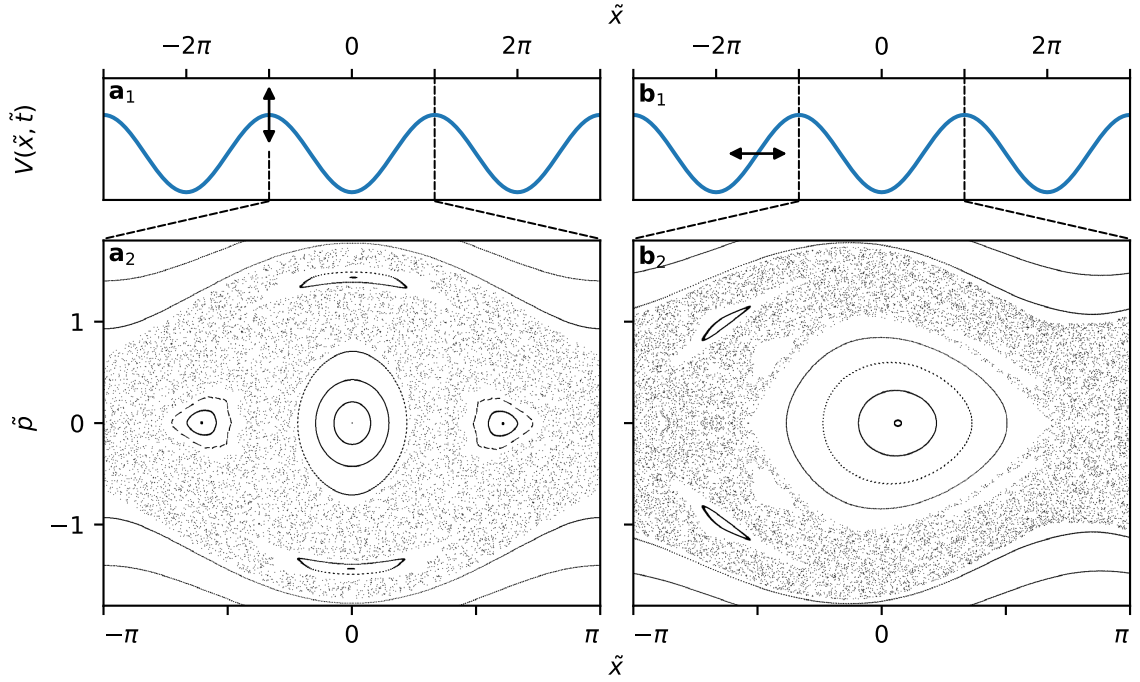
Figure F.1 | Exemples de portraits de phase stroboscopiques. En haut : potentiels sinusoidaux, modulés périodiquement dans le temps, représentés sur trois périodes spatiales. En bas : portraits de phase stroboscopiques correspondants, représentés sur une période spatiale. (a) Modulation de l’amplitude du potentiel, une configuration associée aux Éqs. (F.1) et (F.2), avec les paramètres de modulation \gamma = 0.375 , \varepsilon_0 = 0.24 et un temps de référence pour l’observation sous-stroboscopique \tilde{t}_0 = 0 . (b) Modulation de la phase du potentiel, associée aux Éqs. (F.1) et (F.3), avec \gamma = 0.44 , \varphi_0 = 2\pi/24 = 15^\circ et \tilde{t}_0 = 0 . Les grandeurs “tildées” adimensionnées et le paramètre \gamma sont obtenus à partir des grandeurs dimensionnées en suivant la procédure résumée p. 34.
