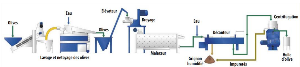
Figure 3: exemple de chaîne continue d'extraction de l'huile d'olive (Ministère de l'agriculture. 2006)
