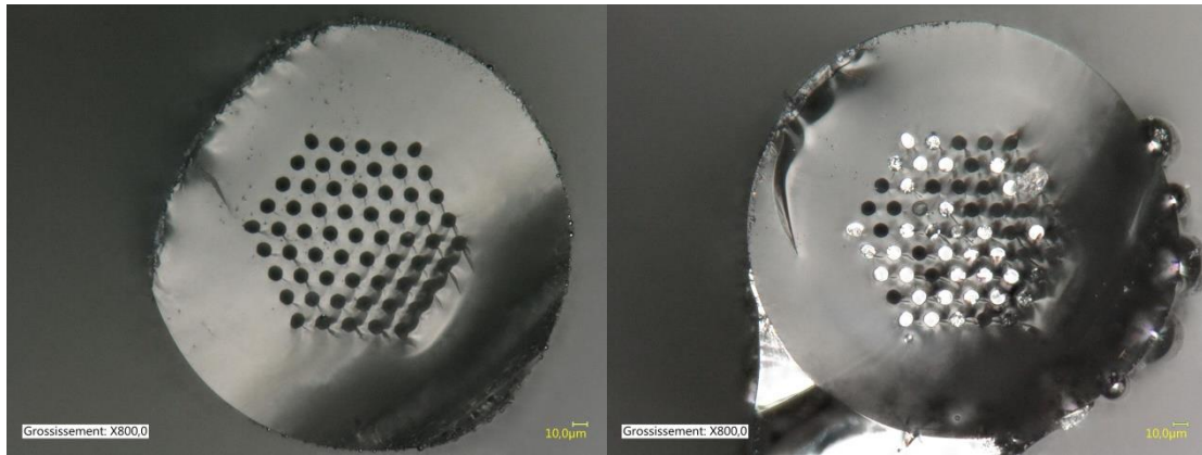
Figure 9: section de fibre en silice microstructurées avant et après remplissage des trous par le verre de chalcogénures
