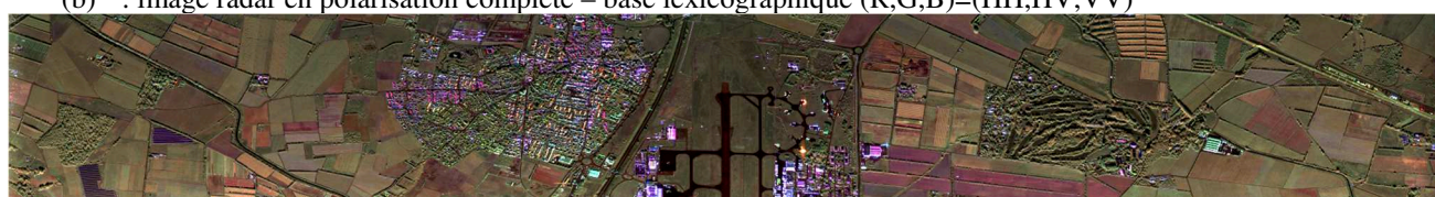
Fig. 13 : Image radar en (a) polarisation unique et en polarisation complète avec représentation en fausses couleurs dans la base (b) lexicographique et (c) de Pauli – Images SAR ONERA/SETHI
