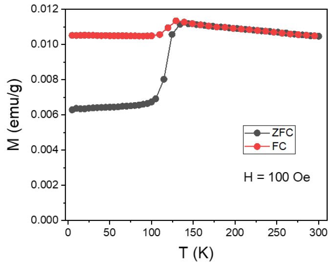
FIGURE IV.7 – Courbes d'aimantation en fonction de la température pour l'échantillon \text{CuFeS}_2 mesurées selon le protocole ZFC-FC sous H=100 Oe pour l'échantillon \text{CuFeS}_2 .
