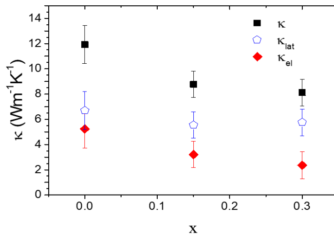
FIGURE V.10 – Conductivité thermique \kappa des composés Co_{1-x}Fe_xS_2 en fonction de x . Les parties élec-tronique \kappa_{el} et réseau \kappa_{lat} ont été calculées à partir de la loi de Wiedemann – Franz [11].
