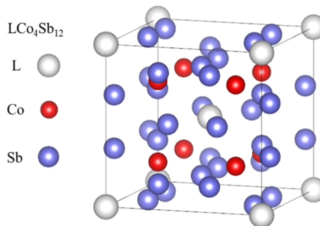
FIGURE I.7 – Structure cristallologique de la phase LCo_4Sb_{12} où L représente une lacune.
