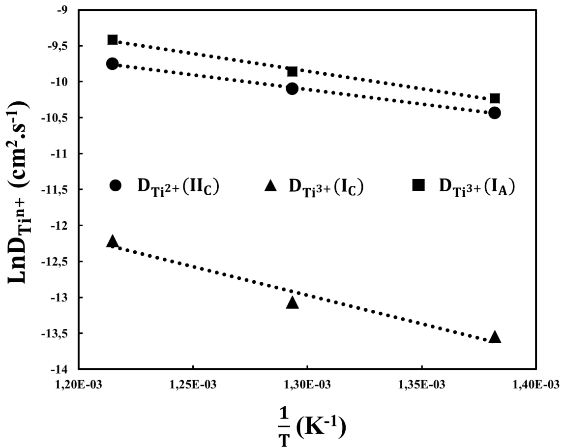
Figure IV-13 : courbes \ln D = f\left(\frac{1}{T}\right) pour la gamme de température 450 – 550 °C.
