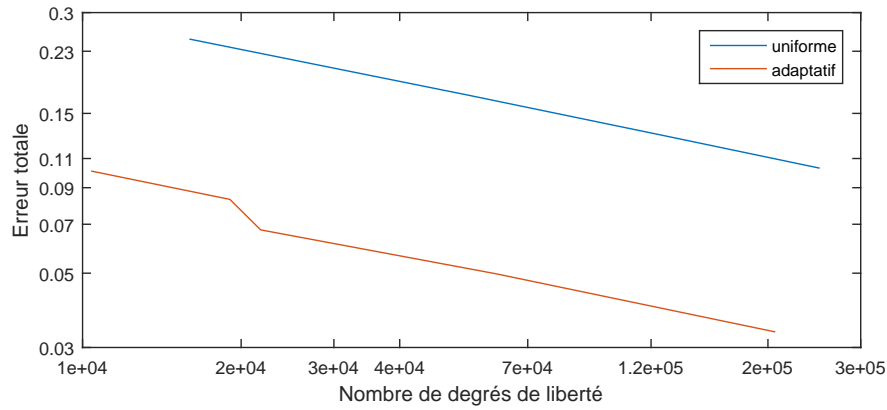
FIGURE 4.13 – Courbe d’erreur totale en échelle logarithmique du cas étudié.
