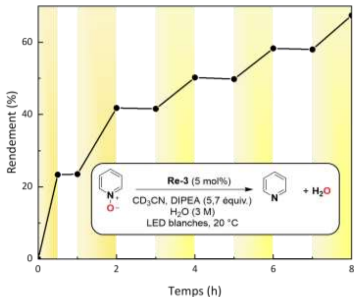
Figure 18 : Etude de l'effet de l'irradiation sur la conversion de 1a – conditions : oxyde de pyridine (100 \mu\text{mol} ), Re-3 (5 \mu\text{mol} ; 5 mol%), DIPEA (570 \mu\text{mol} ; 5,7 équiv.), \text{CD}_3\text{CN} (0,5 mL), 20 °C. Jaune : LED blanc froid, blanc : le tube est conservé dans le noir. Les rendements sont déterminés par analyse RMN ^1\text{H} du brut réactionnel.
