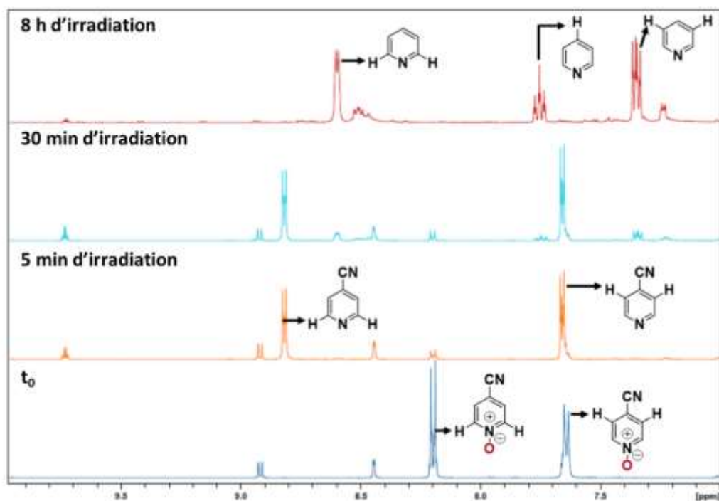
Figure 20 : Réduction et dégradation du dérivé nitrile 1f – conditions : 1f (100 \mu mol), Re-3 (5 \mu mol ; 5 mol%), DIPEA (570 \mu mol ; 5,7 équiv.), CD 3 CN (0,5 mL), LEDs blanc froid, 20 ^\circ C.
