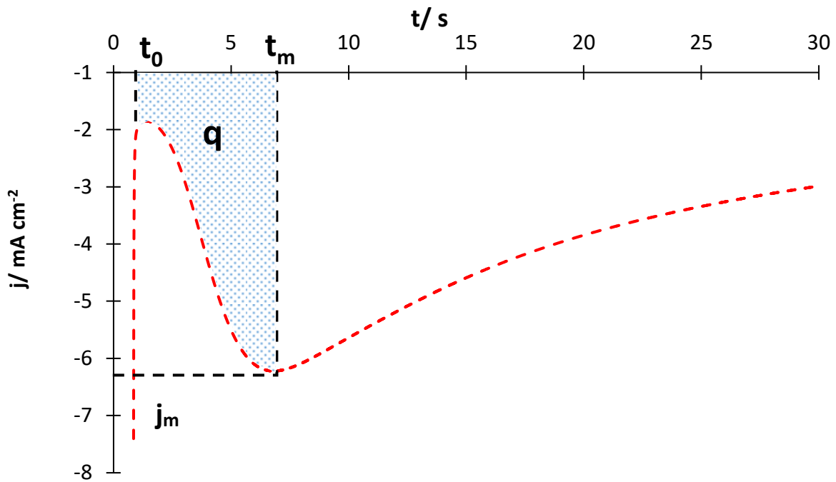
Figure III.8 : Exemple de chronoampérogramme illustrant l'aire sous la courbe entre t_0 et t_m permettant le calcul de la charge optimale
