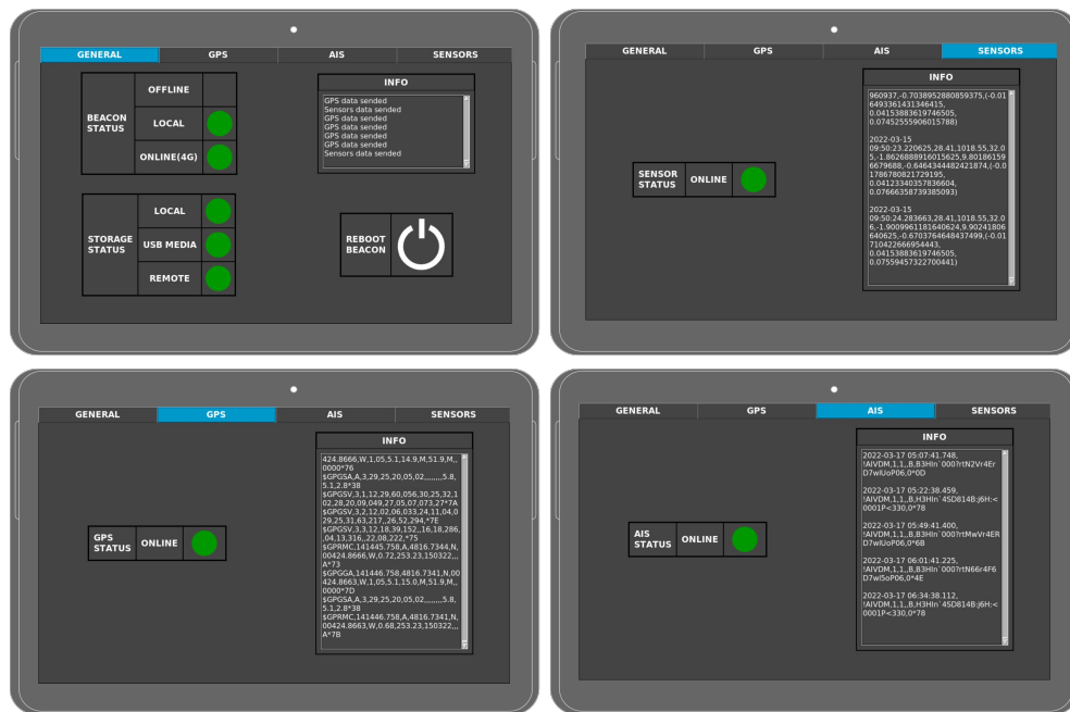
FIGURE V.14 – Exemples d’IHM développées et dédiées aux opérations à bord pour la balise embarquée HAPPINESS.
