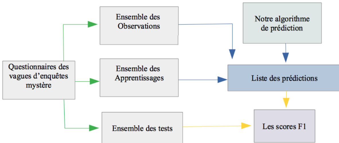
FIGURE 4.10 – Processus d'amélioration de la prédiction
