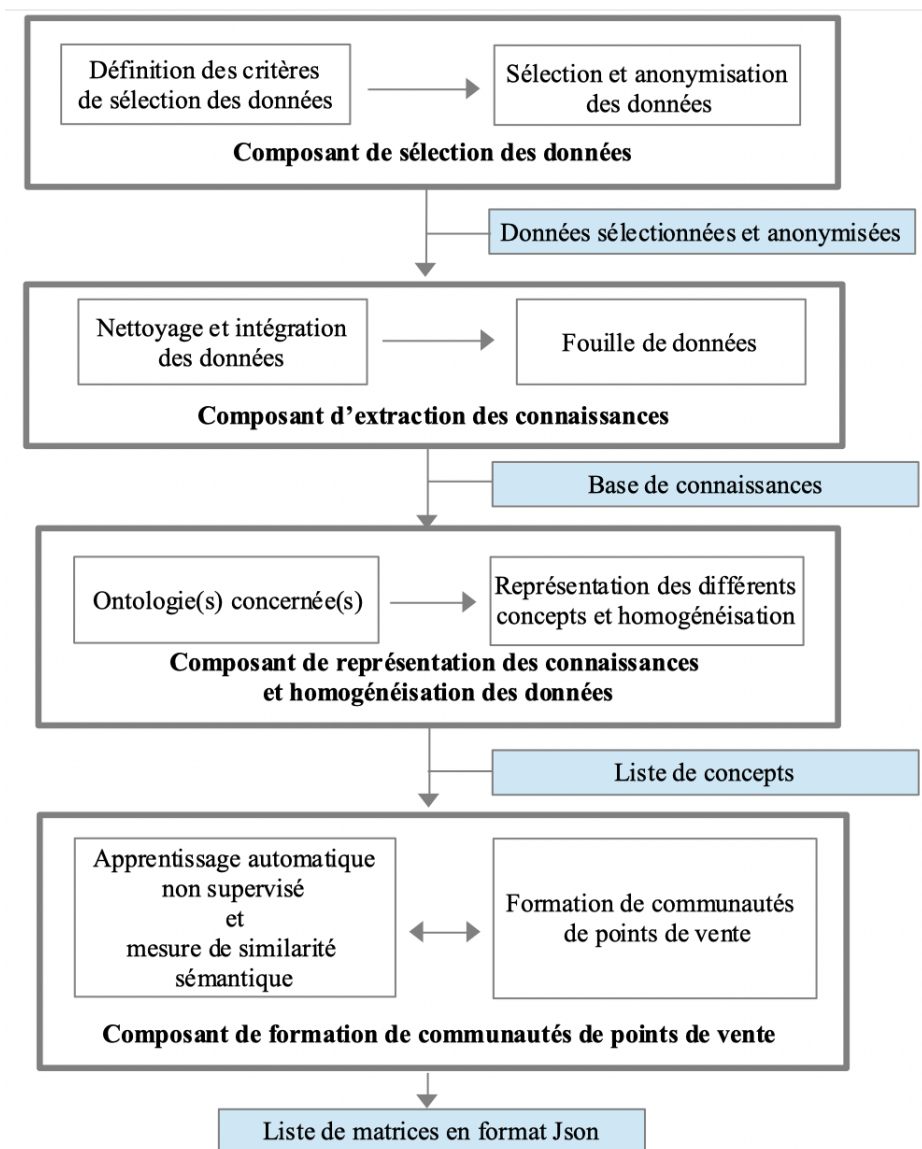
FIGURE 3.6 – Architecture globale détaillé du MoPRD
