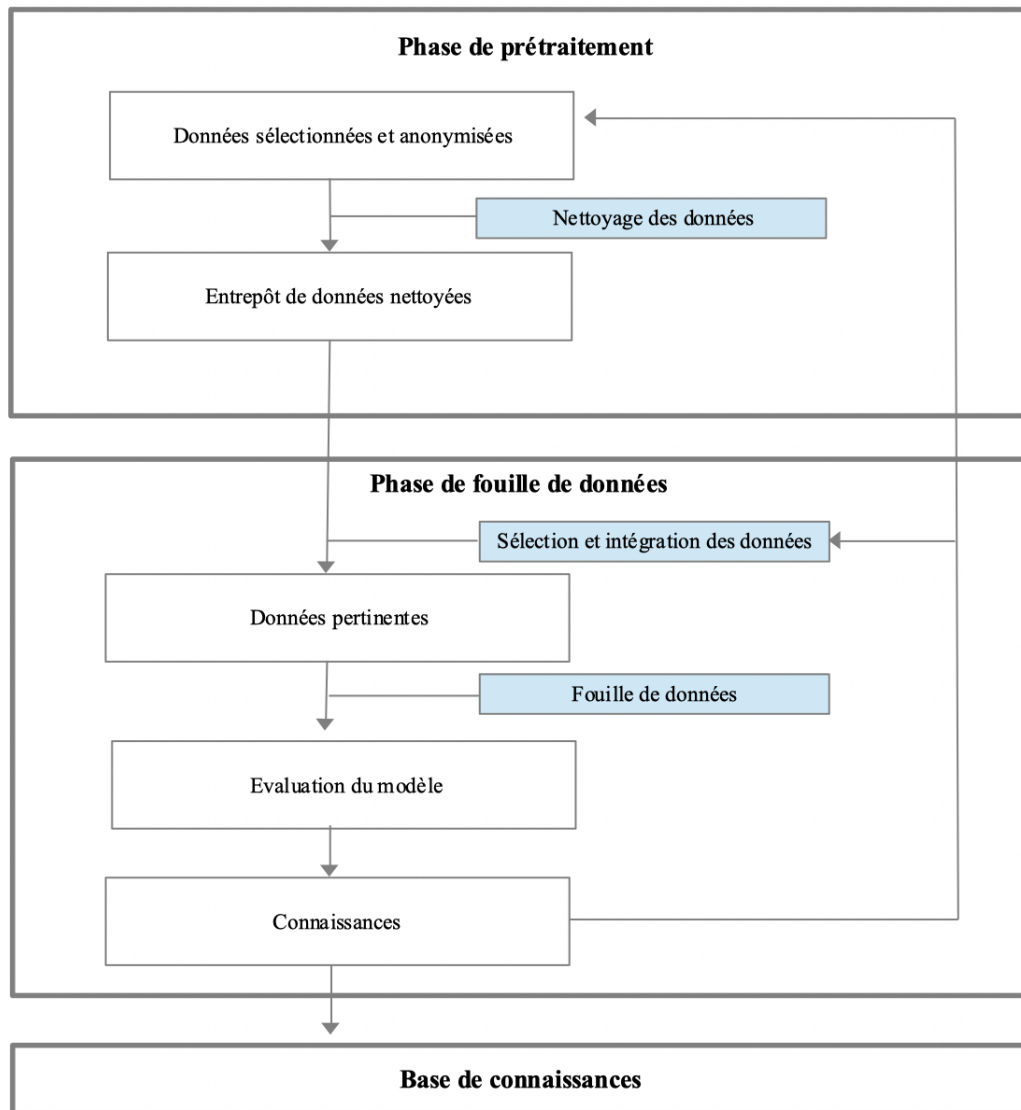
FIGURE 3.4 – Processus d’ECD
