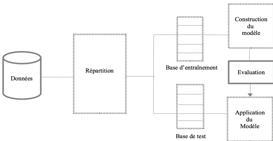
FIGURE 3.9 – Découpage des données par validation croisée
