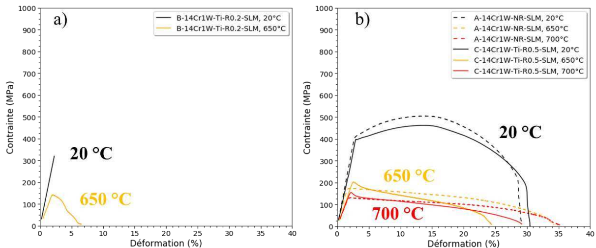
Figure V-5 : Courbes conventionnelles de traction à 20 °C et 650 °C de l'acier ODS B-14Cr1W-Ti-R0.2-SLM (a), et à 20 °C, 650 °C et 700 °C des aciers ODS C-14Cr1W-Ti-R0.5-SLM et non renforcé A-14Cr1W-NR-SLM (b).
