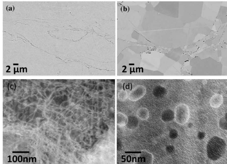
Figure I-31 : Images MEB du dépôt de poudre 14YWT obtenue par procédé GARS avant (a) et après recuit (b), et images MET de ce même dépôt avant (c) et après (d) recuit [196].
