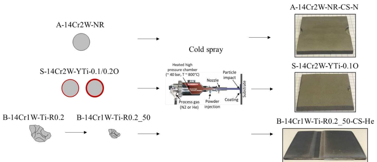
Figure IV-14 : Illustration des poudres et matériaux cold spray étudiés dans cette section.
