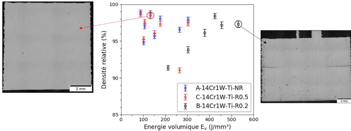
Figure III-2 : Densités relatives des pièces consolidées par SLM en fonction de E_{v,d} .
