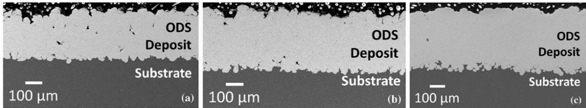
Figure I-30 : Image MEB d'une découpe transverse des dépôts de poudre d'acier ODS 14YWT obtenue par procédé GARS, projetée avec un gaz vecteur (a) 100% N 2 , (b) 50% N 2 - 50% He, (c) 5% N 2 - 95% He [196].
