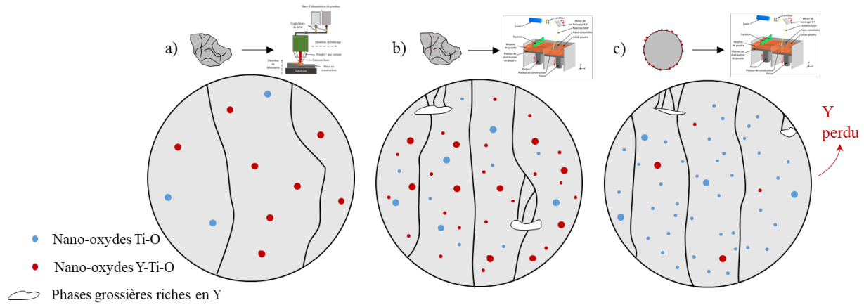
Figure IV-13 : Schéma de la microstructure des aciers ODS élaborés en DMD à partir de la poudre co-broyée (a), en SLM à partir de la poudre co-broyée (b), et en SLM à partir de la poudre composite (c).
