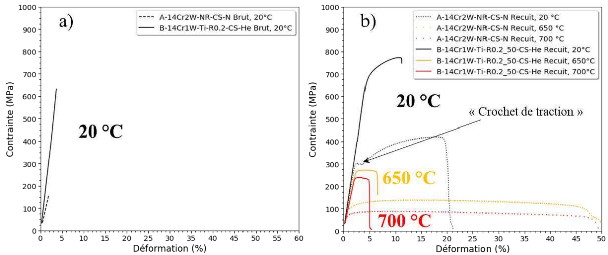
Figure V-8 : Courbes conventionnelles de traction de l'acier ODS B-14Cr1W-Ti-R0.2_50-CS-He et de l'acier non renforcé A-14Cr2W-NR-CS-N , bruts de dépôt à 20 °C (a), et après un recuit à 1100 °C pendant 30 minutes à 20 °C, 650 °C et 700 °C (b).
