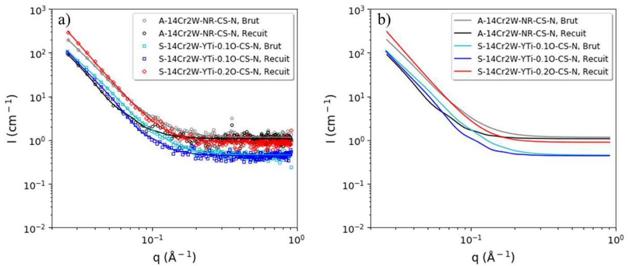
Figure IV-15 : Signaux SAXS expérimentaux et ajustés (a), et ajustés seuls (b) des aciers obtenus par cold spray à partir des poudres non renforcées et ODS STARS fournies par CEIT ( A-14Cr2W-NR et S-14Cr2W-YTi-0.1/0.2O ).
