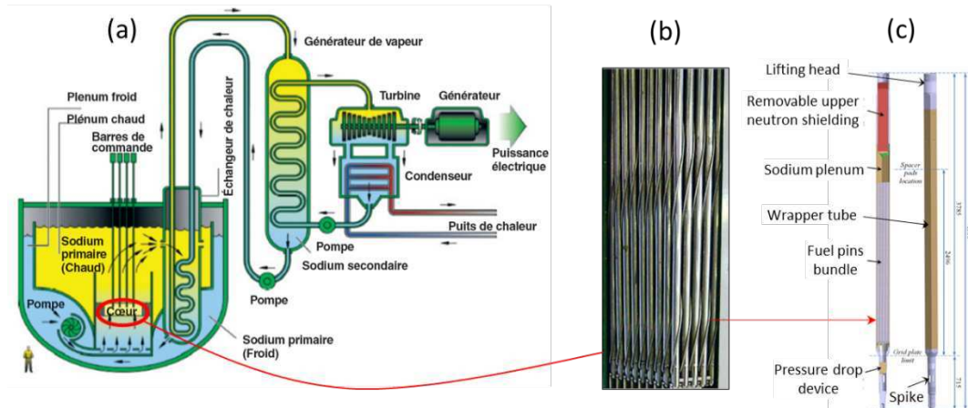
Figure I-2 : Schéma d'un RNR-Na (a), photographie d'un assemblage d'aiguilles de combustibles du réacteur PHENIX (b) [2], schéma de conception d'une aiguille de combustible pour Astrid (c) [4].
