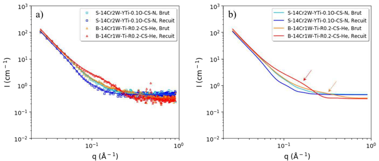
Figure IV-16 : Signaux SAXS expérimentaux et ajustés (a), et ajustés seuls (b) des aciers obtenus par cold spray à partir de la poudre co-broyée ( B-14Cr1W-R0.2_50 ) et STARS ( S-14Cr2W-YTi-0.1 ).
