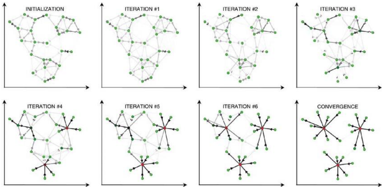
Figure 2.11 Exemple d'exécution de l'algorithme propagation d'affinité d'affinité [Torrent-Fontbona et al. , 2012]
