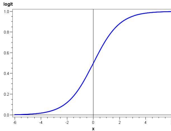
Figure 3.9 Courbe représentative de la fonction Sigmoïde
