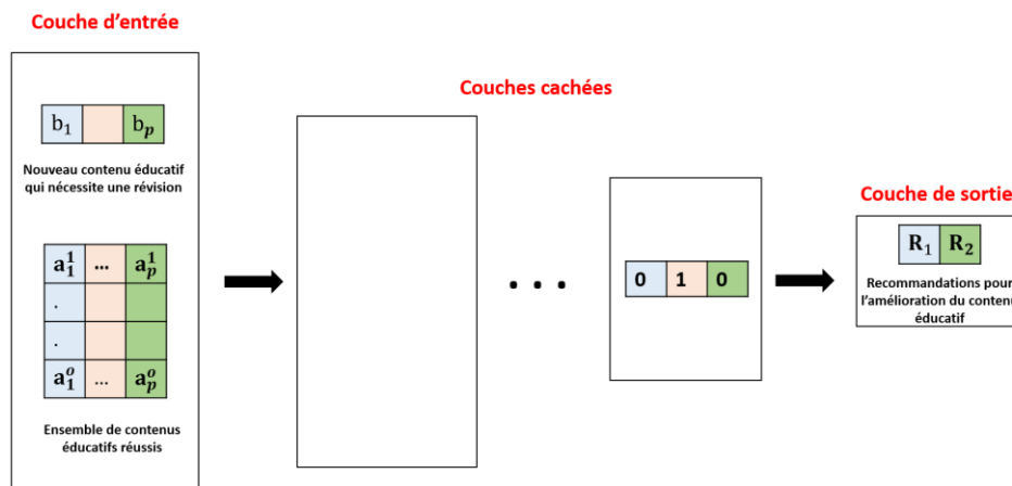
Figure 5.2 Approche basée sur l'apprentissage profond pour la recommandation des améliorations des contenus éducatifs en ligne
