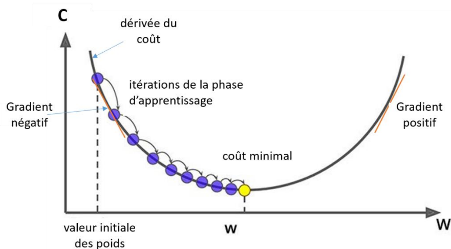
Figure 2.8 Apprentissage avec la descente de gradient
