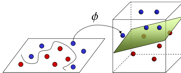
Figure 2.10 Projection des données en dimension 3 [Yue et al., 2010]
