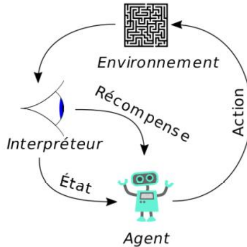
Figure 2.3 Scénario typique de l'apprentissage par renforcement [ Reinforcement Learning, 2017 ]
