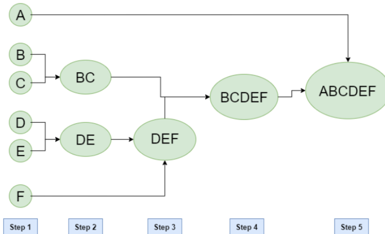
Figure 2.12 Exemple d'exécution de l'algorithme de regroupement aggloméré [Nawrin et al., 2017]
