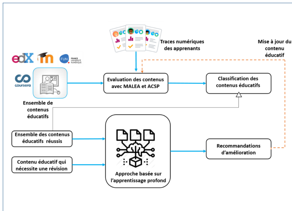
Figure 5.1 Approche basée sur l'apprentissage profond pour la recommandation d'amélioration des contenus éducatifs en ligne
