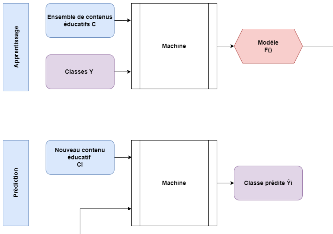
Figure 3.4 Formulation du problème de prédiction de la réussite des contenus éducatifs en ligne
