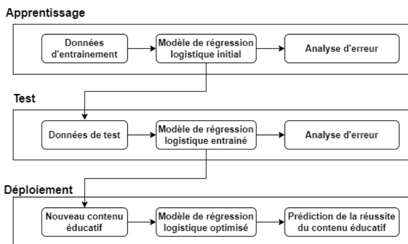
Figure 3.8 Architecture hiérarchique de la prédiction des contenus éducatifs en ligne
