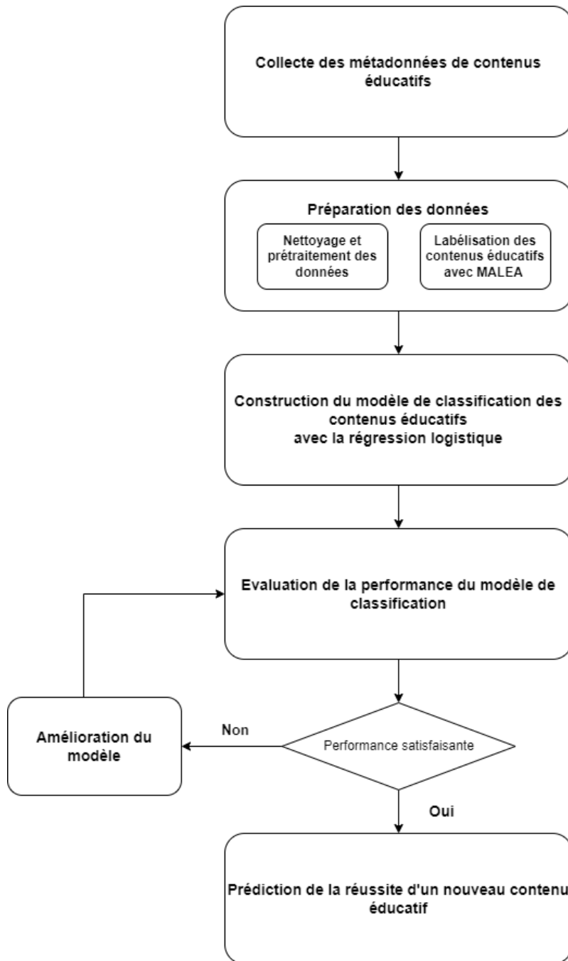
Figure 3.6 Processus de l'approche ACSP
