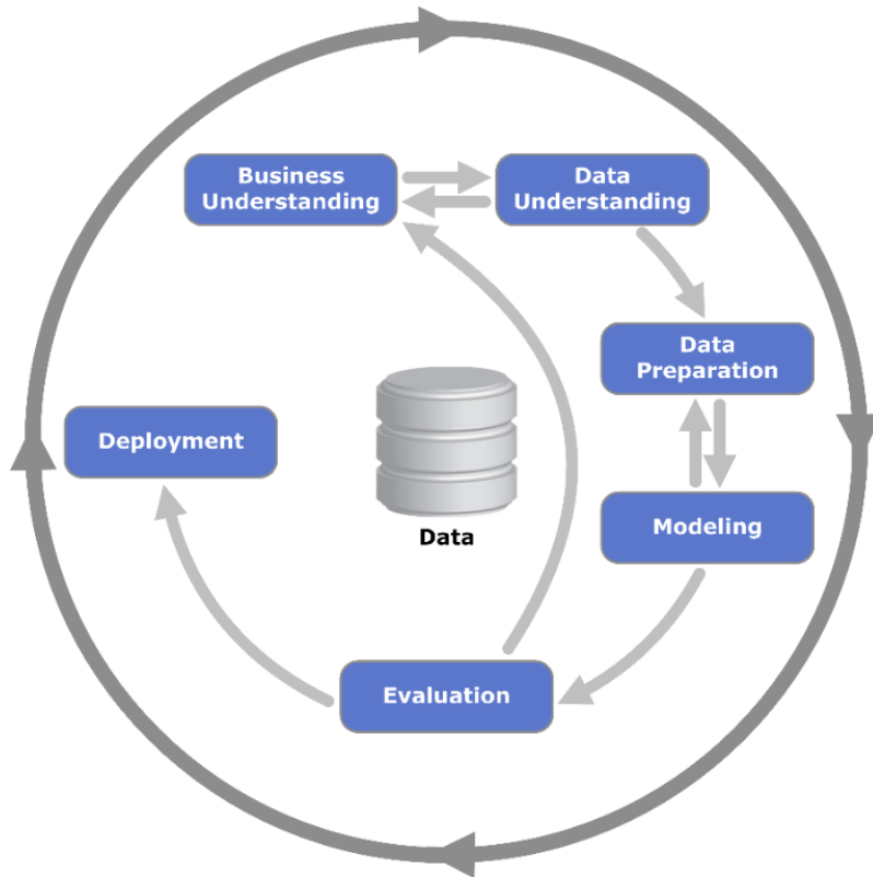
Figure 6.1 Illustration de la méthode CRISP
