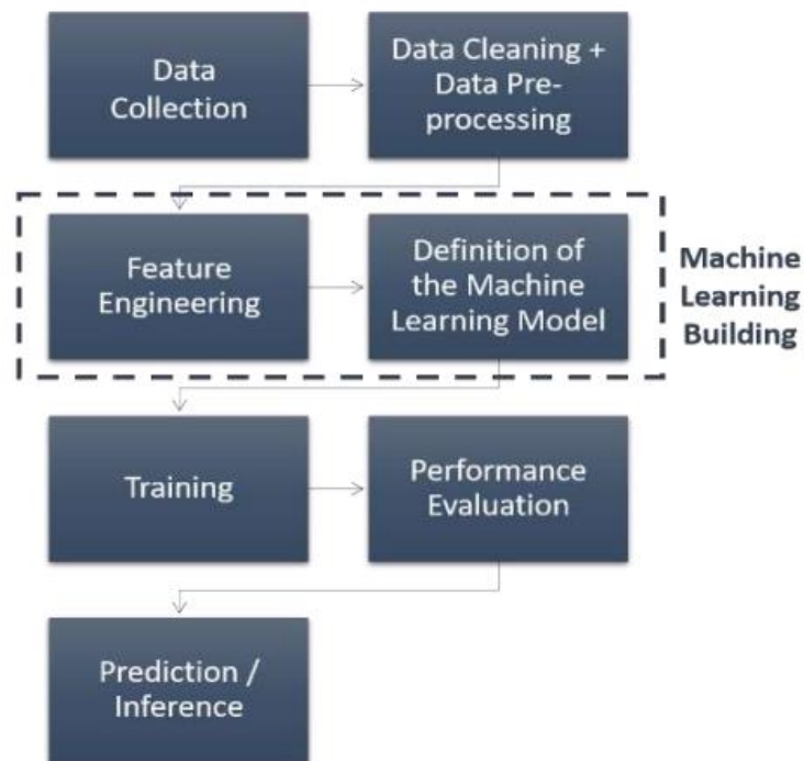
Figure 2.4 Processus général d'apprentissage automatique [Mourali et al. , 2020b]
