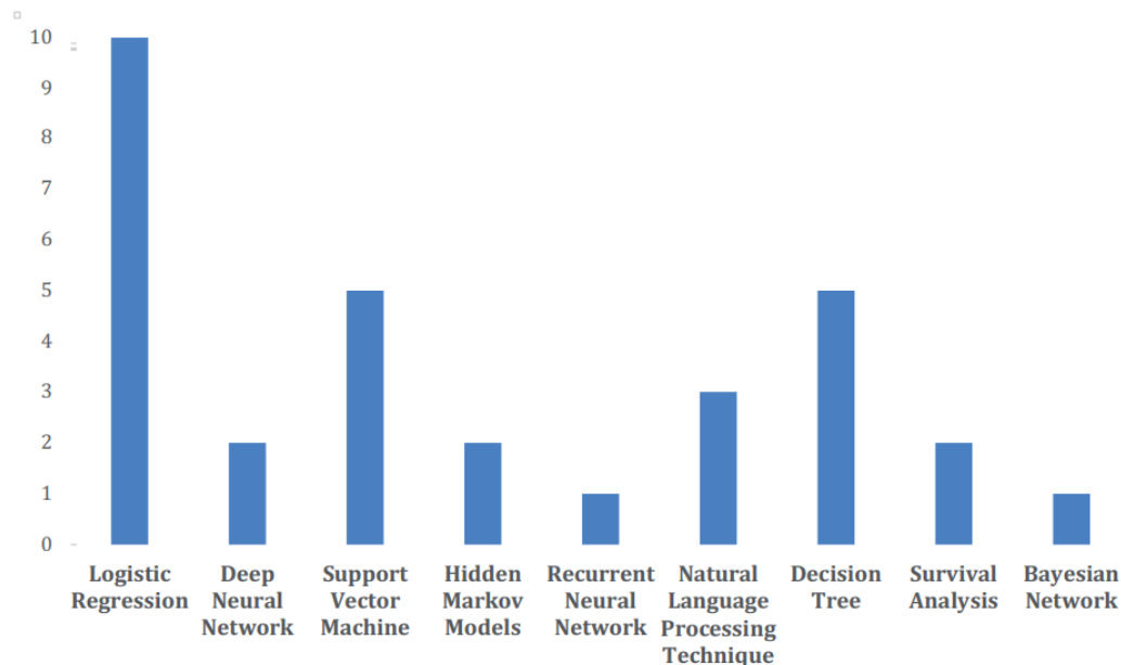
Figure 3.5 Fréquence de l'utilisation de la régression logistique dans la prédiction de l'abandon dans le domaine du e-learning [Dalipi et al., 2018]
