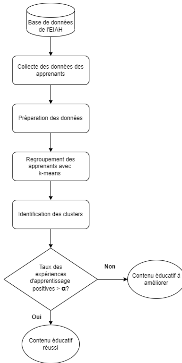
Figure 3.3 Processus de l'approche MALEA
