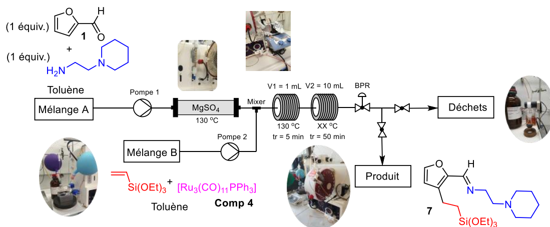
Schéma 45: Système de chimie en flux continu pour la réaction d'alkylation du furfural. Débit pompe A = Débit pompe B, pression \approx 7,5 bars.
