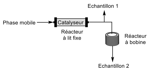
Figure 50 : schéma du réacteur tandem composé d'un réacteur à lit fixe contenant le catalyseur hétérogène et d'un réacteur à bobine utilisé par Hii et coll. pour déterminer la nature de l'espèce active dans une réaction de type Mizoroki-Heck
