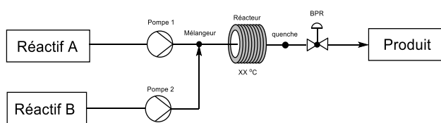
Figure 10 : Système de chimie en flux à deux entrées
