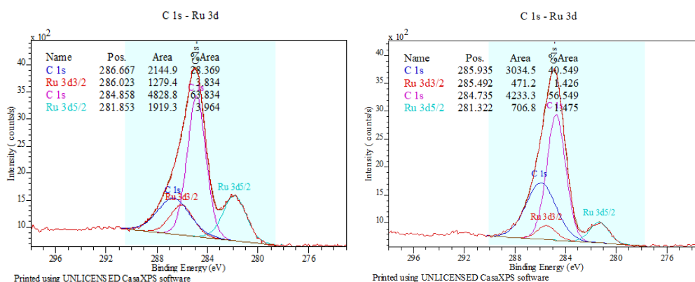
Figure 54 : Analyse XPS du catalyseur hétérogène Cat5 avant (gauche) et après la première réaction (droite)
