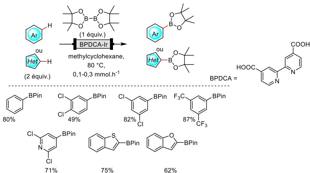
Schéma 103 : Borylation par activation C-H catalysée par un catalyseur d'iridium tassé dans un réacteur à lit fixe
