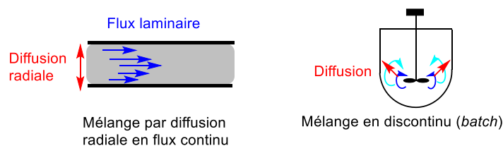
Figure 12 : Représentation d'un écoulement laminaire et d'un mélange par diffusion en flux continu comparé au mélange en discontinu grâce à un agitateur
