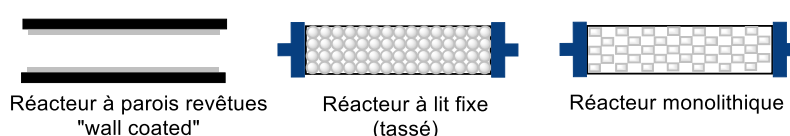
Figure 45 : Approches pour l'application de catalyseurs hétérogènes par chimie en flux continu : réacteurs à lit fixe, monolithiques ou à parois revêtues
