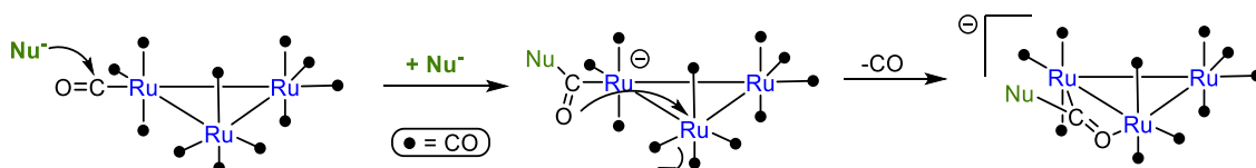
Schéma 38 : Réaction d'un nucléophile anionique avec \text{Ru}_3(\text{CO})_{12} – formation du complexe [\text{Ru}_3\{\mu\text{-O}=\text{C}(\text{Nu})\}(\text{CO})_{10}]^-
