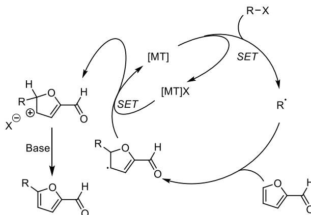
Schéma 22 : Mécanisme réactionnel de l'alkylation du furfural en position 5 avec un halogénure d'alkyle. SET = transfert mono électronique
