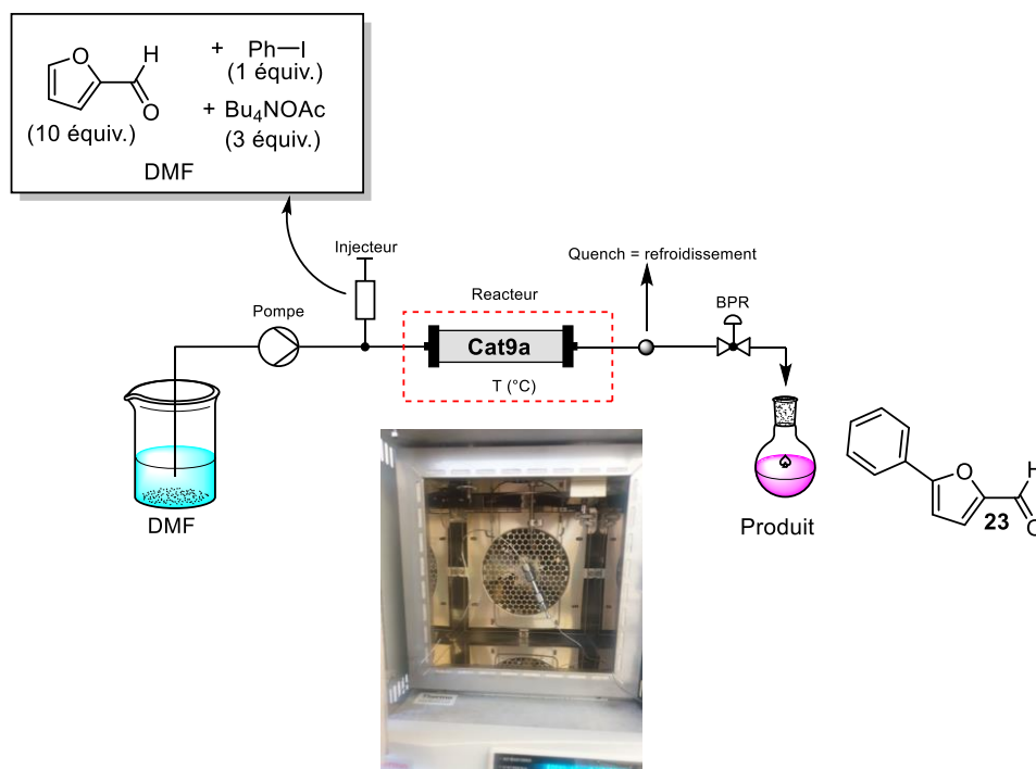
Schéma 119 : Système de chimie en flux pour l'arylation du furfural
