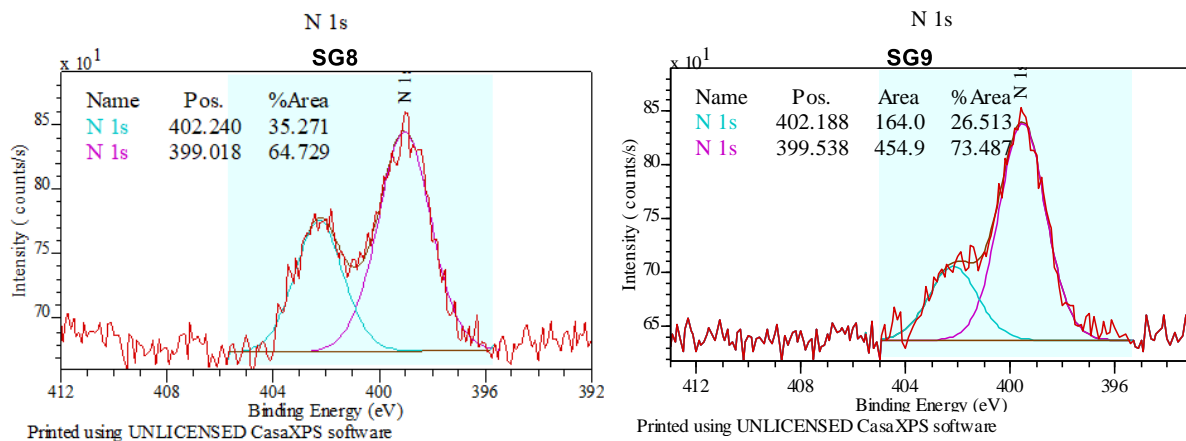
Figure 34 : Analyse XPS montrant les énergies de liaisons des orbitales 1s des azotes sur les solides SG8 et SG9
