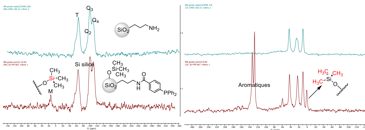
Figure 32 : Analyse RMN CP MAS du silicium 29 à gauche et du carbone 13 à droite de SG4 (contenant du TMS, rouge) comparée à l'analyse de la silice de départ (silice SMB 100-15 fonctionnalisée propylamine) (cyan)
