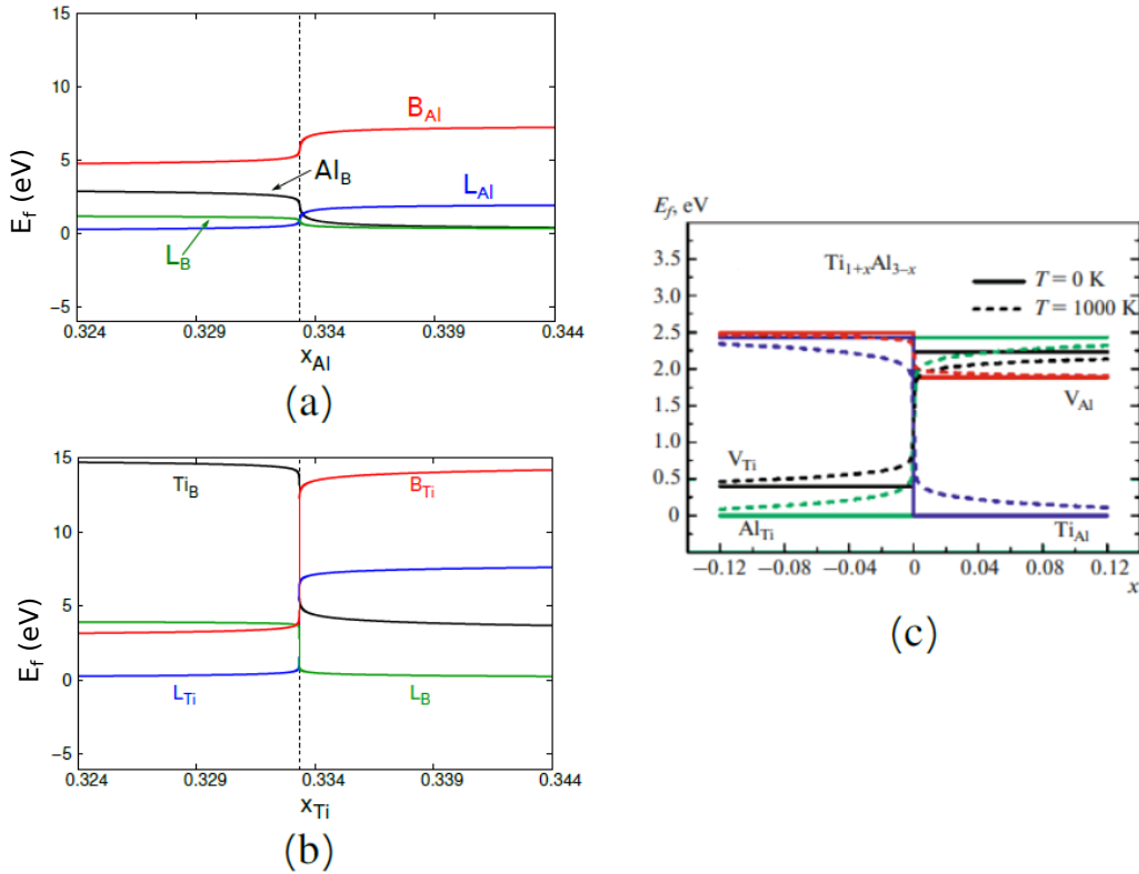
Figure 4.34: Comparaison des énergies de formation des défauts ponctuels des composés (a) \text{AlB}_2 et (b) \text{TiB}_2 issus de cette thèse, avec le composé (c) \text{Al}_3\text{Ti} [88] pour une température de 1000 K.
