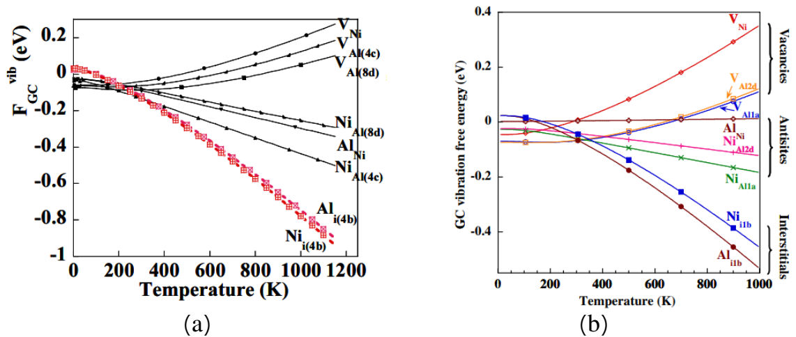
Figure 4.35: Énergies libres grand-canoniques des phonons des défauts ponctuels dans (a) \text{NiAl}_3 et (b) \text{Ni}_2\text{Al}_3 en fonction de la température [96–98].
