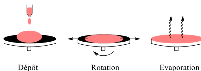
Figure 29 : Principe du « spin coating » schématisé
