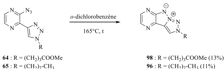
Schéma 112 : Thermolyse appliquée aux substrats aliphatiques
