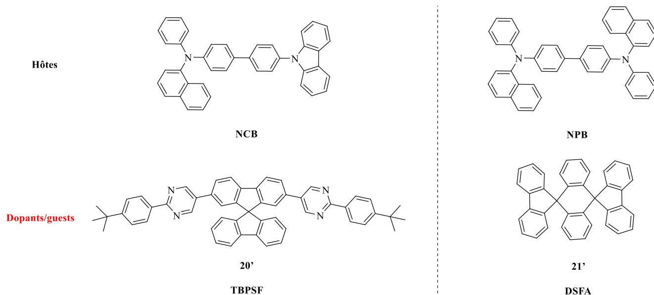
Figure 27 : Dérivés spirocycliques
