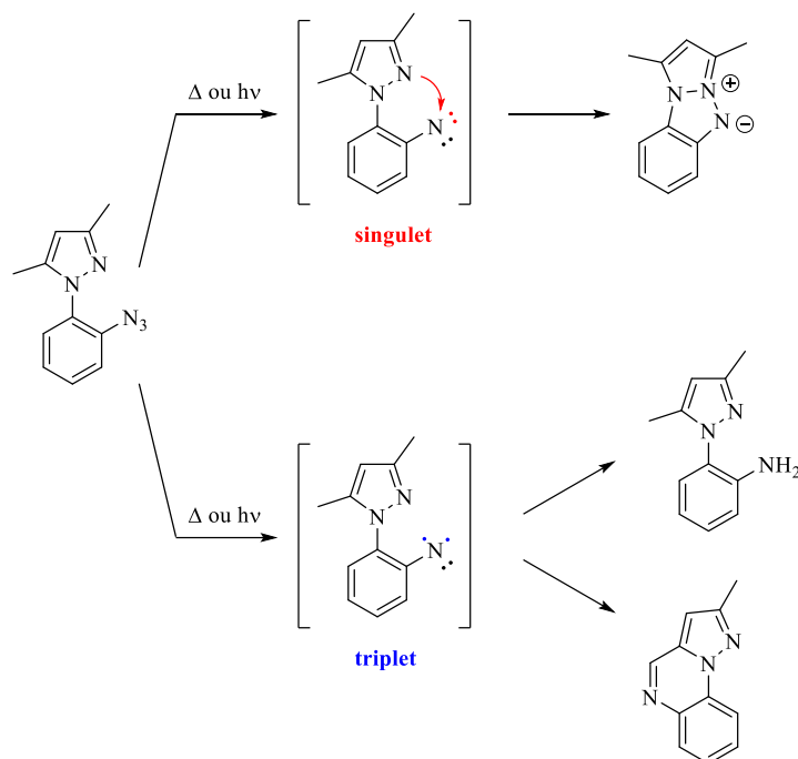
Schéma 15 : Compétition entre le nitrene singulet et triplet
