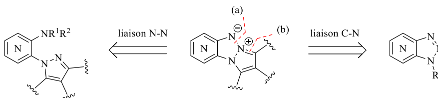
Figure 35 : Fragmentation du TAP fusionné
