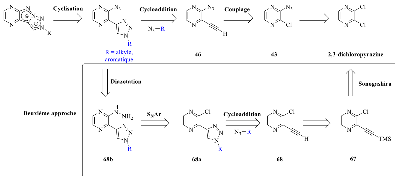
Schéma 92 : Rétrosynthèse alternative des dérivés bicycliques
