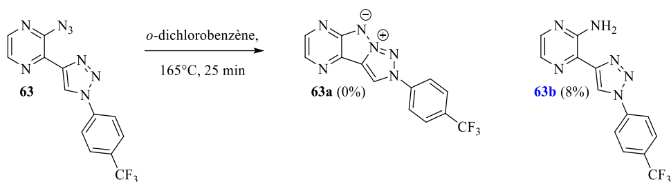
Schéma 111 : Thermolyse du produit 63
