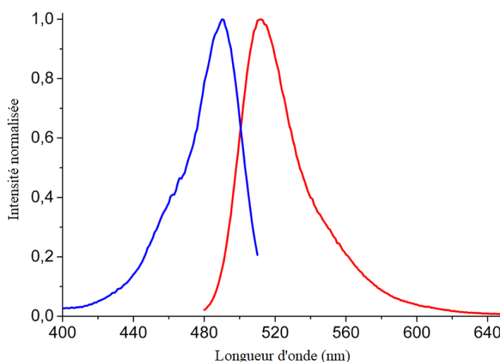
Figure 59 : Spectres d'excitation et d'émission de la fluorescéine en solution
