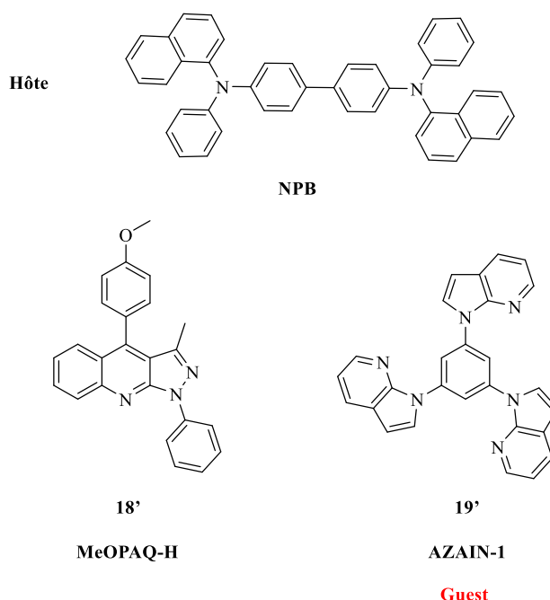
Figure 25 : Dérivés hétérocycliques
