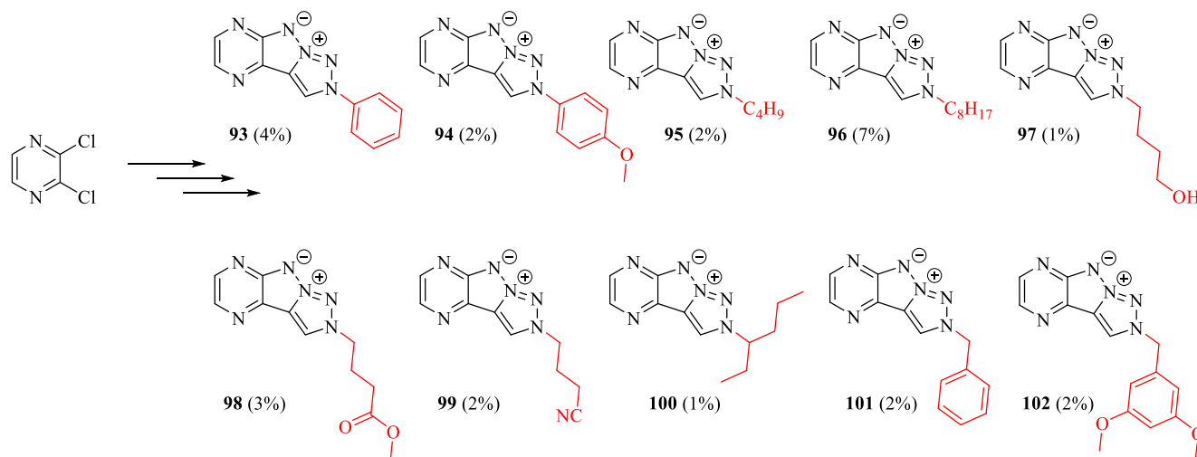
Figure 57 : Obtention des tétrazapentalènes
