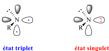
Figure 36 : États de l'espèce nitrène
