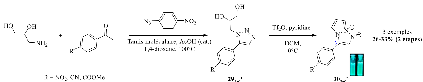
Schéma 6 : 1, 3a, 6a-triazapentalènes substitué en position 3
