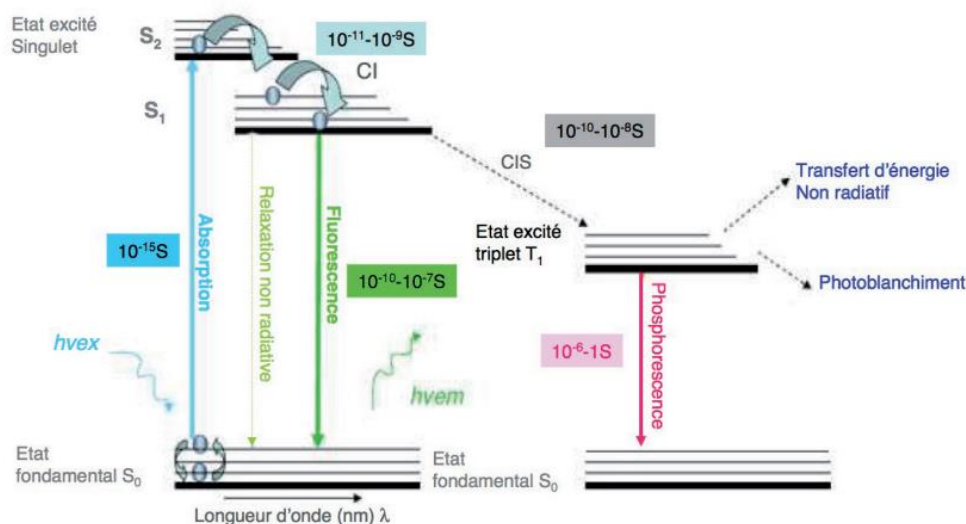
Figure 58 : Diagramme de Perrin-Jablonski
