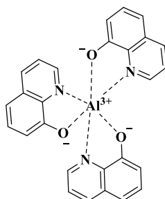
Figure 12 : Structure d'une couche ETL : le tris(8-hydroxyquinoléine)aluminium(III) (Alq 3 )
