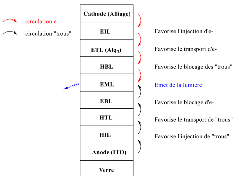
Figure 11 : Composition d'une OLED
