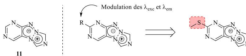
Figure 39 : Analogue comportant le groupement thioéther
