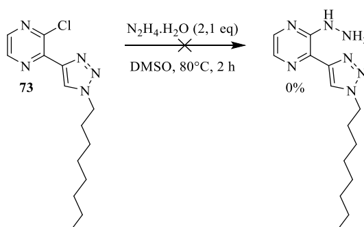
Schéma 104 : Introduction de l'hydrazine en milieu polaire aprotique
