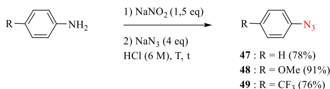
Schéma 86 : Diazotation d'anilines substituées en para
