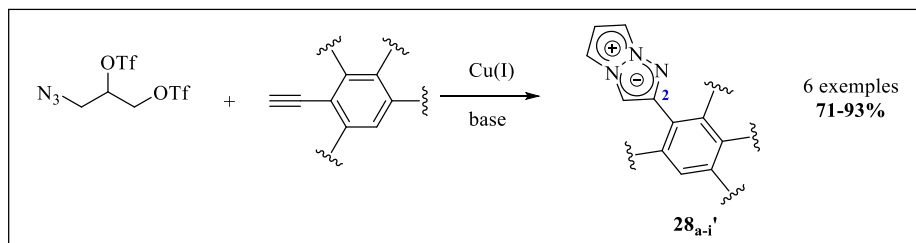
Schéma 5 : Etude de la nature des aromatiques en position 2
