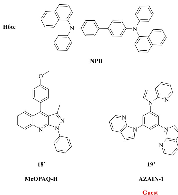
Figure 25 : Dérivés hétérocycliques
