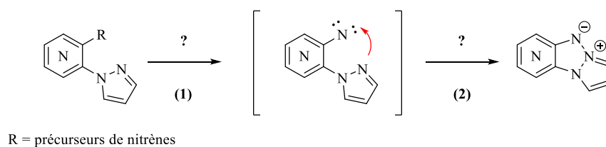
Schéma 7 : Obtention du motif TAP fusionné par liaison N-N
