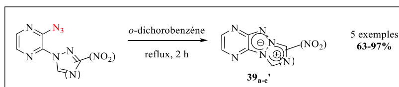
Schéma 18 : Premières synthèses de TAP fusioné développées au sein du laboratoire
