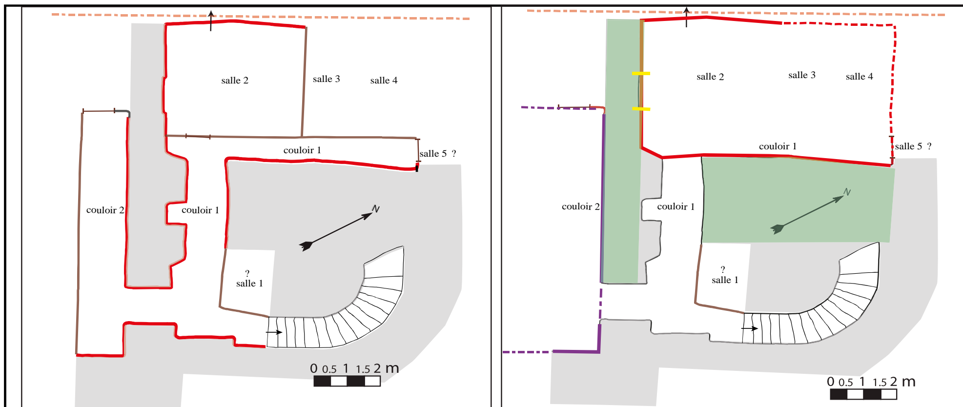
Plan de la cave avec les parois observées et relevées pendant la visite
