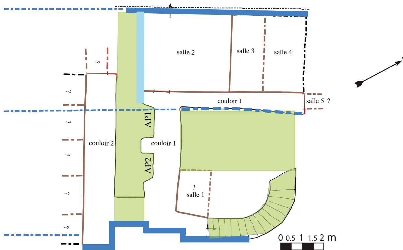
Plan n° 4 bis : Proposition de phasage pour la cave sise au 9, rue des Gouverneurs 64100 Bayonne
