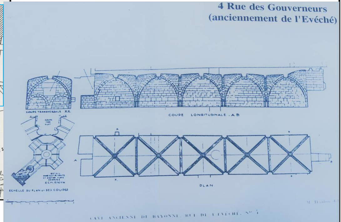
Relevé de Maurice Haulon (1938)
