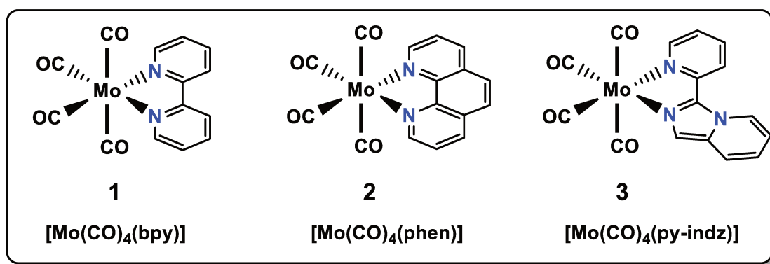
Figure VI.3. Structure des complexes [\text{Mo}(\text{CO})_4(\text{bpy})] ( 1 ), [\text{Mo}(\text{CO})_4(\text{phen})] ( 2 ) et [\text{Mo}(\text{CO})_4(\text{py-indz})] ( 3 ) utilisés dans nos études comparatives.
