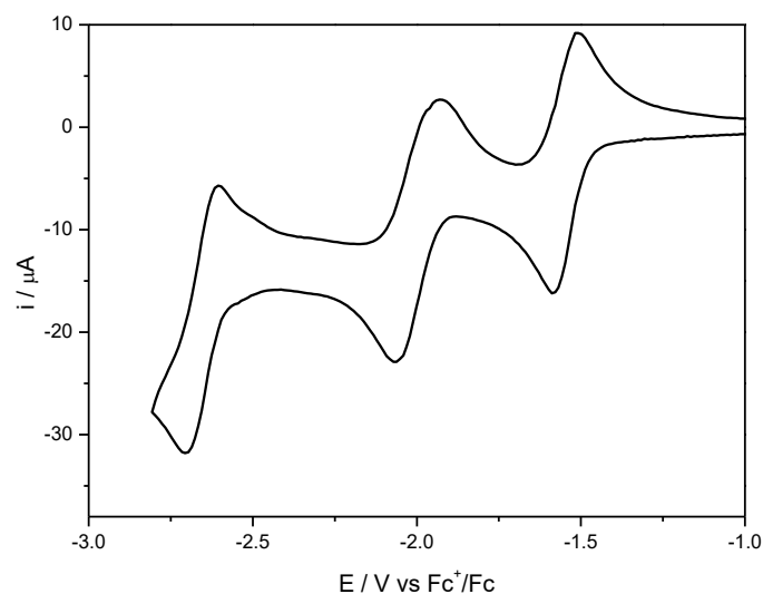
Figure VI.6. Voltammétrie cyclique de \mathbf{1}^{\text{CO}_2\text{Me}} dans THF / 0.1 M \text{NBu}_4\text{PF}_6 sous Ar. Conditions : 1 mM de complexe, électrode de travail BDD, \nu = 0,1 \text{ V s}^{-1} .
