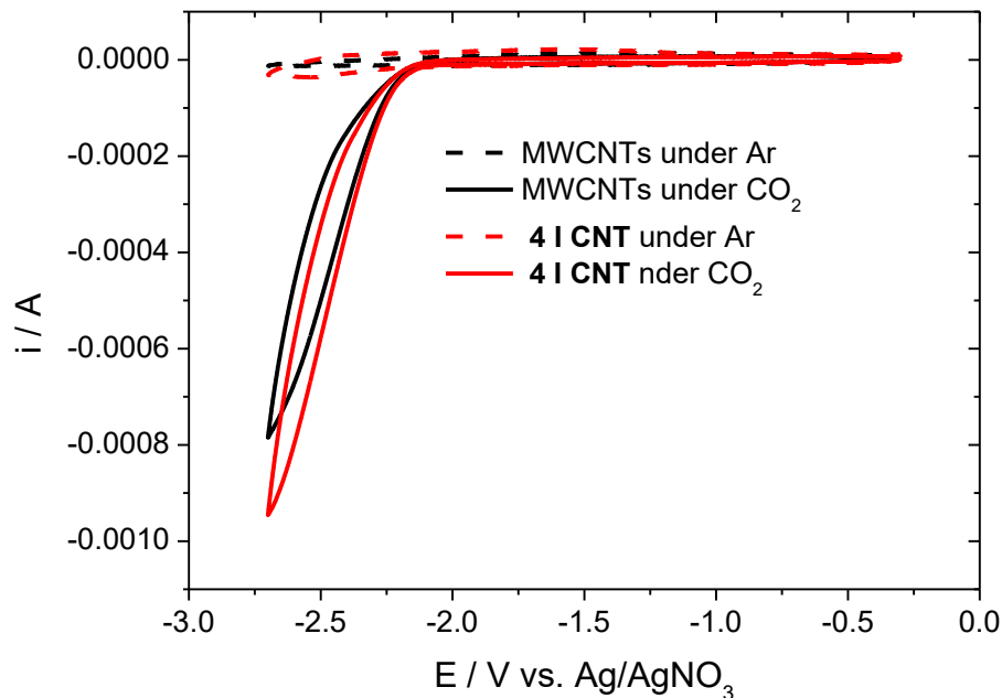
Figure VI.12. Voltammétries cycliques des assemblages 4|CNT accrochés sur des électrodes de carbone vitreux (rouge) et des électrodes GC MWCNT nues (noir) sous Ar (pointillés) et CO 2 (simple) dans THF / 0,1 M NBu 4 PF 6 . Ref. : Ag/AgNO 3 , \nu = 0,1 \text{ V s}^{-1} .
