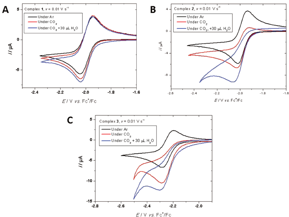
Figure VI.9. Voltammétries cycliques du A) complexe 1, B) complexe 2 and C) complexe 3 dans le THF sous Ar (noir), sous \text{CO}_2 (rouge) et sous \text{CO}_2 avec ajout d'eau (0,5 M, bleu). Conditions : 1 mM de complexe, 0.1 M \text{NBu}_4\text{PF}_6 , électrode de travail BDD, \nu = 0,01 \text{ V s}^{-1} .
