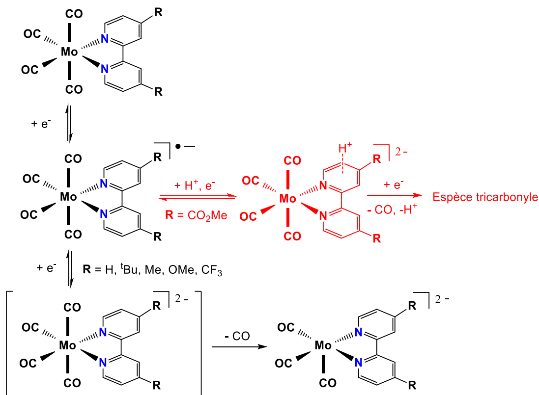
Figure VI.7. Proposition de mécanisme redox pour les complexes [\text{Mo}(\text{CO})_4(\text{bpy}-(\text{R})_2)] ( \text{R} = \text{H}, \text{}^t\text{Bu}, \text{Me}, \text{OMe}, \text{CO}_2\text{Me}, \text{CF}_3 ) dans le THF.
