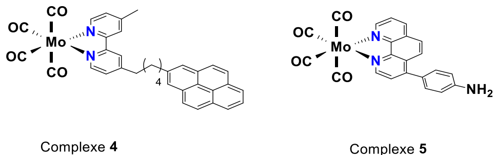
Figure VI.11. Représentation schématique des complexes 4 et 5 étudiés dans ce chapitre.
