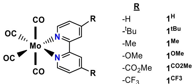
Figure VI.5. Structure générale des dérivés [\text{Mo}(\text{CO})_4(\text{bpy}-(\text{R})_2)] .
