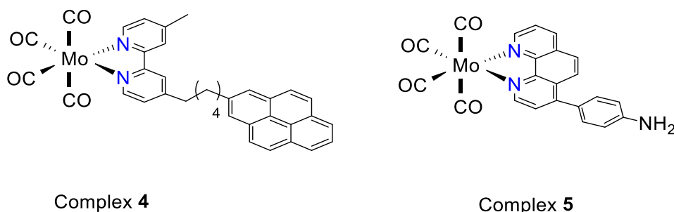
Figure VI.4. Représentation schématique des complexes 4 et 5 .
