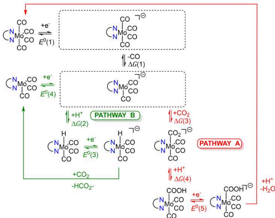
Figure VI.10. Voies mécanistiques suggérées pour la réduction du CO 2 par les complexes Mo-diimine 1 , 2 et 3 .
