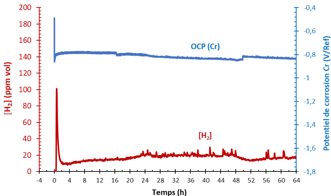
Figure 5.3 : Teneur en \text{H}_2 détectée par chromatographie gazeuse (en ppm volumique) et potentiel à circuit ouvert d'une électrode de chrome, lors de l'introduction de chrome dans \text{NaCl-CaCl}_2 à 600\text{ }^\circ\text{C} sous balayage d'argon.
