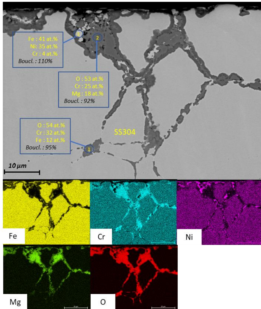
Figure 4.38 : Image MEB-BSE et cartographies élémentaires d'une coupe transverse d'un échantillon de SS304 corrodé dans \text{NaCl-CaCl}_2+\text{MgCl}_2 pendant 336 h à 600 °C.
