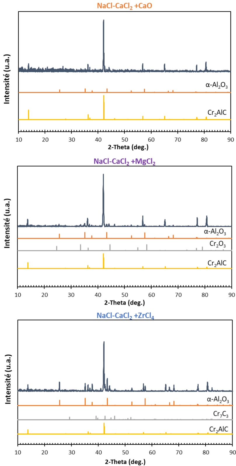
Figure 4.51 : Diffractogrammes des surfaces d'échantillons de Cr 2 AlC exposés à l'argon de balayage au-dessus des différents sels NaCl-CaCl 2 +CaO, NaCl-CaCl 2 +MgCl 2 et NaCl-CaCl 2 +ZrCl 4 pendant 336 h à 600 °C.
