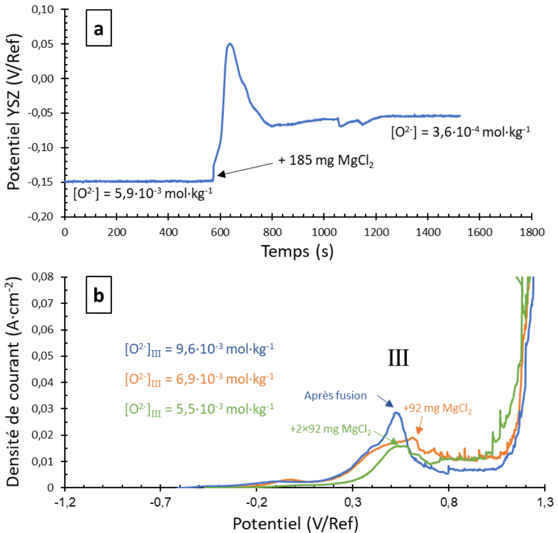
Figure 3.15 : Suivi par (a) sonde de zircon ytriée et (b) voltammétrie cyclique sur électrode de tungstène (vitesse de balayage = 100 \text{ mV} \cdot \text{s}^{-1} ) d'ajouts de \text{MgCl}_2 dans \text{NaCl-CaCl}_2 à 600 \text{ }^\circ\text{C} .
