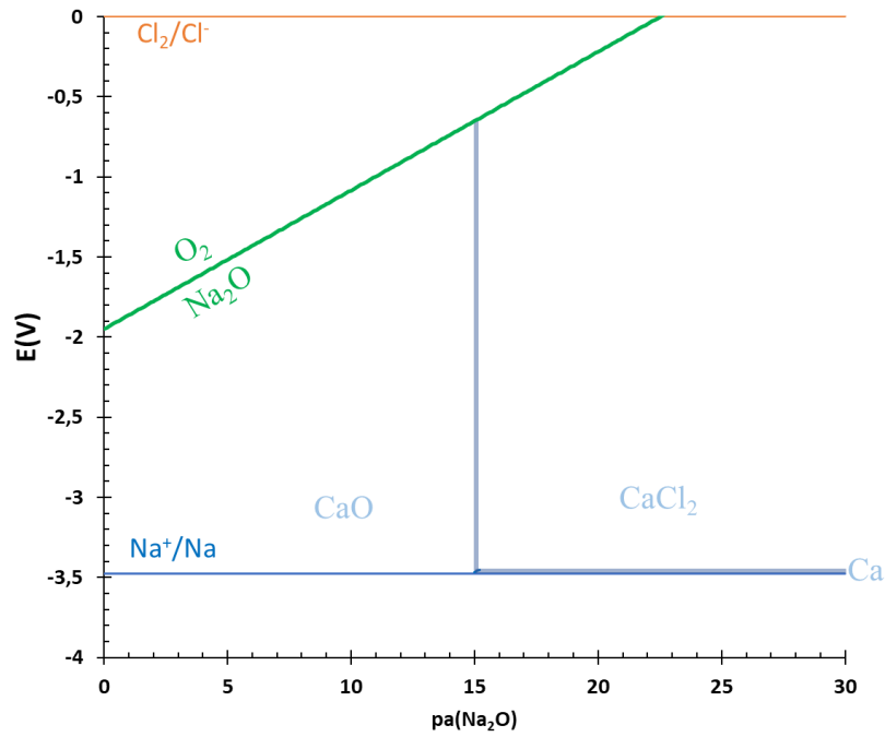
Figure 5.30 : Diagramme potentiel oxoacidité de NaCl-CaCl 2 à 600 °C.
