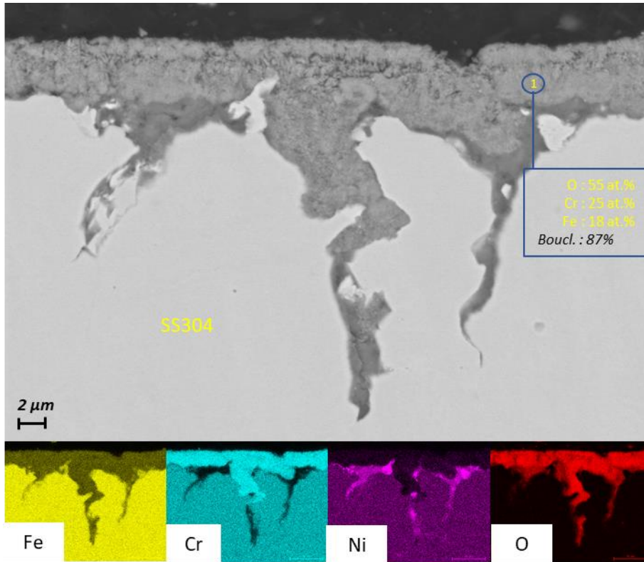
Figure 4.36 : Image MEB-BSE et cartographies élémentaires d'une coupe transverse de la partie exposée à l'argon de balayage d'un d'échantillon de SS304 corrodé dans NaCl-CaCl 2 +CaO pendant 336 h à 600 °C.
