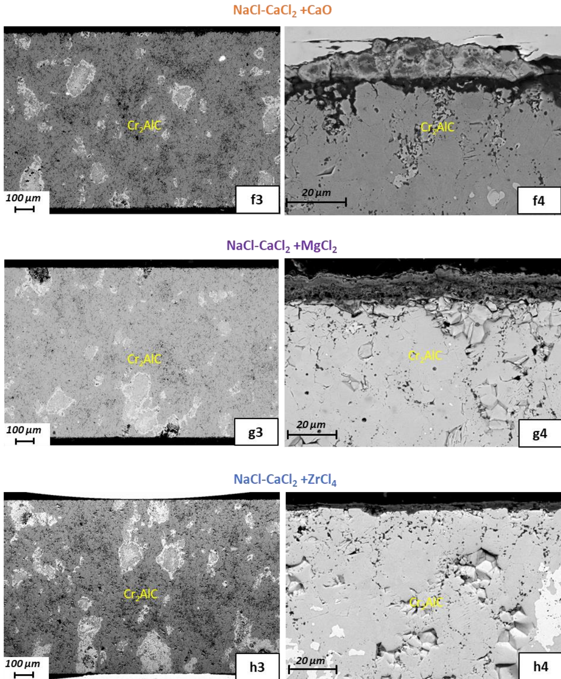
Figure 4.49 : Images MEB mixte SE-BSE de coupes de transverses d'échantillons de Cr 2 AlC exposés à l'argon de balayage au-dessus des sels (f3-f4) NaCl-CaCl 2 +CaO (g3-g4) NaCl-CaCl 2 +MgCl 2 (h3-h4) NaCl-CaCl 2 +ZrCl 4 pendant 336 h à 600 °C.
