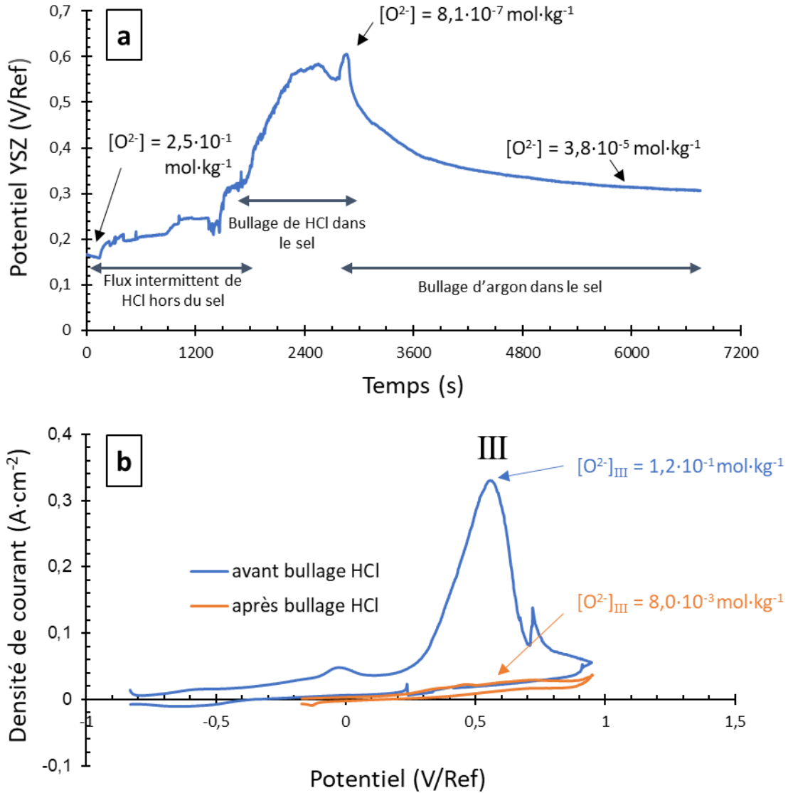
Figure 3.17 : Suivi par (a) sonde de zircone yttrée et (b) voltammétrie cyclique sur électrode de tungstène (vitesse de balayage = 100 \text{ mV} \cdot \text{s}^{-1} ) lors d'une purification NaCl-CaCl 2 par HCl à 600 °C.
