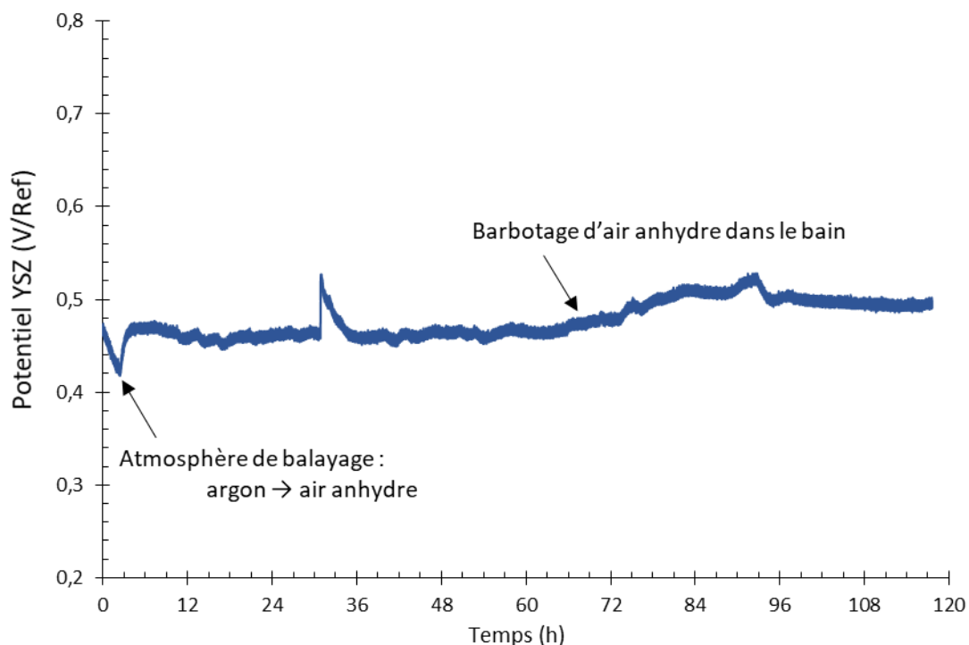
Figure 5.7 : Suivi de potentiel de membrane de l'électrode de zircon ytriée dans \text{NaCl-CaCl}_2 à 600\text{ }^\circ\text{C} lors d'une mise sous balayage d'air anhydre.
