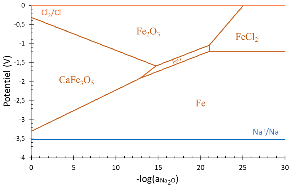
Figure 4.9 : Diagramme potentiel-oxoacidité du fer dans \text{NaCl-CaCl}_2 à 600\text{ }^\circ\text{C} .
