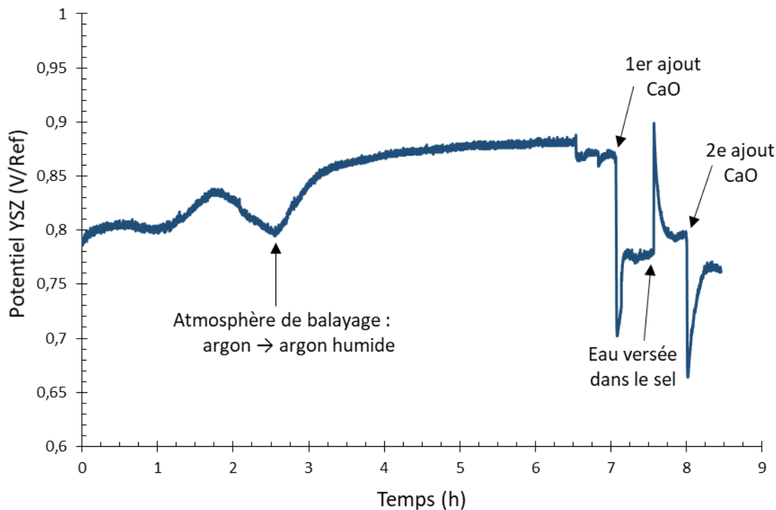
Figure 5.8 : Suivi du potentiel de membrane de l'électrode de zircone yttrée dans NaCl-CaCl 2 à 600 °C lors d'une mise sous balayage d'argon humidifié.
