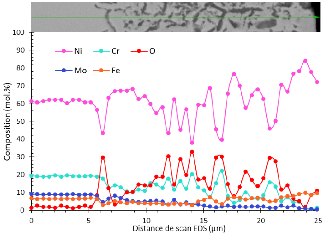
Figure 4.26 : Profil élémentaire d'une coupe transverse du C276 corrodé dans NaCl-CaCl 2 +ZrCl 4 après immersion de 336 h à 600 °C.
