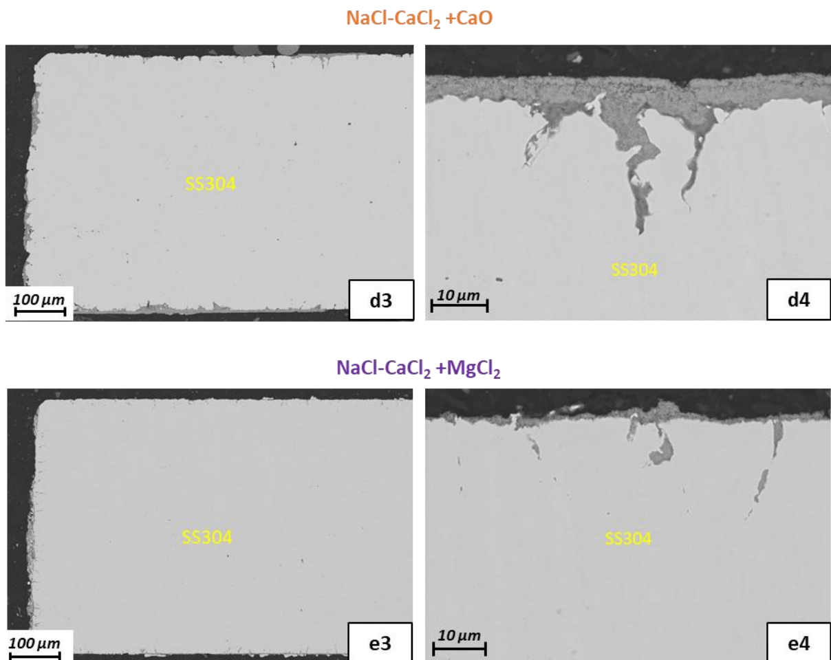
Figure 4.33 : Images BSE de coupes transverses d'échantillons de SS304 exposés à l'argon de balayage pendant 336 h à 600 °C au-dessus de (d3-d4) NaCl-CaCl 2 +CaO (e3-e4) NaCl-CaCl 2 +MgCl 2 .
