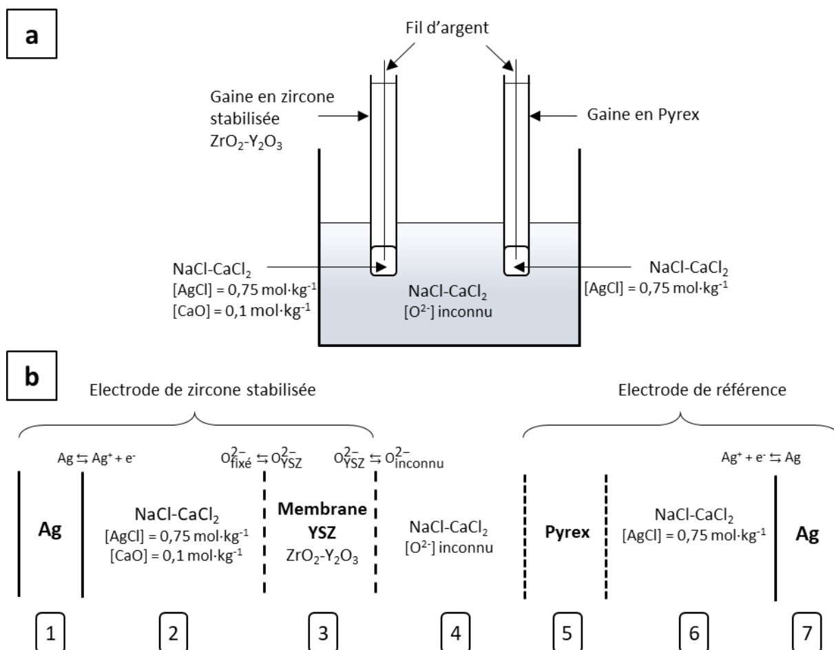
Figure 2.4 : Schéma de (a) du montage expérimental comprenant l'électrode de zircone yttrée et l'électrode de référence de (b) cellule galvanique pour la mesure de l'activité en ions oxyde dans NaCl-CaCl 2 [89] [90].
