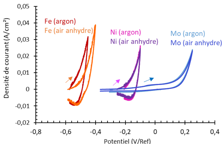
Figure 5.28 : Voltammogrammes du fer, nickel et molybdène sous argon et air anhydre dans \text{NaCl-CaCl}_2 à 600 °C (vitesse de balayage : 100 mV/s).
