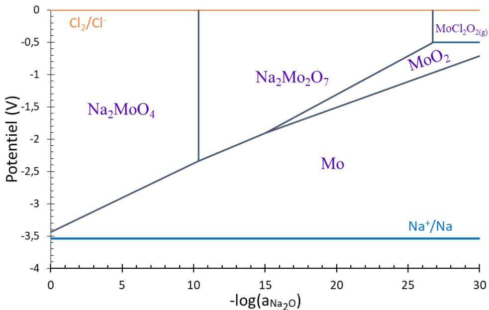
Figure 4.10 : Diagramme potentiel-oxoacidité du molybdène dans \text{NaCl-CaCl}_2 à 600\text{ }^\circ\text{C} .
