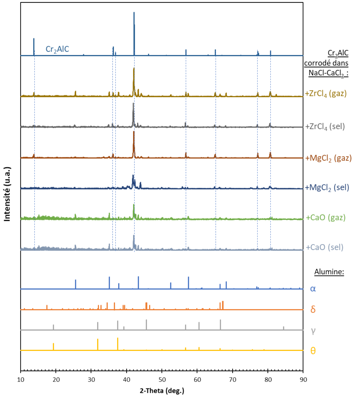
Figure 4.53 : Diffractogrammes des échantillons de \text{Cr}_2\text{AlC} corrodés dans les différents sels à 600\text{ }^\circ\text{C} pendant 336 h.
