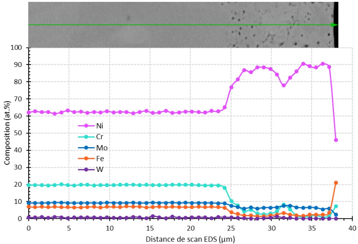
Figure 4.7 : Profil élémentaire EDS d'une coupe transverse de C276 corrodé dans NaCl-CaCl 2 +CaO après immersion de 336 h à 600 °C.
