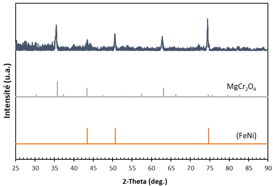
Figure 4.39 : Diffractogramme de la surface du SS304 corrodé dans \text{NaCl-CaCl}_2+\text{MgCl}_2 après immersion de 336 h à 600 °C.
