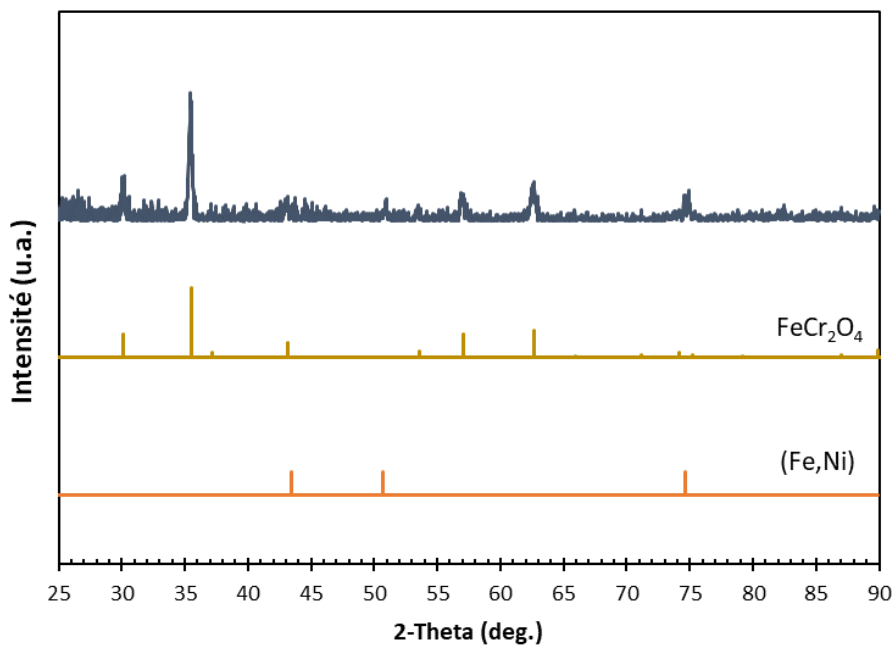
Figure 4.37 : Diffractogramme de la surface du SS304 exposé à l'argon de balayage au-dessus de NaCl-CaCl 2 +CaO pendant 336 h à 600 °C.
