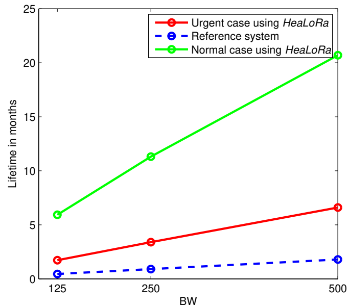
FIGURE 3.9 – Impact de la bande passante sur la durée de vie du système
