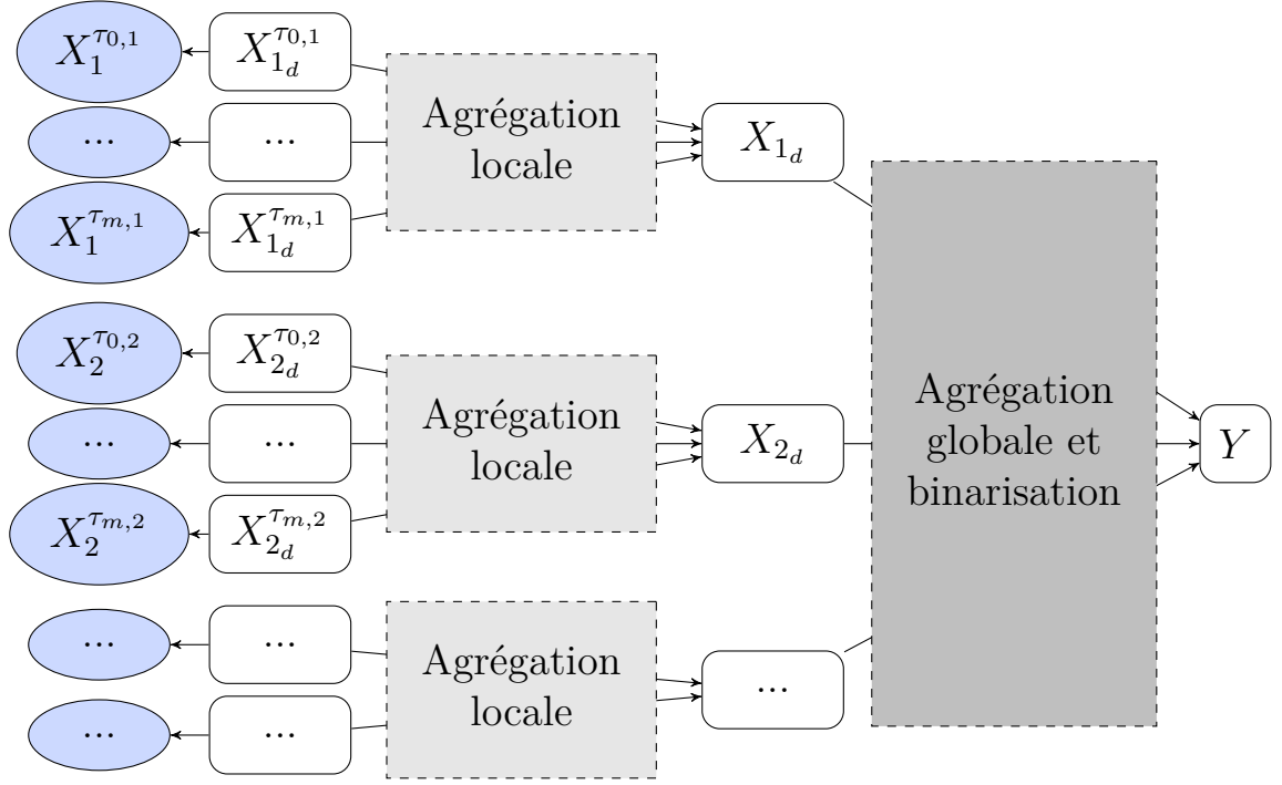
FIGURE 3.3 – Architecture générale de réseau bayésien. Les cercles représentent des variables aléatoires continues et les rectangles (arrondis) des variables discrètes. Les X_i sont les mesures de capteurs en entrée, \tau_{m,i} étant le seuil mentionné dans la partie 3.1 et illustré dans la figure 3.1.
