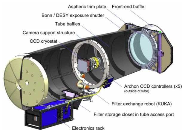
(b) Vue en coupe du télescope Samuel Oschin avec le nouveau système ZTF (DEKANY et al., 2020).
