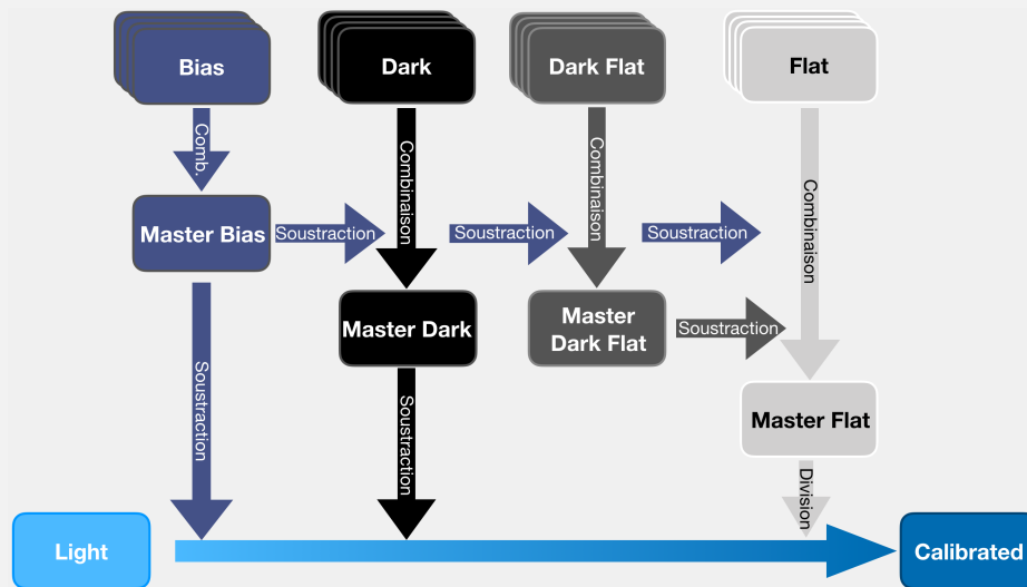
FIGURE 4.3 – Schéma d'application d'images de calibration Bias, Dark et Flat.
