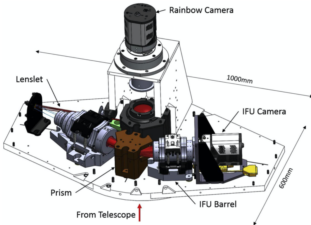
FIGURE 4.2 – Vue d’ensemble de la SEDm (BLAGORODNOVA et al., 2018). La source de lumière du Cassegrain est indiqué par la flèche rouge. L’instrument photométrique, la RC, est situé en haut au centre et récolte directement la lumière. Pour l’IFU, la lumière est redirigée jusqu’à un miroir que l’on peut voir tout à gauche de la représentation. Elle est ensuite réfléchié dans le MLA (Lenslet). La lumière de chaque micro-lentille du MLA passe ensuite dans le prisme (en marron au centre) pour y être dispersée et focalisée par l’optique (IFU Barrel) sur le détecteur (IFU Camera).
