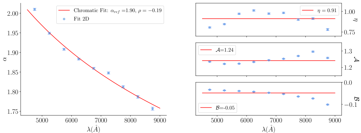
FIGURE 7.18 – Ajustement de la chromaticité des paramètres de forme de la PSF pour l'étoile standard 25d4655. À gauche, l'ajustement du paramètre \alpha avec une loi de puissance. À droite, de haut en bas, l'ajustement par une constante de \eta (poids entre la gaussienne et la Moffat) et des paramètres \mathcal{A} et \mathcal{B} .
