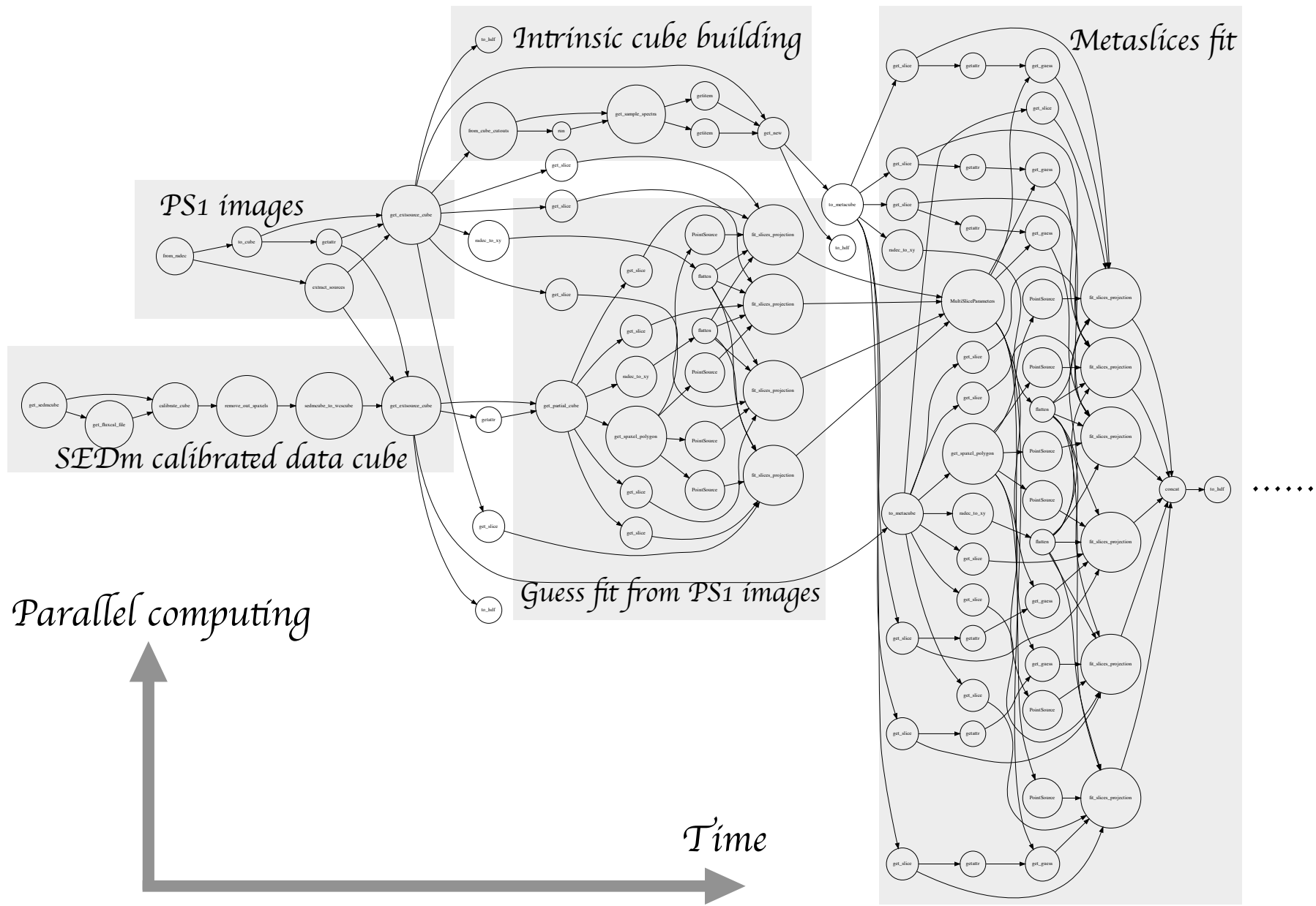
FIGURE 8.16 – Graphique d’une partie des calculs avec Dask et leurs interconnexions du pipeline HYPERGAL, de la requête des données jusqu’à l’ajustement des N méta-tranches.
