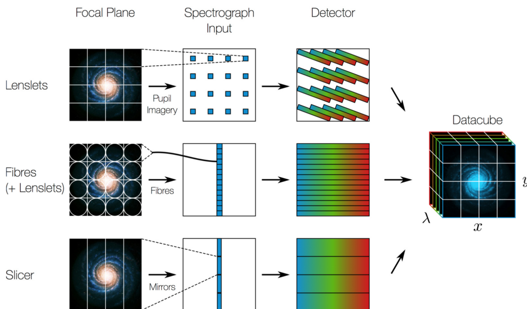
FIGURE 4.1 – Fonctionnement de différents types d’IFS. La SEDm utilise un système d’agencement de micro-lentilles (cas du haut ) (Crédit M. Westmoquette, adaptée de ALLINGTON-SMITH et CONTENT (1998)).
