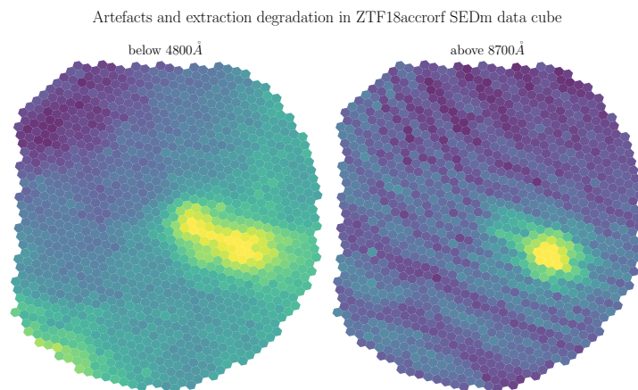
FIGURE 8.2 – Exemples d'artefacts dans les cubes de données SEDm pour ZTF18accrorf. À gauche, toutes les tranches en dessous de 4800\text{\AA} du cube de données empilées. À droite, toutes celles au dessus de 8700\text{\AA} . On peut clairement voir dans le bleu la présence d'un signal de fond structuré et intense, distordant complètement les objets dans le champ de vue et causant la présence d'artefacts sur les bords du cube. Dans le rouge, la forme des sources est également altérée, mais on voit surtout un phénomène de franges dans les données.
