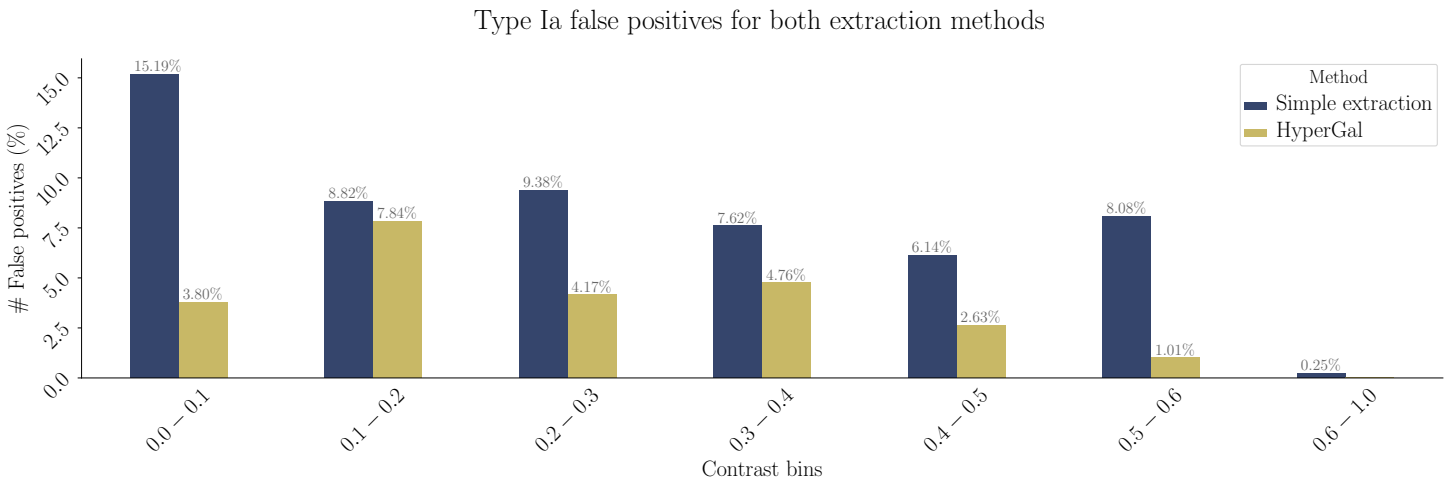
FIGURE 9.15 – Taux de faux positifs dans la classification des SNeIa pour les deux méthodes d'extraction en fonction du contraste.
