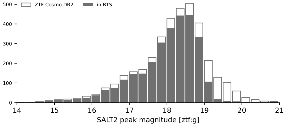
FIGURE 10.3 – Distribution du pic en magnitude dans la bande g de ZTF des SNeIa de la DR2, dérivées à partir de l’ajustement SALT2 des courbes de lumière. La partie noire de la distribution correspond à la proportion de supernovae également incluses dans l’échantillon BTS (FREMLING et al., 2020; PERLEY et al., 2020). Figure de M.Rigault.
