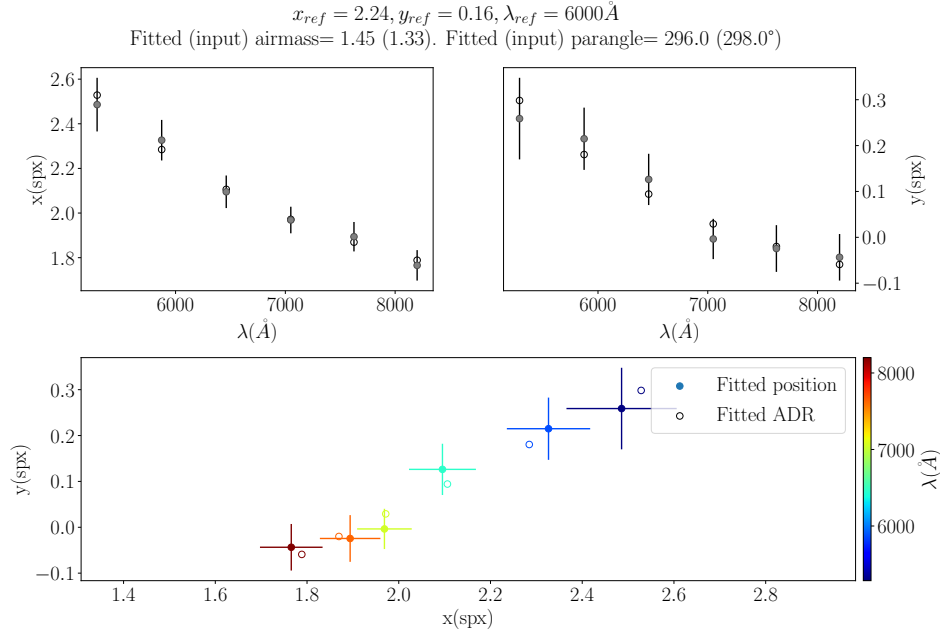
FIGURE 8.7 – Modélisation de la réfraction atmosphérique différentielle pour ZTF18accrorf. Je montre ici l’ajustement de la position d’ancrage (x_0, y_0) qui représente le centroïde de la supernova par le modèle d’ADR présenté dans le chapitre 7. Les deux graphes du haut représentent l’ajustement des deux coordonnées en fonction de la longueur d’onde. Le graphe du bas illustre l’effet de la réfraction atmosphérique.
