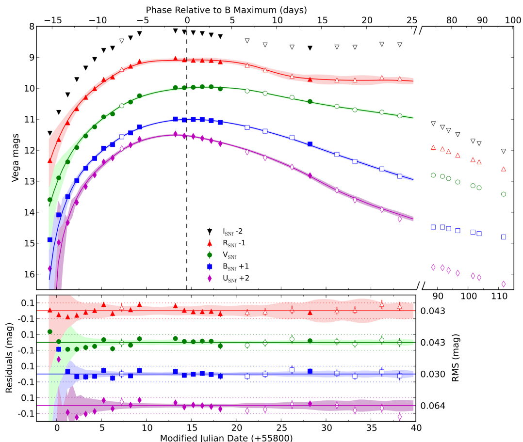
FIGURE 2.4 – Courbe de lumière de la SNIa SN2011fe entre -15 et +100 jours relativement à la phase 0 (pic de luminosité dans la bande B ) et dans les bandes UBVRI . Les courbes indiquent l’ajustement effectué avec le modèle SALT2 (Sec 2.2.4). Le graphique du bas montre les résidus entre les mesures photométriques et le modèle ajusté. Les bandes de couleurs indiquent les incertitudes du modèle. Figure de PEREIRA et al. (2013), dans le cadre de la collaboration SNFactory.
