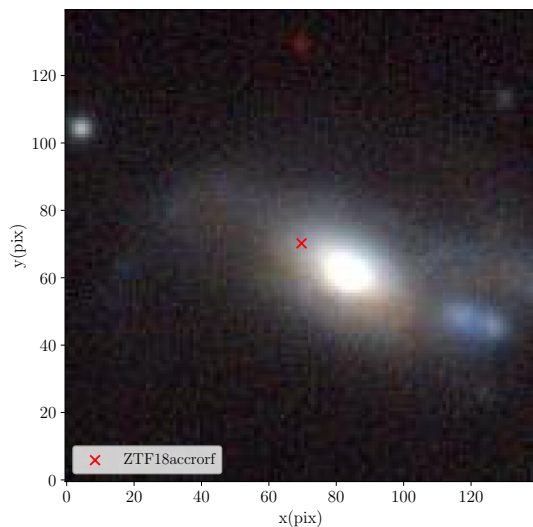
FIGURE 6.3 – Image RGB construite à partir des bandes g_{P1} , r_{P1} et z_{P1} des images PS1. L'image fait 35'' de côté et est centrée sur la position de détection de ZTF18accrorf par ZTF, à (RA, DEC) = (17.1692^\circ, 20.0799^\circ)
