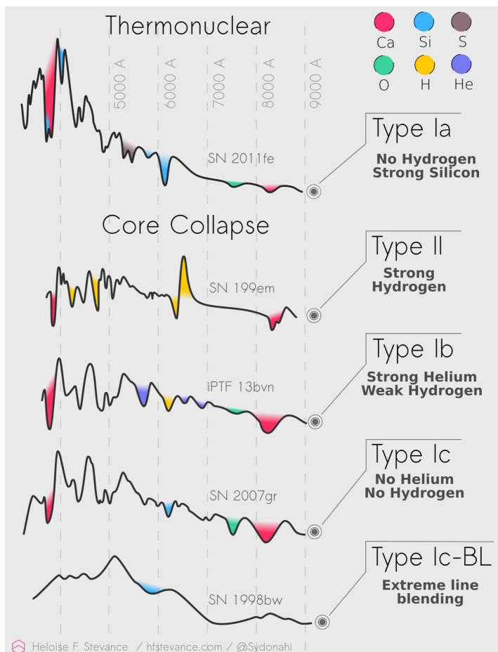
FIGURE 2.1 – Spectre de différents types de supernovae. Image de H. Stevance a
