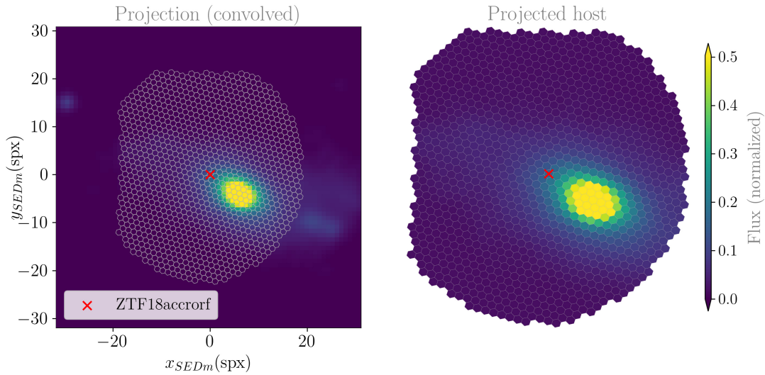
FIGURE 8.1 – Projection de la galaxie hôte dans le MLA pour une méta-tranche du cube intrinsèque. Pour cet exemple, la tranche est convoluée par une gaussienne 2D sans ellipticité d’écart type 1 spaxel. La croix rouge indique la position de la supernova ZTF18accrorf estimée par la Rainbow Camera dans le MLA, qui sert d’ancrage à la projection d’un espace spatial à l’autre.
