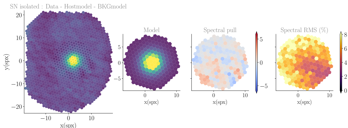
FIGURE 8.11 – Séparation de la supernova ZTF18accrorf dans le cube SEDm. Chaque image de cube 3D correspond à une intégration entre 5000 et 8500Å. De gauche à droite : (a) le cube de données SEDm auquel j’ai soustrait le modèle de la galaxie et celui du fond, ce qui met en évidence la qualité d’isolation de la supernova et, a fortiori , la qualité de modélisation des deux autres composantes. (b) Le cube modèle de la source ponctuelle limité à une ouverture circulaire de 8 spaxels ( \sim 4''5 ) de rayon, définie par les spaxels mis en évidence dans (a) par les losanges noirs. (c) Le pull spectral et (d) la RMS spectrale dans cette ouverture, tout deux définis comme dans la Figure 8.9. On notera ici l’absence de structure résiduelle, et une RMS spectrale de l’ordre de 3-4% au niveau de la position de ZTF18accrorf.
