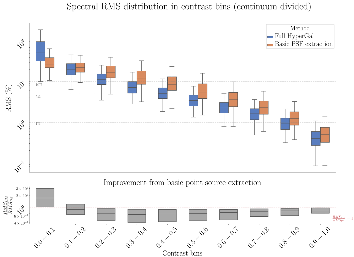
FIGURE 9.11 – Même chose que pour la Figure 9.8 mais après division des spectres par leur continuum.
