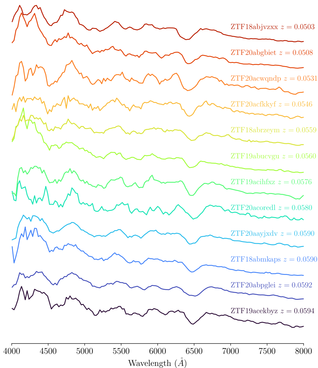
FIGURE 10.6 – Exemple de spectres du golden sample de la DR2 extraits par HYPERGAL au pic de luminosité dans un même intervalle de redshift ( 0.05 < z < 0.06 ).
