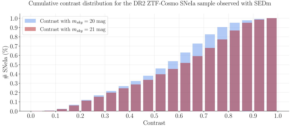
FIGURE 9.13 – Même chose que pour la Figure 9.12 mais avec la distribution cumulative des contrastes
