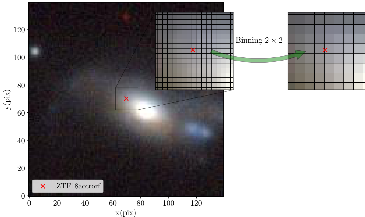
FIGURE 6.4 – Illustration du binning 2 \times 2 sur l'image de la Figure 6.3
