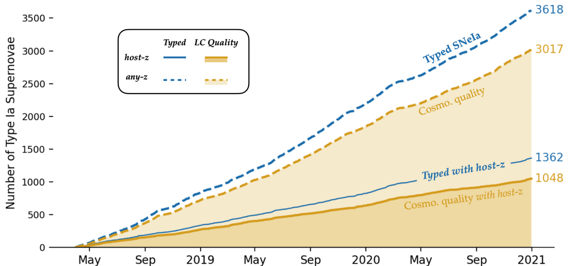
FIGURE 3.7 – Nombre cumulé de SNIa observées par ZTF (phase 1). Les contours dorés correspondent à l'échantillon passant les critères de coupure pour une qualité cosmologique. Le trait plein montre les SN avec un redshift spectroscopique de leur galaxie hôte. À titre de comparaison, le jeu de données le plus récent dans la littérature comptabilise moins de 500 SNIa à un redshift de z < 0.1
