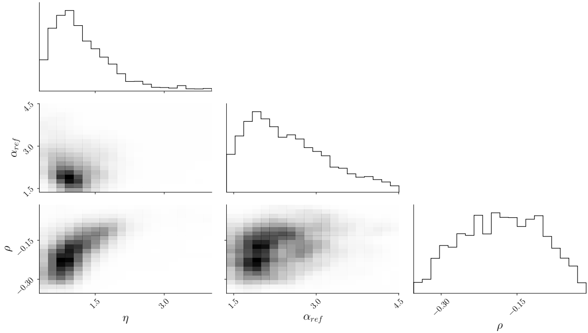
FIGURE 9.3 – Distribution conjointe des paramètres de PSF utilisés pour les simulations. Le niveau de gris indique la densité de simulations dans un intervalle donné.
