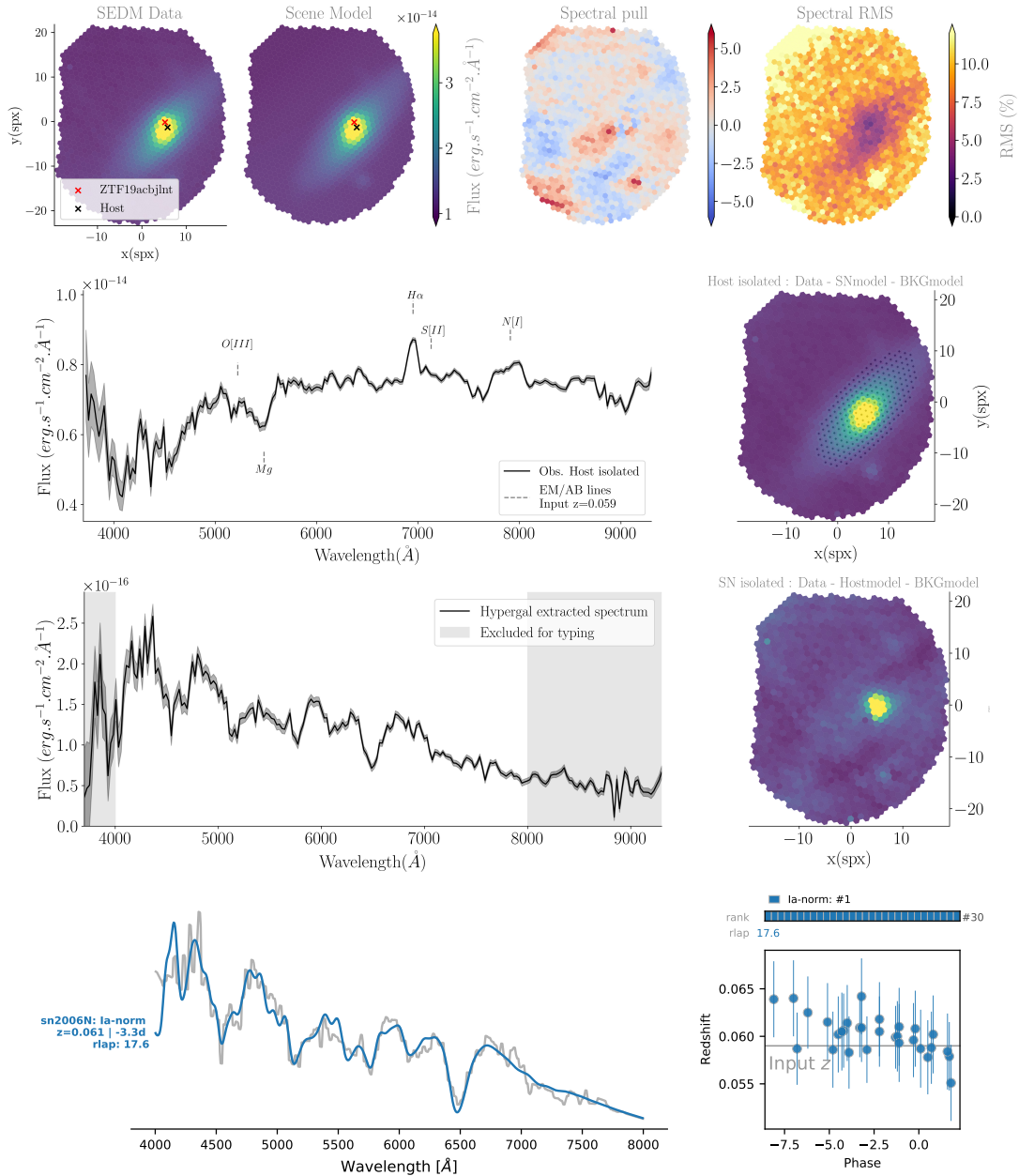
FIGURE 8.18 – Extraction de sources pour ZTF19acbjlnt avec HYPERGAL. De haut en bas : (a) visualisation globale de la modélisation de scène, pull et RMS spectraux, (b) l’isolation de la galaxie hôte, (c) l’isolation de ZTF19acbjlnt, (d) la classification SNID de ZTF19acbjlnt. La distance apparente entre la supernova et la galaxie est d’environ 0''8 avec un redshift d’entrée pour la modélisation hyperspectrale de la galaxie de z_{in} = 0.059 . Cette supernova est classifiée comme une Ia-norm avec un redshift moyen pondéré par le rlap de z_{snid} = 0.060 et nMAD(z_{snid}) = 0.002 .
