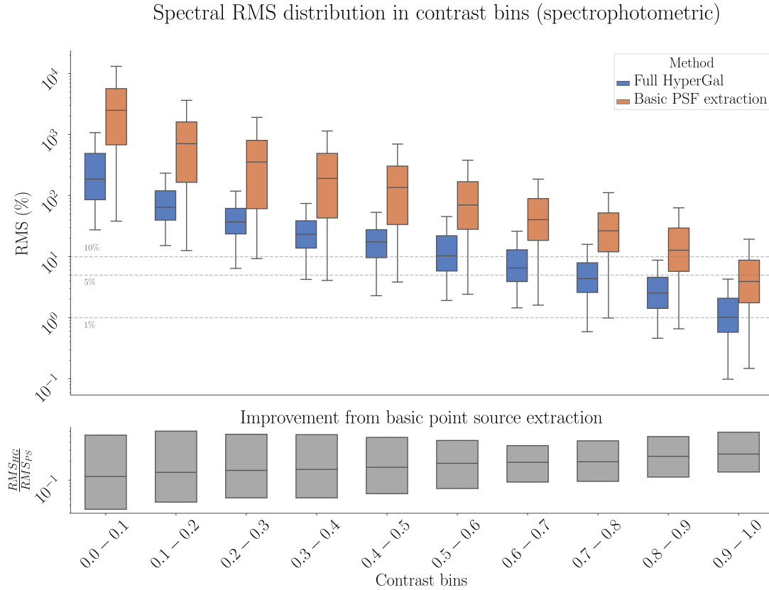
FIGURE 9.8 – Distribution de la RMS spectrale entre le spectre d’entrée de la simulation et le spectre extrait en fonction du contraste sur l’intervalle [4000, 8000]\text{\AA} . Les distributions sont présentées en boîtes, dont les 3 barres centrales représentent les 3 quartiles (25%, médiane et 50%). J’illustre ici une distribution de RMS spectrale pour chacune des deux méthodes d’extraction et pour différents intervalles de contraste, chacun comptabilisant le même nombre de simulations. En haut , la RMS spectrale (en %) obtenue avec les deux méthodes en fonction du contraste. Les traits en pointillés indiquent les niveaux à 1%, 5% et 10%. En bas , le rapport \frac{RMS_{HG}}{RMS_{PS}} pour illustrer l’amélioration apportée par HYPERGAL . Seule la boîte représentant les 3 quartiles de chaque distribution est affichée pour plus de clareté visuelle.
