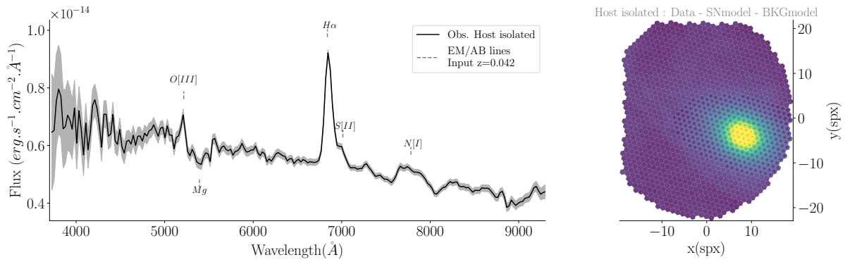
FIGURE 8.10 – Extraction du spectre intégré de la galaxie hôte de ZTF18accrorf. À droite, le cube de données de la SEDm, auquel j’ai soustrait les modèles de fond et de la source ponctuelle afin d’isoler la galaxie hôte. Les spaxels sélectionnés par les losanges noirs indiquent ceux appartenant à l’ouverture utilisée pour l’extraction du spectre intégré. À gauche, le spectre extrait et l’erreur associée contenus dans cette ouverture. Tout le domaine spectral de la SEDm est affiché, bien que nous avons déjà discuté de la faible fiabilité de l’extraction aux extrémités du domaine couvert par la SEDm due aux artefacts présents dans les cubes. Je montre également la position théorique de quelques raies d’émission et d’absorption sachant le redshift utilisé ( z = 0.042 ). On voit ici la bonne cohérence avec le spectre intégré extrait.
