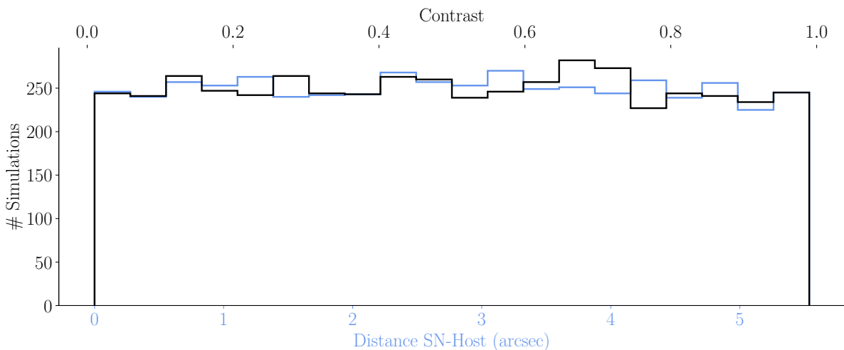
FIGURE 9.5 – Distribution du contraste et de la distance SN-centre de la galaxie des simulations.
