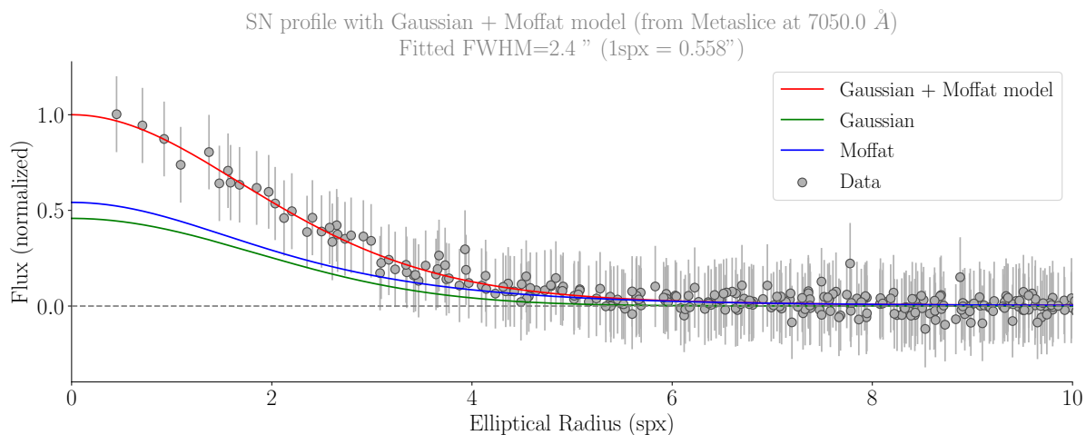
FIGURE 8.12 – Profil radial et modèle de PSF pour la méta-tranche à 7050Å de ZTF18accrorf. Le pic du flux est ici normalisé à 1. Les points noirs indiquent les données de la méta-tranche du cube d’observation de la SEDm après soustraction du modèle de la galaxie et du fond. Les courbes verte, bleue et rouge montrent respectivement l’ajustement de la composante gaussienne, Moffat et profil radial total du modèle de PSF pour cette méta-tranche. Le trait horizontal en pointillés indique un fond de ciel à 0 si cette composante a été parfaitement soustraite. Les ailes du profil tendant clairement vers cette valeur, cela nous conforte quant à la qualité d’ajustement de cette composante. Connaissant la taille d’un spaxel, on peut également déterminer la largeur à mi-hauteur à cette longueur d’onde, ici 2''4 .
