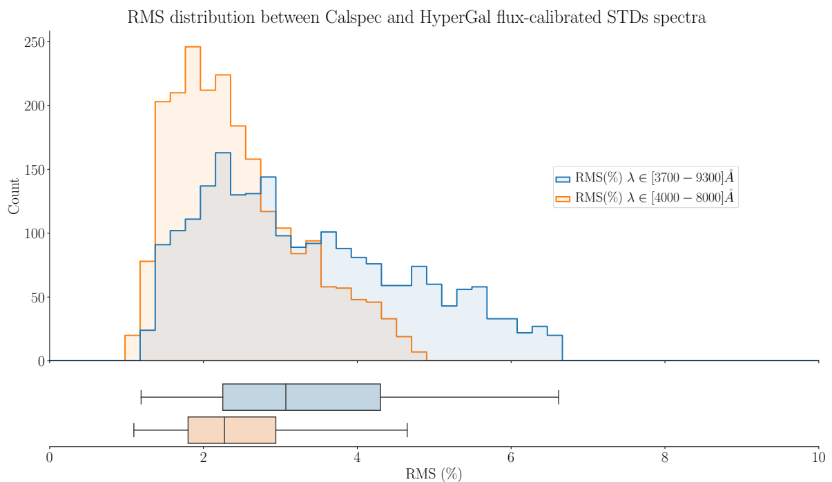
FIGURE 7.24 – Distributions de la RMS spectrale des calibrations en flux de 2202 étoiles standards pour différents intervalles spectraux. En haut sont représentés les histogrammes des distributions et en bas le box plot correspondant. La distribution bleue correspond au domaine spectral entier de la SEDm et celle en orange à l'intervalle \lambda \in [4000-8000] \text{ \AA} , utilisé pour la classification spectrale des supernovae avec la SEDm. Les boxes de la figure du bas montrent pour chaque distribution le minimum, le 1 er quartile (25% des valeurs), la médiane, le 3 ème quartile (75% des valeurs) et le maximum.
