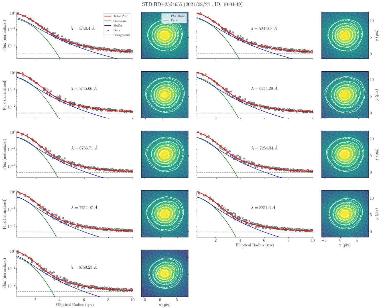
FIGURE 7.16 – Profil radial (à gauche) et contours d’intensité (à droite) des 9 metaslices de la STD 25d4655. Les traits pleins du contour représentent les données et les pointillées l’ajustement du modèle.
