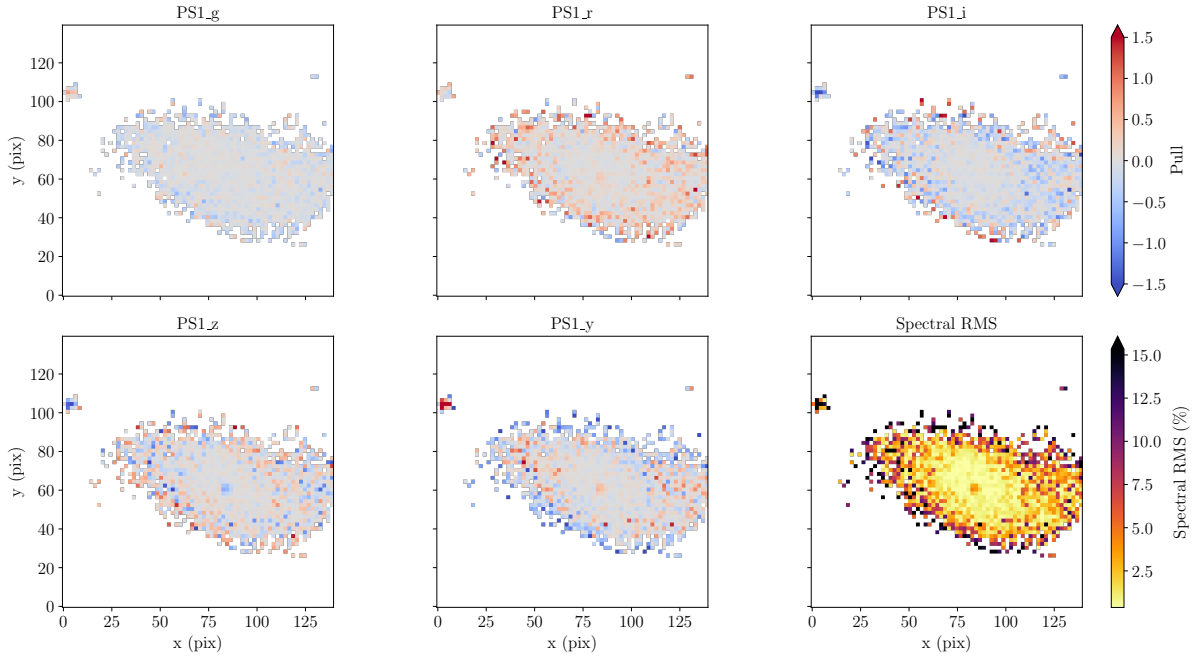
FIGURE 6.7 – Cartographie du pull pour chaque bande PS1 et de la RMS spectrale en sortie de CIGALE
