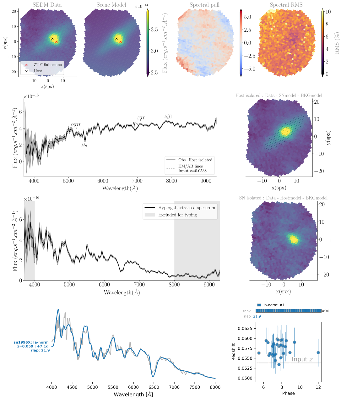
FIGURE 8.19 – Même chose que la Figure 8.18 pour la SN ZTF19abormno. La distance apparente entre la supernova et la galaxie est d'environ 1''5 avec un redshift d'entrée de z_{in} = 0.0538 . Cette supernova est classifiée comme une Ia-norm avec un redshift moyen pondéré par le rlap de \bar{z}_{snid} = 0.058 et nMAD(z_{snid}) = 0.002 .
