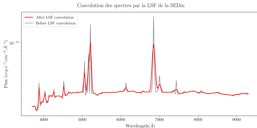
FIGURE 7.7 – Application de la LSF aux spectres du cube intrinsèque obtenue dans le Chapitre 6.3 (Figure 6.9). On montre ici un exemple de la convolution sur le spectre après ré-échantillonnage de la Figure 6.8 (ici en noir ). Le lissage progressif et croissant avec la longueur d’onde dû à la chromaticité de la LSF est clairement visible. Le résultat de la convolution par le kernel variable est représenté par le spectre rouge .
