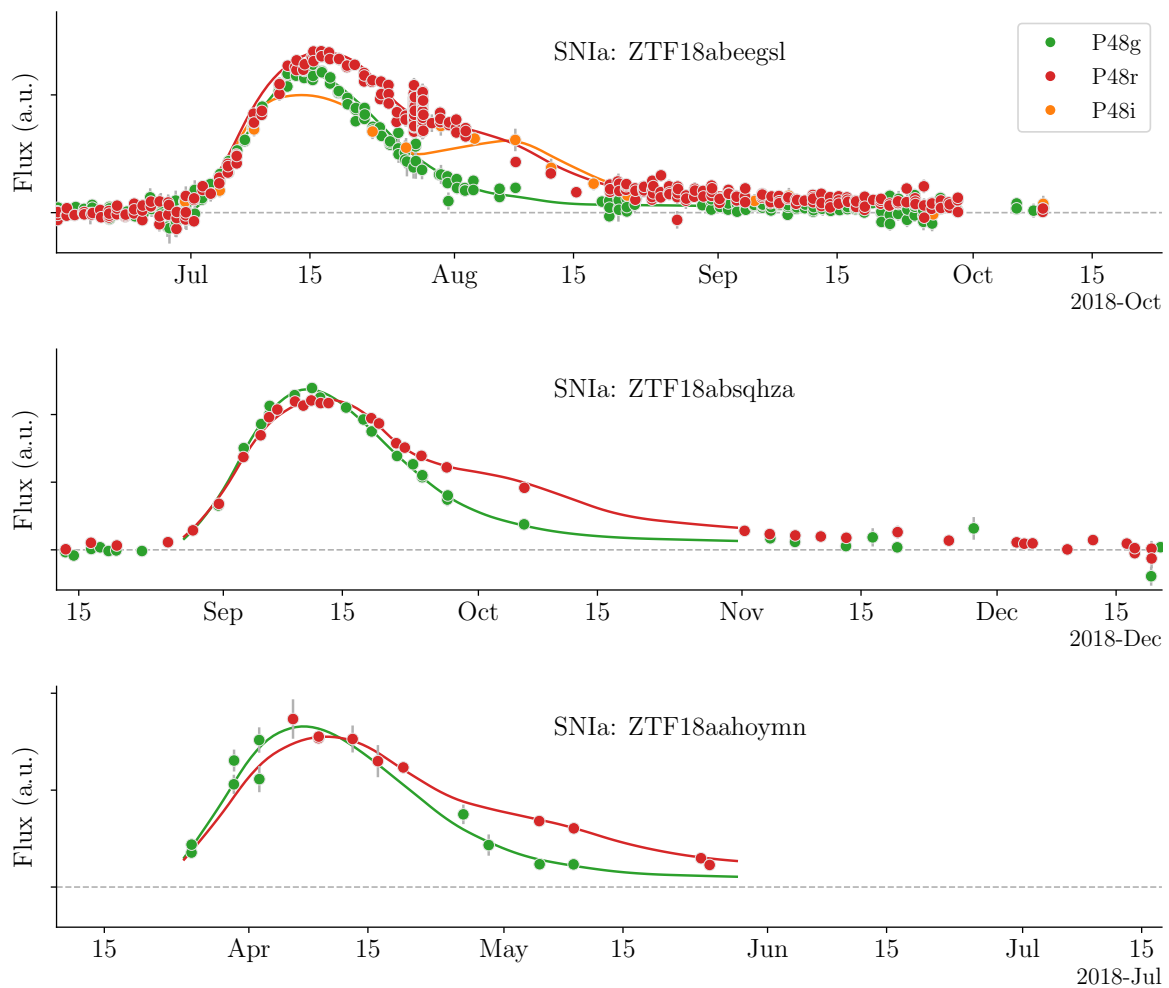
FIGURE 10.8 – Exemples de courbe de lumière de SNeIa du golden sample de la DR2. L'ajustement SALT2 correspondant est également affiché. Le code couleur réfère à la bande ZTF considérée. De haut en bas : Un cas extrême de très haute cadence avec plusieurs centaines de points, un cas typique avec une dizaine (quinzaine) de points avant (après) le maximum, et un cas limite pour intégrer l'échantillon.
