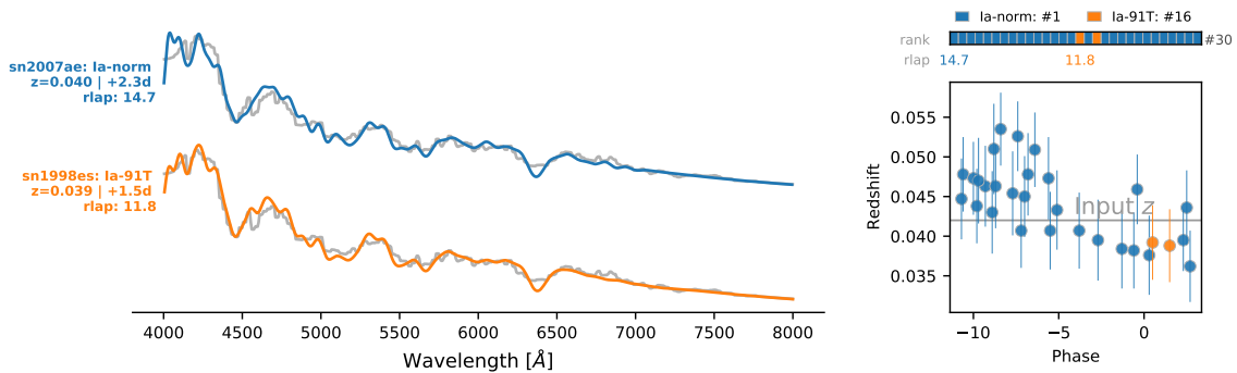
FIGURE 8.17 – Classification de ZTF18accrofrf avec SNID. À gauche, les modèles ayant le plus haut rlap pour chaque sous-type présent dans les 30 meilleurs modèles. Pour chacun je montre le spectre extrait par HYPERGAL en gris, le modèle en couleur, le type et sous-type, le redshift, la phase et le rlap . À droite, la distribution redshift/phase des 30 meilleurs modèles, avec pour le sous-type le même code couleur que pour les spectres de gauche.
