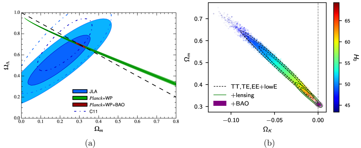
FIGURE 1.7 – (a) Contraintes dans le plan (\Omega_M, \Omega_\Lambda) en combinant les sondes cosmologiques de supernovae de type Ia (JLA, BÉTOULE et al., 2014), du CMB (Planck+WP 2014) et d'oscillations acoustiques des baryons (BAO). Figure de BÉTOULE et al. (2014). (b) Contraintes dans le plan (\Omega_k, \Omega_M) en utilisant le CMB et son lentillage gravitationnelle, et les BAOs. Figure de PLANCK COLLABORATION et al. (2020a).
