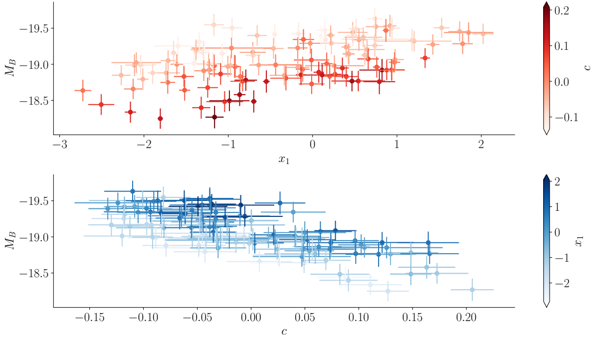
FIGURE 2.6 – Évolution du maximum de luminosité avec le stretch et la couleur pour les SNeIa à bas redshifts de JLA dans la bande B . Le graphe en haut montre l'évolution du pic de magnitude avec le stretch. L'échelle de couleur en rouge indique la couleur, c , associée à chaque SNIa. De même, nous montrons en bas les corrélations avec la couleur, c , où le stretch est indiqué avec l'échelle de couleur bleue.
