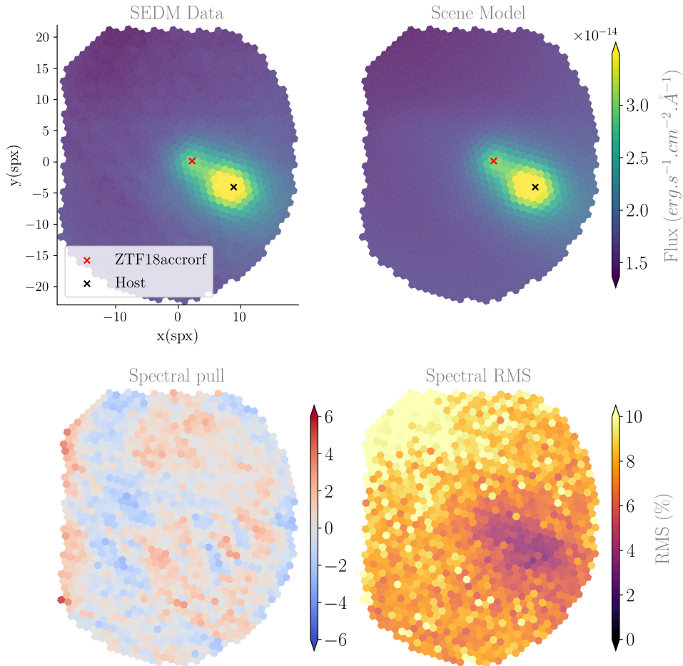
FIGURE 8.9 – Modélisation de scène complète pour ZTF18accrorf. En haut : le cube de données SEDm intégré entre 5000 et 8500 Å, puis le cube modélisé par HYPERGAL intégré également sur le même domaine spectral. La croix rouge indique la position ajustée de ZTF18accrorf à 7000Å et la croix noire la localisation de la galaxie hôte. En bas : le pull spectral tel que défini dans l'équation 8.6, et la RMS spectrale en %. Le pull permet de contrôler la présence éventuelle de structures dans le résidu, ce qui n'est pas le cas ici. La RMS quant à elle nous indique une précision de l'ordre de 4% sur le domaine spectral considéré au niveau des sources présentes dans le champ de vue de la SEDm. Les fluctuations du fond induisent une RMS spectrale de l'ordre de 6-7%, et on peut clairement voir les conséquences de l'artefact en haut à gauche du cube de données.
