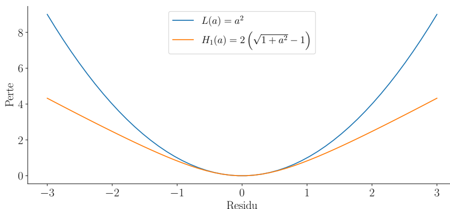
FIGURE 8.8 – Mise en évidence du poids plus faible accordé aux valeurs aberrantes avec la fonction de perte pseudo-Huber d’ordre 1.
