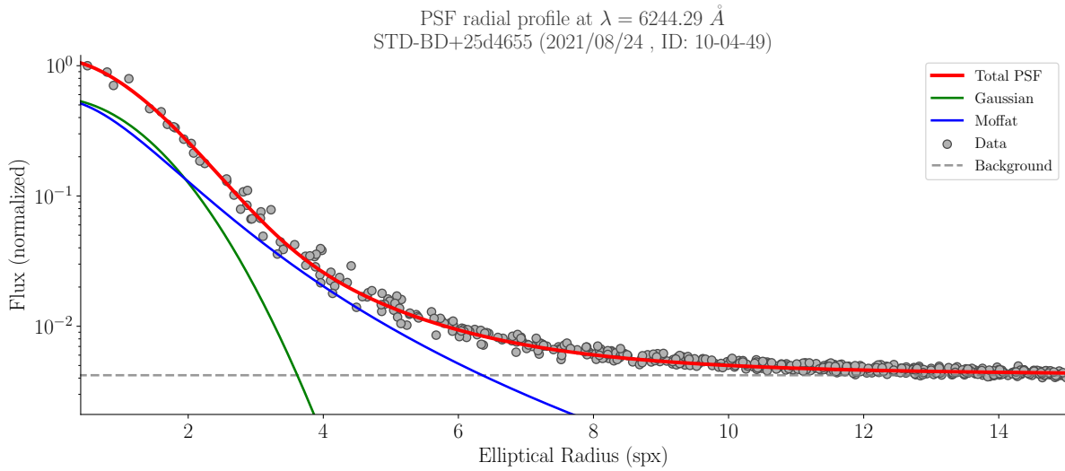
FIGURE 7.8 – Profil radial pour la méta-tranche à 6244\text{\AA} de l'étoile standard 25d4655.
