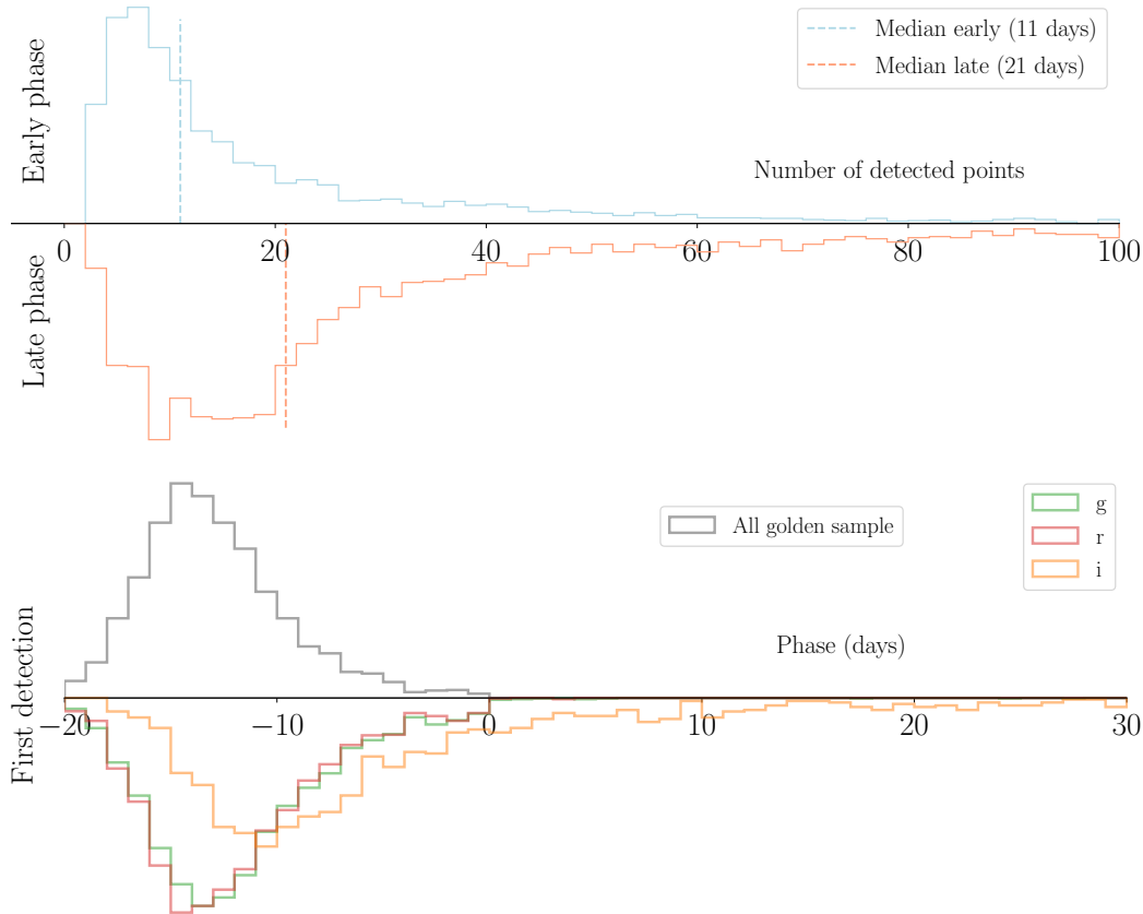
FIGURE 10.9 – En haut : distribution du nombre de points de détection photométrique (toutes bandes confondues) avant et après le maximum de luminosité pour les SNeIa du golden sample de la DR2. On a typiquement \sim 10 points avant le maximum de luminosité, et \sim 20 points après. En bas : distribution de phase de la première détection photométrique pour le même échantillon, toutes bandes confondues (en gris), et dans chaque bande individuelle (couleurs). La première détection survient à une phase médiane de -13.3 jours.
