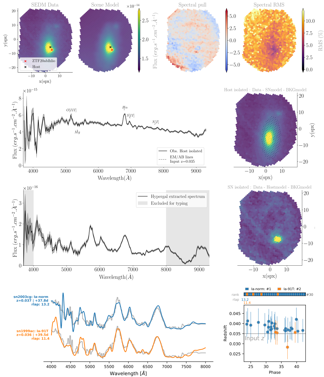
FIGURE 8.20 – Même chose que la Figure 8.18 pour la SN ZTF20abhlhio. La distance apparente entre la supernova et la galaxie est d'environ 1''2 avec un redshift d'entrée de z_{in} = 0.035 . Cette supernova est classifiée comme une Ia-norm avec un redshift moyen pondéré par le rlap de \bar{z}_{snid} = 0.036 et nMAD(z_{snid}) = 0.001 .
