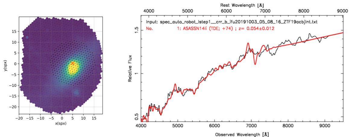
FIGURE 4.7 – Exemple de situation extrême de contamination de supernova par la galaxie hôte : ZTF19acbjlnt, située à \sim 0''.8 du centre. À gauche est représenté une image 2D du cube intégré entre [5000 - 8000]\text{\AA} . La croix orange indique la position estimée de la supernova à partir des images de guidage de la RC. Les marqueurs noirs indiquent les spaxels considérés pour l’extraction de source ponctuelle. À droite le spectre extrait en noir et la tentative de classification par SNID. On voit ici clairement que c’est à la fois le coeur de la galaxie et la supernova qui ont été extraits. L’extraction avec CONTSEP ne change pas le résultat, le module ne faisant pas de distinction entre la SN et la galaxie.
