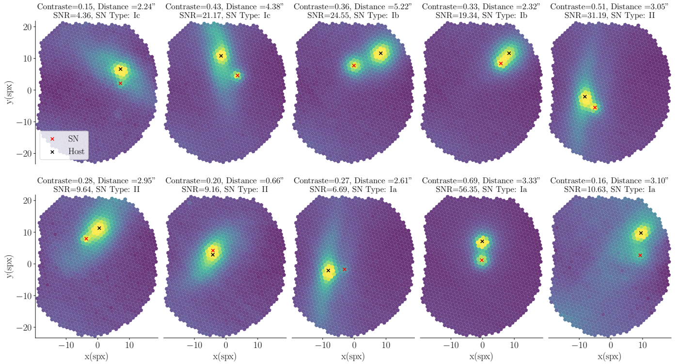
FIGURE 9.6 – Exemples de cubes de simulation pour différentes valeurs de contraste, distance, type de SN et SNR.
