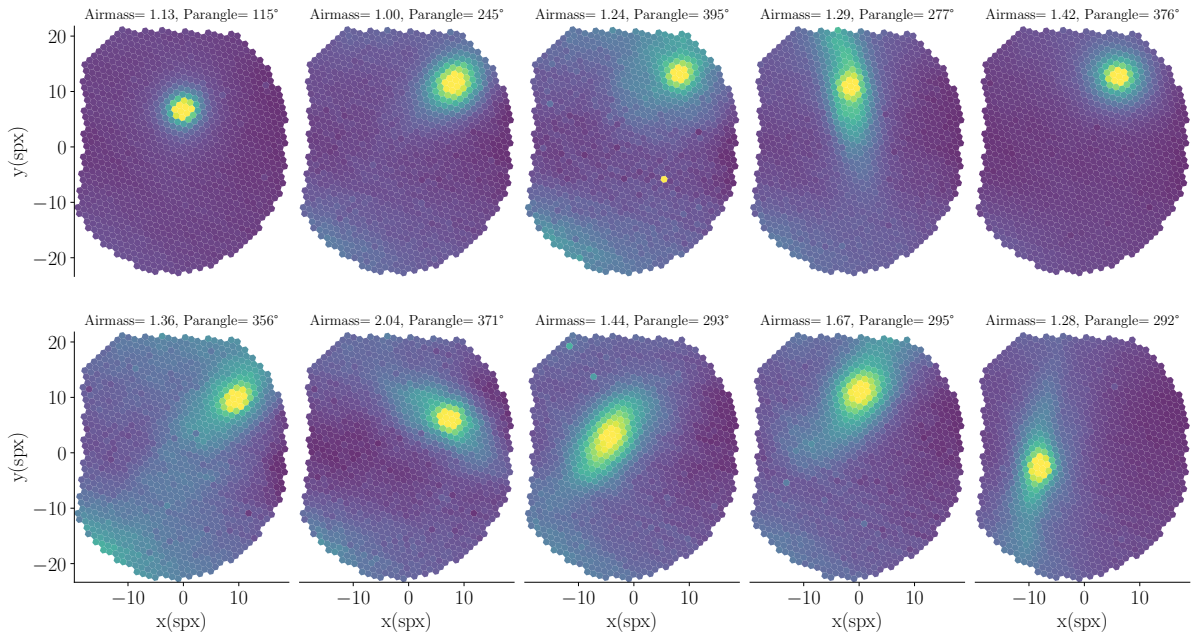
FIGURE 9.1 – Cubes intégrés (sur l’ensemble du domaine spectral de la SEDm) des galaxies hôtes utilisés pour les simulations. Bien que nous n’ayons pas eu l’opportunité d’avoir un grand nombre d’observations de galaxies isolées avec la SEDm, nous avons fait l’hypothèse que les morphologies et localisations variées de ces galaxies étaient suffisamment représentatives des observations pour constituer une base suffisante pour les simulations.
