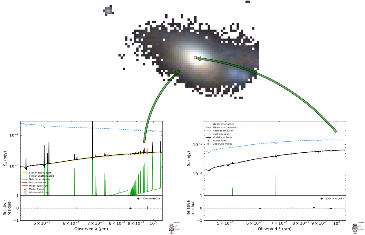
FIGURE 6.6 – Exemples de SED ajustées pour deux pixels. À gauche, un pixel à l'extérieur du coeur de la galaxie, à droite, un pixel à l'intérieur. Les différentes composantes de la SED totale sont indiquées dans les figures de sortie de CIGALE.
