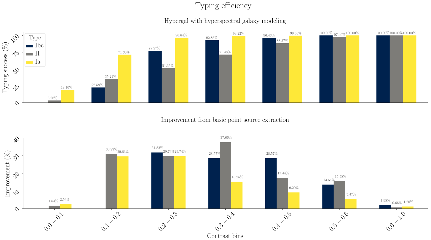
FIGURE 9.14 – Efficacité de classification des simulations. En haut , le pourcentage de classification réussie avec HYPERGAL pour chaque type de supernova et différents intervalles de contraste. Les 4 derniers intervalles sont concaténés car les résultats ne varient plus ou très peu au delà d'un contraste c > 0.6 . En bas , l'amélioration de classification par rapport à la méthode d'extraction simple.
