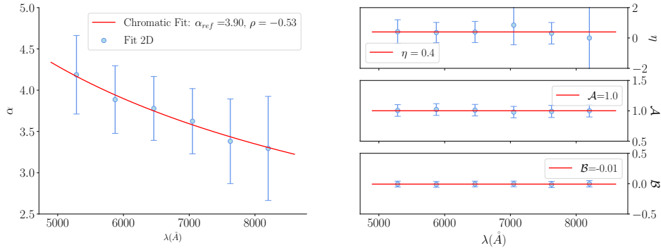
FIGURE 8.5 – Ajustement de la chromaticité des paramètres de forme de la PSF pour la supernova ZTF18accrorf, à partir des 6 méta-tranches. À gauche, l’ajustement du paramètre \alpha avec une loi de puissance. À droite, de haut en bas, l’ajustement par une constante de \eta (poids entre la gaussienne et la Moffat) et des paramètres \mathcal{A} et \mathcal{B} .
