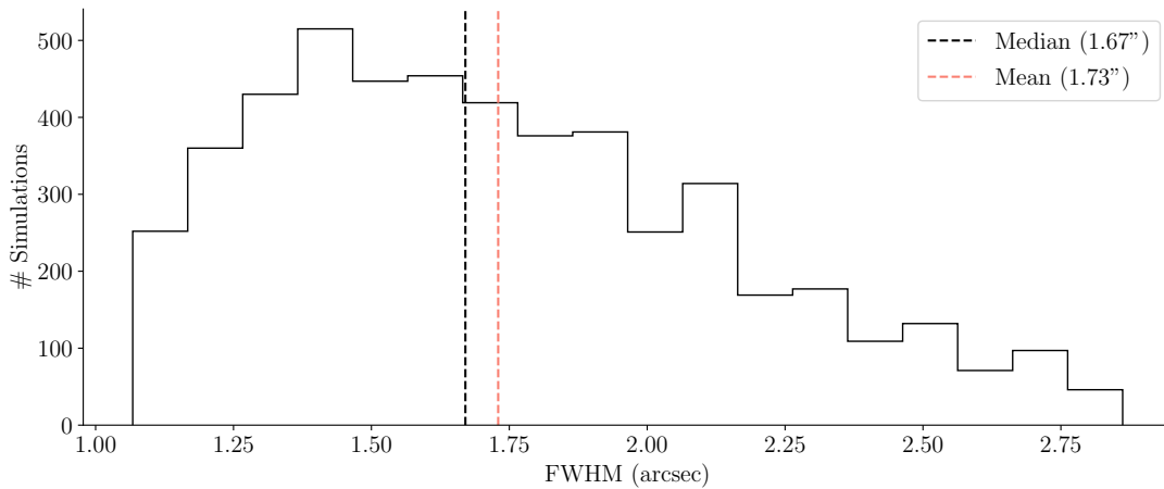
FIGURE 9.4 – Distribution du seeing pour les simulations en arcsec.
