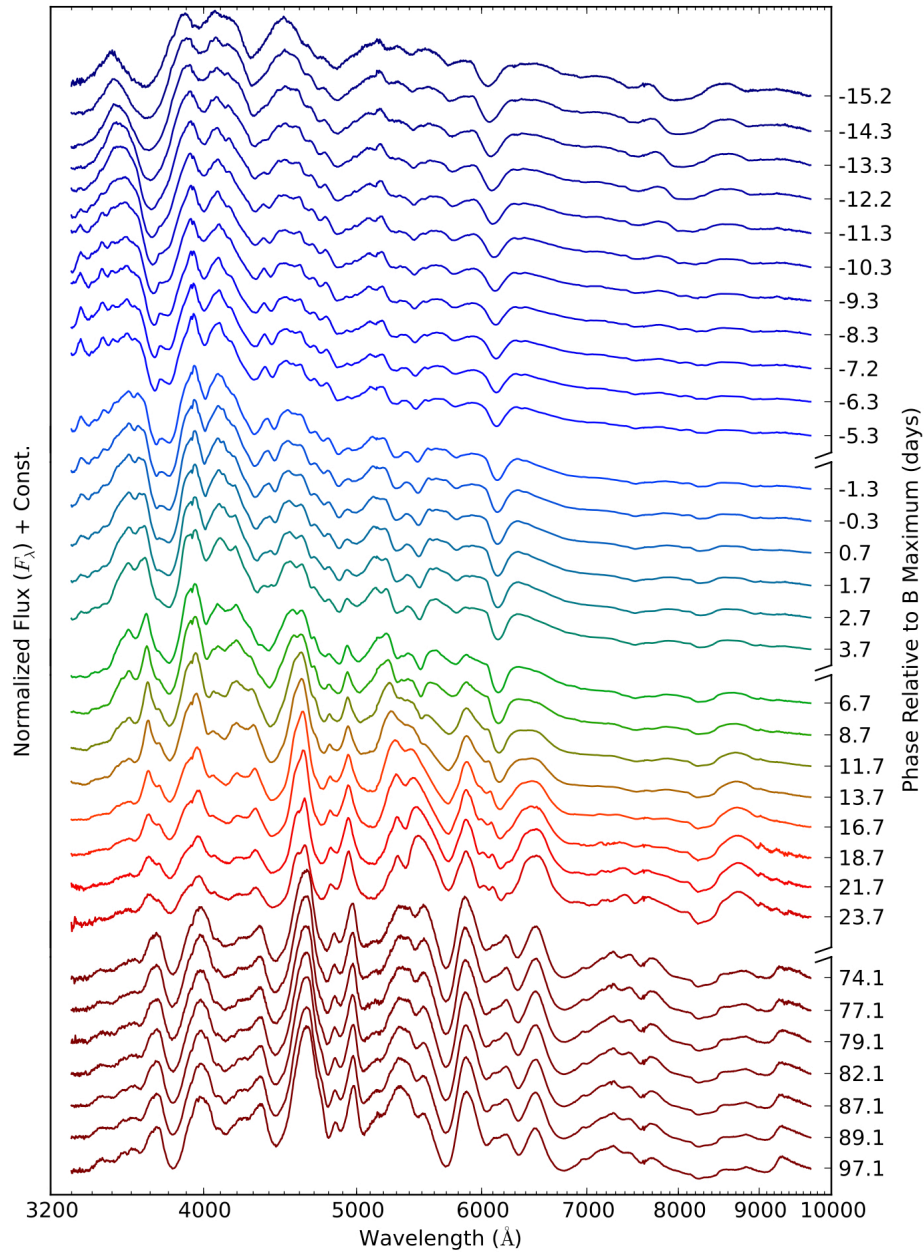
FIGURE 2.3 – Évolution temporelle du spectre de la SNIa SN2011fe entre -15 et +100 jours relativement à la phase 0 (pic de luminosité dans la bande B ). Figure de PEREIRA et al. (2013) , dans le cadre de la collaboration SNFactory.
