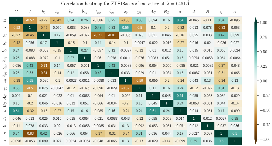
FIGURE 8.4 – Matrice de corrélation des paramètres d’ajustement de scène de ZTF18accrorf pour la méta-tranche à \lambda = 6461\text{\AA} .
