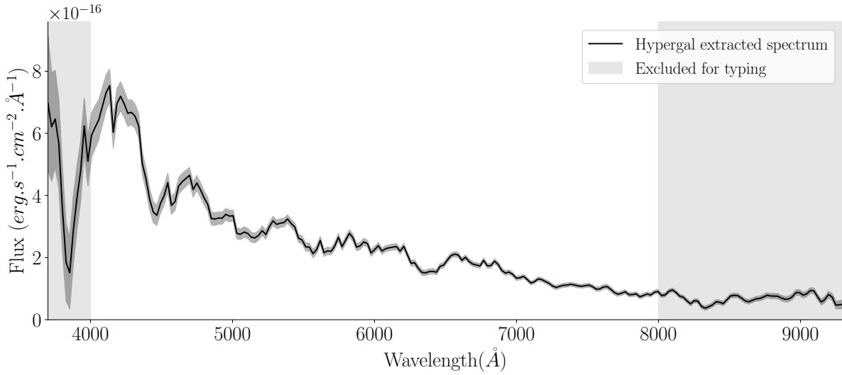
FIGURE 8.13 – Spectre extrait de ZTF18accrorf avec HYPERGAL. Tout le domaine spectral de la SEDm est affiché et les bandes grises indiquent les zones qui ne sont pas utilisées pour la classification de la SN avec SNID.
