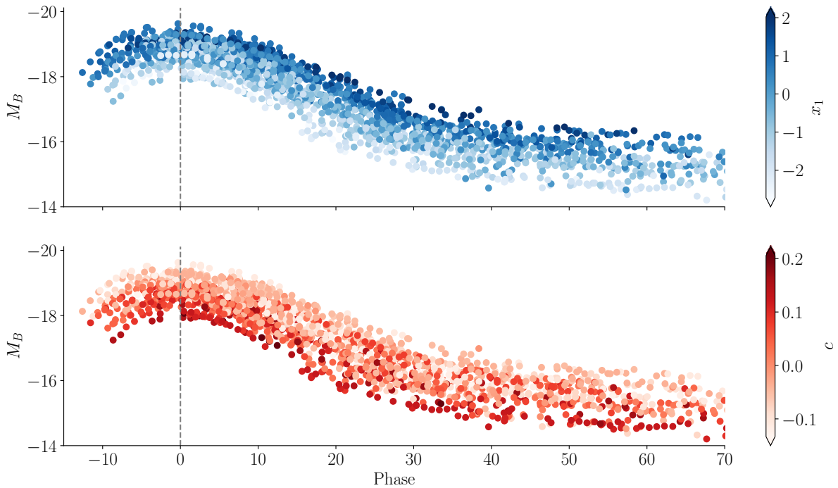
FIGURE 2.5 – Courbes de luminosité absolue de SNeIa à bas redshifts de JLA dans la bande B . La ligne verticale correspond à la phase 0, exprimée en jours sur l'axe des abscisses. L'axe des ordonnées est inversé pour que les fortes luminosité soient vers le haut. En haut , le code couleur indique la valeur de l'étirement temporel x_1 . En bas , on montre les mêmes courbes de lumière mais avec l'information de la couleur c . On notera la dispersion en luminosité de l'ordre de 0.5 mag et surtout la variabilité avec le stretch et la couleur.
