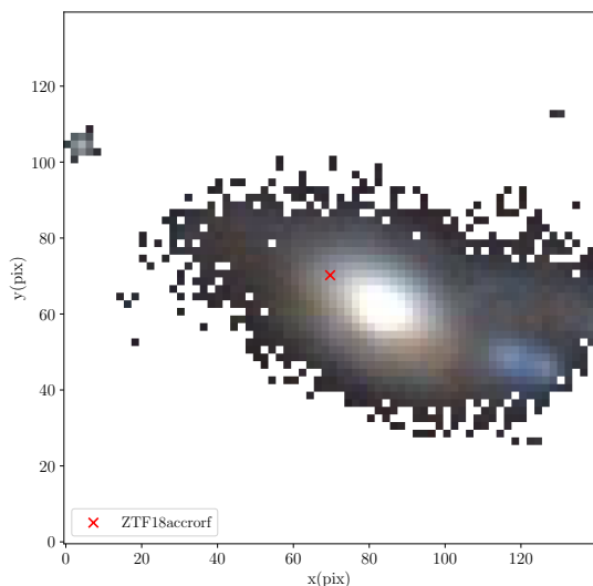
FIGURE 6.5 – Illustration de la coupure \text{SNR} > 3 dans toutes les bandes PS1 avec l’image de la Figure 6.3, après binning 2 \times 2 .
