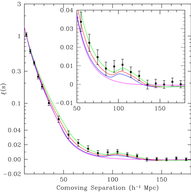
FIGURE 1.5 – Mise en évidence du pic de BAO avec le relevé SDSS. Cette figure de EISENSTEIN et al. (2005) montre la fonction de corrélation à deux points des galaxies du relevé SDSS. Le pic à environ 105 \text{ Mpc} \cdot h^{-1} est clairement visible, et caractérise le pic des BAOs. Les lignes vertes, rouges et bleues correspondent au modèle de concordance \Lambda CDM que nous introduirons plus tard, pour différentes valeurs de \Omega_{M,0}h^2 . La ligne magenta correspond à un modèle sans pic de BAO.
