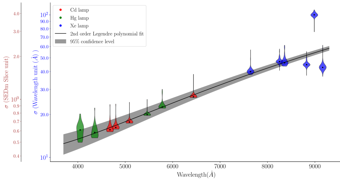
FIGURE 7.5 – Chromaticité de la LSF. On montre ici l'évolution de l'écart type \sigma de la modélisation gaussienne des différentes raies d'émission pour les lampes à arc Cd, Hg et Xe en fonction de la longueur d'onde. L'écart type \sigma est présenté en unité de longueur d'onde ( \lambda[\text{Å}] ) et en unité d'épaisseur de tranche dans les cubes 3D de la SEDm. Cette étude est réalisée à partir des solutions en longueurs d'onde de 65 nuits étalées entre 2018 et 2022. Le code couleur indique la lampe à arc dont est issue la raie d'émission et le modèle quadratique ajusté est présenté en courbe noire.
