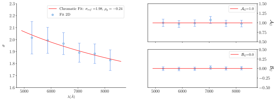
FIGURE 8.6 – Ajustement de la chromaticité des paramètres de forme de la PSF différentielle SEDm/PS1 pour la galaxie hôte de la supernova ZTF18accrorf, à partir des 6 méta-tranches. À gauche, l’ajustement du paramètre \sigma avec une loi de puissance. À droite, de haut en bas, les paramètres \mathcal{A}_G et \mathcal{B}_G .
