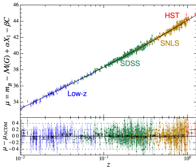
FIGURE 1.6 – Diagramme de Hubble à partir de 740 SNeIa de plusieurs relevés (SDSS, SNLS, HST). La partie haute de cette figure montre l'évolution du module de distance en fonction du redshift des SNeIa de l'échantillon. La courbe noire correspond au modèle cosmologique \Lambda CDM ajusté aux données. La partie du bas montre les résidus entre les données et le modèle \Lambda CDM. Figure de BETOULE et al. (2014).
