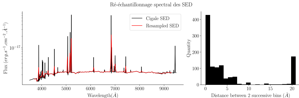
FIGURE 6.8 – Échantillonnage spectral d'une SED obtenue avec CIGALE . À gauche, la SED de sortie de CIGALE entre 3500 et 9500Å (courbe noire) et le ré-échantillonnage dans l'espace spectral de la SEDm (courbe rouge). À droite, l'histogramme de la taille d'échantillonnage de cette SED à la sortie de CIGALE .
