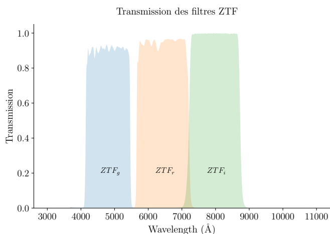
FIGURE 3.5 – Transmission des filtres g , r et i de ZTF (DEKANY et al., 2020).
