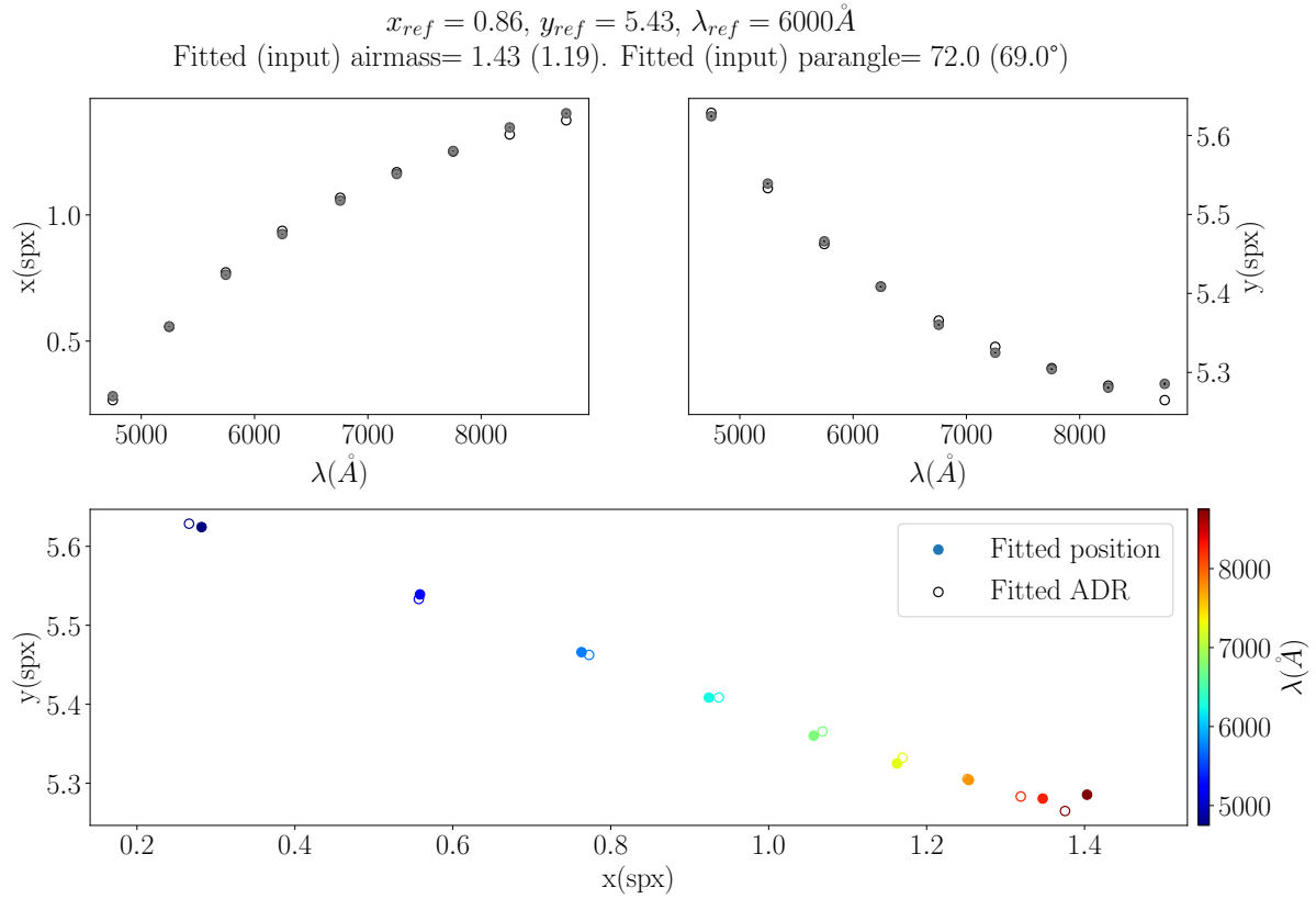
FIGURE 7.17 – Modélisation de la réfraction atmosphérique différentielle pour l'étoile standard 25d4655. Je montre ici l'ajustement du centroïde (x,y) de la PSF par le modèle d'ADR. Les deux graphes du haut représentent l'ajustement des deux coordonnées en fonction de la longueur d'onde. Le graphe du bas illustre l'effet de la réfraction atmosphérique dans le plan du MLA.
