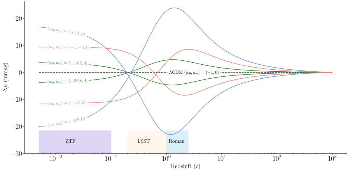
FIGURE 2.7 – Différence de module de distance en fonction du redshift pour différentes équations d'état de l'énergie sombre par rapport à \Lambda CDM ( w = 0 ). Les modèles sont normalisés pour se rejoindre à l'époque du CMB. Nous illustrons ici l'importance des échantillons à bas redshift, et la précision nécessaire sur le module de distance pour détecter une variation de quelques pourcents de w . Les bandes de couleurs sur l'axe des abscisses indiquent la profondeur en redshifts des différents relevés. ZTF est en opération depuis 2018, LSST le sera en 2023 et tous deux sont des relevés sol. Le Nancy Grace Roman Space Telescope sera lancé dans le meilleur des cas en 2027 et sondera le ciel profond jusqu'à des redshifts de l'ordre de z \sim 2.5 .
