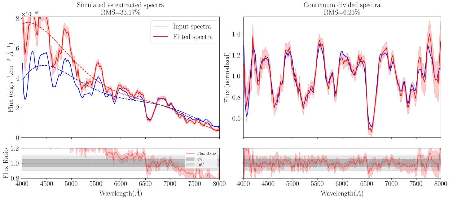
FIGURE 9.10 – Exemple de RMS spectrale après correction du continuum (contraste de 0.27 et une distance hôte/SN de 0.86). À gauche, la comparaison du spectre simulé (en bleu) et du spectre extrait par HYPERGAL (en rouge), ainsi que le rapport entre les flux. On observe un effet de couleur dégradant fortement le RMS spectrophotométrique sur l'intervalle [4000,8000]Å, atteignant plus de 33%. Les courbes en pointillés représentent le continuum ajusté avec un polynôme d'ordre 5. À droite sont présentés les mêmes spectres après division par le continuum. La structure du spectre simulé est très bien retrouvée et cette correction ramène le RMS spectral à \approx 6\% .
