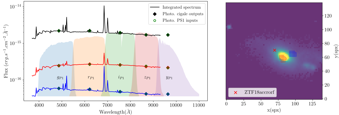
FIGURE 6.9 – Cube intrinsèque de la galaxie hôte de ZTF18accroff. À droite, l'image 2D du cube 3D intégré spectralement. La croix rouge indique la position prédite de ZTF18accroff. Les spaxels sélectionnés en rouge et bleu servent à illustrer l'aspect 3D du cube en montrant la SED correspondante. À gauche sont représentés les spectres intégrés de 3 différentes zones spatiales du cube. Les spectres bleu et rouge correspondent aux spaxels de même couleur, et le spectre noir à l'intégration total. La couverture spectrale des filtres de PS1 est également représentée, avec pour chaque spectre les données photométriques d'entrée (cercles verts) et le résultat obtenu avec CIGALE (losanges) à la longueur d'onde pivot du filtre.
