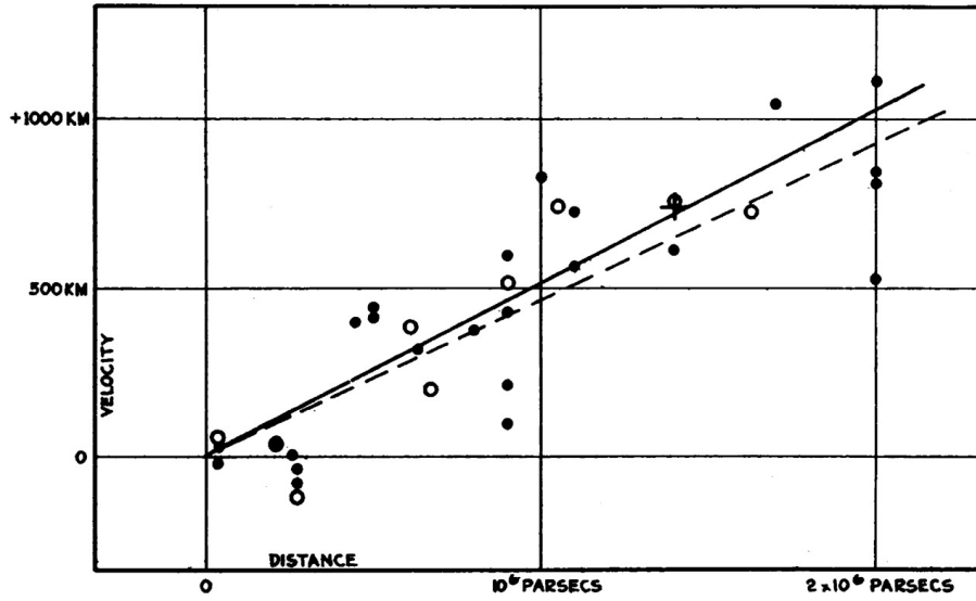
FIGURE 1.3 – Figure originale d’Edwin Hubble (HUBBLE, 1929) de la vitesse d’éloignement, en \text{km.s}^{-1} , de galaxies en fonction de leur distance, en parsecs. Cette première estimation montre une constante de Hubble H_0 \sim 500 \text{ km.s}^{-1}.\text{Mpc}^{-1} .
