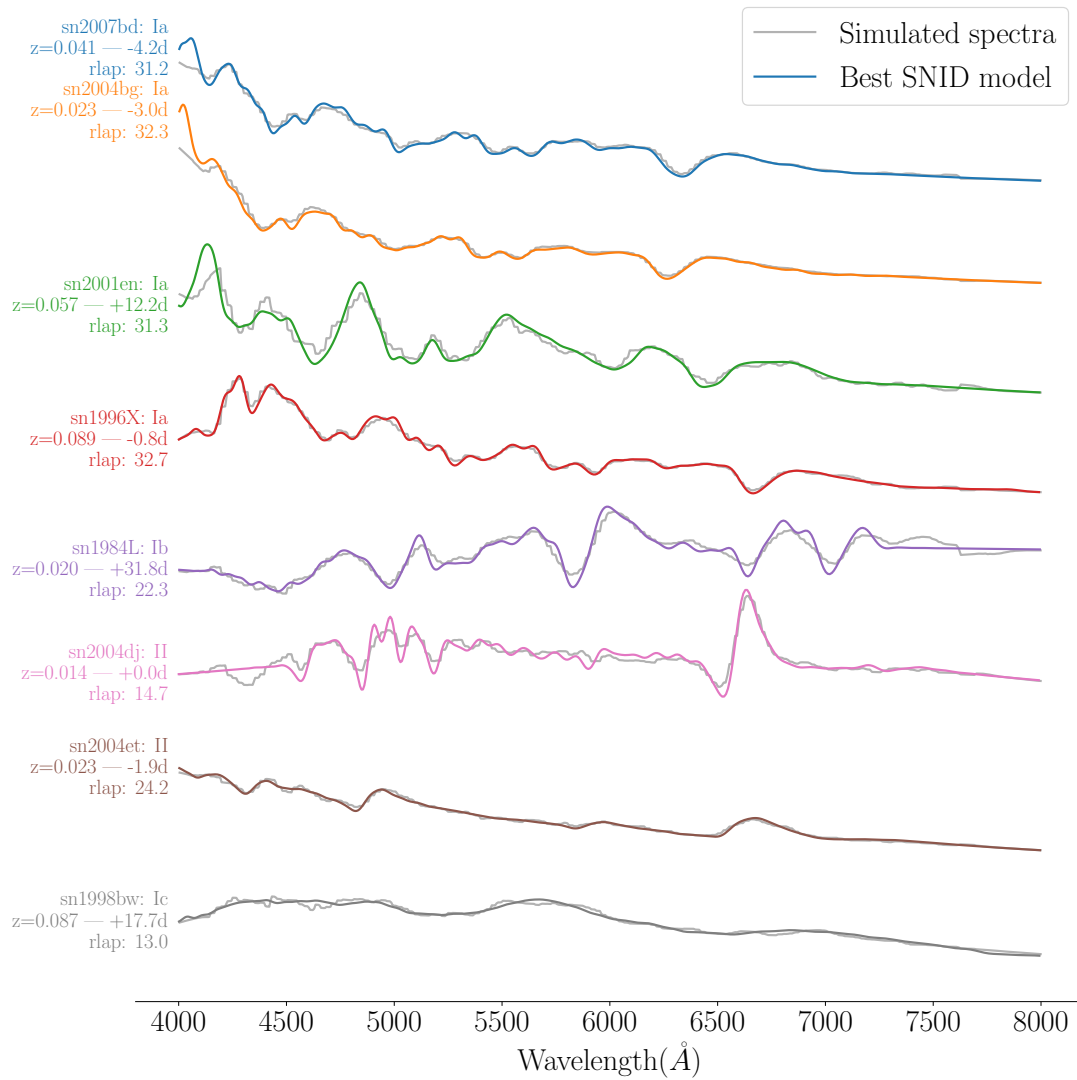
FIGURE 9.2 – Exemple de quelques spectres pour chaque type de supernova pour les simulations : en gris le spectre utilisé pour les simulations qui provient d’une observation de la SEDm et en couleur, le meilleur modèle de classification SNID avec le rlap , le redshift et la phase associés.
