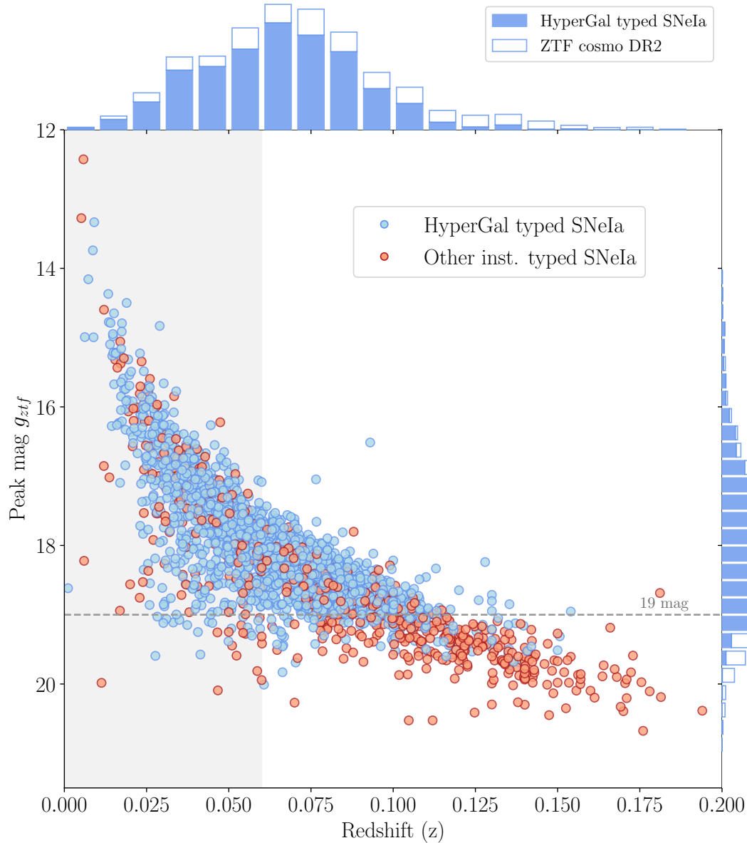
FIGURE 10.7 – Corrélation redshift/pic de magnitude dans la bande g_{ztf} des SNeIa du golden sample de la DR2 de ZTF. J'indique la limite à 19 mag, à laquelle la vaste majorité des classifications a été effectuée grâce à la SEDm et HYPERGAL. La bande grise indique le sous échantillon à volume limité au redshift z = 0.06 , profondeur à laquelle l'échantillon est potentiellement exempt de fonction de sélection.
