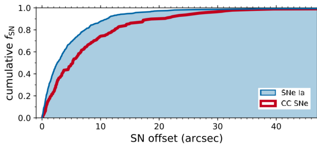
FIGURE 4.6 – Distribution cumulée du décalage angulaire, en secondes d’arc, entre les supernovae de l’échantillon BTS ( Bright Transient Survey ) et leur galaxie hôte. Figure 6 de FREMLING et al. (2020). L’acronyme “CC” fait référence au terme “Core-Collapse”. Les supernovae de type Ia ont un redshift en moyenne plus élevé, ce qui explique cette distribution de plus faible distance angulaire comparée aux autres types.
