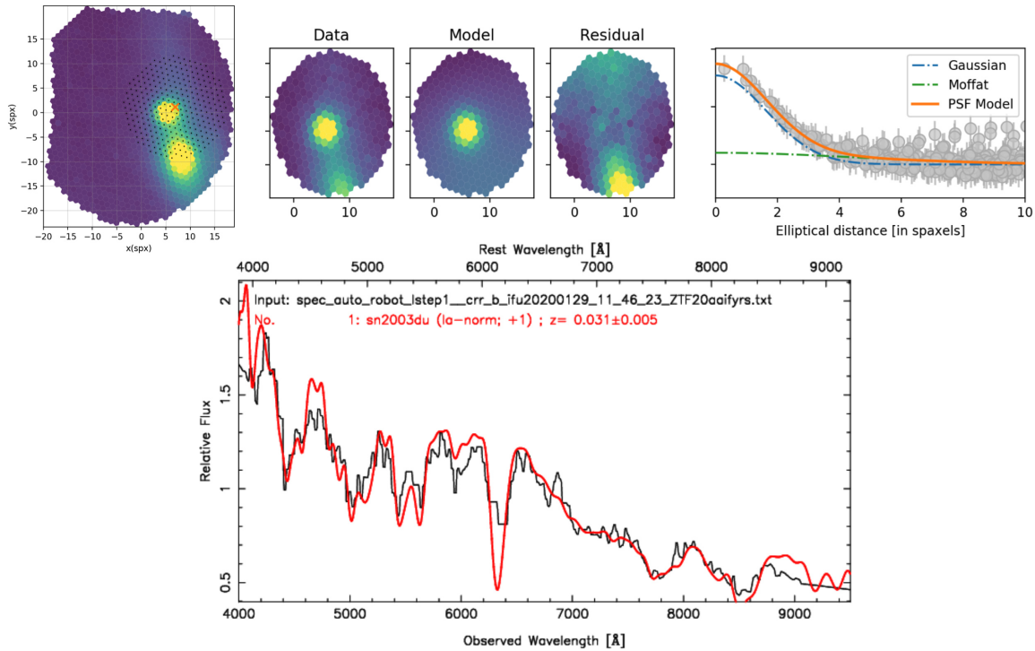
FIGURE 4.5 – Exemple d’extraction de source ponctuelle avec PYSEDM : ZTF20aifys. En haut, de gauche à droite : (a) Image 2D intégrée du cube 3D extrait suivant les étapes de la section 4.2. La croix orange indique la position estimée de la source ponctuelle à partir des images de guidages de la RC (section 4.3.1). Les marqueurs noirs correspondent aux spaxels considérés pour l’extraction de la source. (b) Meta-tranche intégrée entre \lambda = [5750 - 6167]\text{\AA} centrée sur la position estimée de la source ponctuelle et de rayon 10 spaxels. (c) Modèle ajusté avec la composante de fond et la PSF (section 4.3.2). (d) Résidu données-modèle, le signal résiduel en bas correspond à un bout de la galaxie hôte. (e) Profil radial de la source ponctuelle, exprimé en pseudo-ADU (échelle linéaire) en fonction du rayon elliptique après soustraction du modèle de fond. La courbe bleue représente la composante Gaussienne, la courbe verte la Moffat et la courbe orange le profil modélisé total. Les données sont représentées par les marqueurs gris avec leur barre d’erreur. En bas : Spectre extrait en noir et le meilleur modèle de supernova ajusté par SNID en rouge. Ce modèle est celui d’une SNIa proche de son maximum de luminosité (phase p = +1 jour). On peut clairement voir ici que la source ponctuelle extraite est une supernova de type Ia.
