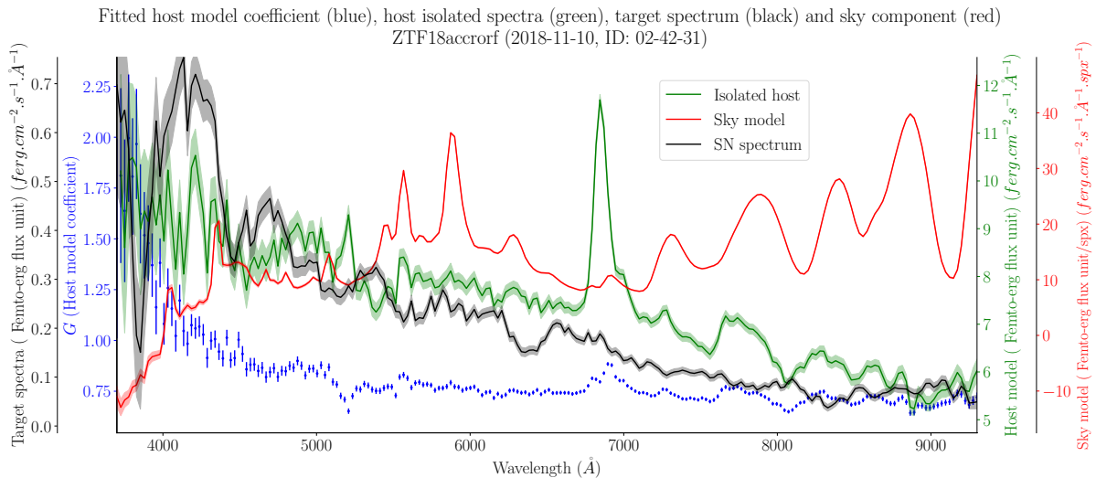
FIGURE 8.14 – Superposition du spectre des 3 composantes de la scène d'observation de ZTF18accrorf : fond de ciel en rouge, galaxie en vert, supernova en noir. Je montre également l'évolution chromatique de l'ajustement du coefficient de correction G du cube intrinsèque. Le but de cette superposition est de mettre en évidence l'absence de contamination évidente entre les spectres, notamment par les raies d'émission de la galaxie. L'évolution du paramètre G montre l'adaptation partielle de l'intensité des raies O[III] et H \alpha aux observations.
