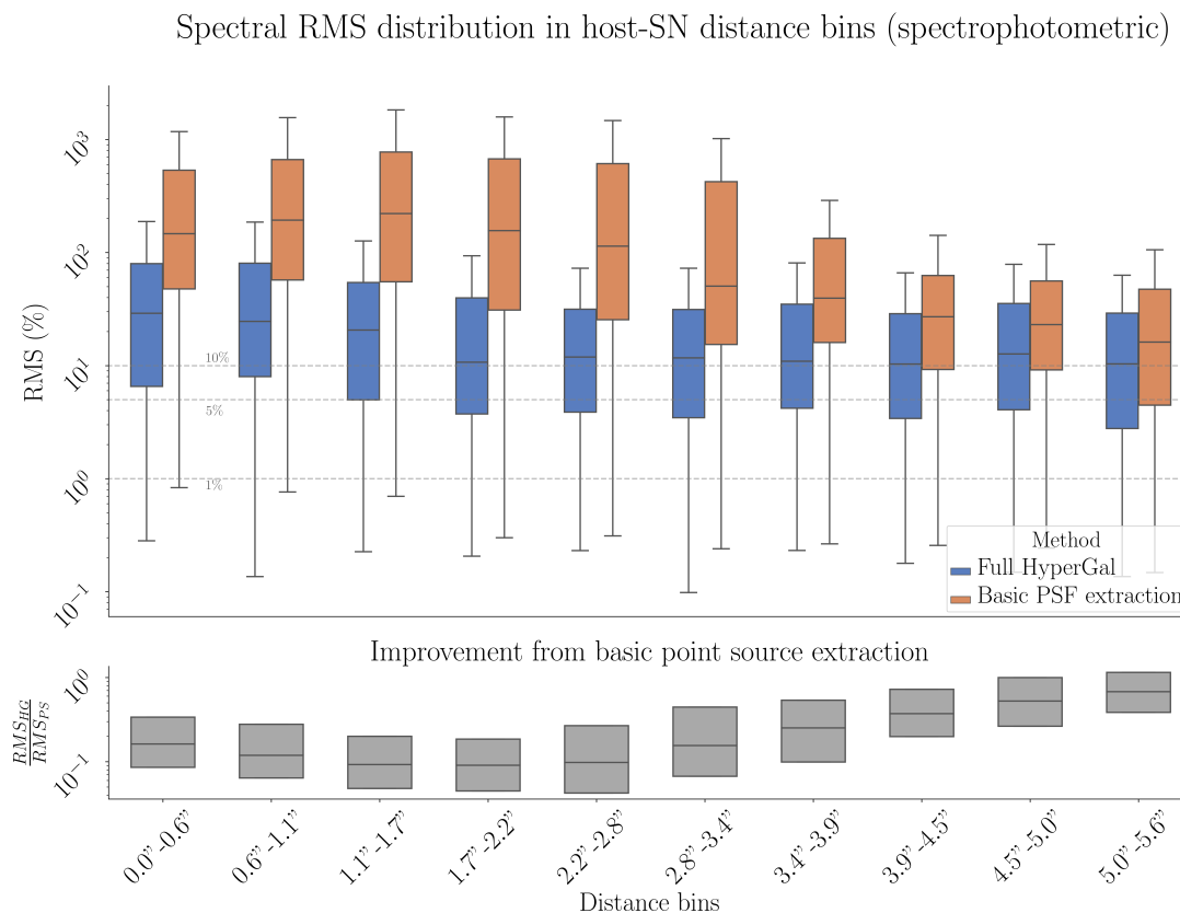
FIGURE 9.9 – Même chose que pour la Figure 9.8 mais en fonction de la distance.
