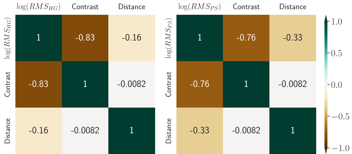
FIGURE 9.7 – Carte des coefficients de corrélation de Pearson des paramètres principaux de la simulation dans l’étude spectrophotométrique. À gauche, les corrélations pour la modélisation de scène complète. La corrélation entre la distance SN-centre de la galaxie et la RMS spectre d’entrée-spectre de sortie est quasiment inexistante pour la méthode HYPERGAL. À droite, les mêmes corrélations pour la méthode d’extraction de référence, sans modélisation hyperspectrale de la galaxie. Bien que modérée, la distance montre une plus forte corrélation avec la RMS pour cette méthode.
