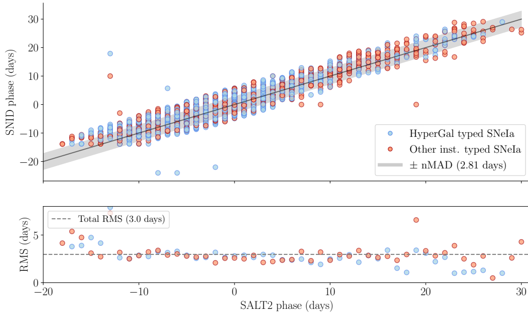
FIGURE 10.11 – En haut : corrélation entre les phases SNID et les phases SALT2 du golden sample de la DR2 de ZTF. La fonction identité est indiquée en noir et le nMAD comme estimateur de la déviation standard. En bas : la RMS par intervalle (1 jour) de phase déterminé avec SALT2, sachant la date d’acquisition spectrale.
