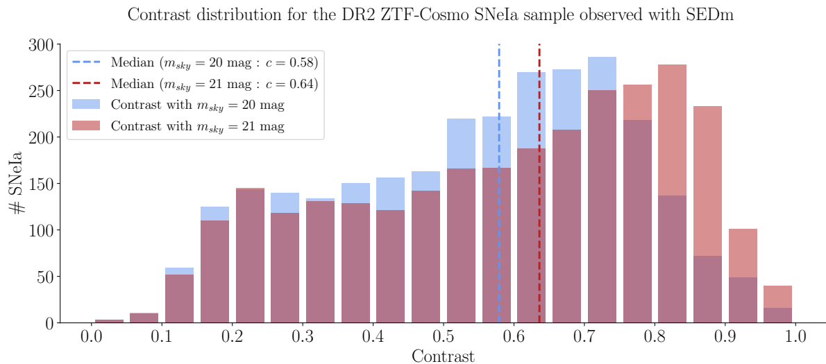
FIGURE 9.12 – Distribution du contraste d’environ 3000 SNeIa de la DR2 de ZTF-Cosmo. Le contraste est calculé à partir d’une ouverture de 2'' dans les images PS1 autour de la SNIa pour la mesure du signal de fond et de la magnitude dans la bande r_{PS1} de la SNIa à partir de l’ajustement SALT2 de la courbe de lumière. Le signal de fond étant mesuré sans la contribution du ciel, je rajoute cette composante à deux valeurs effectives : m_{sky} = 20 pour une valeur réaliste (BLAGORODNOVA et al., 2018), et m_{sky} = 21 pour une valeur conservative.
