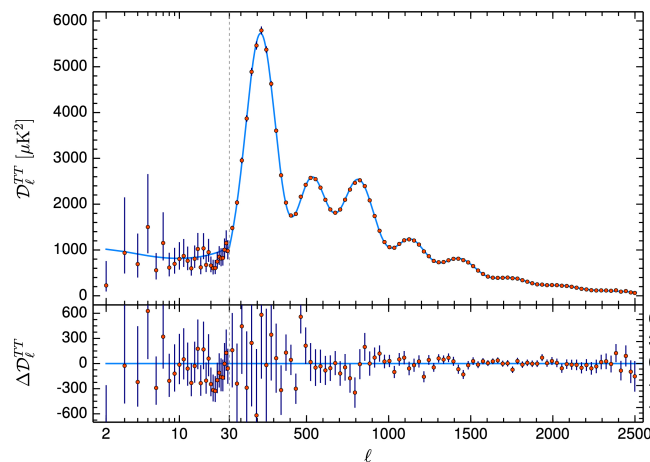
FIGURE 1.4 – Spectre de puissance des anisotropies en température du CMB. L'axe des abscisses représente le multipôle, où les grandes échelles angulaires correspondent à un petit l et inversement. Les points rouges représentent les données, et la courbe bleue le meilleur ajustement du modèle \Lambda CDM. En bas sont illustrés les résidus entre le modèle et les données. Figure de PLANCK COLLABORATION et al. (2020a) .
