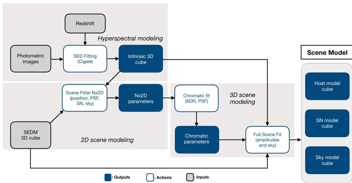
FIGURE 5.2 – Présentation du pipeline HYPERGAL.
