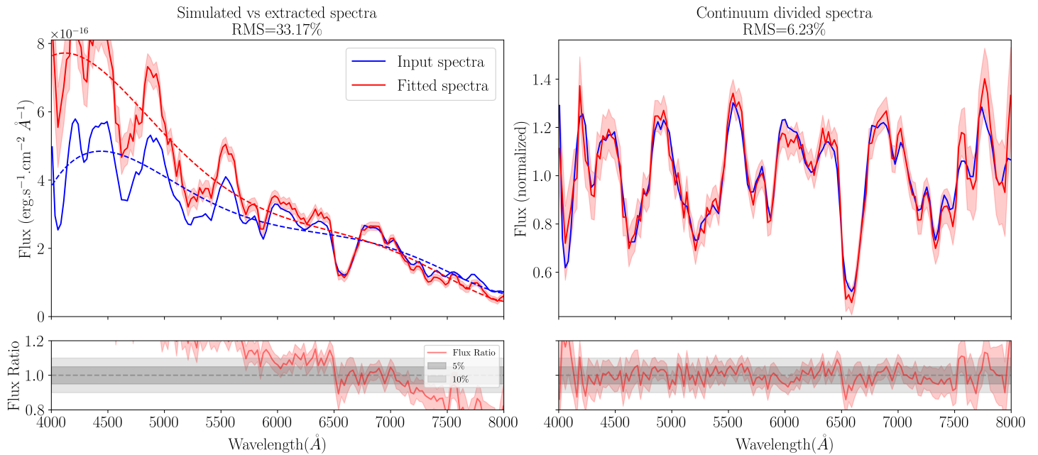
FIGURE 9.10 – Exemple de RMS spectrale après correction du continuum (contraste de 0.27 et une distance hôte/SN de 0.86). À gauche, la comparaison du spectre simulé (en bleu) et du spectre extrait par HYPERGAL (en rouge), ainsi que le rapport entre les flux. On observe un effet de couleur dégradant fortement le RMS spectrophotométrique sur l'intervalle [4000,8000]Å, atteignant plus de 33%. Les courbes en pointillés représentent le continuum ajusté avec un polynôme d'ordre 5. À droite sont présentés les mêmes spectres après division par le continuum. La structure du spectre simulé est très bien retrouvée et cette correction ramène le RMS spectral à \approx 6\% .
