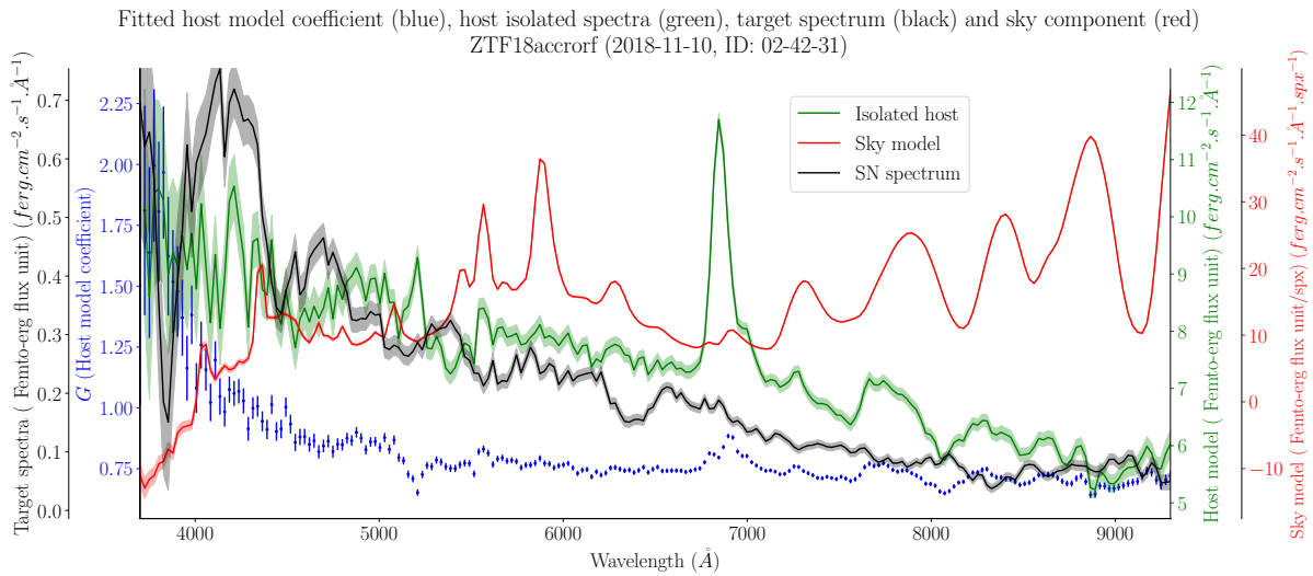
FIGURE 8.14 – Superposition du spectre des 3 composantes de la scène d'observation de ZTF18accrorf : fond de ciel en rouge, galaxie en vert, supernova en noir. Je montre également l'évolution chromatique de l'ajustement du coefficient de correction G du cube intrinsèque. Le but de cette superposition est de mettre en évidence l'absence de contamination évidente entre les spectres, notamment par les raies d'émission de la galaxie. L'évolution du paramètre G montre l'adaptation partielle de l'intensité des raies O[III] et H \alpha aux observations.
