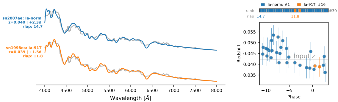
FIGURE 8.17 – Classification de ZTF18accrof avec SNID. À gauche, les modèles ayant le plus haut rlap pour chaque sous-type présent dans les 30 meilleurs modèles. Pour chacun je montre le spectre extrait par HYPERGAL en gris, le modèle en couleur, le type et sous-type, le redshift, la phase et le rlap . À droite, la distribution redshift/phase des 30 meilleurs modèles, avec pour le sous-type le même code couleur que pour les spectres de gauche.
