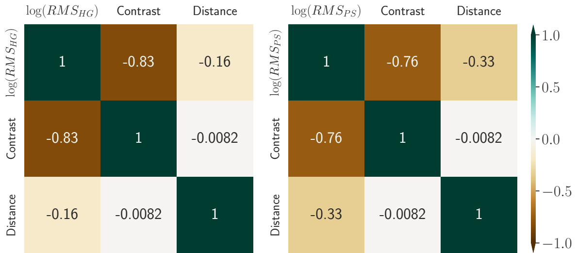
FIGURE 9.7 – Carte des coefficients de corrélation de Pearson des paramètres principaux de la simulation dans l’étude spectrophotométrique. À gauche , les corrélations pour la modélisation de scène complète. La corrélation entre la distance SN-centre de la galaxie et la RMS spectre d’entrée-spectre de sortie est quasiment inexistante pour la méthode HYPERGAL . À droite , les mêmes corrélations pour la méthode d’extraction de référence, sans modélisation hyperspectrale de la galaxie. Bien que modérée, la distance montre une plus forte corrélation avec la RMS pour cette méthode.
