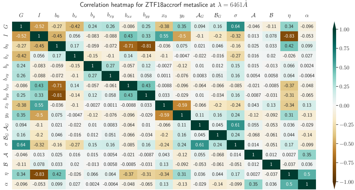
FIGURE 8.4 – Matrice de corrélation des paramètres d’ajustement de scène de ZTF18accrorf pour la méta-tranche à \lambda = 6461\text{\AA} .
