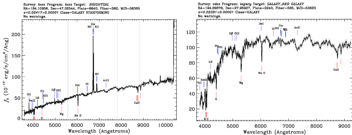
FIGURE 5.1 – Exemple de spectres de galaxies (crédit SDSS). À gauche, le spectre d’une galaxie spirale avec présence d’une forte raie d’émission H\alpha . Cela se traduit par une forte présence d’étoiles jeunes (bleues) et de gaz qui favorise la formation stellaire. À droite, le spectre d’une galaxie elliptique. On peut remarquer d’une part l’absence de raie d’émission H\alpha , d’autre part une forte perte en flux vers 4000Å. Cela trahit la très faible présence d’étoiles jeunes (bleues) dans la galaxie et un faible taux de formation stellaire.
