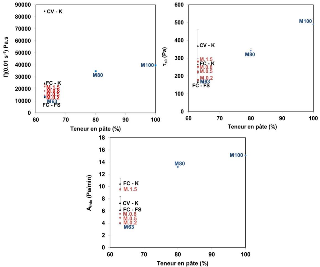
Fig. 2.12 : Paramètres d’ouvrabilité des mélanges étudiés
