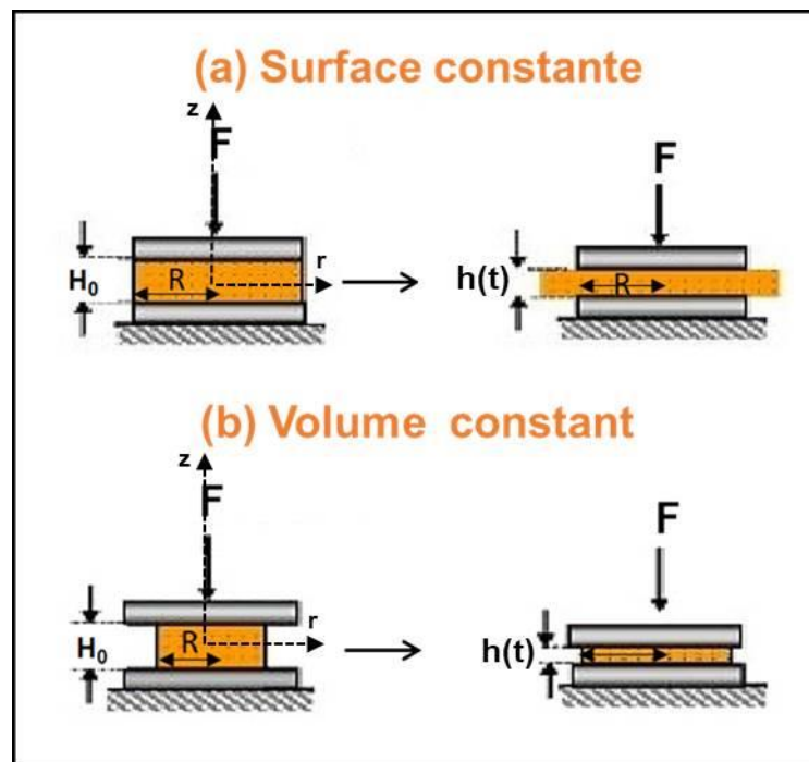
Fig. 4.2 : Configurations géométriques du « squeeze test »
