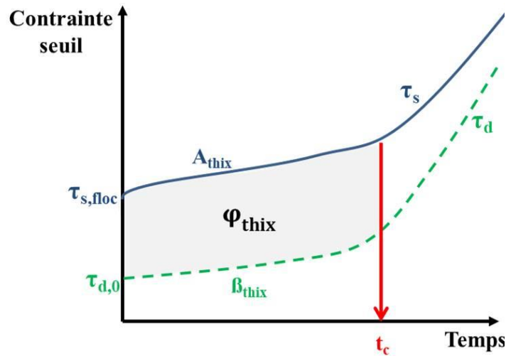
Fig. 3.15 : Représentation de l'indice ( \Phi_{thix} )
