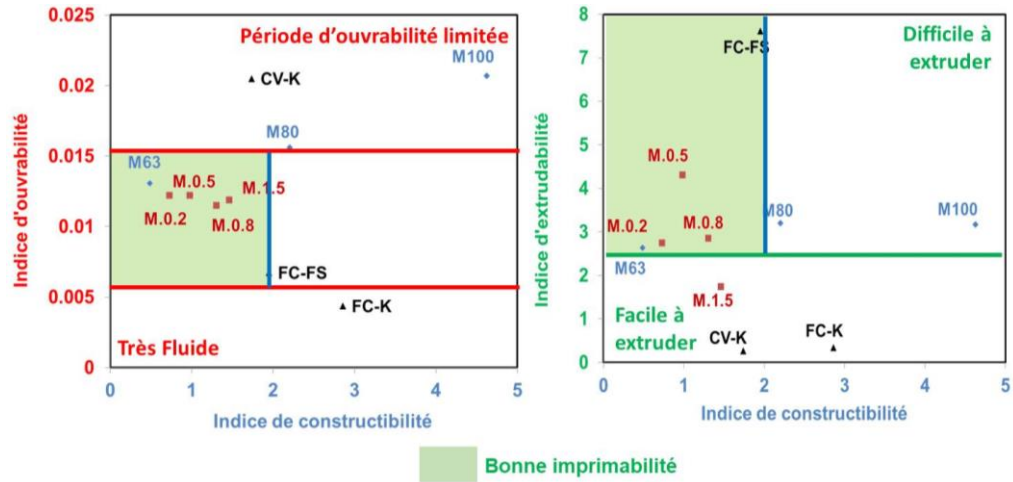
Fig. 2.17 : Paramètres W.E.B des mélanges étudiés
