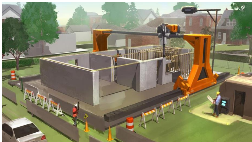
Fig. 1 : Procédé d'impression 3D « Contour Crafting » [3]
