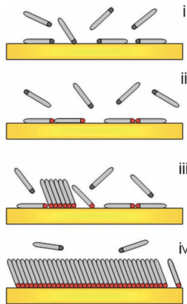
Figure 1. Schéma de la formation de SAMs d'alcanethiolate sur Au(111) : physisorption (i), formation de la phase de dépôt (ii), nucléation de la phase de maintien (iii), achèvement de la phase de maintien (iv). Illustration utilisée avec la permission de la réf. [6]
