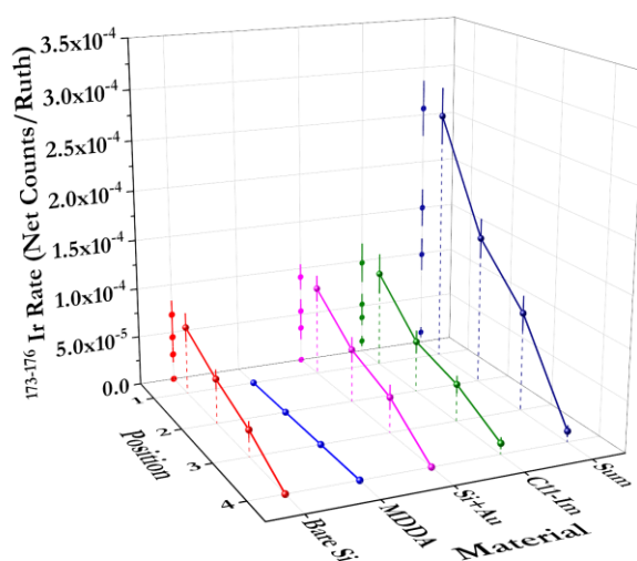
Figure 6. Graphique 3D pour l'activité de ^{173-176}\text{Ir} en fonction de la position du détecteur et de matériaux de détecteur.
