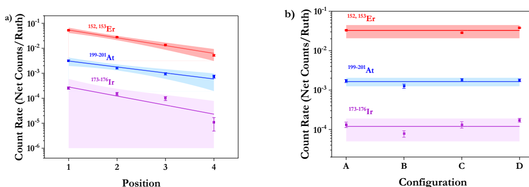
Figure 7. Taux de comptage pour ^{173-176}\text{Ir} , ^{152,153}\text{Er} , et ^{199-201}\text{At} en fonction de: a) la position de détecteur; b) la configuration de détecteur.
