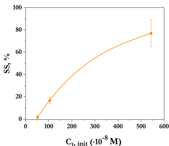
Figure 3 La saturation de surface des SAMs Im-C 11 -SH avec Ir (IV) en fonction de la concentration initiale d'Ir (IV) dans des solutions de HCl 0,55 M.
