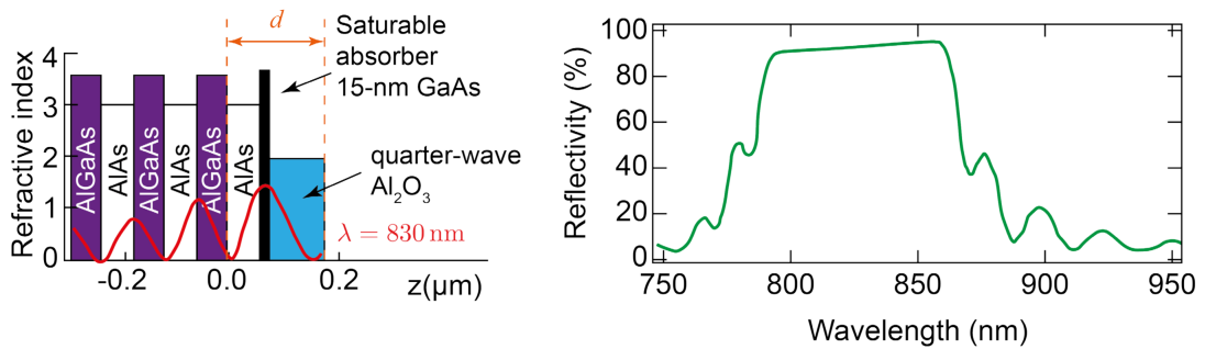
FIGURE 1.20 – Structure miroir absorbant saturable à semiconducteur (SESAM).
