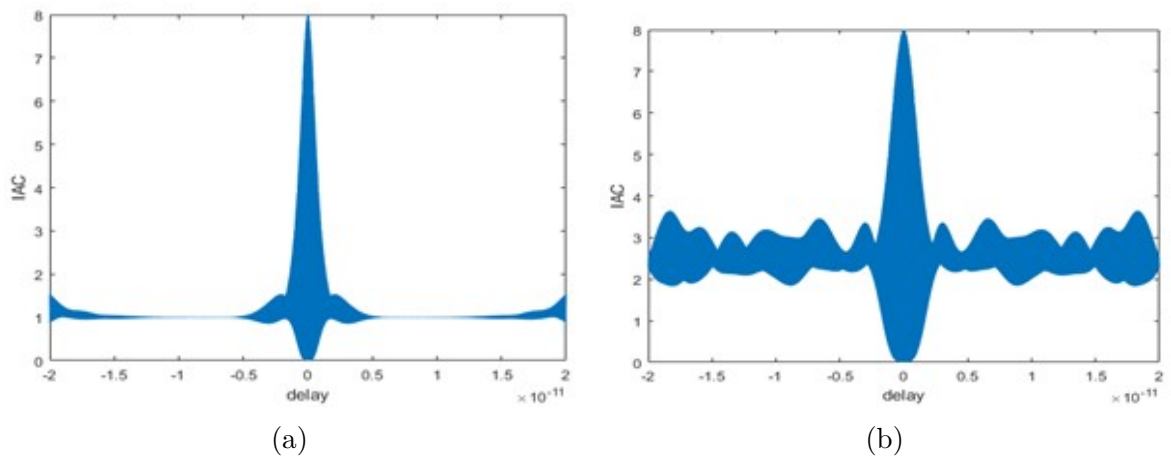
FIGURE 3.6 – IAC simulé pour a_p = 1, 1 , L = 2.6 mm, L_a = 240 \mu\text{m} et a_m de (a) 3,5 et (b) 0,5.
