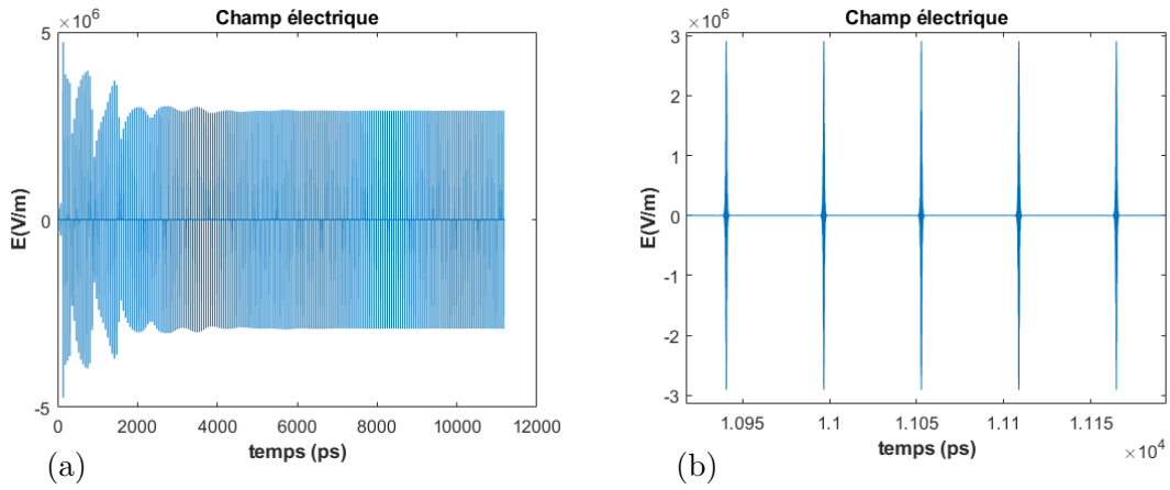
FIGURE 3.20 – Résultat de simulation pour a_m = 5 , a_{p,a} = 0,7 et a_p = 1,6 (a) profil du champ électrique et (b) une fenêtre temporelle contenant cinq impulsions.
