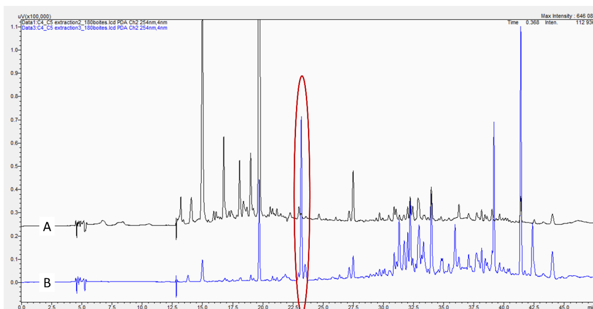
Figure 17 Comparaison des chromatogrammes obtenus par HPLC analytique (observation à \lambda 254 nm) entre les différents extraits de la série 3 de coculture A) extraction AcOEt:CH 2 Cl 2 (v:v) et B) extraction n -hexane
