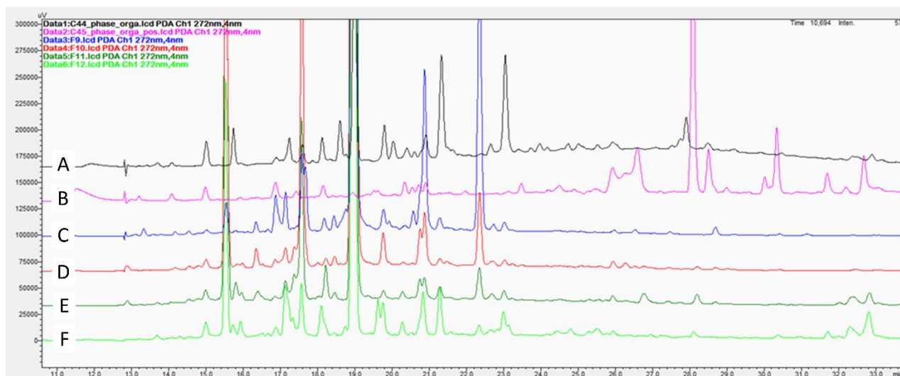
Figure 32 Chromatogrammes des fractionnements obtenus après purification par HPLC-semipréparative. A) extrait brut organique de la monoculture de C44 ; B) extrait brut organique de la monoculture de C45 ; C) fraction F9 ; D) fraction F10 ; E) fraction F11 et F) fraction F12
