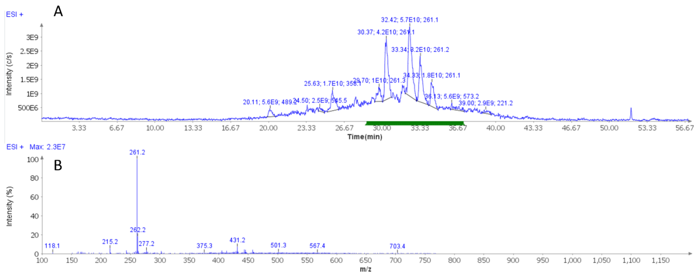
Figure 21 Analyse en HPLC-ESI-MS en mode positif de l'extrait brut de la fraction F6-8. A) chromatogramme de la fraction F6-8 et B) spectre de masse
