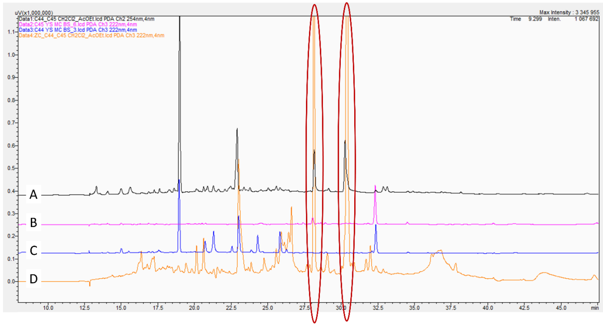
Figure 30 Comparaison des chromatogrammes entre : A) l'extrait brut de la co-culture de la 3ème série ; B) l'extrait de la mono-culture de C45 ; C) l'extrait de la mono-culture de C44 et D) l'extrait de la zone de confrontation entre C44 et C45
