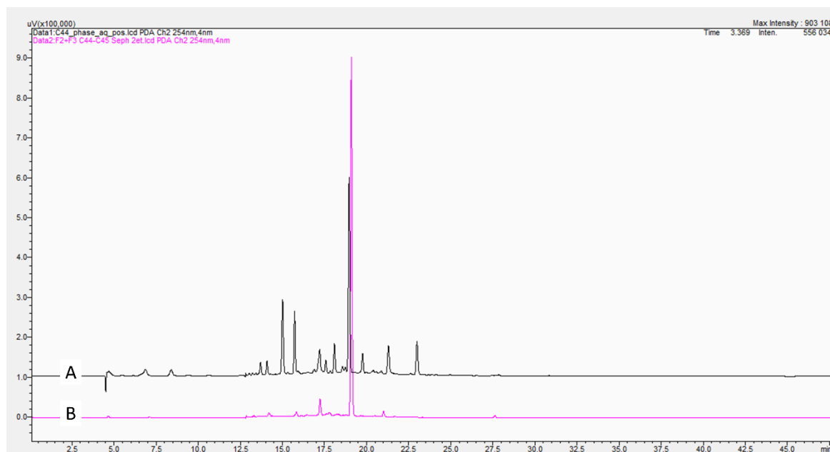
Figure 34 Chromatogrammes de : A) extrait brut aqueux de la mono-culture de C44 et B) fraction F*2 de la co-culture de C44-C45
