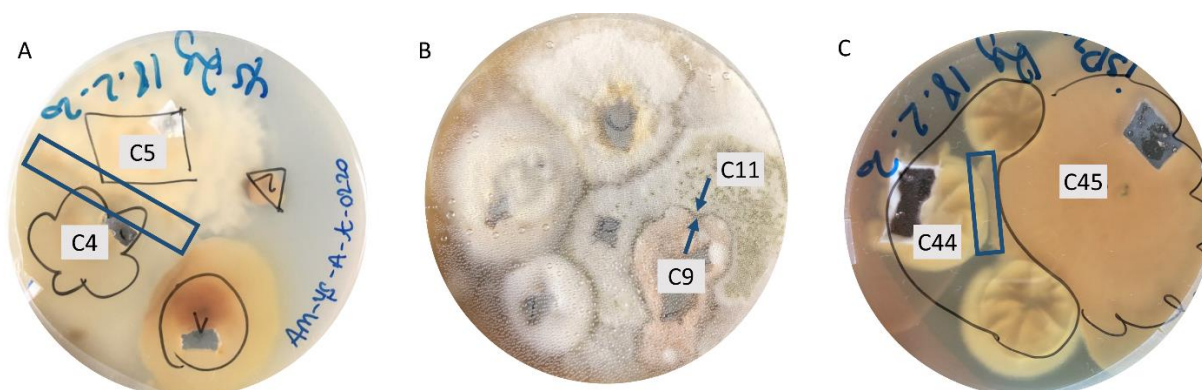
Figure 3 Boîtes de Petri d'isolements issues de la campagne d'hiver 2020. (A) Zone de compétition encadrée en bleu entre Dendrothyrium variisporum C4 et Xylaria hypoxylon C5. (B) Zone de compétition fléchée en bleu entre Coccinonectria rusci C9 et Melanconium hedericola C11. (C) Zone de compétition encadrée en bleu entre Microdochium phragmitis C44 et Tolypocladium sp. C45.
