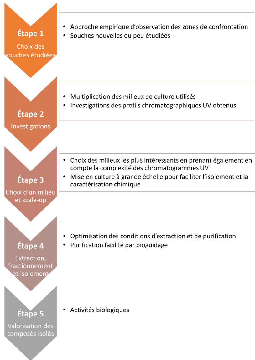
Figure 6 « Workflow » suivi pour l'étude chimique des champignons lichéniques
