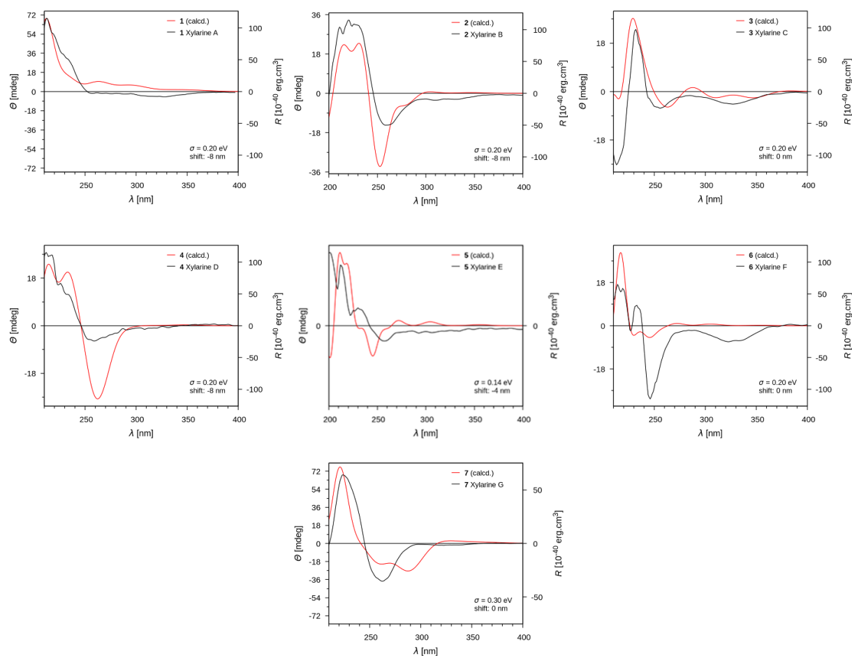
Figure 26 Superposition des spectres DCE expérimentaux et calculés pour la configuration 1R, 4S, 5R, 7S pour les composés 1-7
