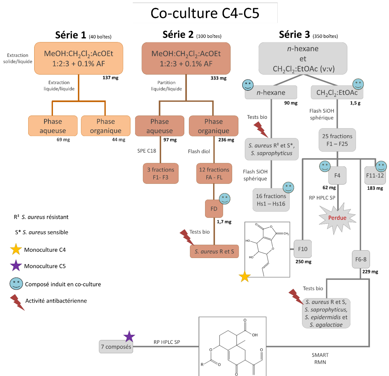
Figure 16 Fractionnement et purification des extraits bruts de la co-culture C4-C5 et évaluation biologique de certaines fractions
