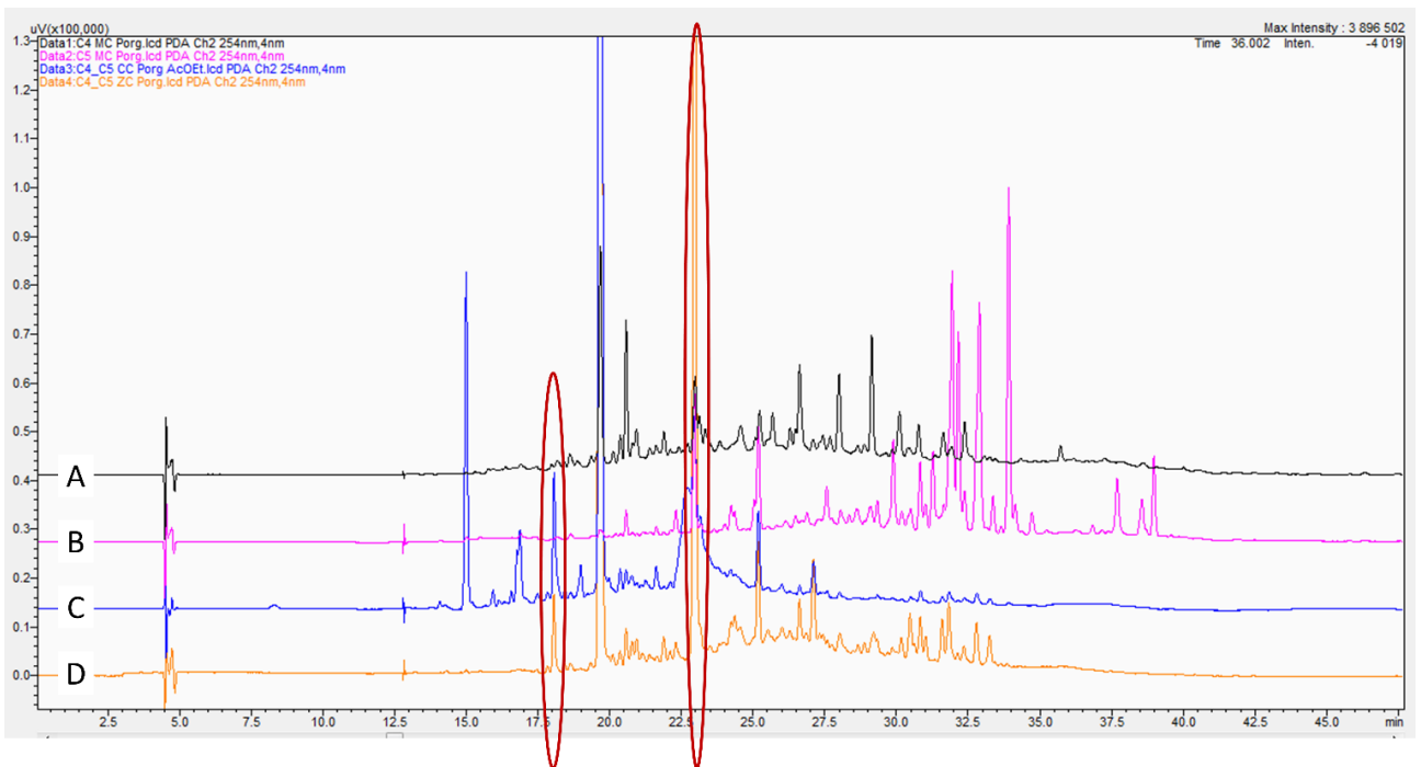
Figure 15 Comparaison des chromatogrammes obtenus par HPLC analytique (observation à \lambda 254 nm) entre les mono- (20 boîtes) et co-cultures (40 boîtes) A) C4 monoculture ; B) C5 monoculture, C) C4-C5 coculture et D) zone de confrontation de la coculture C4-C5
