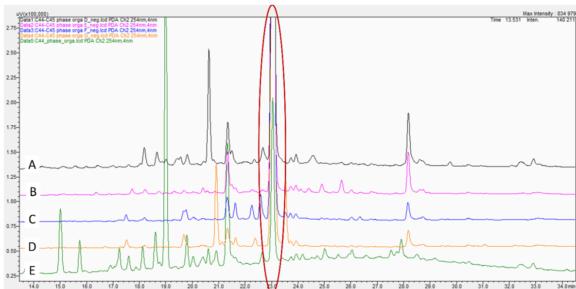
Figure 33 Chromatogrammes A) fraction 4 de l'extrait brut organique de la co-culture C44-C45 ; B) fraction 5 de l'extrait brut organique de la co-culture C44-C45 ; C) fraction 6 de l'extrait brut organique de la co-culture C44-C45 et D) fraction 7 de l'extrait brut organique de la co-culture C44-C45 et E) extrait brut organique de la mono-culture C44
