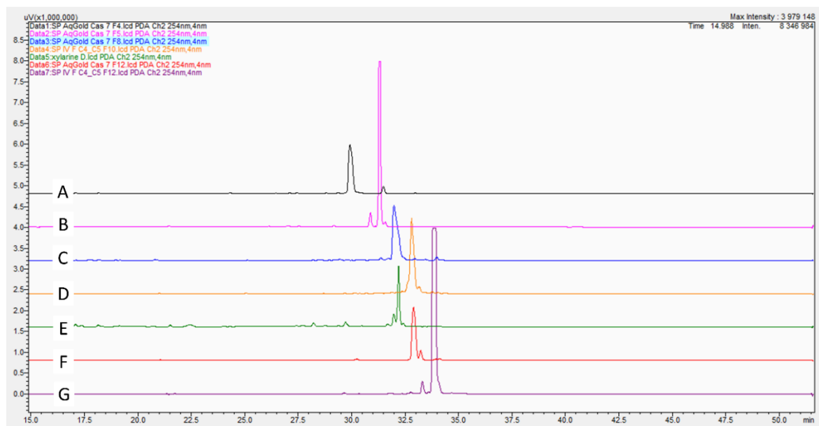
Figure 22 Chromatogrammes de la série de sept molécules obtenues après purification de la fraction F6-8. A) xylarine A 1 ; B) xylarine B 2 ; C) xylarine C 3 ; D) xylarine D 4 ; E) xylarine E 5 ; F) xylarine F 6 ; G) xylarine G 7
