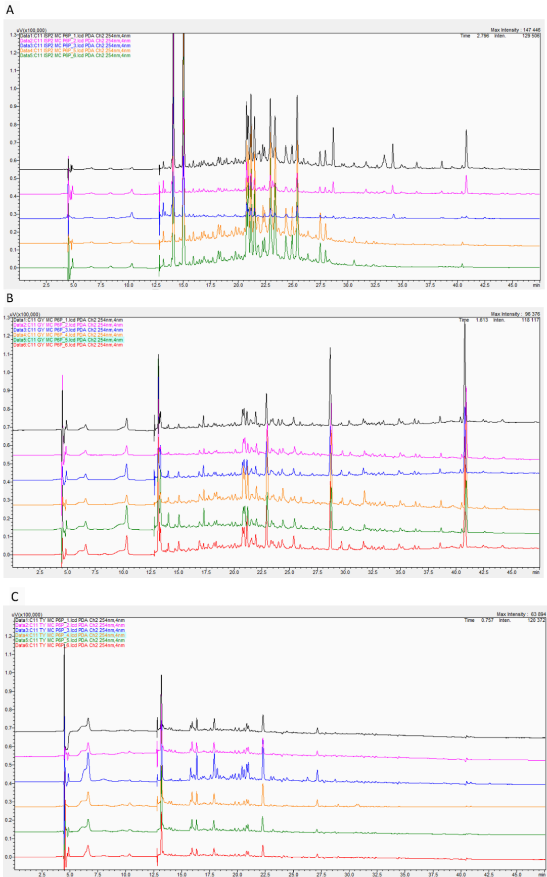
Figure 9 Chromatogrammes obtenus par HPLC-DAD analytique (observation à \lambda 254 nm) des répliques de co-culture en plaque 6 puits pour A) C11 sur le milieu ISP2 ; B) C11 sur le milieu GY et C) C11 sur milieu TY.
