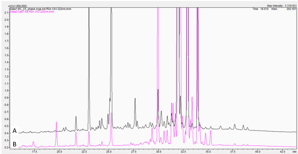
Figure 23 Comparaison des chromatogrammes entre A) l'extrait de monoculture de C5 et B) la fraction F6-8
