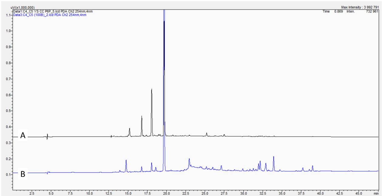
Figure 14 Comparaison des chromatogrammes en fonction du support de culture : A) co-culture C4-C5 en plaque 6 puits et B) co-culture de C4-C5 en boîtes de Petri classique à grande échelle (100 boîtes)
