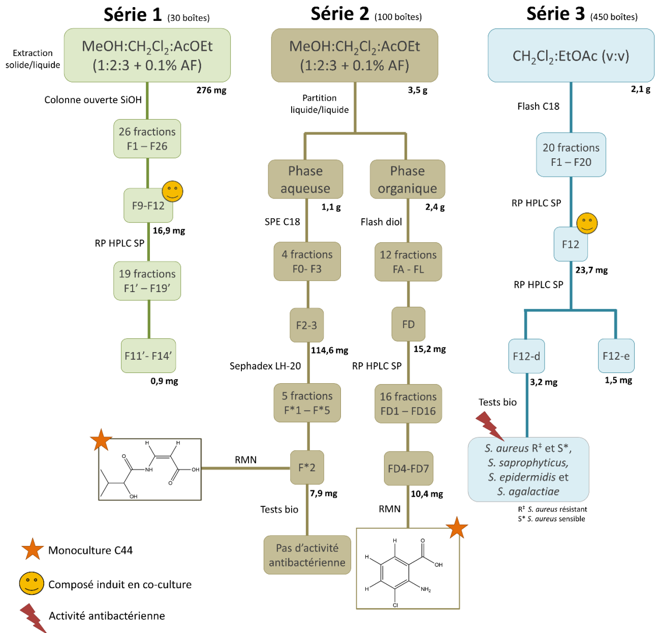
Figure 31 Fractionnements et purification des extraits bruts de la co-culture C44 – 45 et évaluation biologique de certaines fractions
