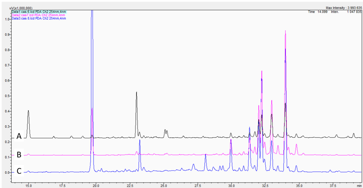
Figure 20 Chromatogrammes obtenus par HPLC analytique (observation à \lambda 254 nm) A) fraction F6; B) fraction F7 et C) fraction F8
