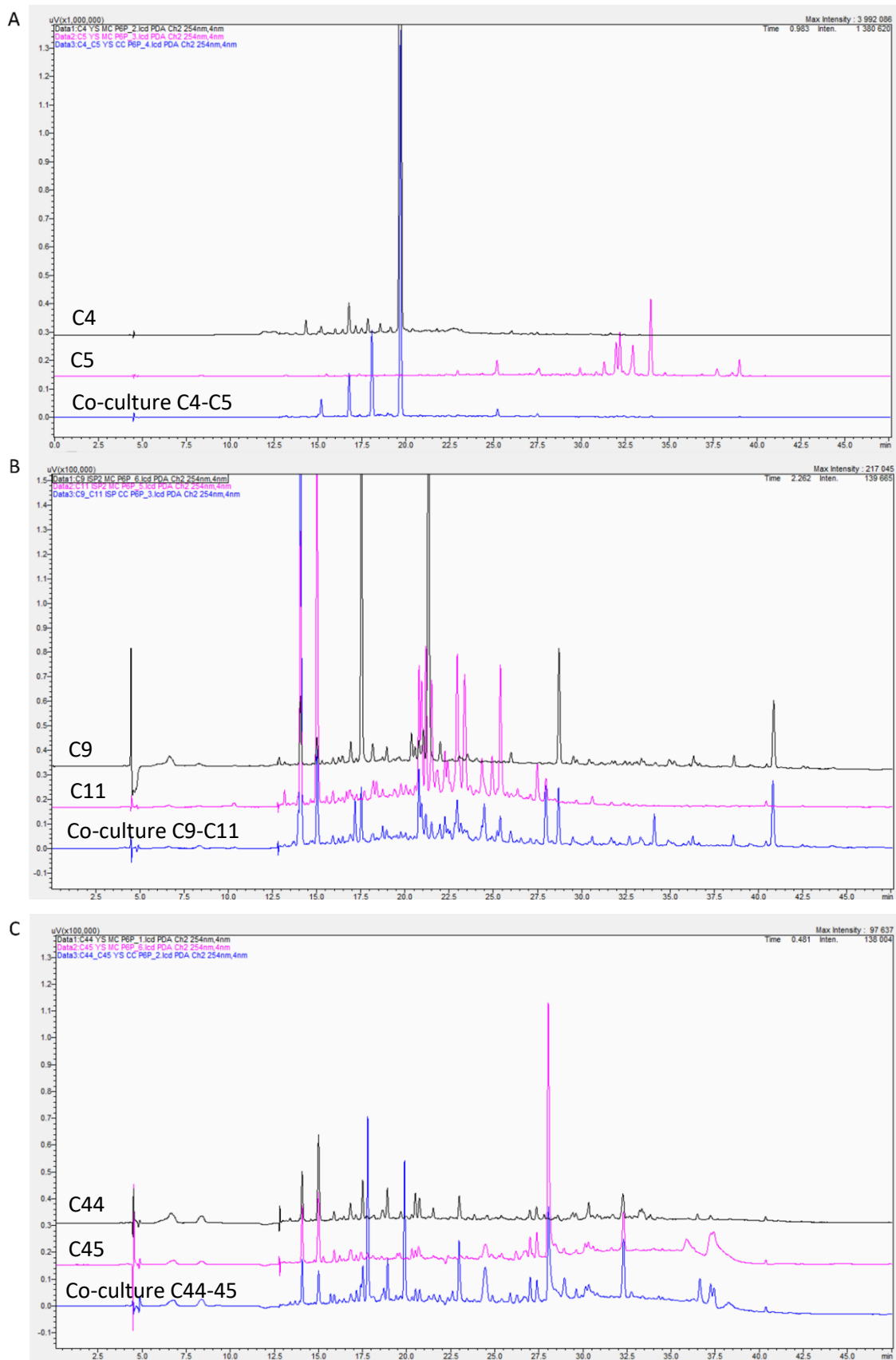
Figure 11 Comparaison des chromatogrammes obtenus par HPLC-DAD analytique (observation à \lambda 254 nm) entre les mono- et co-cultures en plaque 6 puits pour A) C4-C5 sur le milieu YS ; B) C9-C11 sur le milieu ISP2 et C) C44-C45 sur milieu YS.
