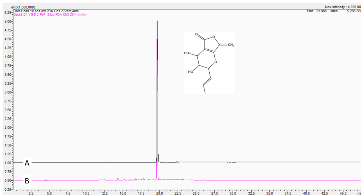
Figure 27 Comparaison des chromatogrammes pour le composé 8 . A) Massarilactone H ( 8 ) et B) chromatogramme de l'extrait de monoculture de C4
