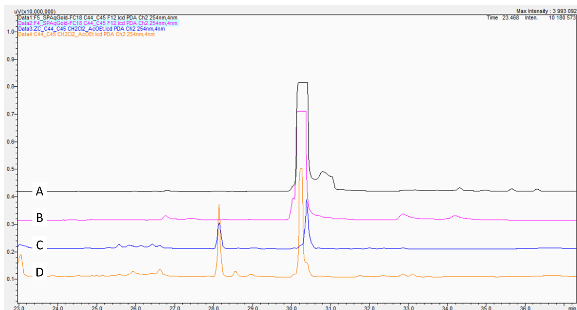
Figure 35 Chromatogrammes UV, \lambda à 254 nm : A) sous fraction F12-e ; B) sous-fraction F12-d ; C) extrait brut de la zone de confrontation de la troisième série de co-culture C44-C45 et D) extrait brut total de la troisième série
