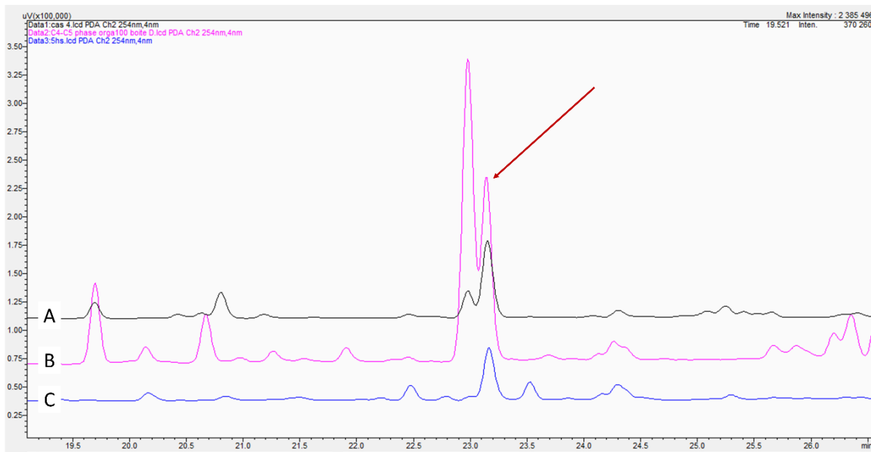
Figure 18 Chromatogrammes obtenus par HPLC analytique (observation à \lambda 254 nm) A) fraction F4; B) fraction D de l'extrait MeOH:CH 2 Cl 2 :AcOEt 1:2:3 + 0.1% d'AF de la série 2 et C) fraction Hs5 de l'extrait hexanique de la troisième série
