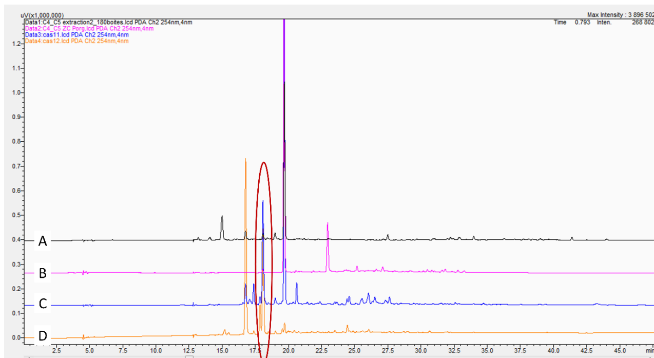
Figure 19 Comparaison des chromatogrammes : A) extrait CH 2 Cl 2 :AcOEt (v:v) de la co-culture C-C5 ; B) extrait CH 2 Cl 2 :AcOEt (v:v) de la zone de confrontation de la co-culture de C4-C5 ; C) fraction F11 et D) fraction F12
