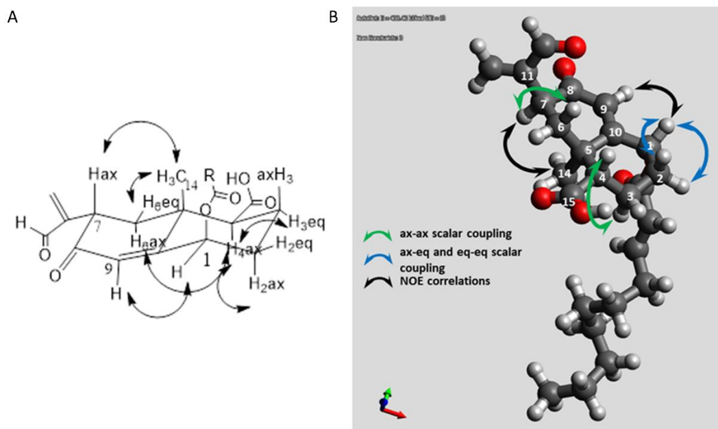
Figure 25 Conformation chaise du motif éremophilane et corrélations NOESY ; la Figure B représentant la structure 3D du composé 3 a été réalisée par le logiciel Avogadro 1.2 ( http://avogadro.cc/ )
