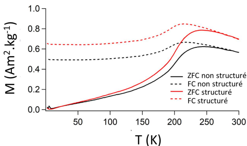
Figure III.30 : Mesures de magnétométrie SQUID Zero Field Cooled-Field Cooled (ZFC-FC) sous un champ magnétique statique de 50 Oe d'un échantillon \text{AzoCO}_2\text{Me} + \text{NP Fe}_3\text{O}_4 à 0,05 \text{ mol.L}^{-1} non structuré puis structuré à l'aide d'une lumière interférentielle polarisée p/p à 240 \text{ mW.cm}^{-2} pendant 1 h.
