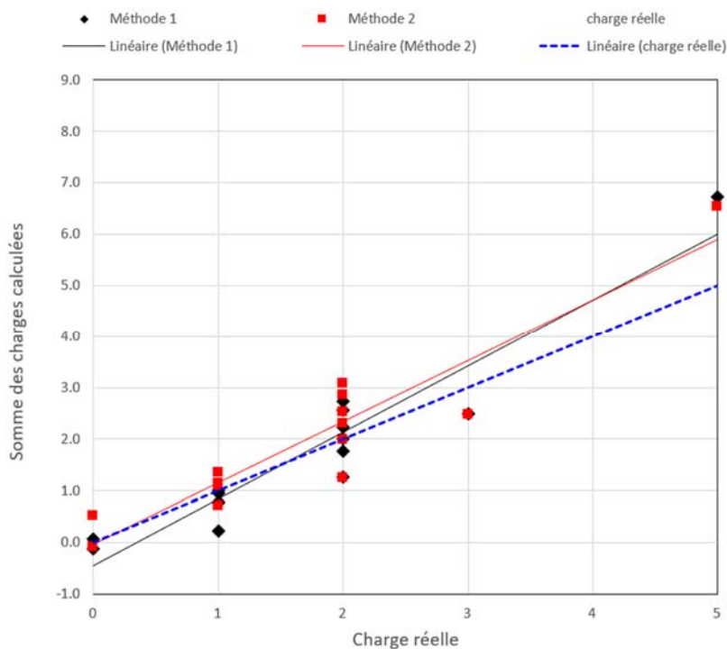
Figure II.5.5 : Somme totale des charges calculées pour selon la méthode 1 (noire) et 2 (rouge) à partir des quinze références du Tableau II.5.4 en fonction de la charge réelle de chaque sel (courbe de tendance en bleu).
