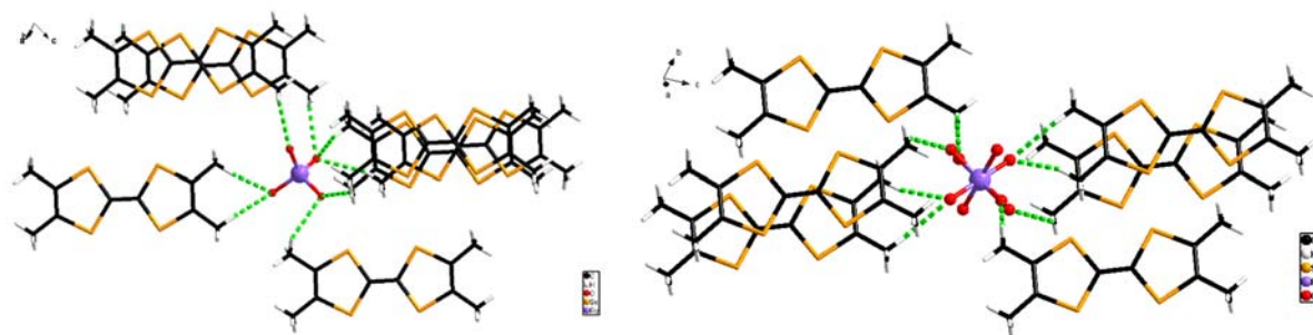
Figure II.4.13 : Liaisons hydrogène dans IT-(TMTSF) 2 ReO 4 avec des distances C-H...O à partir de 2.41 Å pour la structure IT à 150 K (gauche) et à partir de 2.57 Å pour la structure HT (droite).
