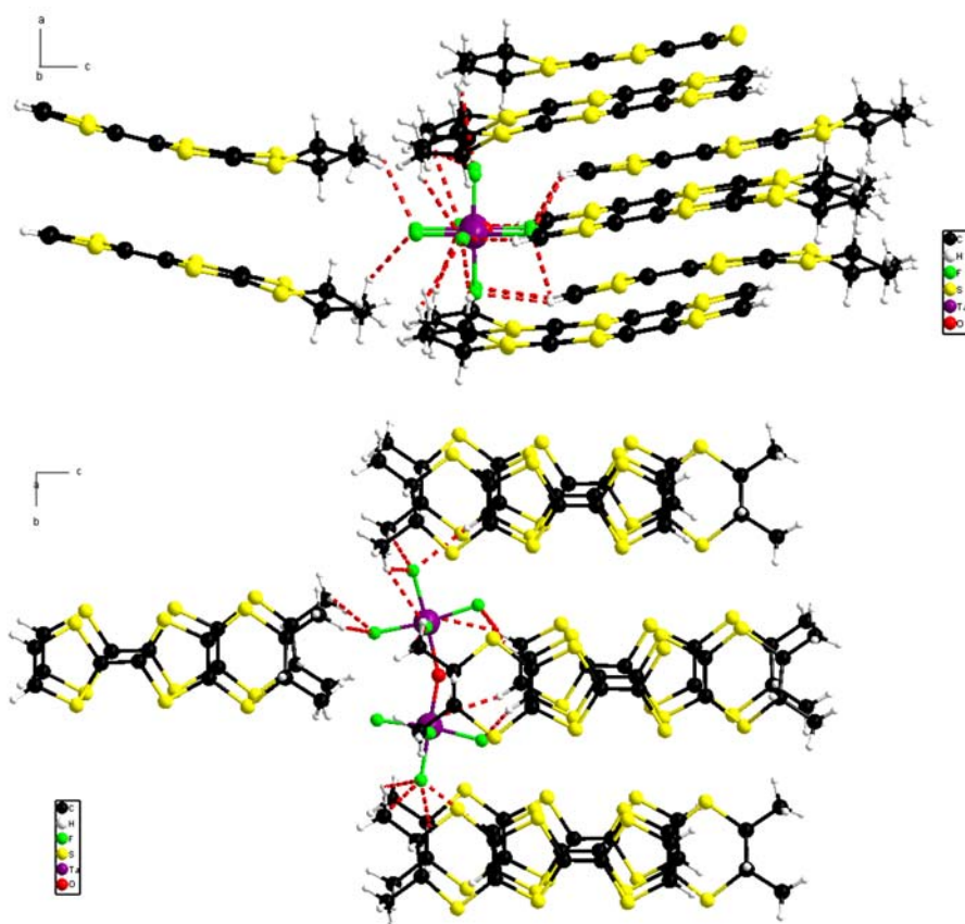
Figure II.1.20: Liaisons hydrogène dans [(S,S)\text{-DM-EDT-TTF}]_3\text{Ta}_2\text{F}_{10}\text{O} avec des distances C-H...F comprises entre 2.22 et 2.669Å
