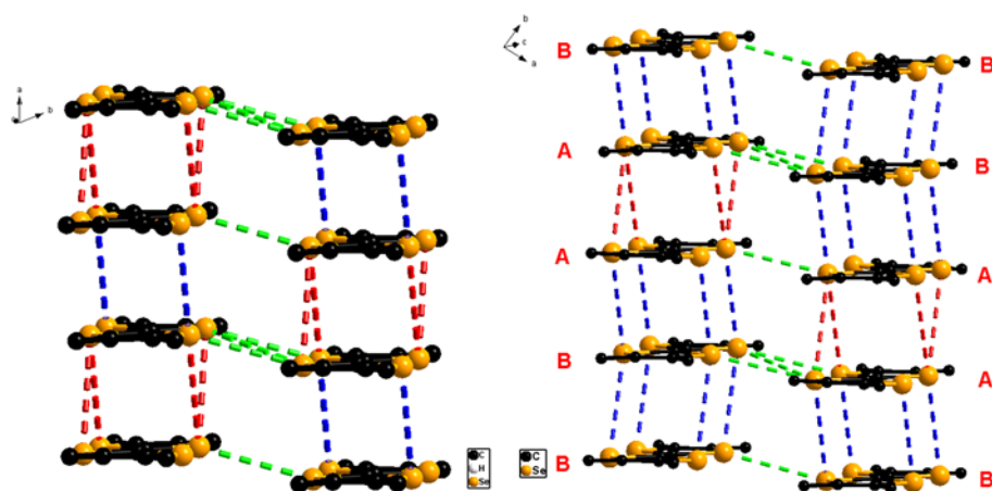
Figure II.4.10 : Empilement des donneurs dans la phase 1 (TMTSF) 2 ReO 4 enregistrée à 293 K (gauche) et à 150 K (droite) montrant les contacts Se...Se : en bleu, les contacts inférieurs à 3.90 Å; en rouge les contacts supérieurs à 3.90 Å; en vert, les contacts transverses entre les TMTSF (voir Tableau II.4.13) pour les distances de contacts.
