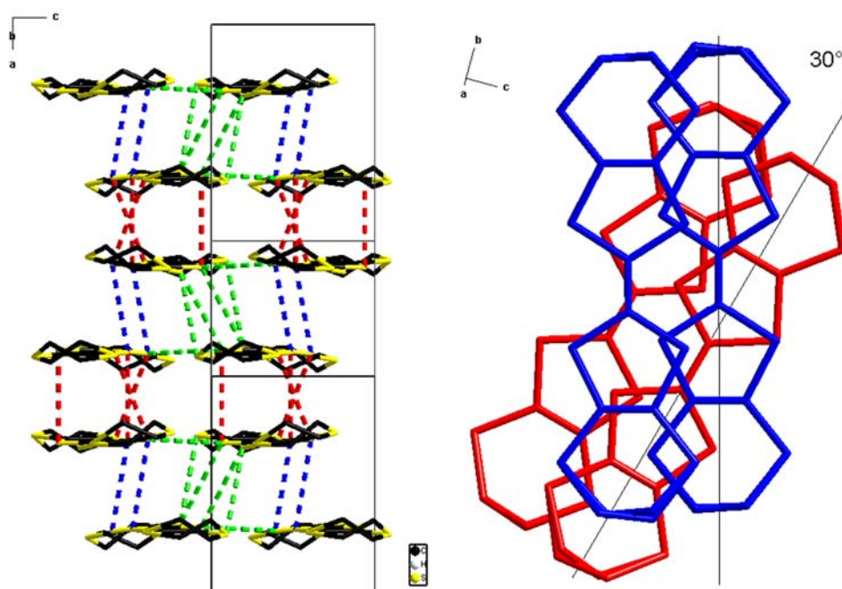
Figure II.2.7 : Empilement des donneurs dans \delta_{o^-} -(BEDT-TTF) 2 (TaF 6 ) 0.43 (PF 6 ) 0.57 montrant les contacts S...S entre les BEDT-TTF : en bleu, les contacts intra-dimères (3.724(1) Å) ; en rouge les contacts inter-dimères selon a (3.825-3.836 Å) ; en vert, les contacts entre donneurs selon c (3.826-3.855 Å)
