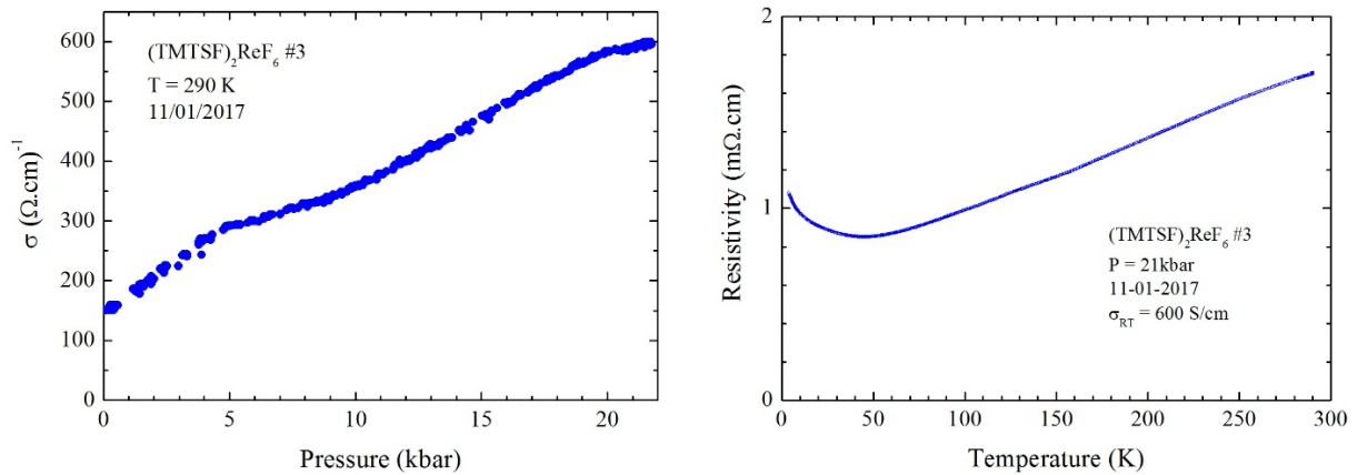
Figure II.3.10 : (gauche) Conductivité à température ambiante en fonction de la pression et (droite) résistivité électrique \rho en fonction de la température d'un 3 ème échantillon de (\text{TMTSF})_2\text{ReF}_6 (enduit d'huile)
