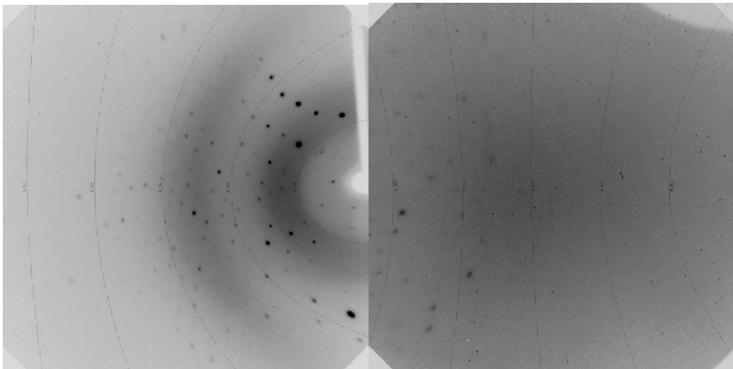
Figure I.3.1 : (gauche) Images de diffraction à bas angle \theta à 100 secondes d'exposition par image (diffraction visible jusqu'à environ 1.40 \text{ \AA} ) ; (droite) Image de diffraction à haut angle \theta à 400 secondes d'exposition par image d'une cage diffraction visible jusqu'à environ 1.04 \text{ \AA} )
