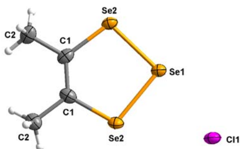
Figure II.6.2 : Vues ORTEP (ellipsoïdes dessinées à 50% de probabilité) avec numérotation atomique (sauf H) de C_4H_6Se_3,Cl .
