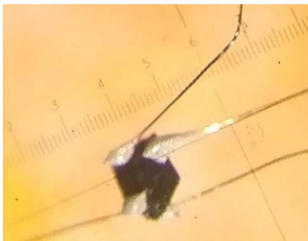
Figure II.1.16: Résistivité électrique en fonction de la température (haut) avec \log \rho versus T (gauche) et avec \log \rho versus 1/T (droite) pour un monocristal de (\text{BEDT-TTF})_3\text{Ta}_2\text{F}_{10}\text{O} . La ligne rouge est la régression linéaire donnant l'énergie d'activation à partir de la loi \rho = \rho_0 \exp(E_a/T) déterminée entre 135 et 300 K. (bas) Vue du cristal utilisé pour mesurer la résistivité dans le plan avec les 4 points de contacts.
