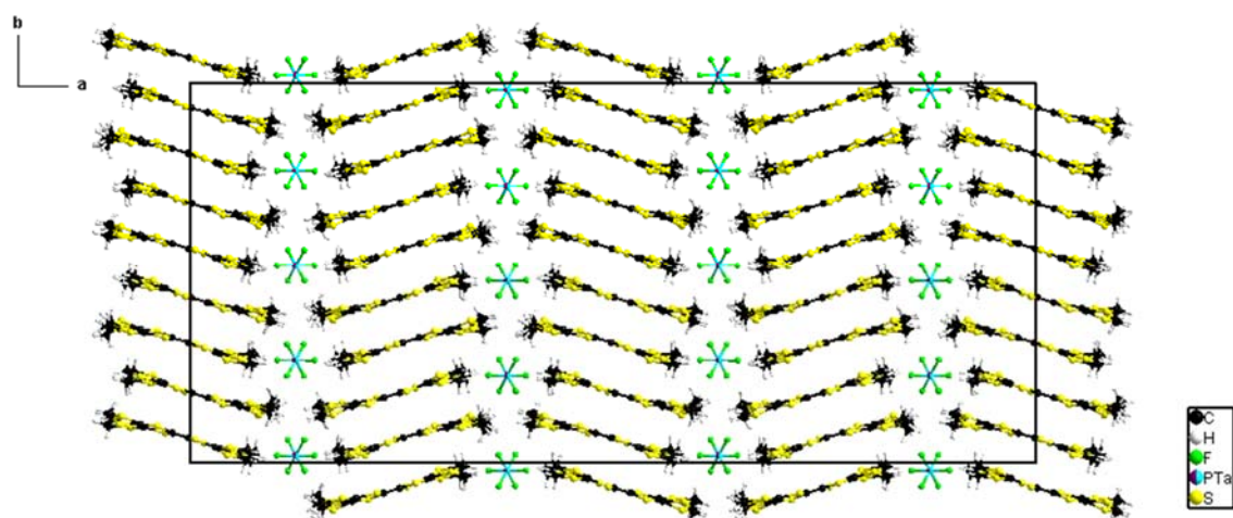
Figure II.2.19 : Empilement des donneurs dans (\text{BEDT-TTF})_4(\text{TaF}_6)_{0.86}(\text{PF}_6)_{1.14} selon c montrant la ségrégation entre les BEDT-TTF et les anions selon l'axe a
