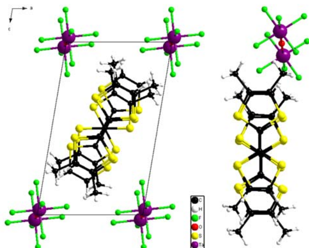
Figure II.1.23 : (gauche) Vue selon l'axe b de l'empilement des donneurs et la ségrégation organique-inorganique et (droite) vue décalée des donneurs dans un trimère de (o-DM-TTF) 3 Ta 2 F 10 O
