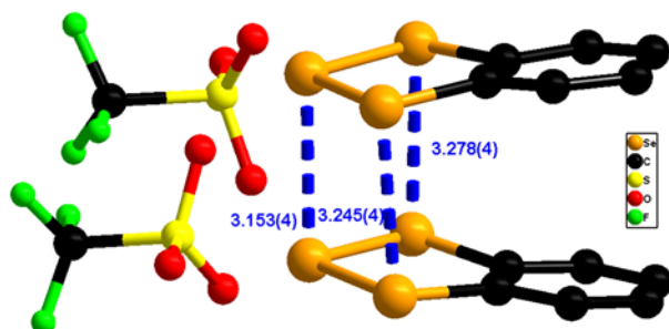
Figure II.6.1 : Empilements des dimères de C_6H_4Se_3,CF_3SO_3 montrant les contacts Se...Se
