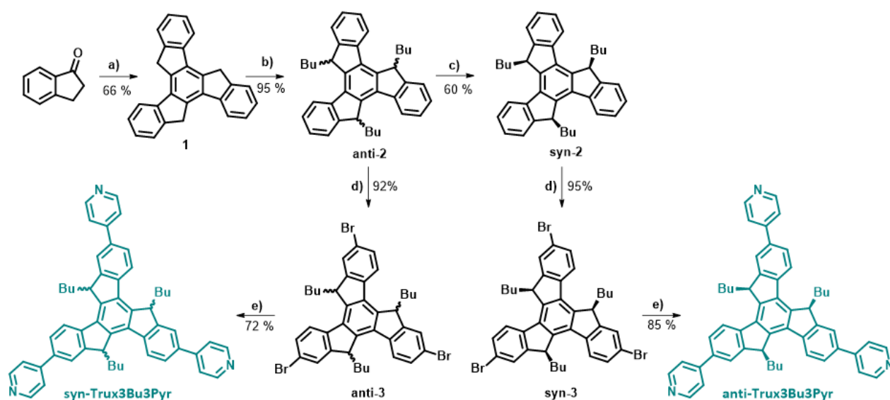
Schéma I.1.2 : Synthèse du truxène et du dérivé truxène. a) APTS.H 2 O, acide propanoïque, 1,2-dichlorobenzène, 20h, 105 °C ; b) n -BuLi, 1-bromobutane, THF, 18h, -78°C à t.a ; c) t -BuOK, t -BuOH, 1h, 90 °C ; d) Br 2 , dichlorométhane, une nuit, t.a ; e) Acide 4-pyridineboronique, Pd(PPh 3 ) 4 , K 2 CO 3 (aq), toluène, éthanol, 72 h, 90°C.
