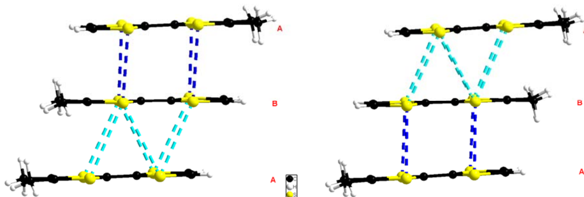
Figure II.1.24 : Empilement des donneurs dans (o\text{-DM-TTF})_3\text{Ta}_2\text{F}_{10}\text{O} montrant les contacts S...S entre les donneurs, le donneur B étant positionné dans un sens (gauche) ou dans l'autre (droite) : en bleu foncé, les contacts intra-trimère A-B (3.431-3.543 Å) ; en bleu clair, les contacts intra-trimère A-B avec le donneur désordonné opposé (3.697-3.847 Å)
