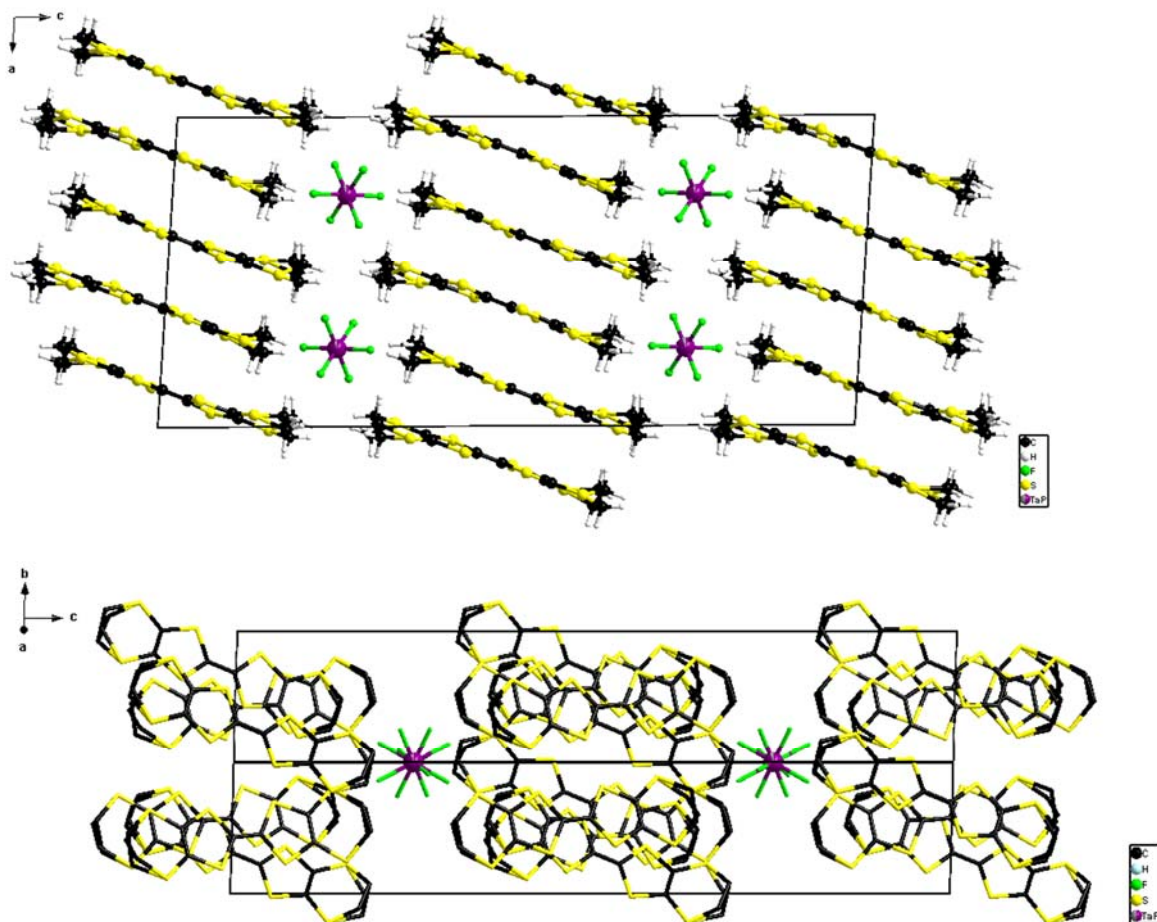
Figure II.2.9 : Empilement des donneurs selon b dans \delta_0 -(BEDT-TTF) _2 (TaF _6 ) _{0.94} (PF _6 ) _{0.06} selon b (haut) et selon (110) (bas) montrant la ségrégation entre les BEDT-TTF et les anions selon l'axe c
