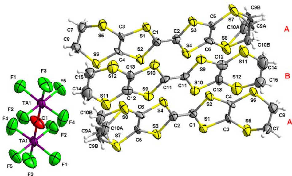
Figure II.1.12 : (gauche) Vue ORTEP (ellipsoïdes dessinées à 50% de probabilité) avec numérotation atomique (sauf H) dans (\text{BEDT-TTF})_3\text{Ta}_2\text{F}_{10}\text{O}
