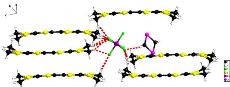
Figure II.2.14: Liaisons hydrogène dans (\text{BEDT-TTF})_2(\text{TaF}_6)_2 \cdot \text{CH}_2\text{Cl}_2 avec des distances \text{C-H} \dots \text{F} comprises entre 2.37 et 2.71 Å
