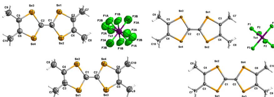
Figure II.2.1 : : Vues ORTEP (ellipsoïdes dessinées à 50% de probabilité) avec numérotation atomique (sauf H) de (TMTSF) 2 TaF 6 à 293 K (Gauche) et à 100 K (droite), montrant les anions TaF 6 - désordonnés et ordonnés respectivement.
