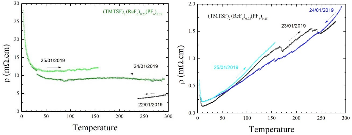
Figure II.3.18 : Résistivité électrique \rho à pression ambiante en fonction de la température T (K) de (TMTSF)_2(ReF_6)_{0.25}(PF_6)_{0.75} (gauche) et de (TMTSF)_2(ReF_6)_{0.75}(PF_6)_{0.25} (droite)
