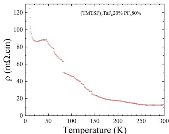
Figure II.2.5 : Résistivité électrique \rho à pression ambiante en fonction de la température T (K) de (\text{TMTSF})_2(\text{TaF}_6)_{0.2}(\text{PF}_6)_{0.8}
