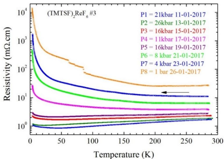
Figure II.3.11: Résistivité électrique en fonction de la pression et de la température avec \log \rho versus T sur le 3 ème échantillon de (\text{TMTSF})_2\text{ReF}_6 (enduit d'huile)
