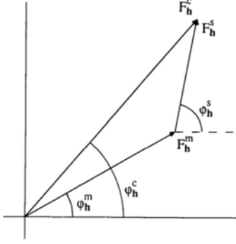
Figure.I.4.1 : Diagramme d'Argand montrant les facteurs de structure calculés F_h^c , utilisés dans l'affinement par moindres carrés contre les facteurs de structures observés |F_h^o|^2 , et étant égaux à la somme vectorielle de F_h^m (modèle principal) et F_h^s (solvant). F_h^s est déterminé de façon itérative en utilisant SQUEEZE avec F_h^m fixé, F_h^c égal à |F_h^o| avec la phase \varphi_h^c et en commençant avec \varphi_h^s = \varphi_h^m . (Figure issue de la référence [41])
