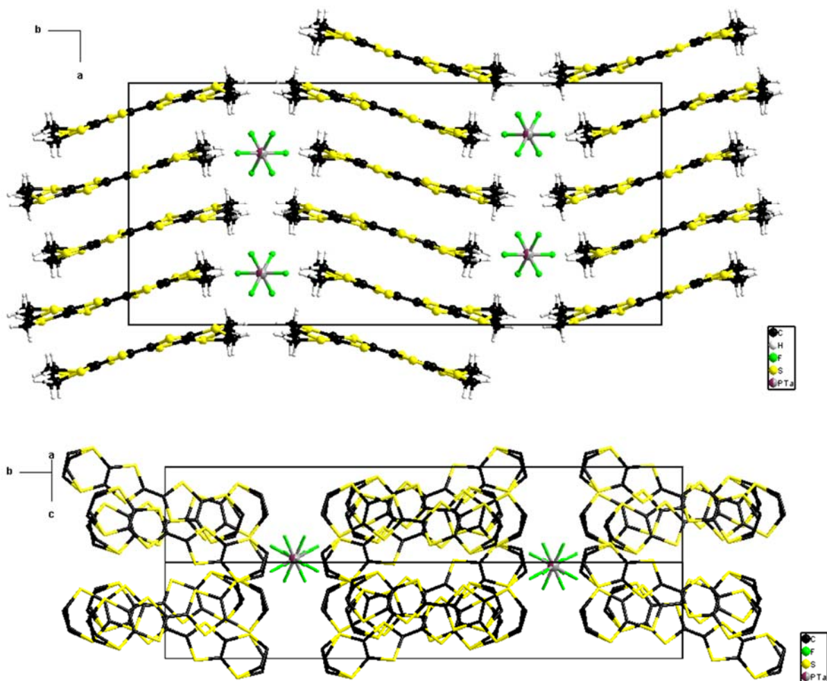
Figure II.2.8 : Empilement des donneurs dans \delta_o -(BEDT-TTF) _2 (TaF _6 ) _{0.43} (PF _6 ) _{0.57} selon c (haut) et selon (101) (bas) montrant la ségrégation entre les BEDT-TTF et les anions selon l'axe b
