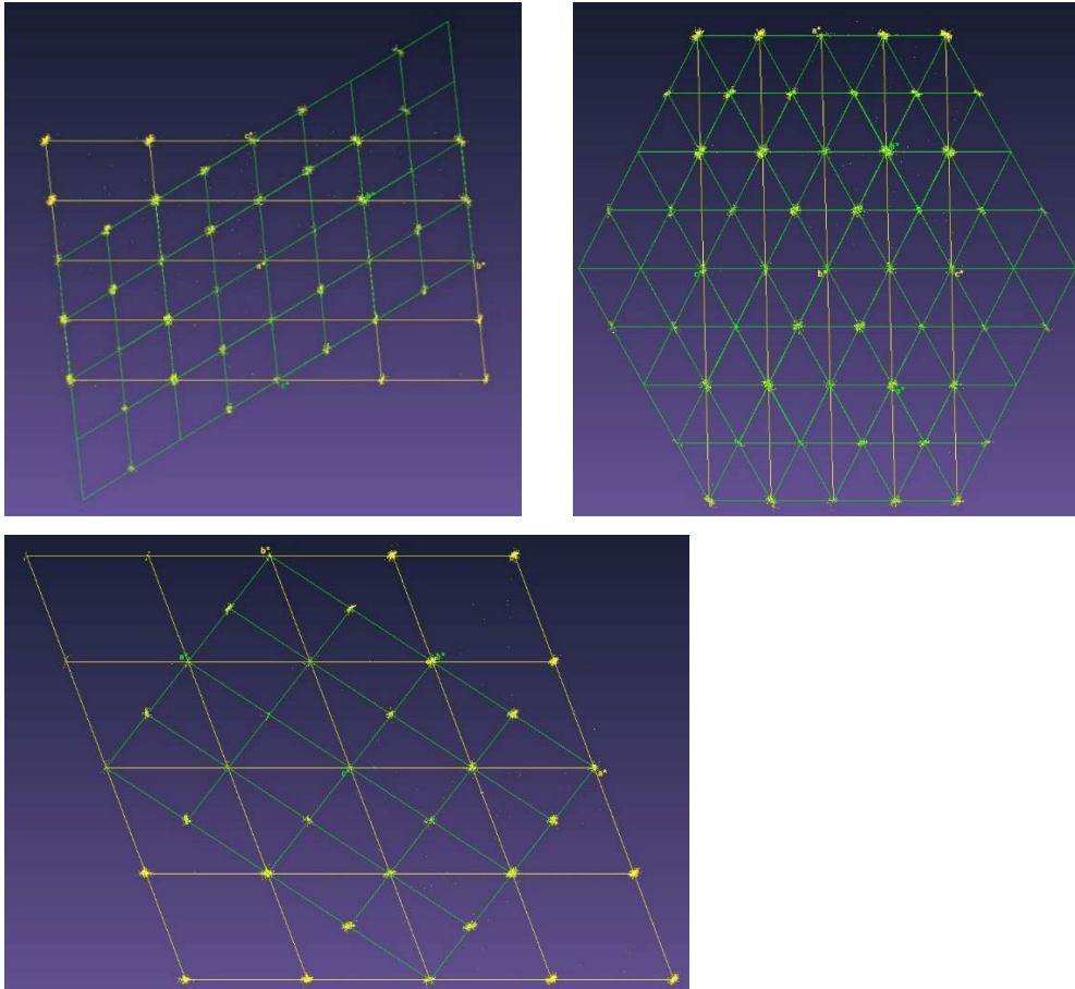
Figure II.4.8 : Clichés de diffraction (vue selon a^* (haut-gauche), selon b^* (haut-droite) et selon c^* (bas-gauche)) des nœuds du réseau réciproque de la phase IT-(TMTSF) 2 ReO 4 avec indication des mailles HT (en jaune) et IT (en vert).
