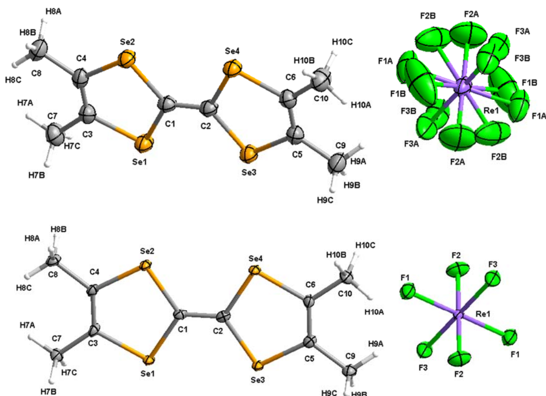
Figure II.3.5 : Vues ORTEP (ellipsoïdes dessinées à 50% de probabilité) avec numérotation atomique de (TMTSF) 2 ReF 6 à 293 K (haut) et à 100 K (bas)
