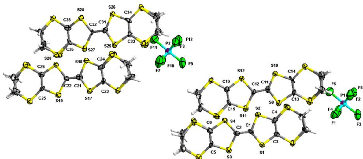
Figure II.2.18 : Vue ORTEP (ellipsoïdes dessinées à 50% de probabilité) avec numérotation atomique partiel (sauf H) de (\text{BEDT-TTF})_4(\text{TaF}_6)_{0.86}(\text{PF}_6)_{1.14} à 200 K
