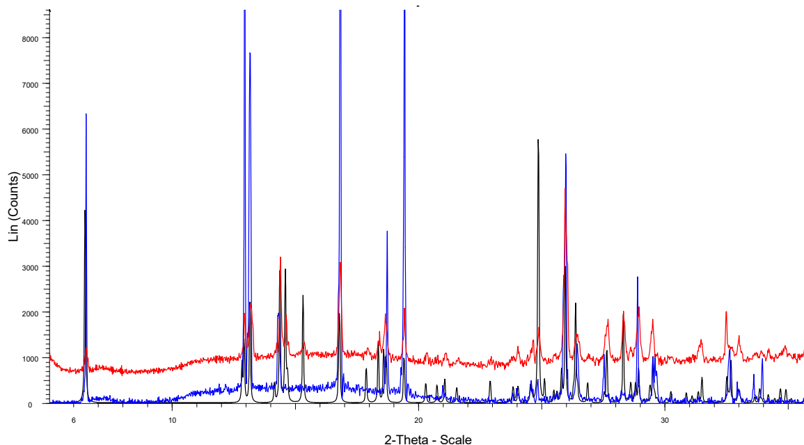
Figure II.3.13 : Diagrammes de poudre des cristaux non broyés de (\text{TMTSF})_2\text{ReF}_6 à 293 K avant (courbe bleue) et après le refroidissement à 100 K (courbe rouge). En noir, le diagramme simulé à partir d'une structure résolue sur monocristal de (\text{TMTSF})_2\text{ReF}_6 à 293 K
