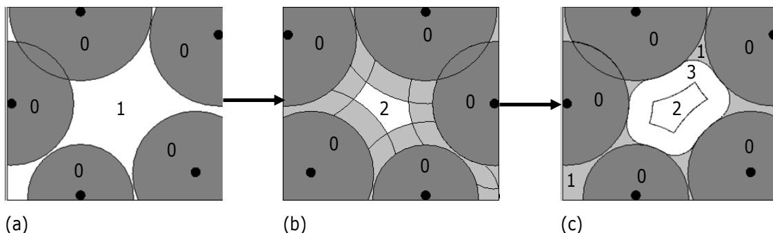
Figure I.4.2 : procédure schématisée de la détermination de l'aire du solvant accessible
