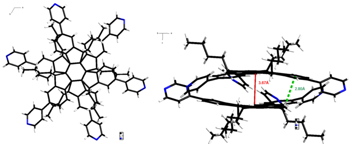
Figure I.5.3 : (gauche) Vue éclipée selon l'axe c entre deux molécules et (droit) distance entre deux molécules dimérisées (rouge) et interaction C-H... \pi (vert) de syn -Trux3Bu3Pyr
