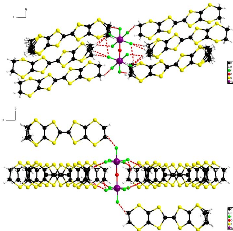
Figure II.1.15: Liaisons hydrogène dans (\text{BEDT-TTF})_3\text{Ta}_2\text{F}_{10}\text{O} avec des distances C-H...F comprises entre 2.14 et 2.63 Å
