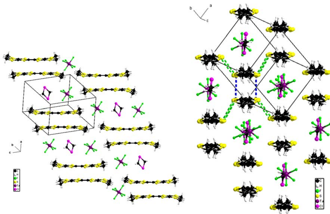
Figure II.2.13 : Vues de l'empilement des donneurs et des anions/molécules de solvant dans (\text{BEDT-TTF})_2(\text{TaF}_6)_2 \cdot \text{CH}_2\text{Cl}_2 pour deux colonnes d'empilement consécutives selon c (gauche) et une feuille de colonnes dans le plan (ab) (droite) montrant les contacts \text{S} \dots \text{S} intra dimère (bleu) et latéralement entre les dimères (vert).
