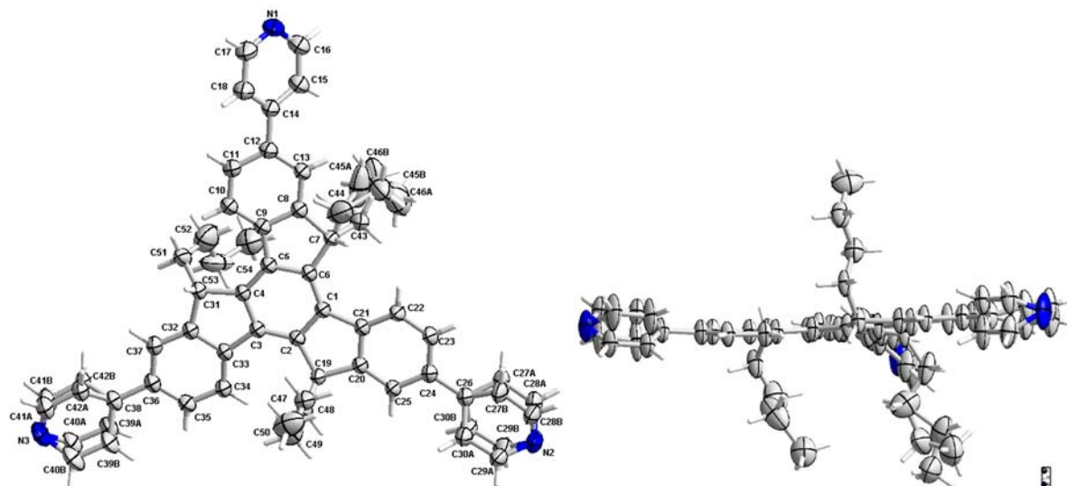
Figure I.5.5 : (gauche) Vue ORTEP de dessus avec numérotation atomique (sauf H) et (droite) vue de profil d' anti -Trux3Bu3Pyr (ellipses dessinées avec une probabilité de 50%).
