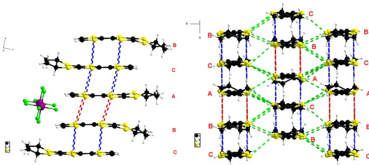
Figure II.1.19 : Empilement des donneurs dans [(S,S)-DM-EDT-TTF] 3 Ta 2 F 10 O montrant les contacts S...S dans et entre les donneurs : en bleu, les contacts intra-trimère (3.538-3.631 Å) ; en rouge les contacts inter-trimères selon a (3.748-3.817 Å) ; en vert, les contacts inter-trimères selon b (3.64-4.04 Å)
