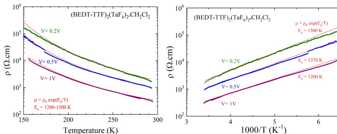
Figure II.2.17: Résistivité électrique en fonction de la température pour le monocristal #3 de (\text{BEDT-TTF})_2(\text{TaF}_6)_2 \cdot \text{CH}_2\text{Cl}_2 avec \log \rho versus T (gauche) et \log \rho versus 1/T (droite), mesurée avec différentes tensions : 0.2, 0.5 et 1V. La ligne rouge est la régression linéaire donnant l'énergie d'activation à partir de la loi \rho = \rho_0 \exp(E_a/T) déterminée entre 150 K et 295 K.
