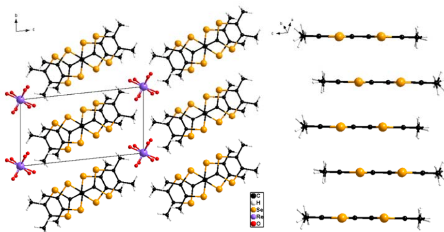
Figure II.4.12 : (Haut) Empilement des donneurs de la phase monoclinique C2/c \mu'' - (TMTSF)_2ReO_4 et (bas) Empilement des donneurs de la phase triclinique P-1 (TMTSF)_2ReO_4 montrant leur différence d'orientation selon l'axe c .
