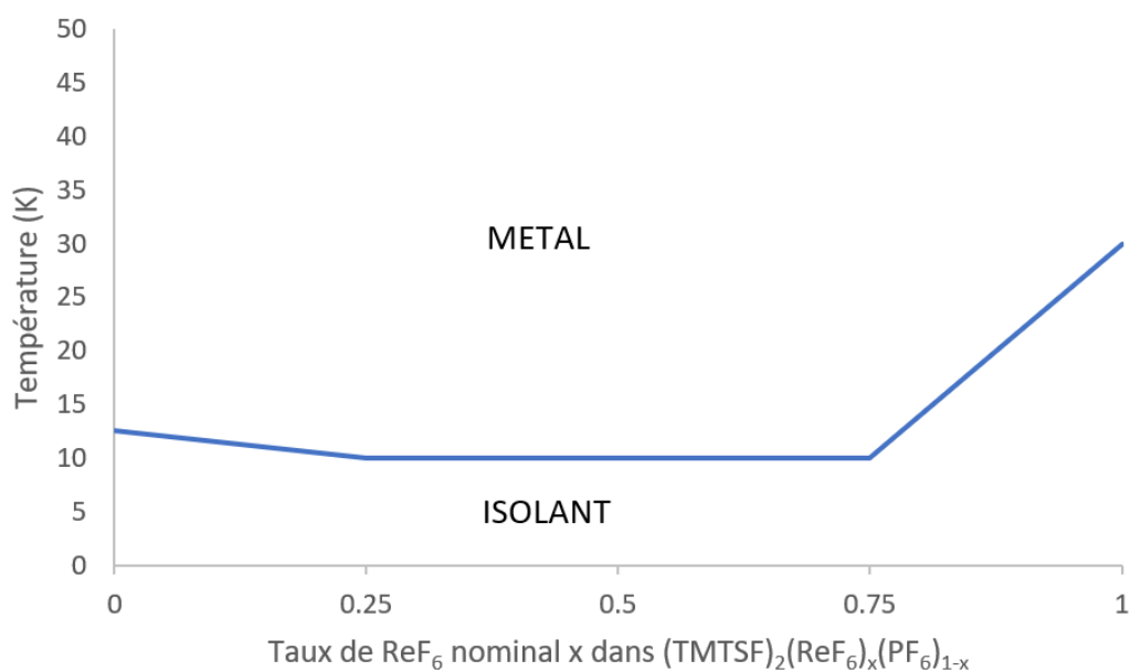
Figure II.3.20 : Diagramme de phase montrant l'état conducteur des alliages (\text{TMTSF})_2(\text{ReF}_6)_x(\text{PF}_6)_{1-x} en fonction de la température à pression ambiante
