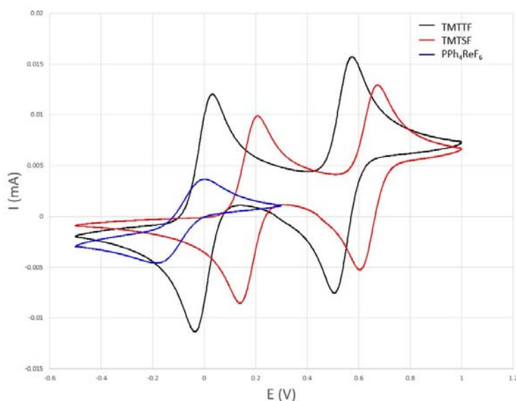
Figure II.3.4 : Voltammogrammes de TMTTF (noir), TMTSF (rouge) et (PPh_4)Re^VF_6 (bleu) (ref Ag/AgNO_3 , n-Bu_4NPF_6 0.1M dans le dichlorométhane, 0.1 V/s) à T_{ambiante}
