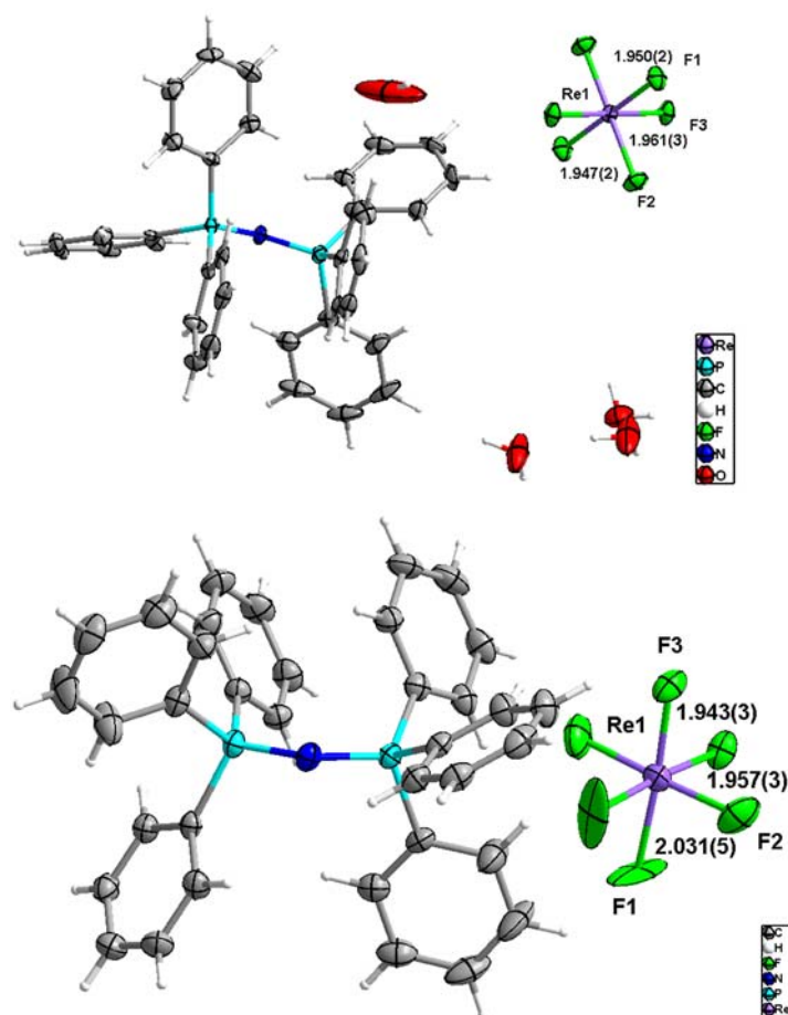
Figure II.3.1 : (haut) Vue ORTEP (ellipsoïdes dessinées à 50% de probabilité) avec numérotation atomique des anions et distances de liaisons Re-F de (Ph_3-PPN-Ph_3)_2ReF_6 \cdot 6(H_2O) et (bas) de (Ph_3-PPN-Ph_3)_2ReF_6
