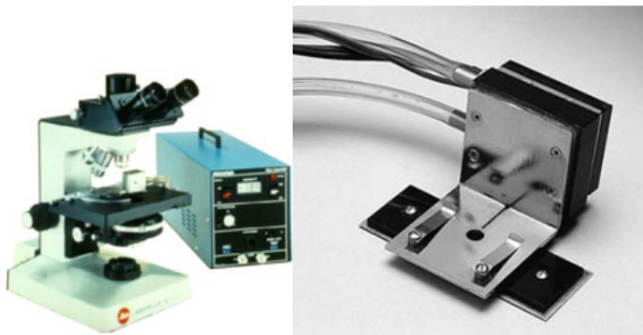
Figure I.2.4 : Platine thermique pour microscope (-20°C - +100°C) 23
