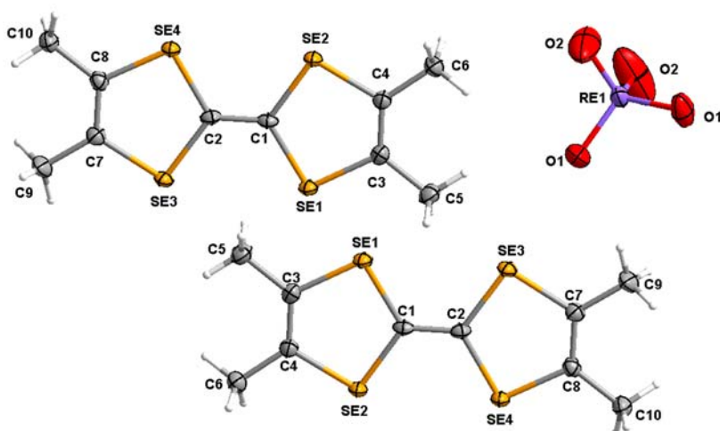
Figure II.4.11 : Vue ORTEP (ellipsoïdes dessinées à 50% de probabilité) avec numérotation atomique (sauf H) de la phase \mu''\text{-(TMTSF)}_2\text{ReO}_4 à 150K.
