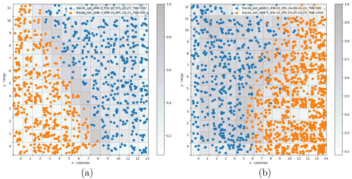
Figure E.2 – Résultat du partitionnement pour les jeux C (a) et D (b), présenté en E.1, et composés de deux classes. Le fond de la figure présente la U-matrix
