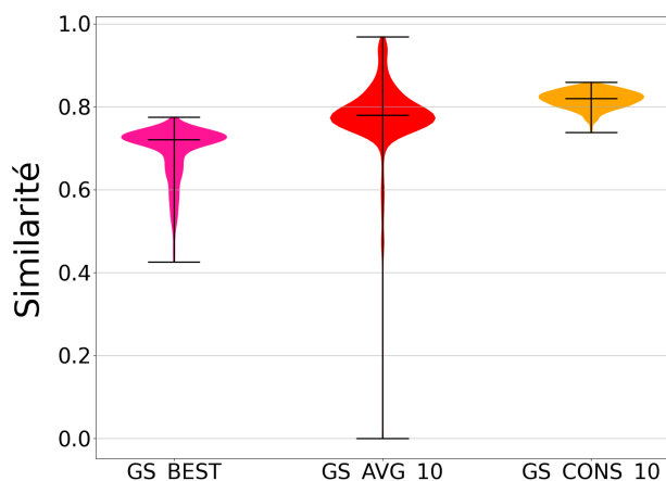
Figure 5.6 – Distribution des similarités entre séquence simulée et séquence réelle, pour les trois stratégies. Chaque violon décrit la distribution de la mesure de similarité Sim_k entre les séries temporelles multivariées réelles et simulées, pour les 1000 patients réels du jeu de données, pour une stratégie k donnée. Les barres supérieures et inférieures donnent l'étendue de la distribution, la barre centrale indique la médiane
